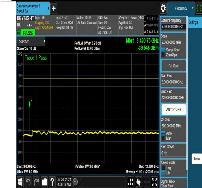
NTNV-N66-PC3-15-10-L-DFT-QPSK-Edge_1RB_Left-3000-1200 0-Ant1-PASS
