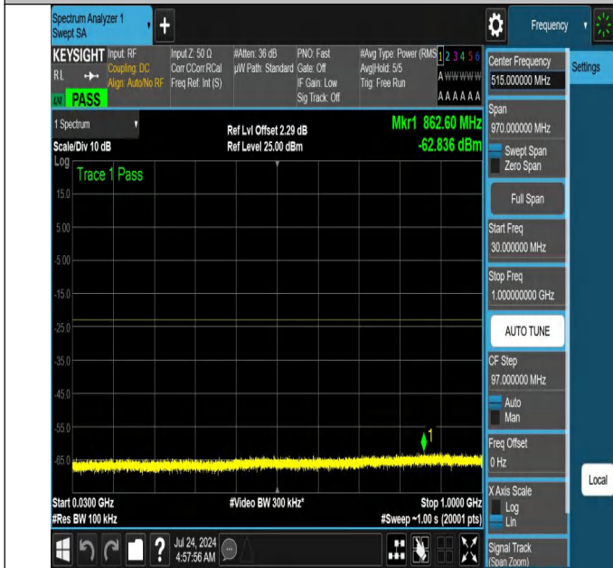
NTNV-N66-PC3-15-10-L-DFT-QPSK-Edge_1RB_Left-30-1000-Ant1-PASS
