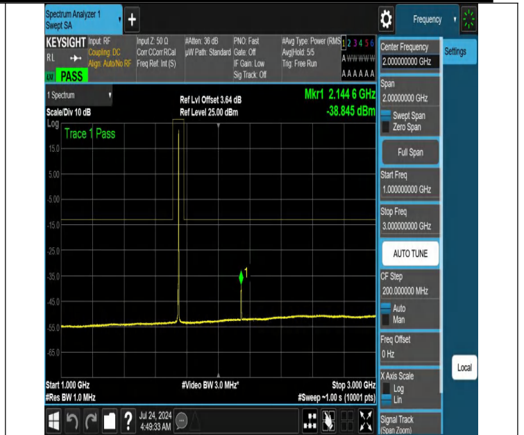
NTNV-N66-PC3-15-5-M-DFT-QPSK-Edge_1RB_Right-1000-3000-Ant1-PASS
