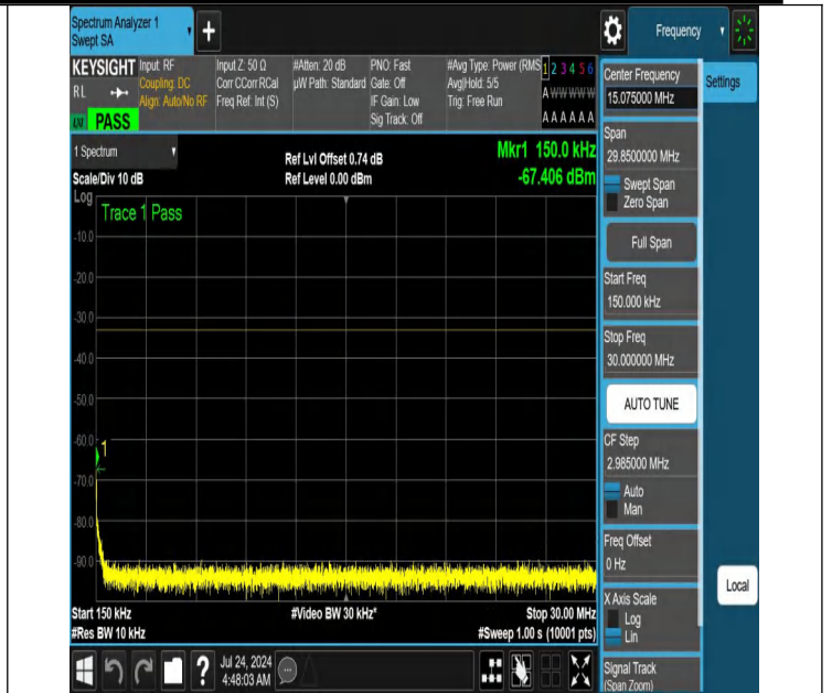
NTNV-N66-PC3-15-5-M-DFT-QPSK-Edge_1RB_Left-0.15-30-Ant1-PASS
