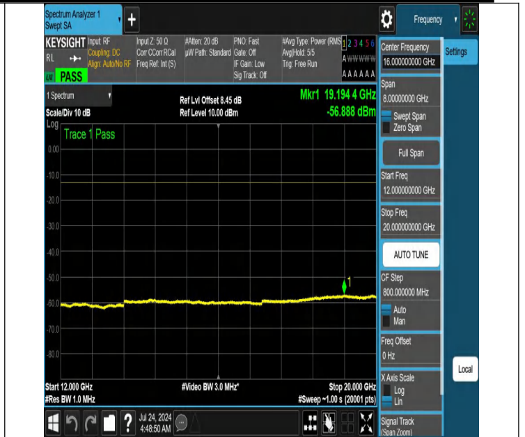
NTNV-N66-PC3-15-5-M-DFT-QPSK-Edge_1RB_Left-12000-2000 0-Ant1-PASS
