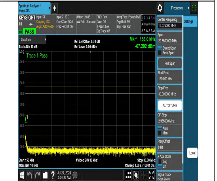
NTNV-N66-PC3-15-10-M-DFT-PI2BPSK-Edge_1RB_Right-0.15-3 0-Ant1-PASS
