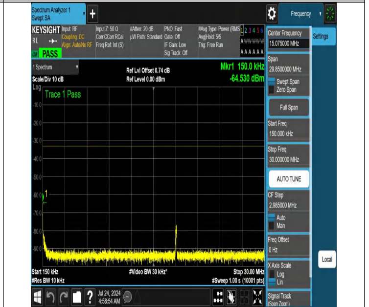
NTNV-N66-PC3-15-10-L-DFT-QPSK-Edge_1RB_Right-0.15-30-A nt1-PASS
