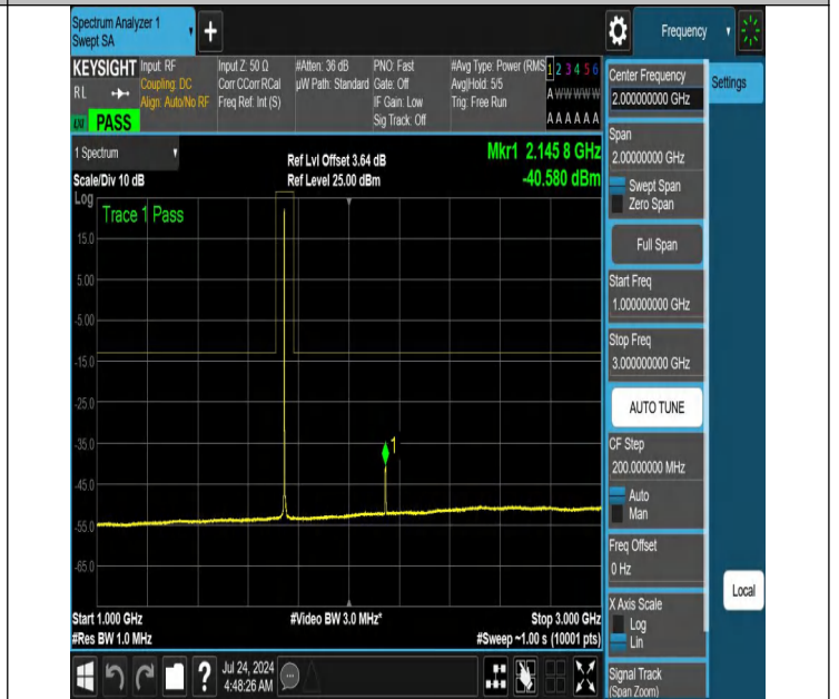
NTNV-N66-PC3-15-5-M-DFT-QPSK-Edge_1RB_Left-1000-3000-Ant1-PASS
