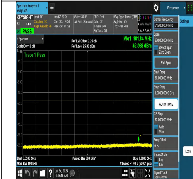
NTNV-N66-PC3-15-5-M-DFT-QPSK-Edge_1RB_Left-30-1000-Ant1-PASS
