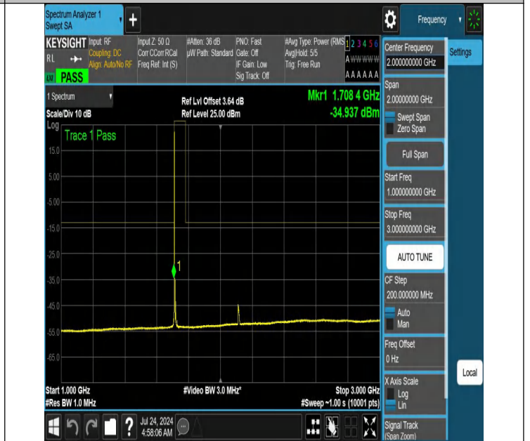
NTNV-N66-PC3-15-10-L-DFT-QPSK-Edge_1RB_Left-1000-3000-Ant1-PASS
