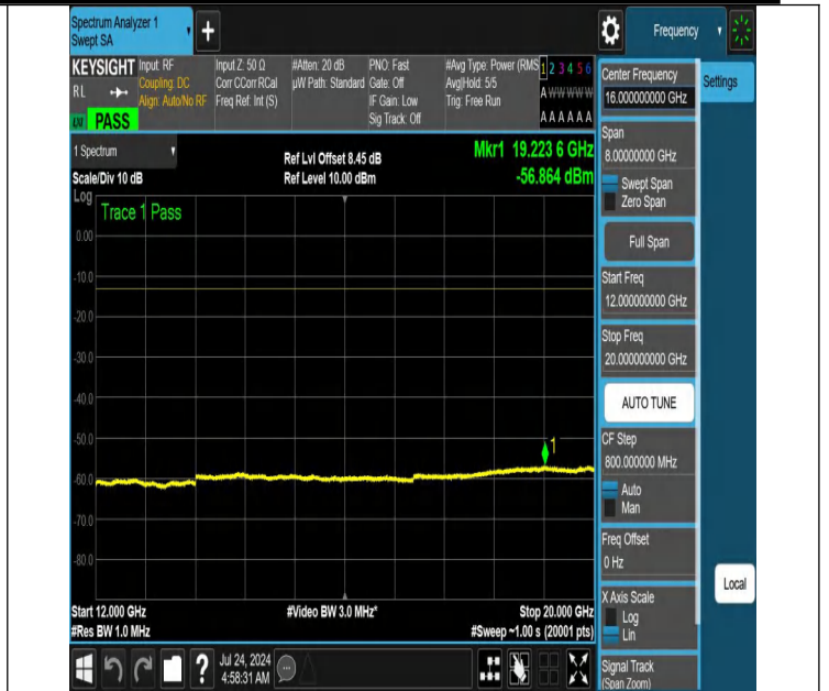
NTNV-N66-PC3-15-10-L-DFT-QPSK-Edge_1RB_Left-12000-2000 0-Ant1-PASS
