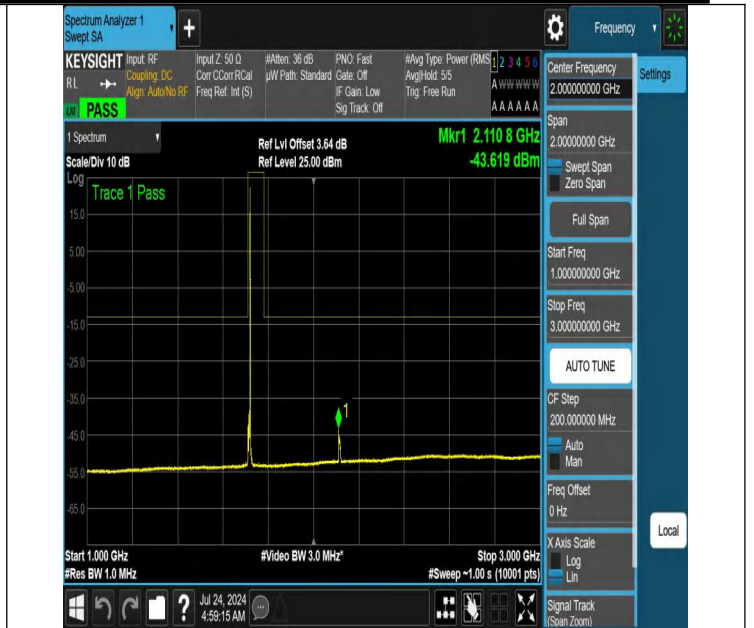
NTNV-N66-PC3-15-10-L-DFT-QPSK-Edge_1RB_Right-1000-3000-Ant1-PASS
