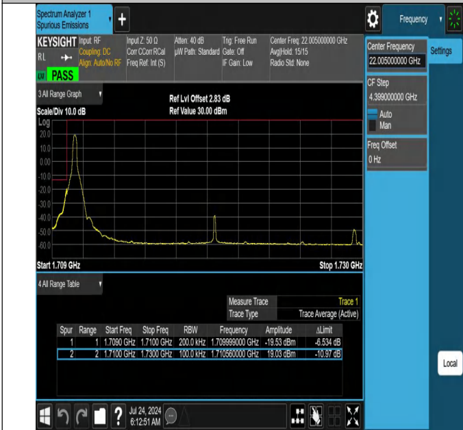
NTNV-N66-PC3-15-20-L-DFT-QPSK-Edge_1RB_Left-Ant1-PAS S
