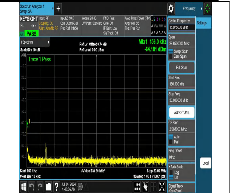
NTNV-N66-PC3-15-5-L-DFT-QPSK-Edge_1RB_Left-0.15-30-Ant1-PASS
