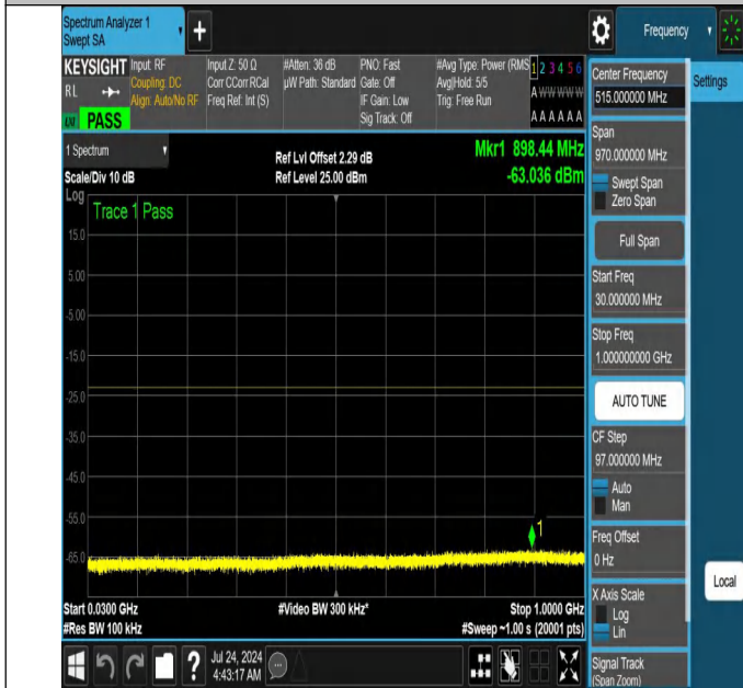
NTNV-N66-PC3-15-5-L-DFT-QPSK-Edge_1RB_Left-30-1000-Ant1-PASS
