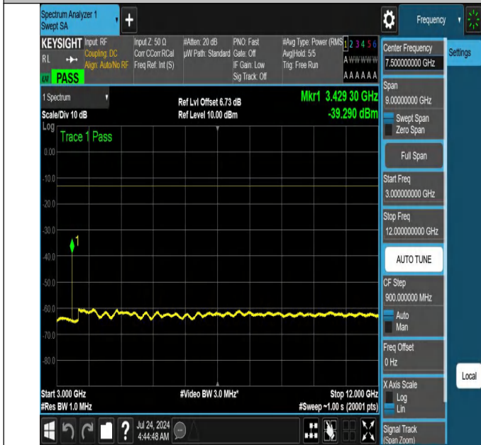
NTNV-N66-PC3-15-5-L-DFT-QPSK-Edge_1RB_Right-3000-1200 0-Ant1-PASS
