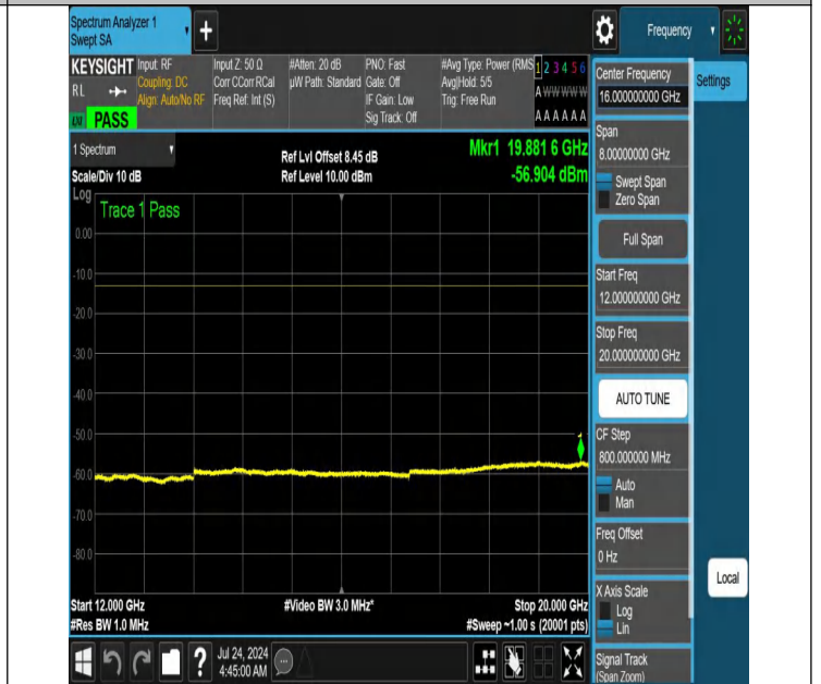
NTNV-N66-PC3-15-5-L-DFT-QPSK-Edge_1RB_Right-12000-2000 0-Ant1-PASS
