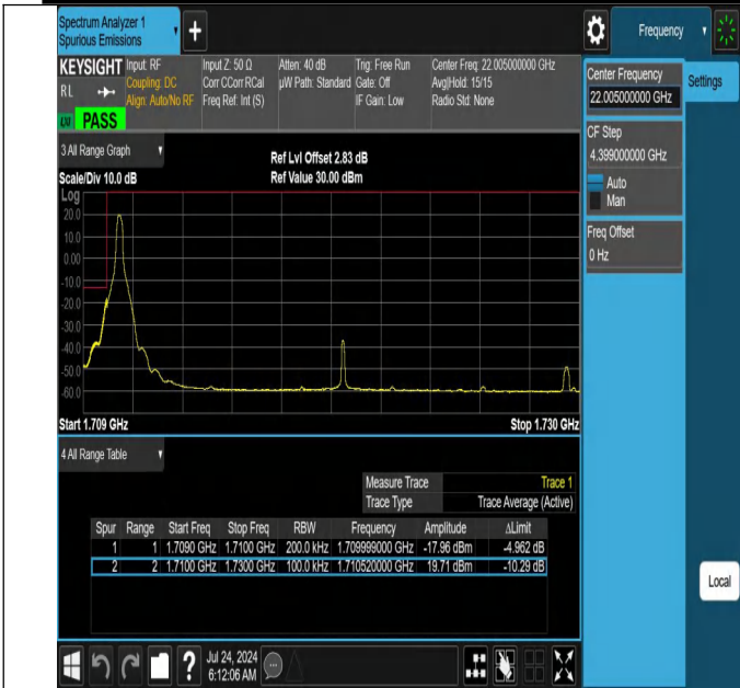
NTNV-N66-PC3-15-20-L-DFT-PI2BPSK-Edge_1RB_Left-Ant1-P ASS
