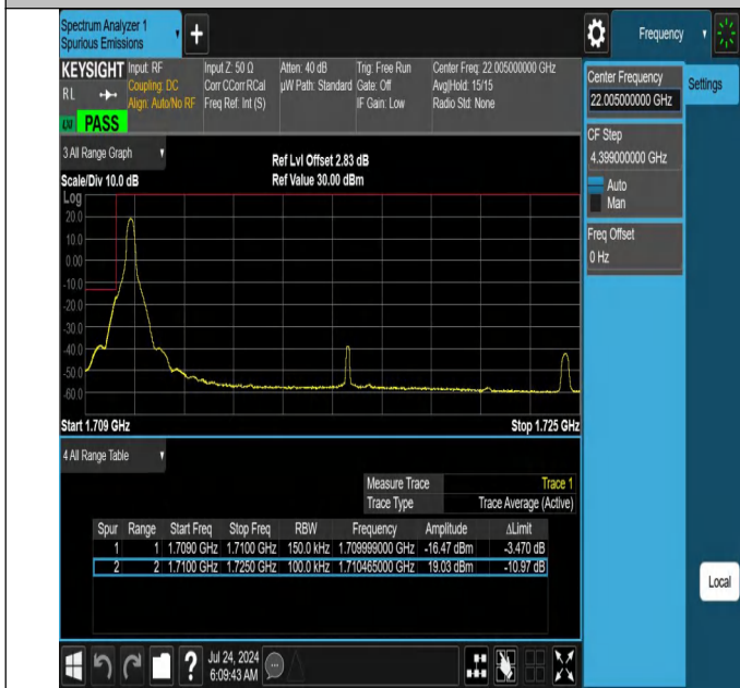
NTNV-N66-PC3-15-15-L-DFT-QPSK-Edge_1RB_Left-Ant1-PAS S
