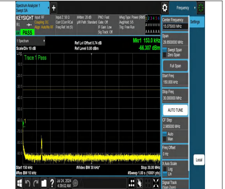
NTNV-N66-PC3-15-5-L-DFT-PI2BPSK-Edge_1RB_Left-0.15-30-A nt1-PASS
