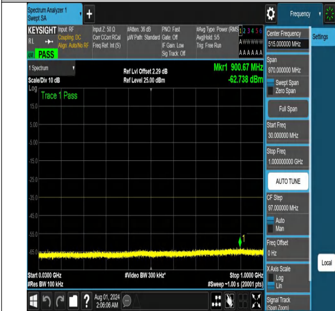
NTNV-N41-PC2-30-60-H-DFT-QPSK-Edge_1RB_Left-30-1000-A nt1-PASS
