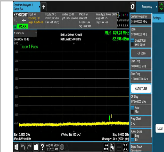
NTNV-N41-PC2-30-60-M-DFT-QPSK-Edge_1RB_Left-30-1000-A nt1-PASS
