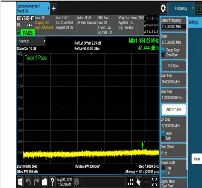
NTNV-N41-PC2-30-60-L-DFT-QPSK-Edge_1RB_Left-30-1000-A nt1-PASS
