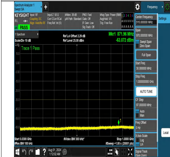
NTNV-N41-PC2-30-20-H-DFT-QPSK-Edge_1RB_Left-30-1000-A nt1-PASS
