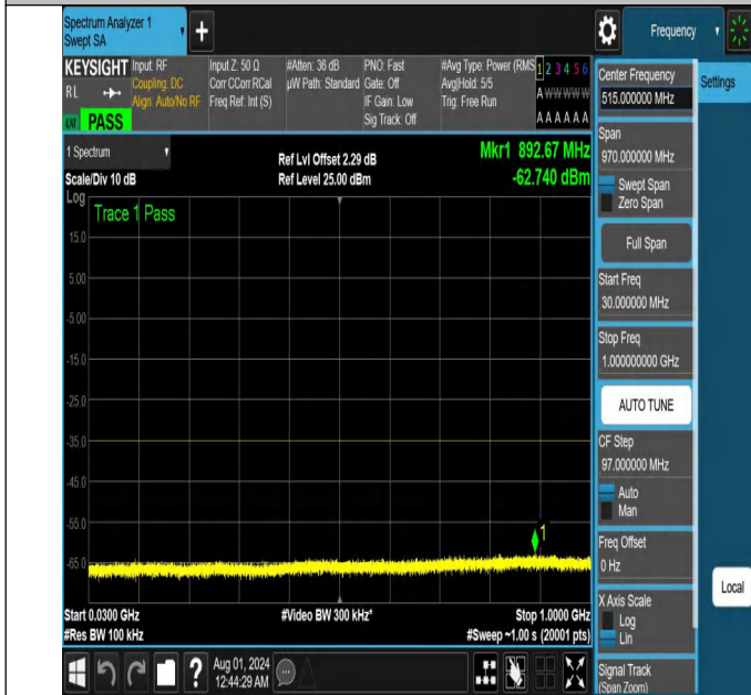
NTNV-N41-PC2-30-10-H-DFT-QPSK-Edge_1RB_Left-30-1000-A nt1-PASS
