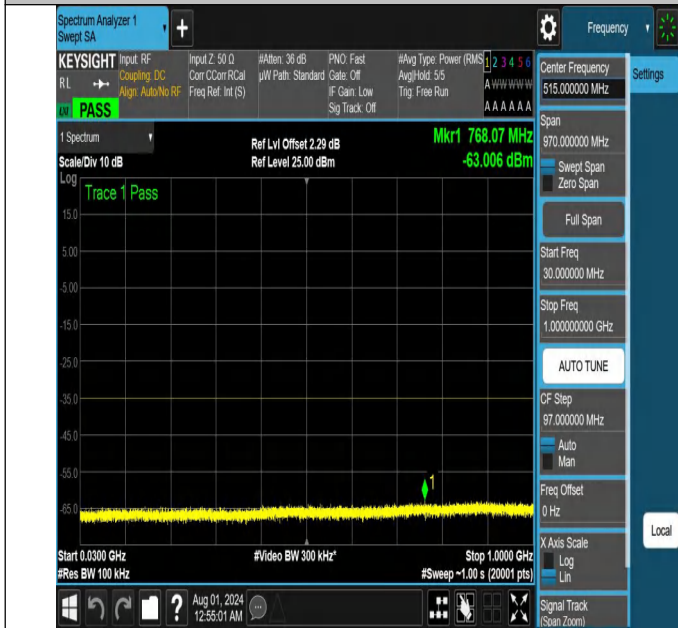
NTNV-N41-PC2-30-15-M-DFT-QPSK-Edge_1RB_Left-30-1000-A nt1-PASS
