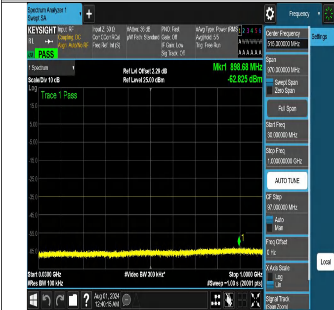
NTNV-N41-PC2-30-10-M-DFT-QPSK-Edge_1RB_Left-30-1000-A nt1-PASS
