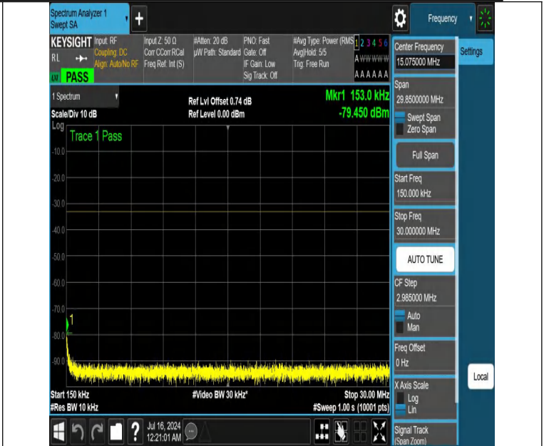
NTNV-DC_12A_n25A-PC3-15-5+30-M+L-N/A-N/A-DFT-QPSK-Edge _1RB_Left-0.15-30-PASS
