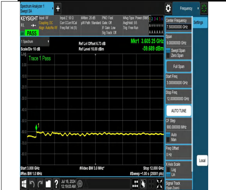
NTNV-DC_12A_n25A-PC3-15-5+30-M+L-N/A-N/A-DFT-PI2BPSK-Edge_1RB_Left-3000-12000-PASS
