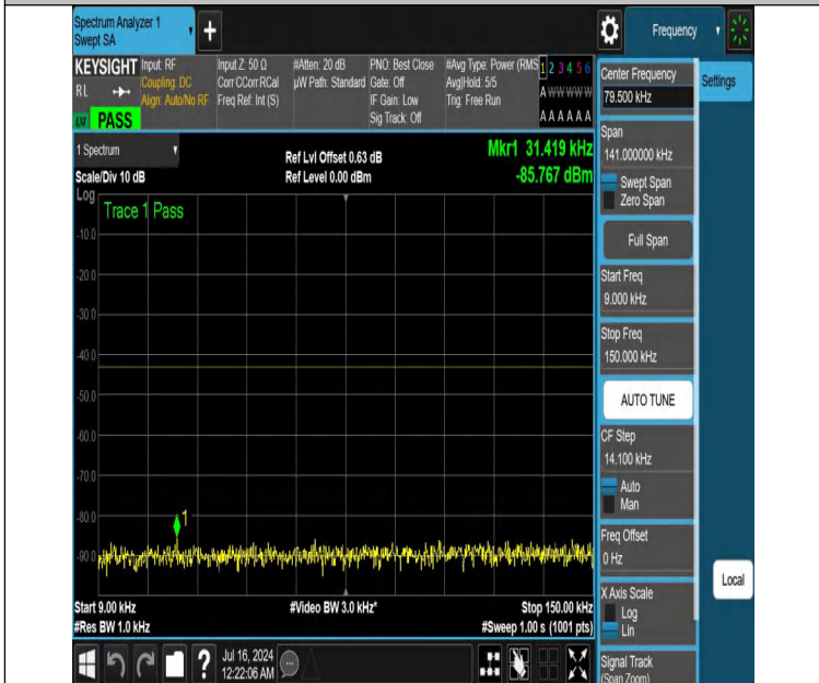
NTNV-DC_12A_n25A-PC3-15-5+30-M+L-N/A-N/A-DFT-QPSK-Edge e_1RB_Right-0.009-0.15-PASS
