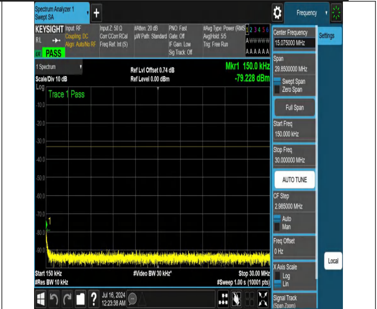
NTNV-DC_12A_n25A-PC3-15-5+30-M+M-N/A-N/A-DFT-PI2BPSK-E dge_1RB_Left-0.15-30-PASS
