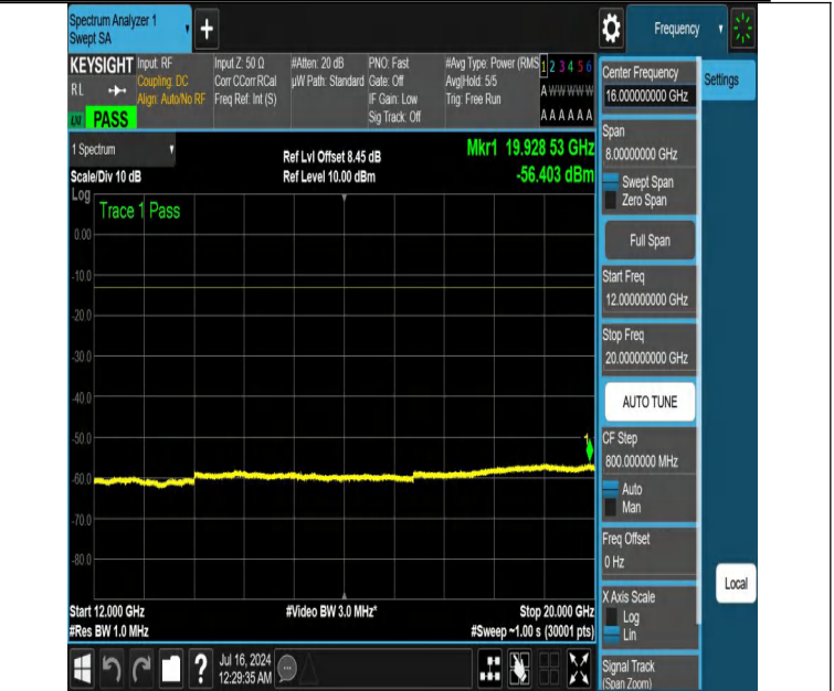
NTNV-DC_12A_n25A-PC3-15-5+30-M+H-N/A-N/A-DFT-PI2BPSK-E dge_1RB_Left-12000-20000-PASS
