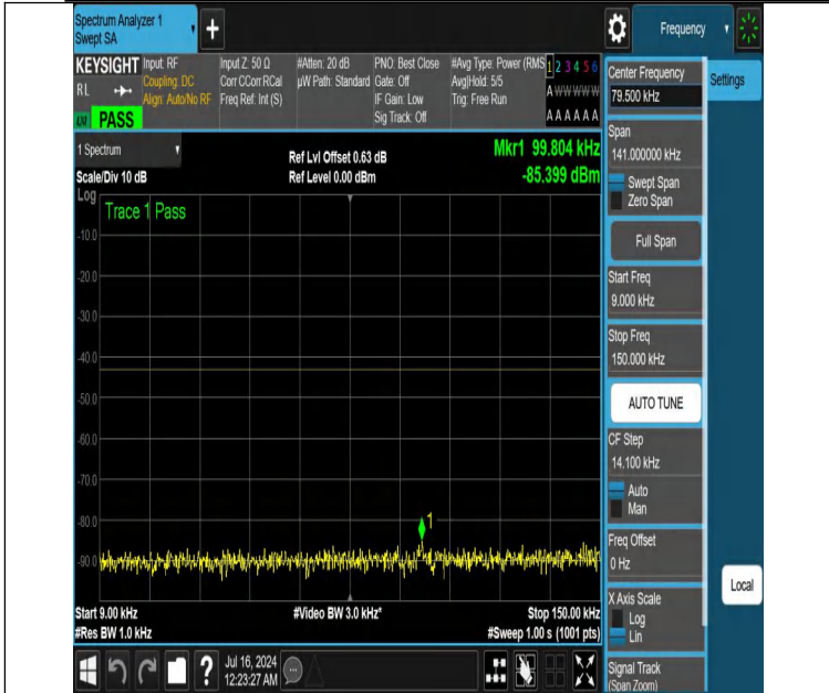
NTNV-DC_12A_n25A-PC3-15-5+30-M+M-N/A-N/A-DFT-PI2BPSK-Edge_1RB_Left-0.009-0.15-PASS
