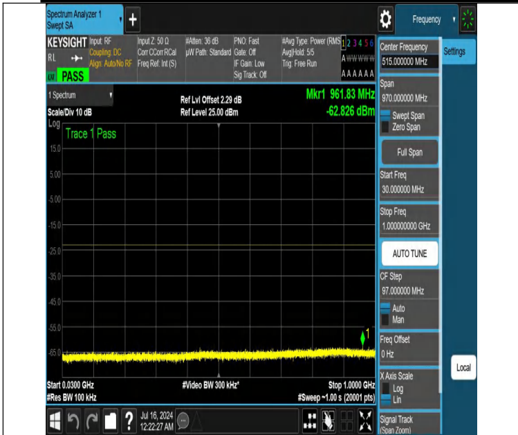
NTNV-DC_12A_n25A-PC3-15-5+30-M+L-N/A-N/A-DFT-QPSK-Edge e_1RB_Right-30-1000-PASS
