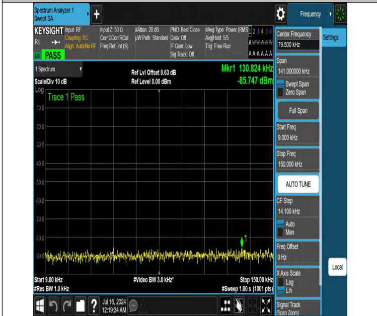
NTNV-DC_12A_n25A-PC3-15-5+30-M+L-N/A-N/A-DFT-PI2BPSK-Edge_1RB_Right-0.009-0.15-PASS
