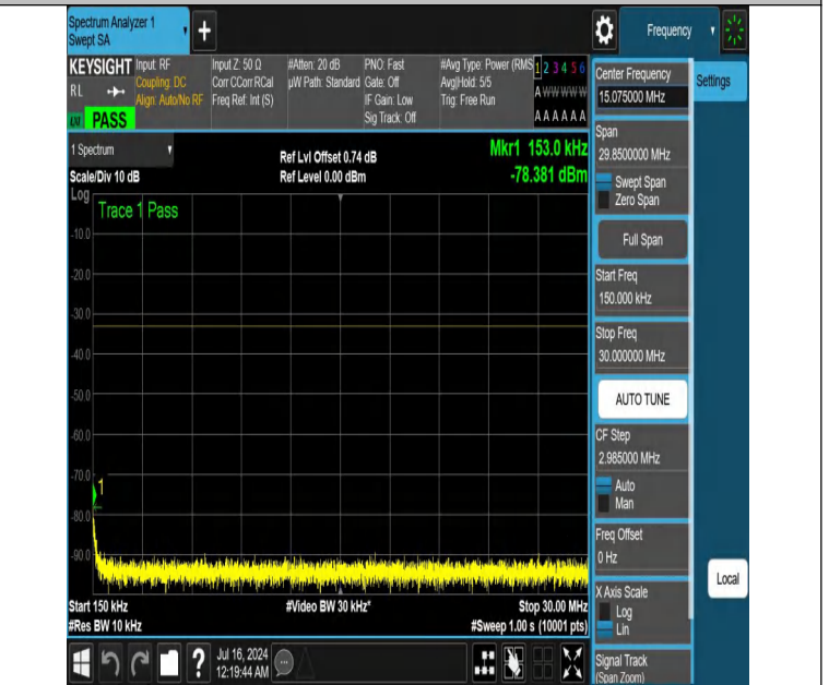
NTNV-DC_12A_n25A-PC3-15-5+30-M+L-N/A-N/A-DFT-PI2BPSK-E dge_1RB_Right-0.15-30-PASS
