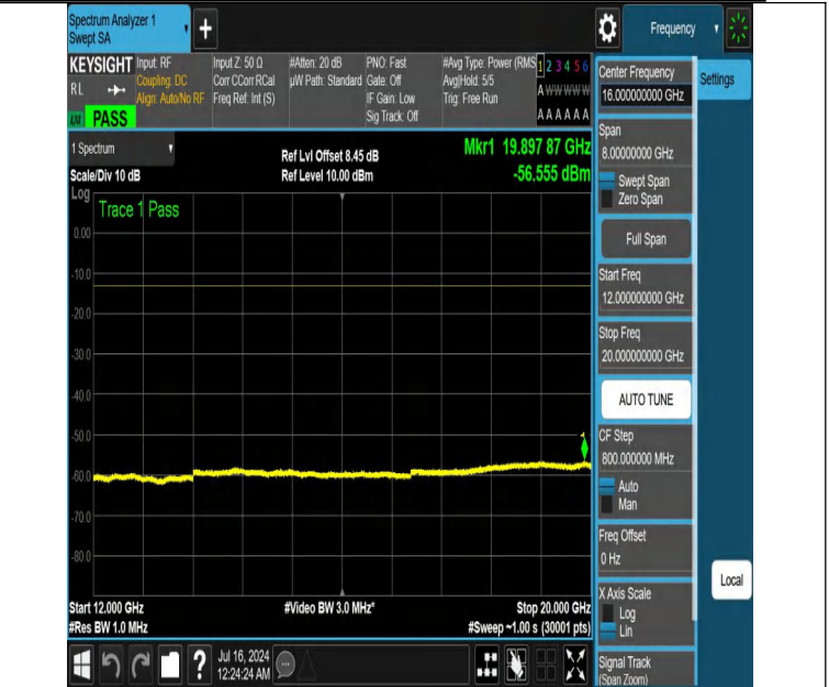
NTNV-DC_12A_n25A-PC3-15-5+30-M+M-N/A-N/A-DFT-PI2BPSK-E dge_1RB_Left-12000-20000-PASS
