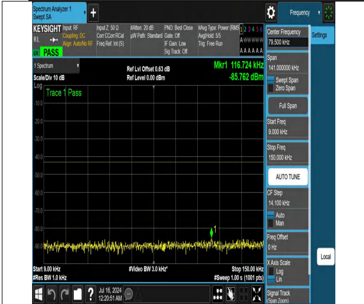
NTNV-DC_12A_n25A-PC3-15-5+30-M+L-N/A-N/A-DFT-QPSK-Edge e_1RB_Left-0.009-0.15-PASS
