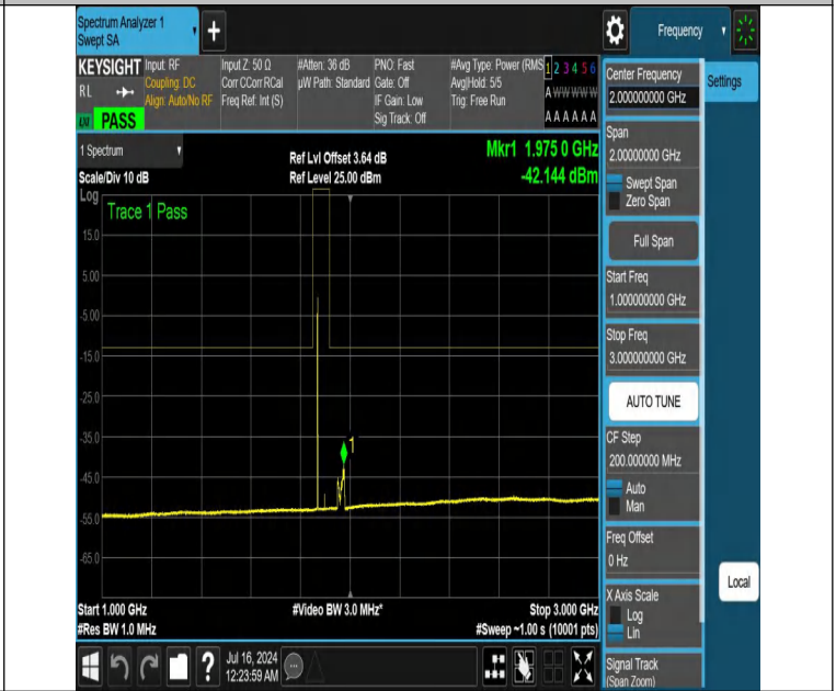
NTNV-DC_12A_n25A-PC3-15-5+30-M+M-N/A-N/A-DFT-PI2BPSK-E dge_1RB_Left-1000-3000-PASS
