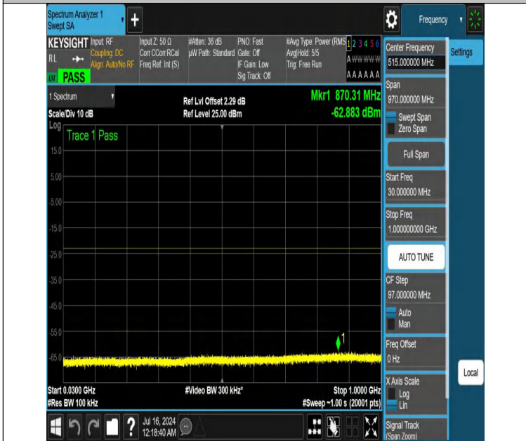
NTNV-DC_12A_n25A-PC3-15-5+30-M+L-N/A-N/A-DFT-PI2BPSK-Edge_1RB_Left-30-1000-PASS
