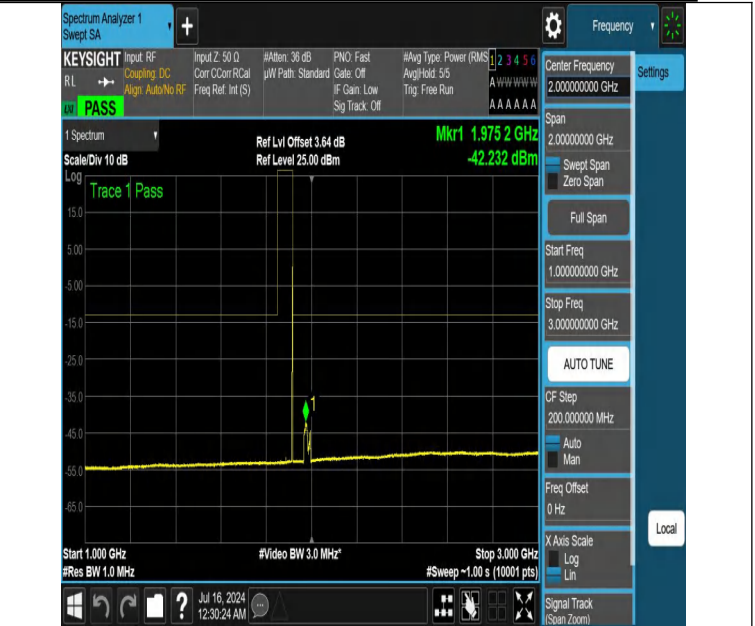
NTNV-DC_12A_n25A-PC3-15-5+30-M+H-N/A-N/A-DFT-PI2BPSK-E dge_1RB_Right-1000-3000-PASS
