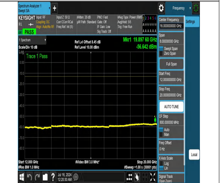
NTNV-DC_12A_n25A-PC3-15-5+30-M+L-N/A-N/A-DFT-PI2BPSK-E dge_1RB_Right-12000-20000-PASS
