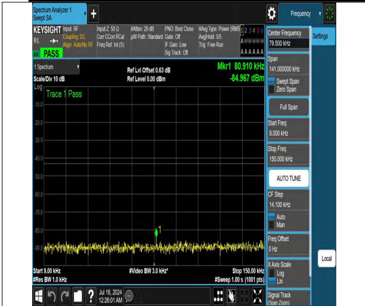
NTNV-DC_12A_n25A-PC3-15-5+30-M+M-N/A-N/A-DFT-QPSK-Edge_1RB_Left-0.009-0.15-PASS
