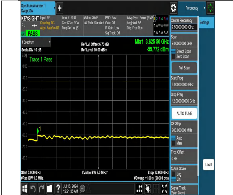
NTNV-DC_12A_n25A-PC3-15-5+30-M+L-N/A-N/A-DFT-QPSK-Edge e_1RB_Left-3000-12000-PASS
