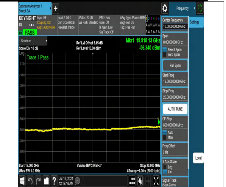
NTNV-DC_12A_n25A-PC3-15-5+30-M+L-N/A-N/A-DFT-PI2BPSK-E dge_1RB_Left-12000-20000-PASS
