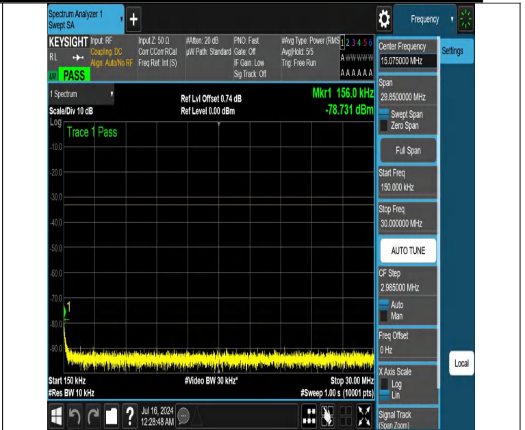
NTNV-DC_12A_n25A-PC3-15-5+30-M+H-N/A-N/A-DFT-PI2BPSK-E dge_1RB_Left-0.15-30-PASS
