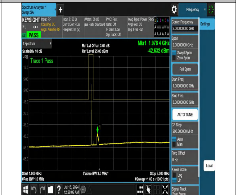
NTNV-DC_12A_n25A-PC3-15-5+30-M+H-N/A-N/A-DFT-PI2BPSK-E dge_1RB_Left-1000-3000-PASS
