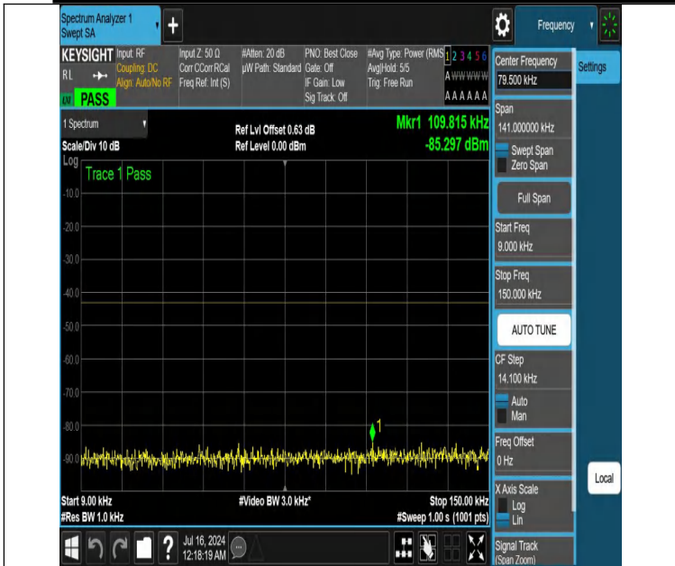
NTNV-DC_12A_n25A-PC3-15-5+30-M+L-N/A-N/A-DFT-PI2BPSK-Edge_1RB_Left-0.009-0.15-PASS
