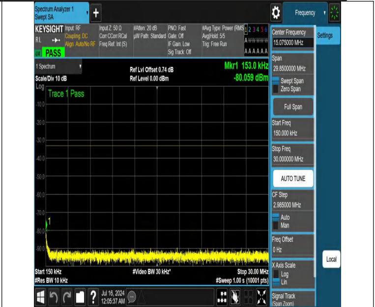
NTNV-DC_12A_n25A-PC3-15-5+25-M+L-N/A-N/A-DFT-QPSK-Edge _1RB_Left-0.15-30-PASS
