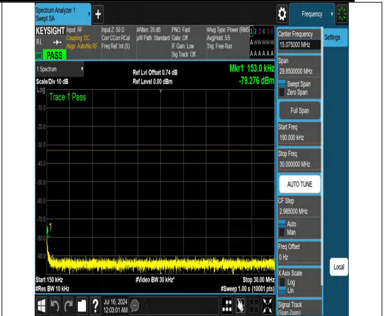
NTNV-DC_12A_n25A-PC3-15-5+25-M+L-N/A-N/A-DFT-PI2BPSK-E dge_1RB_Left-0.15-30-PASS
