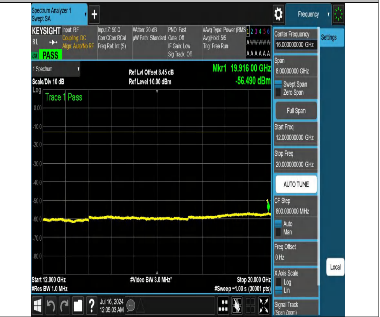
NTNV-DC_12A_n25A-PC3-15-5+25-M+L-N/A-N/A-DFT-PI2BPSK-E dge_1RB_Right-12000-20000-PASS
