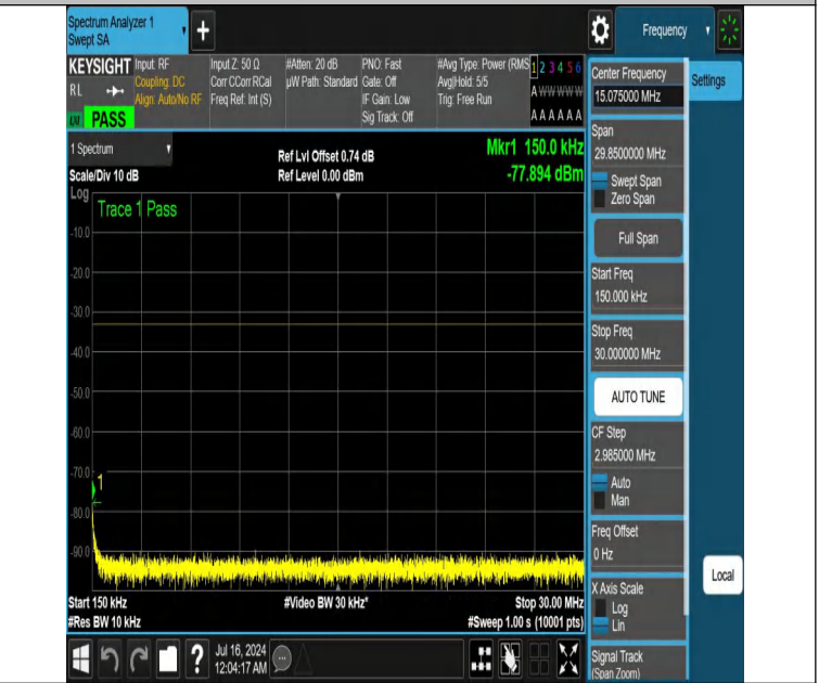
NTNV-DC_12A_n25A-PC3-15-5+25-M+L-N/A-N/A-DFT-PI2BPSK-E dge_1RB_Right-0.15-30-PASS
