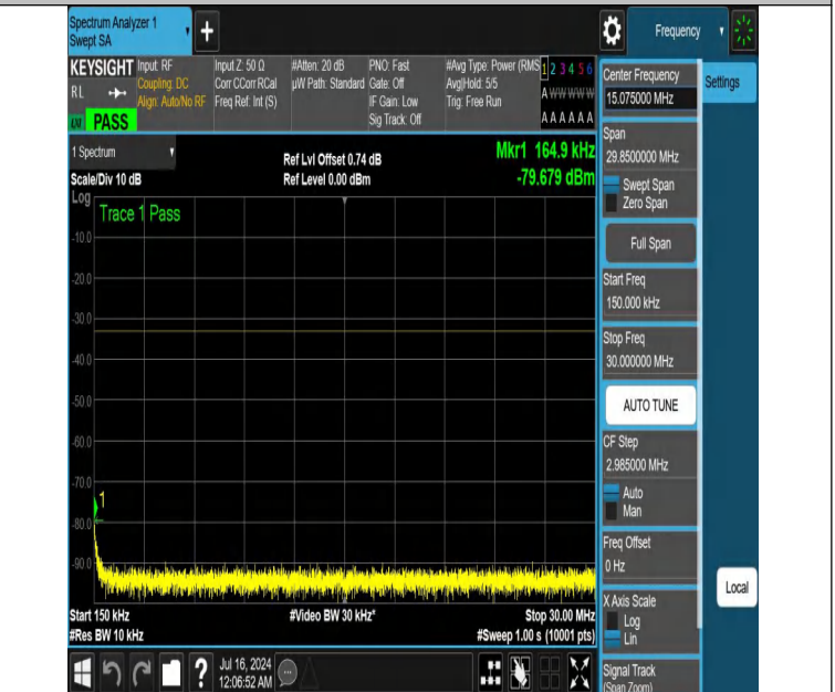
NTNV-DC_12A_n25A-PC3-15-5+25-M+L-N/A-N/A-DFT-QPSK-Edge _1RB_Right-0.15-30-PASS
