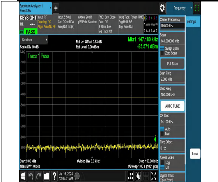
NTNV-DC_12A_n25A-PC3-15-5+25-M+L-N/A-N/A-DFT-PI2BPSK-Edge_1RB_Left-0.009-0.15-PASS
