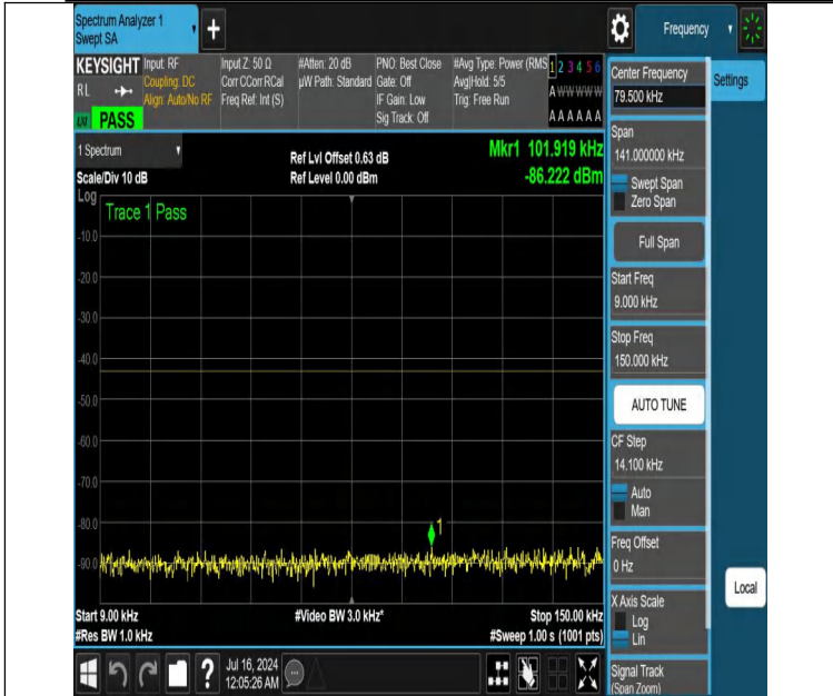
NTNV-DC_12A_n25A-PC3-15-5+25-M+L-N/A-N/A-DFT-QPSK-Edge e_1RB_Left-0.009-0.15-PASS
