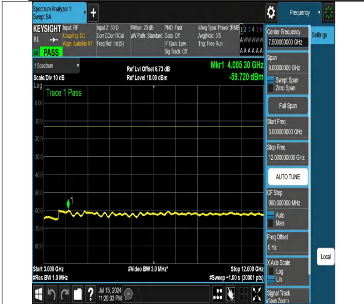
NTNV-DC_12A_n25A-PC3-15-5+10-M+L-N/A-N/A-DFT-QPSK-Edge e_1RB_Left-3000-12000-PASS
