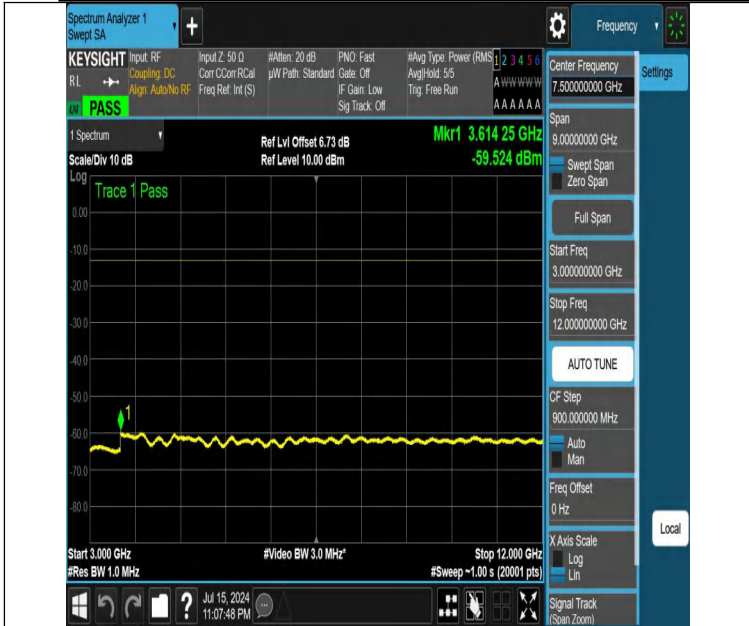
NTNV-DC_12A_n25A-PC3-15-5+5-M+M-N/A-N/A-DFT-PI2BPSK-E dge_1RB_Left-3000-12000-PASS
