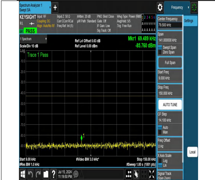
NTNV-DC_12A_n25A-PC3-15-5+10-M+L-N/A-N/A-DFT-QPSK-Edge e_1RB_Left-0.009-0.15-PASS
