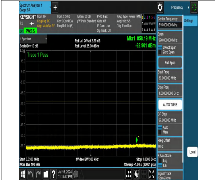
NTNV-DC_12A_n25A-PC3-15-5+5-M+H-N/A-N/A-DFT-PI2BPSK-E dge_1RB_Left-30-1000-PASS
