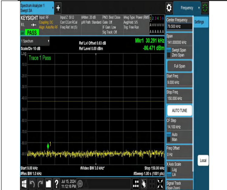
NTNV-DC_12A_n25A-PC3-15-5+5-M+H-N/A-N/A-DFT-PI2BPSK-E dge_1RB_Left-0.009-0.15-PASS
