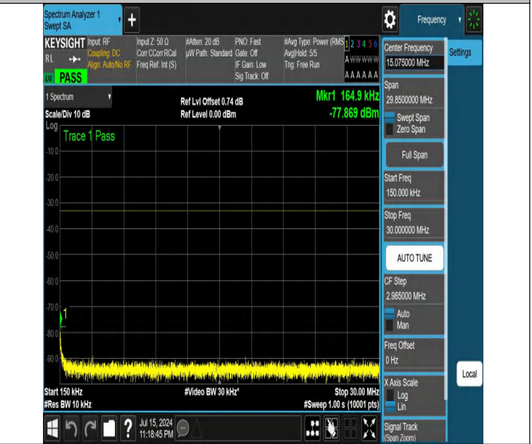
NTNV-DC_12A_n25A-PC3-15-5+10-M+L-N/A-N/A-DFT-PI2BPSK-E dge_1RB_Right-0.15-30-PASS
