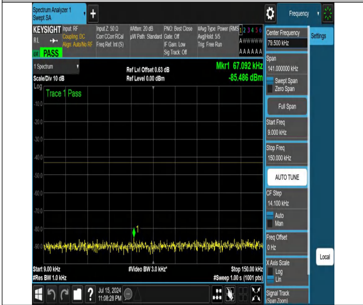
NTNV-DC_12A_n25A-PC3-15-5+5-M+M-N/A-N/A-DFT-PI2BPSK-E dge_1RB_Right-0.009-0.15-PASS
