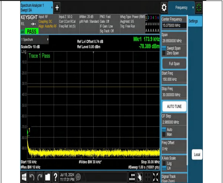
NTNV-DC_12A_n25A-PC3-15-5+10-M+L-N/A-N/A-DFT-PI2BPSK-E dge_1RB_Left-0.15-30-PASS
