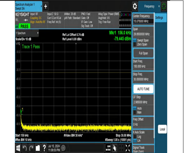
NTNV-DC_12A_n25A-PC3-15-5+5-M+M-N/A-N/A-DFT-QPSK-Edge _1RB_Left-0.15-30-PASS
