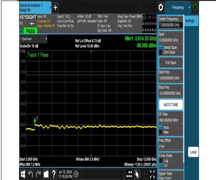
NTNV-DC_12A_n25A-PC3-15-5+5-M+H-N/A-N/A-DFT-QPSK-Edge _1RB_Left-3000-12000-PASS
