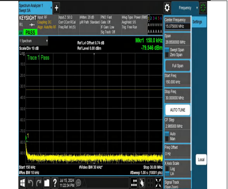
NTNV-DC_12A_n25A-PC3-15-5+10-M+M-N/A-N/A-DFT-PI2BPSK-E dge_1RB_Left-0.15-30-PASS
