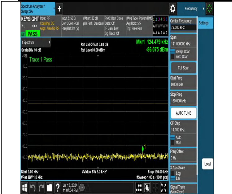
NTNV-DC_12A_n25A-PC3-15-5+5-M+M-N/A-N/A-DFT-PI2BPSK-E dge_1RB_Left-0.009-0.15-PASS
