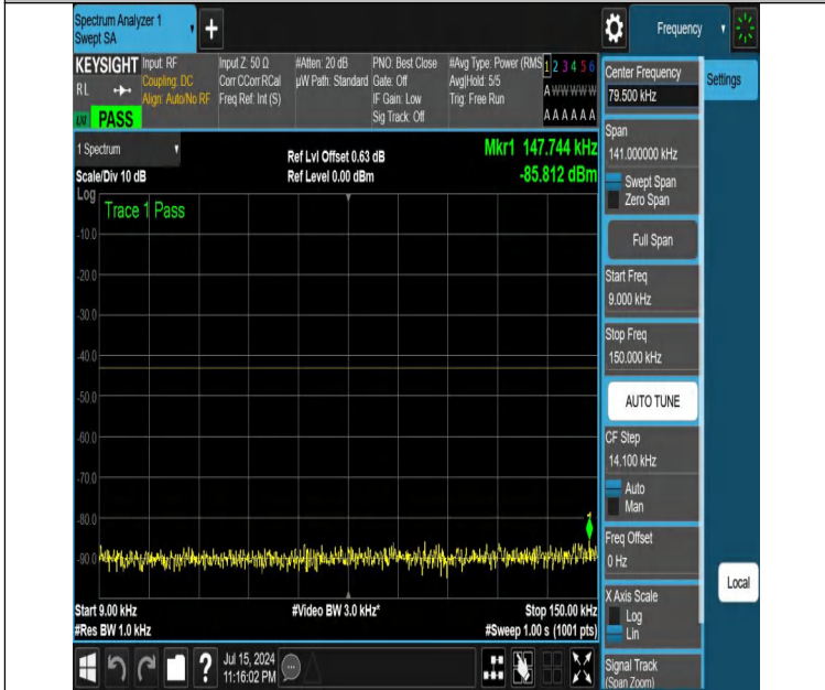
NTNV-DC_12A_n25A-PC3-15-5+5-M+H-N/A-N/A-DFT-QPSK-Edge _1RB_Right-0.009-0.15-PASS
