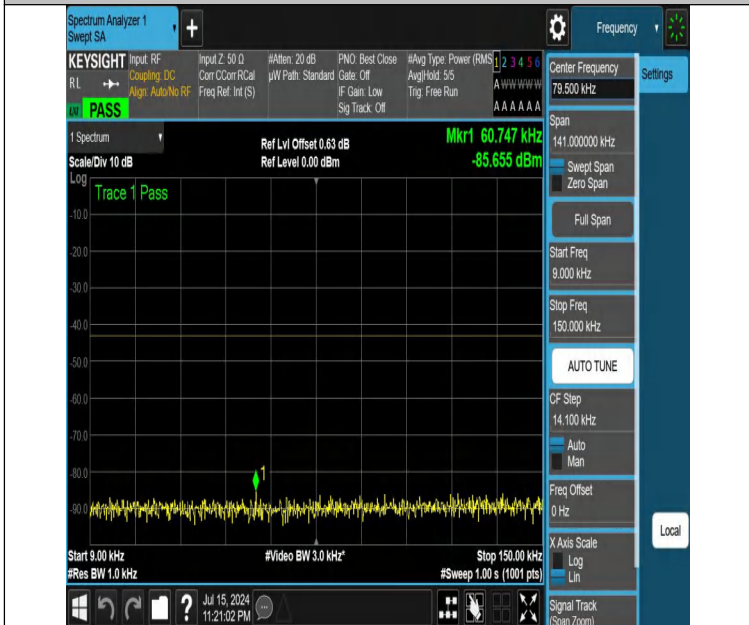
NTNV-DC_12A_n25A-PC3-15-5+10-M+L-N/A-N/A-DFT-QPSK-Edge e_1RB_Right-0.009-0.15-PASS
