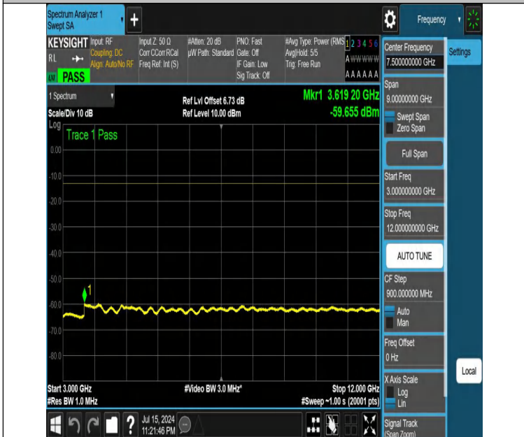
NTNV-DC_12A_n25A-PC3-15-5+10-M+L-N/A-N/A-DFT-QPSK-Edge e_1RB_Right-3000-12000-PASS
