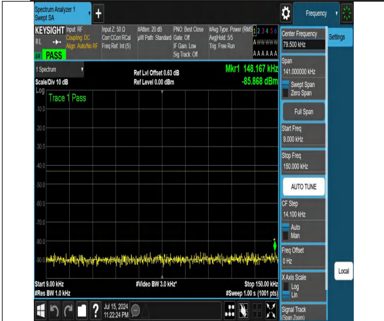
NTNV-DC_12A_n25A-PC3-15-5+10-M+M-N/A-N/A-DFT-PI2BPSK-Edge_1RB_Left-0.009-0.15-PASS
