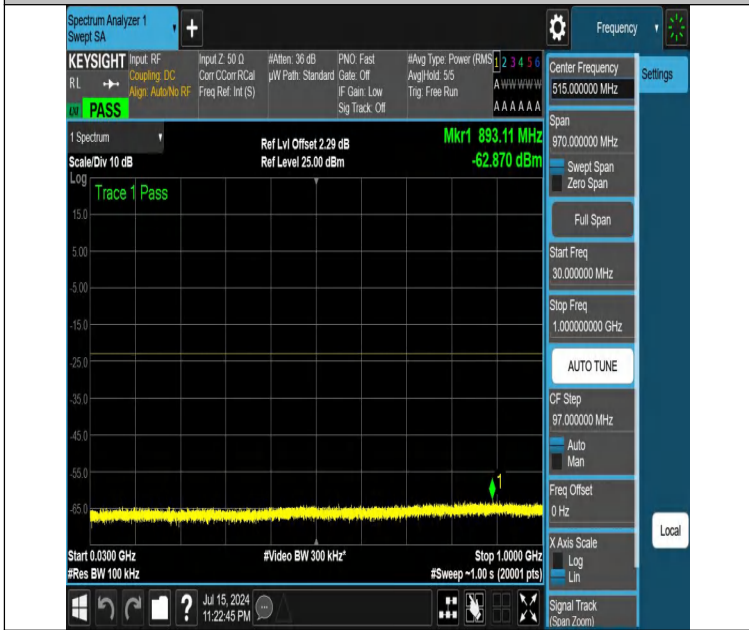
NTNV-DC_12A_n25A-PC3-15-5+10-M+M-N/A-N/A-DFT-PI2BPSK-Edge_1RB_Left-30-1000-PASS
