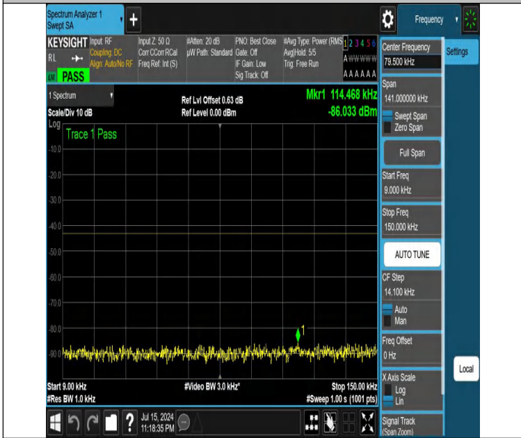
NTNV-DC_12A_n25A-PC3-15-5+10-M+L-N/A-N/A-DFT-PI2BPSK-Edge_1RB_Right-0.009-0.15-PASS
