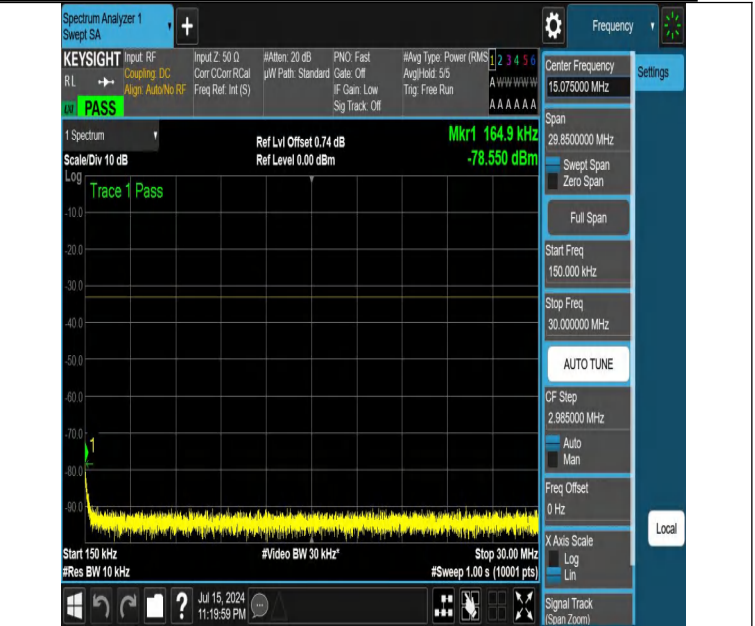
NTNV-DC_12A_n25A-PC3-15-5+10-M+L-N/A-N/A-DFT-QPSK-Edge _1RB_Left-0.15-30-PASS
