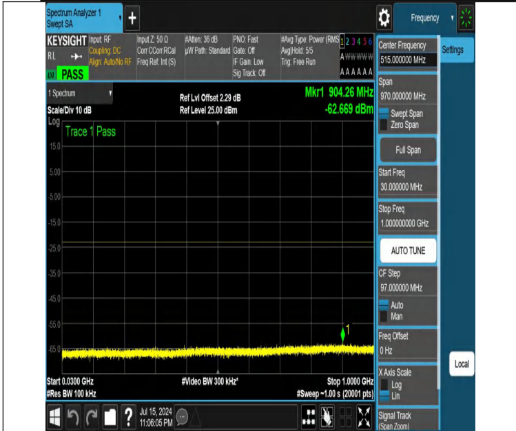
NTNV-DC_12A_n25A-PC3-15-5+5-M+L-N/A-N/A-DFT-QPSK-Edge_1RB_Right-30-1000-PASS
