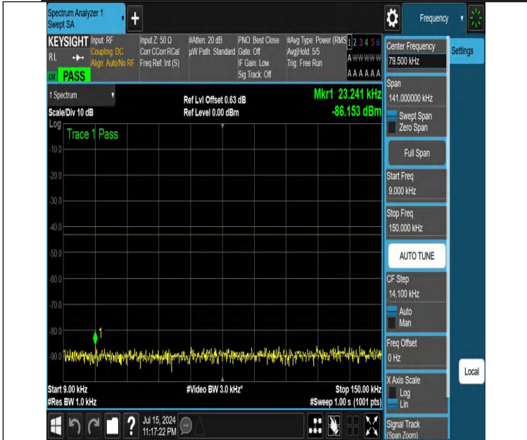
NTNV-DC_12A_n25A-PC3-15-5+10-M+L-N/A-N/A-DFT-PI2BPSK-Edge_1RB_Left-0.009-0.15-PASS
