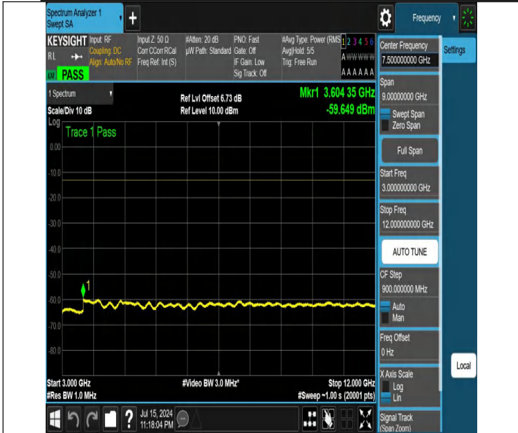
NTNV-DC_12A_n25A-PC3-15-5+10-M+L-N/A-N/A-DFT-PI2BPSK-Edge_1RB_Left-3000-12000-PASS
