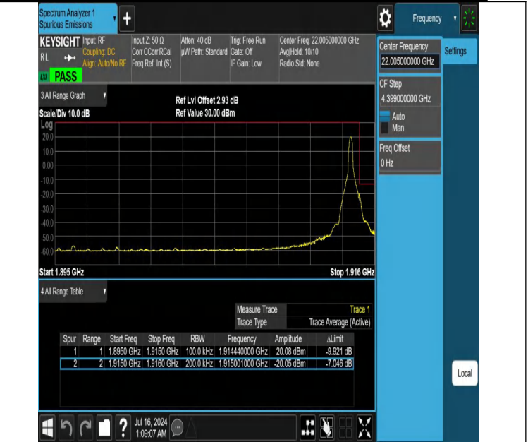
NTNV-DC_12A_n25A-PC3-15-5+20-M+H-N/A-N/A-DFT-PI2BPSK-E dge_1RB_Right-PASS
