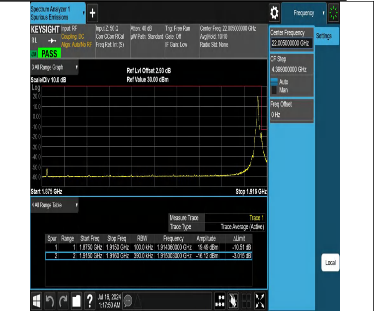
NTNV-DC_12A_n25A-PC3-15-5+40-M+H-N/A-N/A-DFT-PI2BPSK-E dge_1RB_Right-PASS
