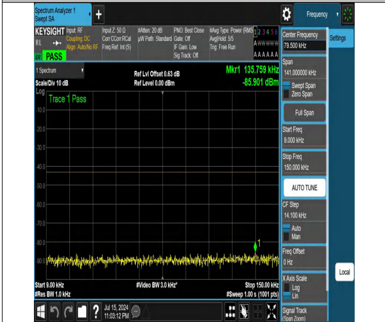
NTNV-DC_12A_n25A-PC3-15-5+5-M+L-N/A-N/A-DFT-PI2BPSK-E dge_1RB_Right-0.009-0.15-PASS
