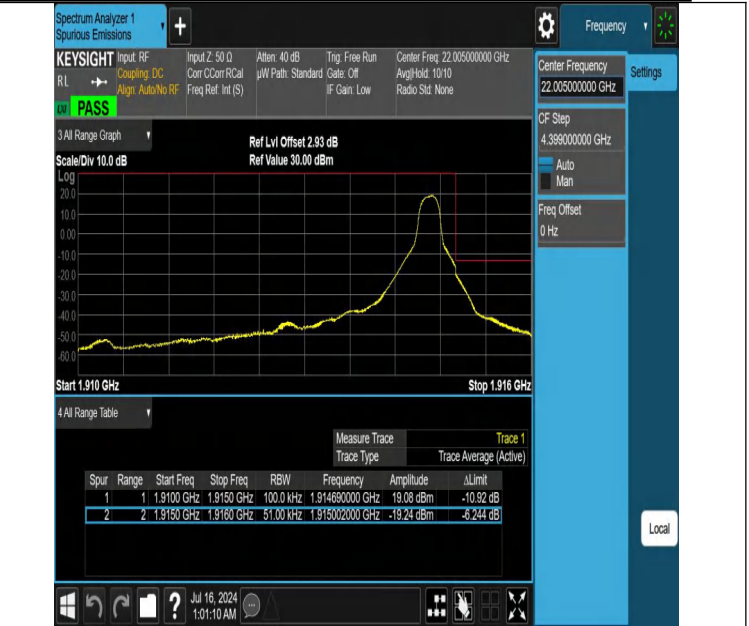
NTVN-DC_12A_n25A-PC3-15-5+5-M+H-N/A-N/A-DFT-QPSK-Edge_1RB_Right-PASS
