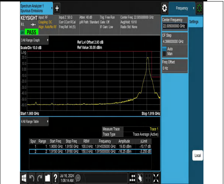
NTNV-DC_12A_n25A-PC3-15-5+15-M+H-N/A-N/A-DFT-PI2BPSK-E dge_1RB_Right-PASS
