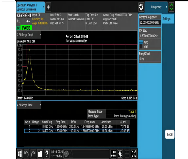
NTNV-DC_12A_n25A-PC3-15-5+25-M+L-N/A-N/A-DFT-QPSK-Edge_1RB_Left-PASS
