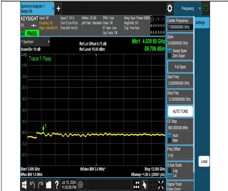
NTNV-DC_12A_n25A-PC3-15-5+5-M+L-N/A-N/A-DFT-PI2BPSK-E dge_1RB_Right-3000-12000-PASS
