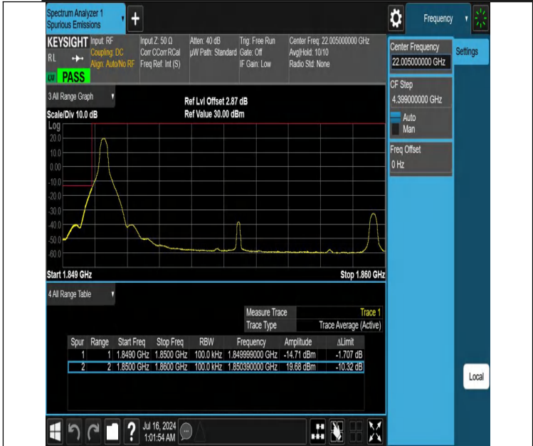
NTVN-DC_12A_n25A-PC3-15-5+10-M+L-N/A-N/A-DFT-PI2BPSK-Edge_1RB_Left-PASS
