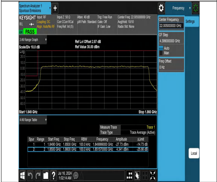
NTVN-DC_12A_n25A-PC3-15-5+10-M+L-N/A-N/A-DFT-PI2BPSK-Outer_Full-PASS
