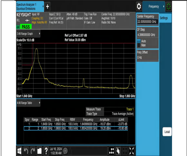
NTNV-DC_12A_n25A-PC3-15-5+10-M+L-N/A-N/A-DFT-QPSK-Edge_1RB_Left-PASS
