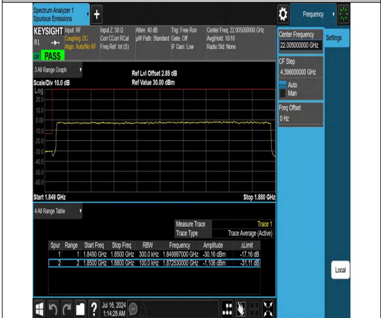
NTNV-DC_12A_n25A-PC3-15-5+30-M+L-N/A-N/A-DFT-QPSK-Outer_Full-PASS
