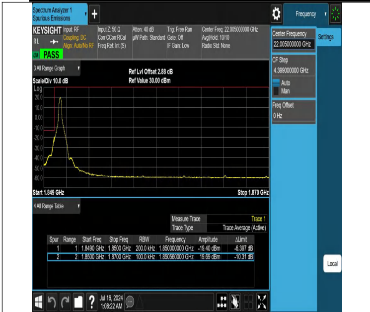
NTNV-DC_12A_n25A-PC3-15-5+20-M+L-N/A-N/A-DFT-QPSK-Edge_1RB_Left-PASS
