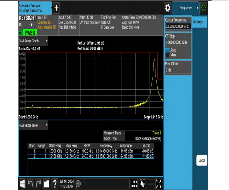
NTNV-DC_12A_n25A-PC3-15-5+25-M+H-N/A-N/A-DFT-PI2BPSK-E dge_1RB_Right-PASS
