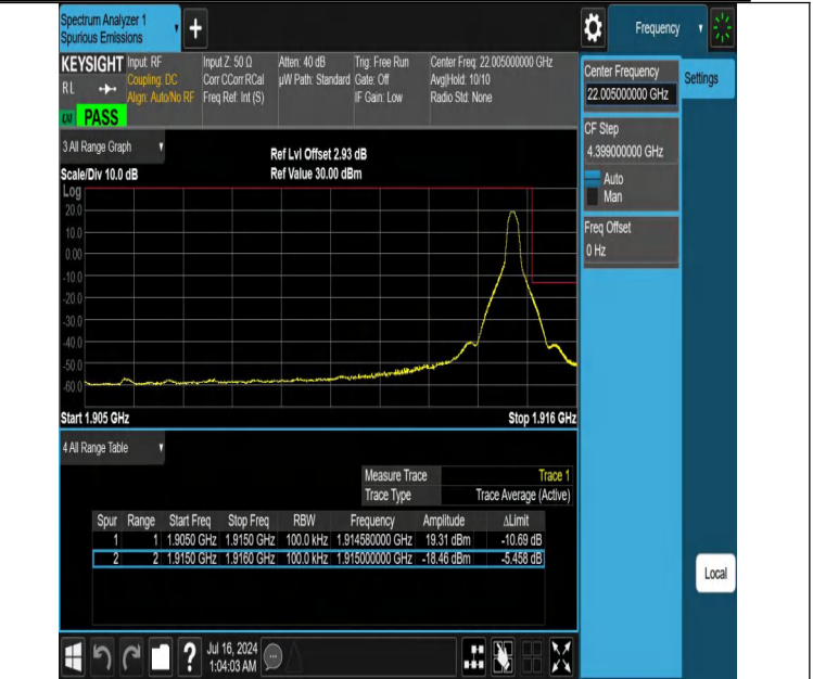
NTNV-DC_12A_n25A-PC3-15-5+10-M+H-N/A-N/A-DFT-QPSK-Edge_1RB_Right-PASS
