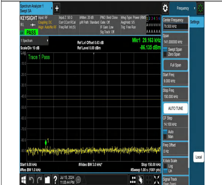
NTNV-DC_12A_n25A-PC3-15-5+5-M+L-N/A-N/A-DFT-QPSK-Edge_1RB_Right-0.009-0.15-PASS
