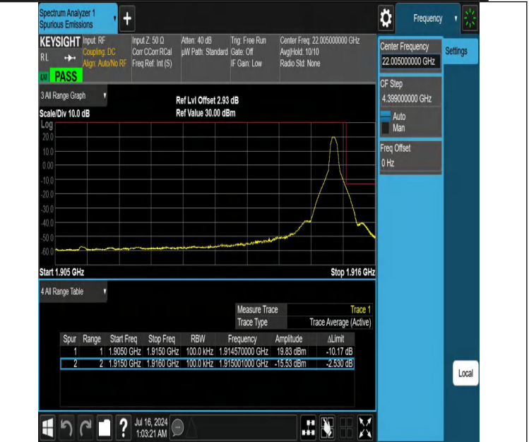
NTVN-DC_12A_n25A-PC3-15-5+10-M+H-N/A-N/A-DFT-PI2BPSK-E dge_1RB_Right-PASS
