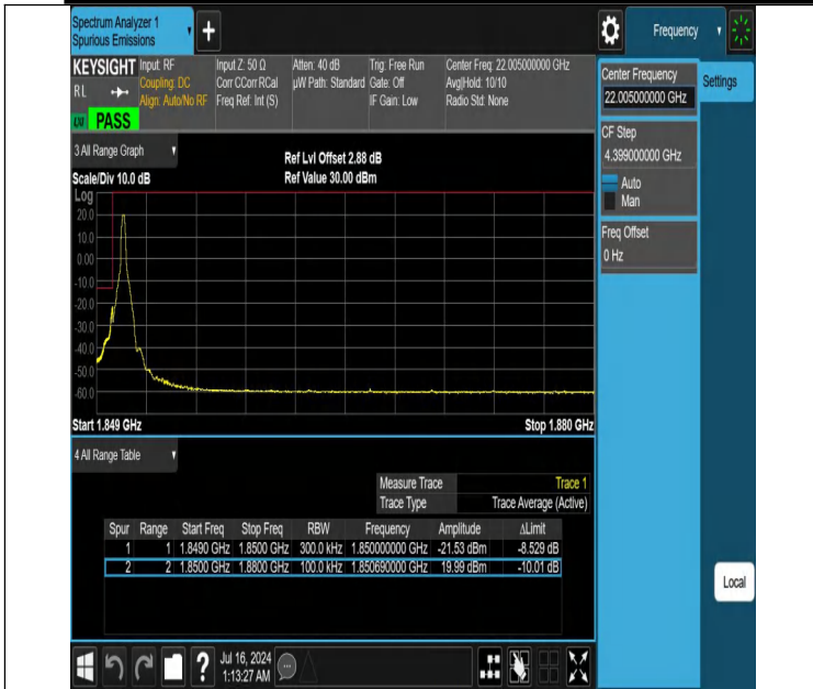
NTNV-DC_12A_n25A-PC3-15-5+30-M+L-N/A-N/A-DFT-PI2BPSK-Edge_1RB_Left-PASS
