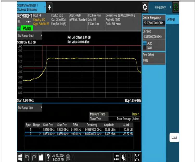
NTVN-DC_12A_n25A-PC3-15-5+5-M+L-N/A-N/A-DFT-QPSK-Outer_Full-PASS
