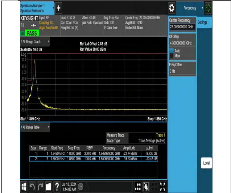
NTNV-DC_12A_n25A-PC3-15-5+30-M+L-N/A-N/A-DFT-QPSK-Edge_1RB_Left-PASS
