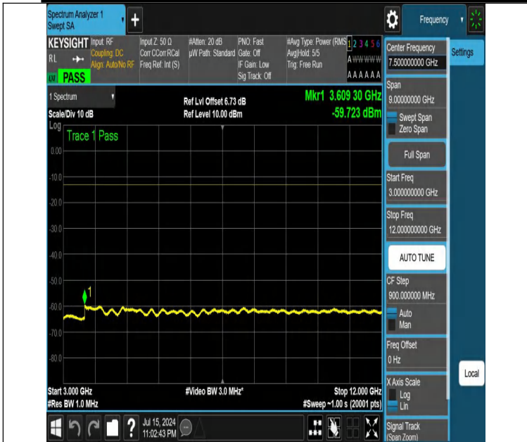
NTNV-DC_12A_n25A-PC3-15-5+5-M+L-N/A-N/A-DFT-PI2BPSK-E dge_1RB_Left-3000-12000-PASS
