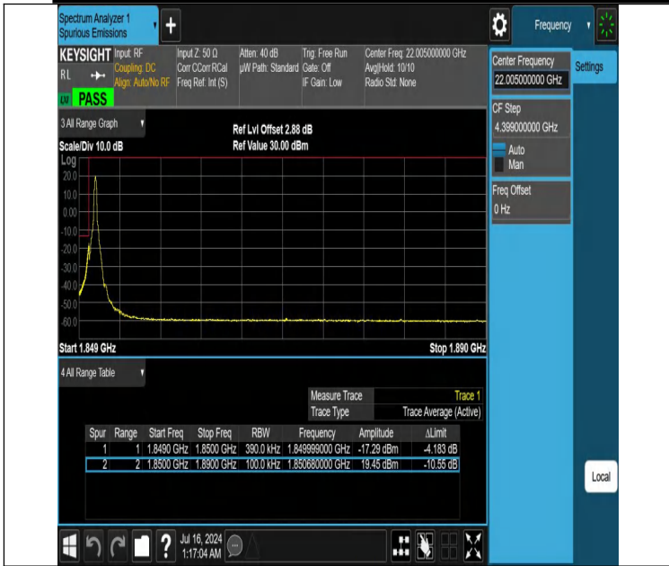
NTNV-DC_12A_n25A-PC3-15-5+40-M+L-N/A-N/A-DFT-QPSK-Edge_1RB_Left-PASS
