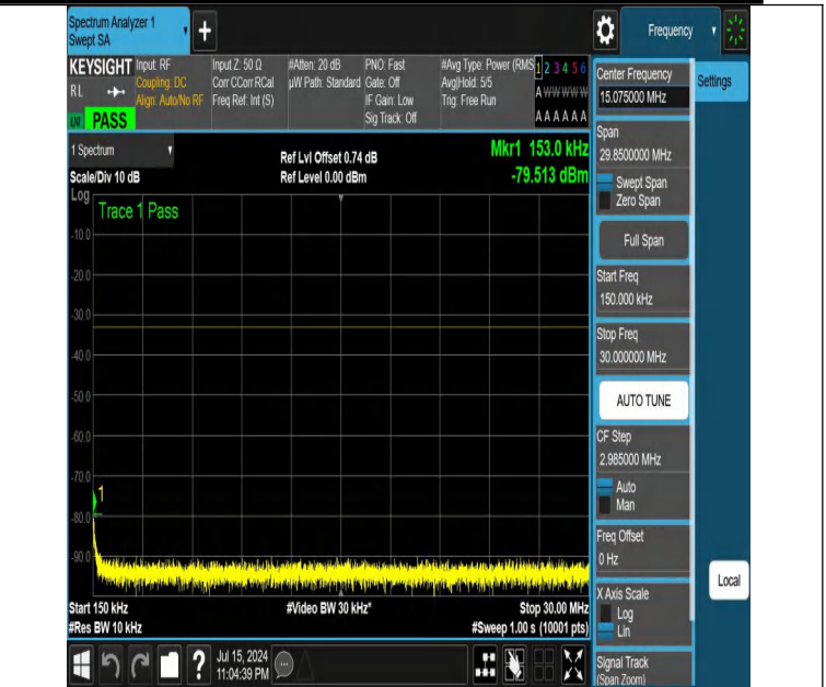
NTNV-DC_12A_n25A-PC3-15-5+5-M+L-N/A-N/A-DFT-QPSK-Edge_1RB_Left-0.15-30-PASS
