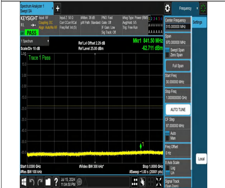
NTNV-DC_12A_n25A-PC3-15-5+5-M+L-N/A-N/A-DFT-QPSK-Edge_1RB_Left-30-1000-PASS
