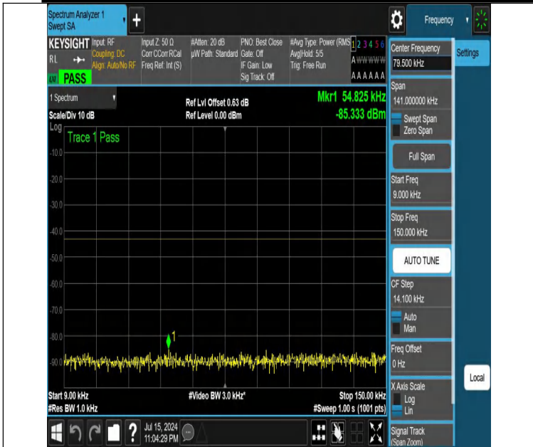
NTNV-DC_12A_n25A-PC3-15-5+5-M+L-N/A-N/A-DFT-QPSK-Edge_1RB_Left-0.009-0.15-PASS
