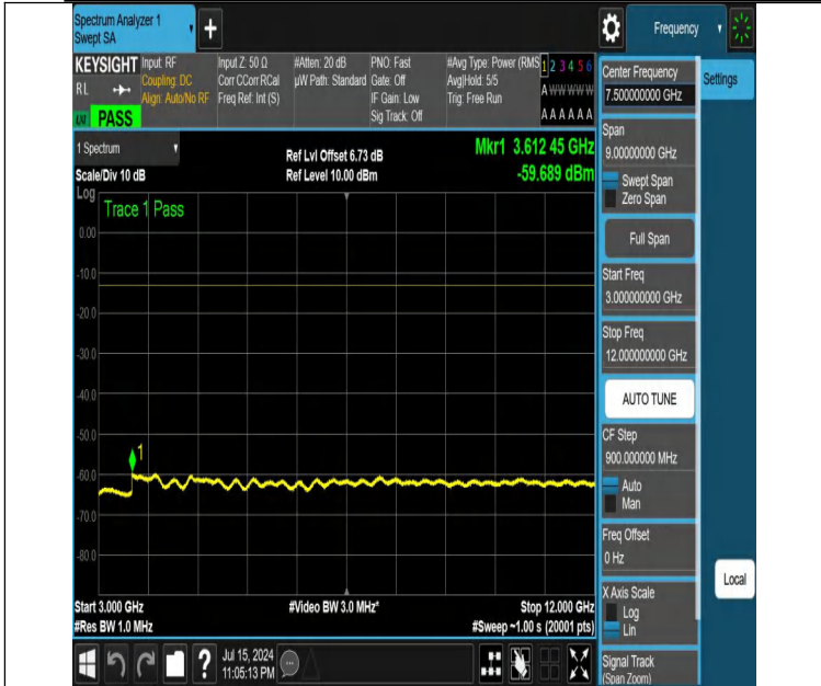
NTNV-DC_12A_n25A-PC3-15-5+5-M+L-N/A-N/A-DFT-QPSK-Edge_1RB_Left-3000-12000-PASS
