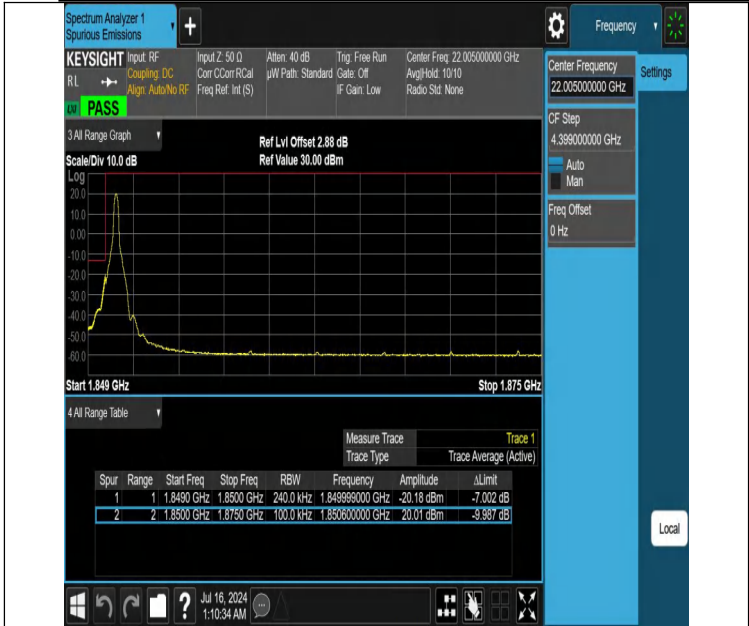
NTNV-DC_12A_n25A-PC3-15-5+25-M+L-N/A-N/A-DFT-PI2BPSK-Edge_1RB_Left-PASS
