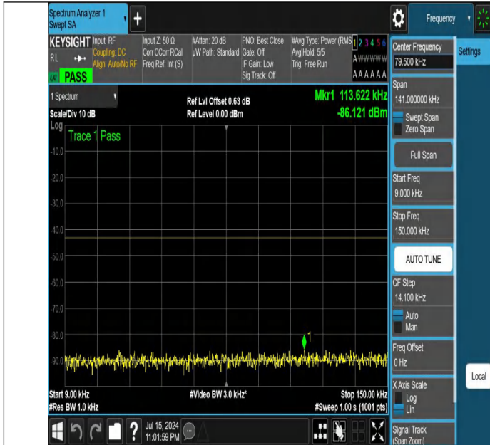
NTNV-DC_12A_n25A-PC3-15-5+5-M+L-N/A-N/A-DFT-PI2BPSK-E dge_1RB_Left-0.009-0.15-PASS
