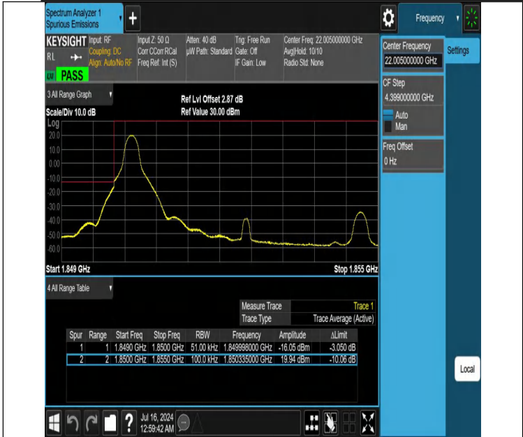
NTVN-DC_12A_n25A-PC3-15-5+5-M+L-N/A-N/A-DFT-QPSK-Edge_1RB_Left-PASS
