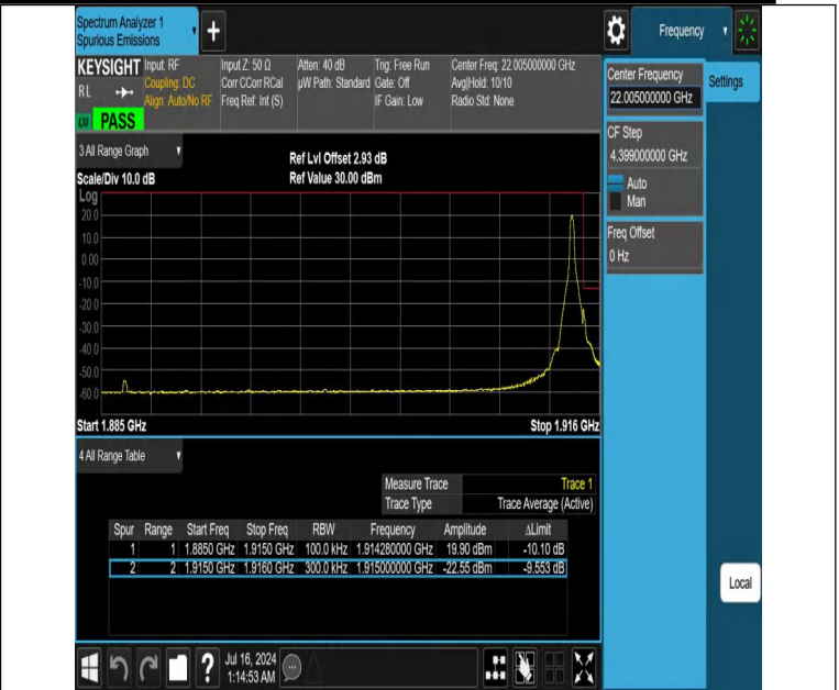
NTNV-DC_12A_n25A-PC3-15-5+30-M+H-N/A-N/A-DFT-PI2BPSK-E dge_1RB_Right-PASS
