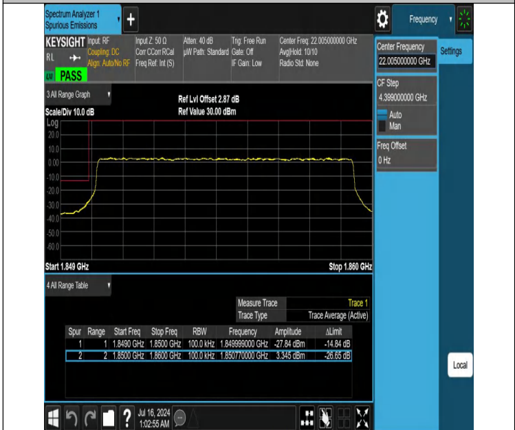
NTNV-DC_12A_n25A-PC3-15-5+10-M+L-N/A-N/A-DFT-QPSK-Outer_Full-PASS
