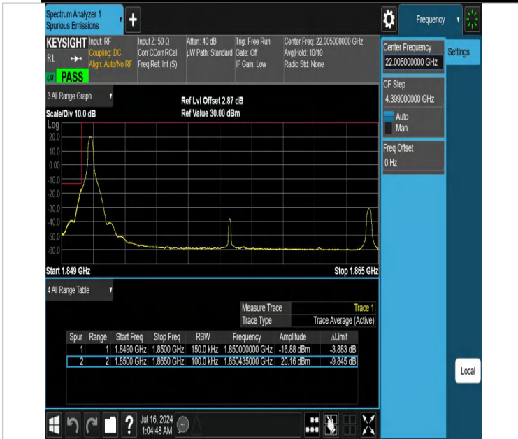
NTNV-DC_12A_n25A-PC3-15-5+15-M+L-N/A-N/A-DFT-PI2BPSK-Edge_1RB_Left-PASS
