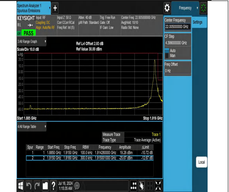
NTNV-DC_12A_n25A-PC3-15-5+30-M+H-N/A-N/A-DFT-QPSK-Edge_1RB_Right-PASS
