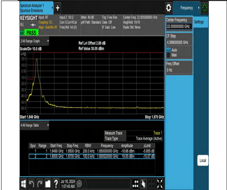
NTNV-DC_12A_n25A-PC3-15-5+20-M+L-N/A-N/A-DFT-PI2BPSK-Edge_1RB_Left-PASS
