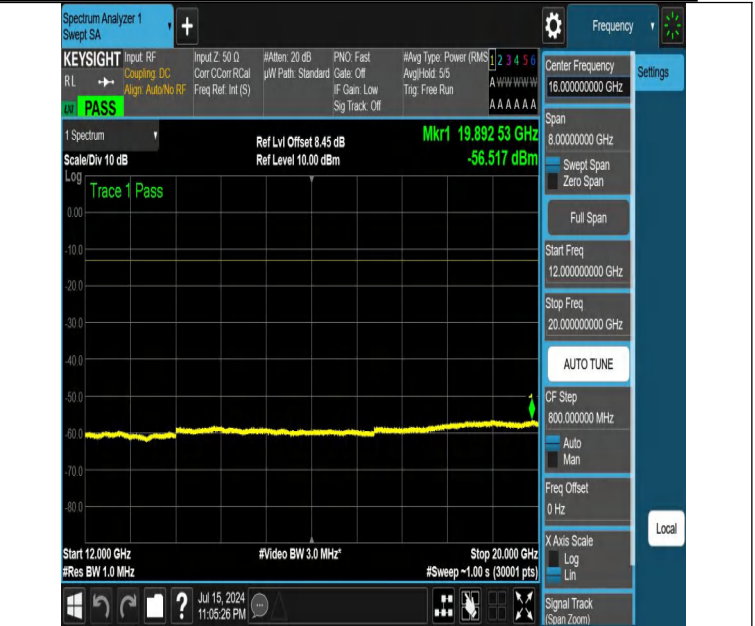
NTNV-DC_12A_n25A-PC3-15-5+5-M+L-N/A-N/A-DFT-QPSK-Edge_1RB_Left-12000-20000-PASS
