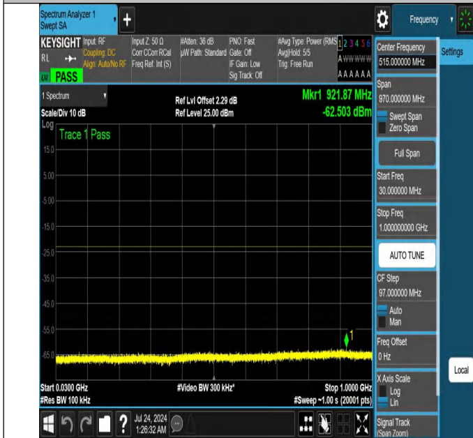
NTNV-N25-PC3-15-40-M-DFT-QPSK-Edge_1RB_Left-30-1000-A nt1-PASS
