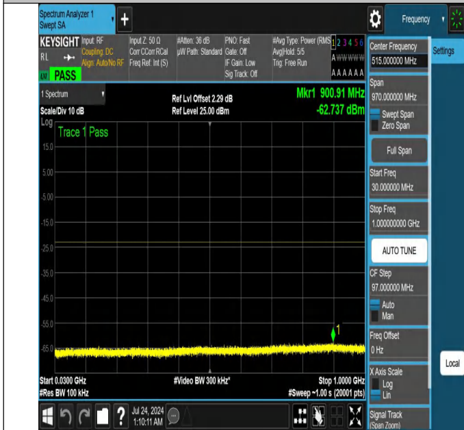
NTNV-N25-PC3-15-30-M-DFT-QPSK-Edge_1RB_Left-30-1000-A nt1-PASS
