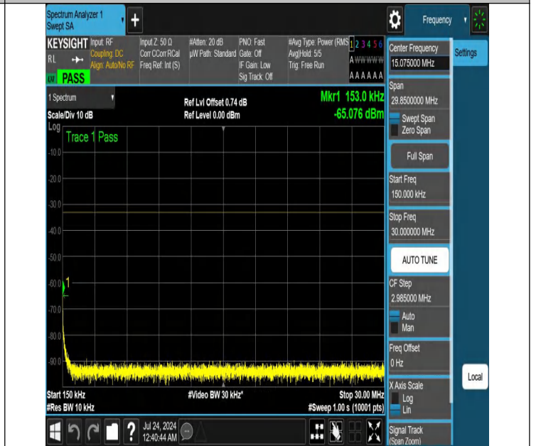
NTNV-N25-PC3-15-20-M-DFT-QPSK-Edge_1RB_Right-0.15-30-A nt1-PASS
