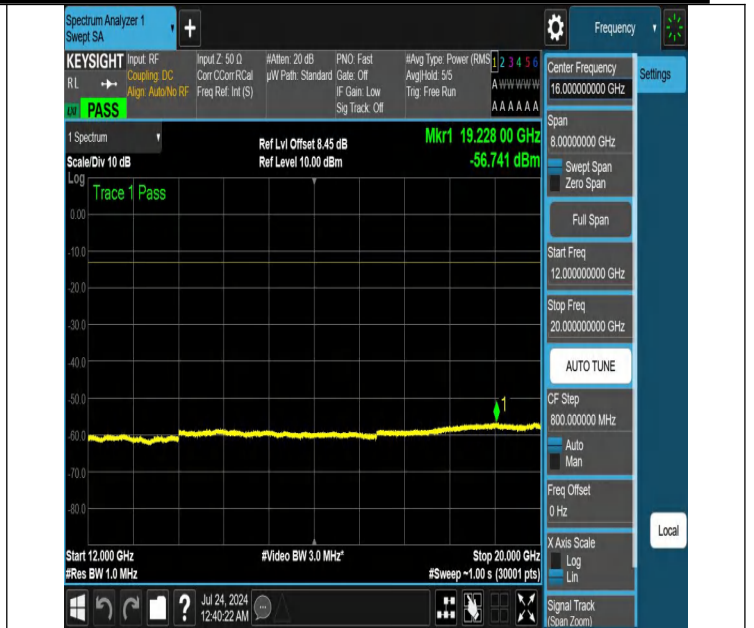
NTNV-N25-PC3-15-20-M-DFT-QPSK-Edge_1RB_Left-12000-200 00-Ant1-PASS
