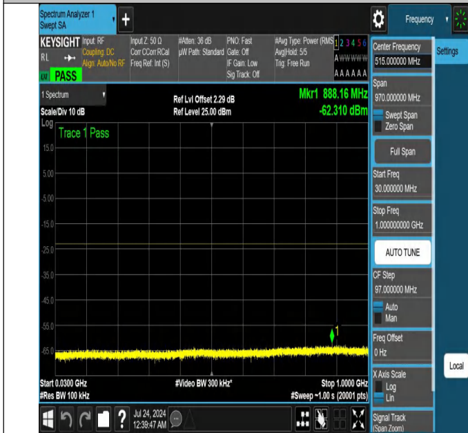
NTNV-N25-PC3-15-20-M-DFT-QPSK-Edge_1RB_Left-30-1000-A nt1-PASS
