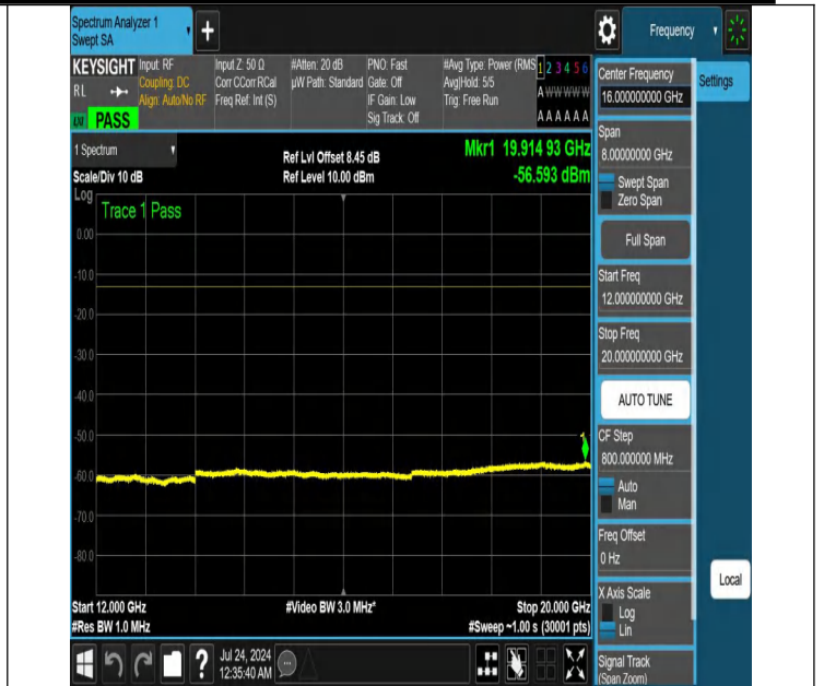
NTNV-N25-PC3-15-20-L-DFT-QPSK-Edge_1RB_Left-12000-2000 0-Ant1-PASS
