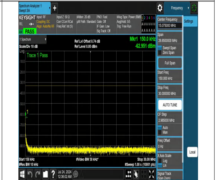
NTNV-N25-PC3-15-20-L-DFT-QPSK-Edge_1RB_Right-0.15-30-A nt1-PASS
