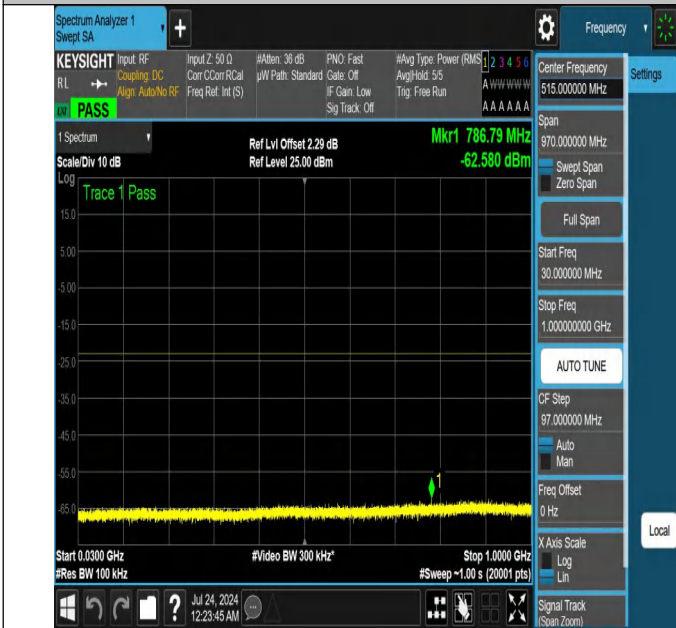
NTNV-N25-PC3-15-15-M-DFT-QPSK-Edge_1RB_Left-30-1000-A nt1-PASS
