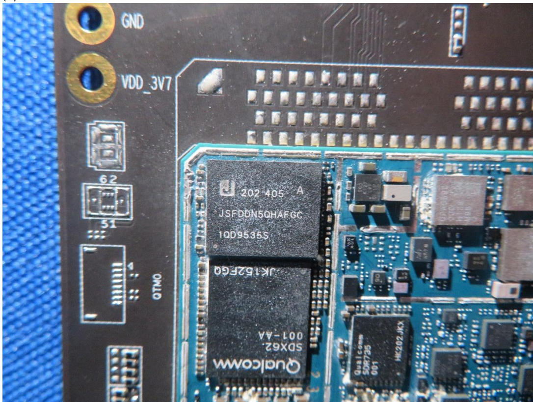
(6) EUT Photo
