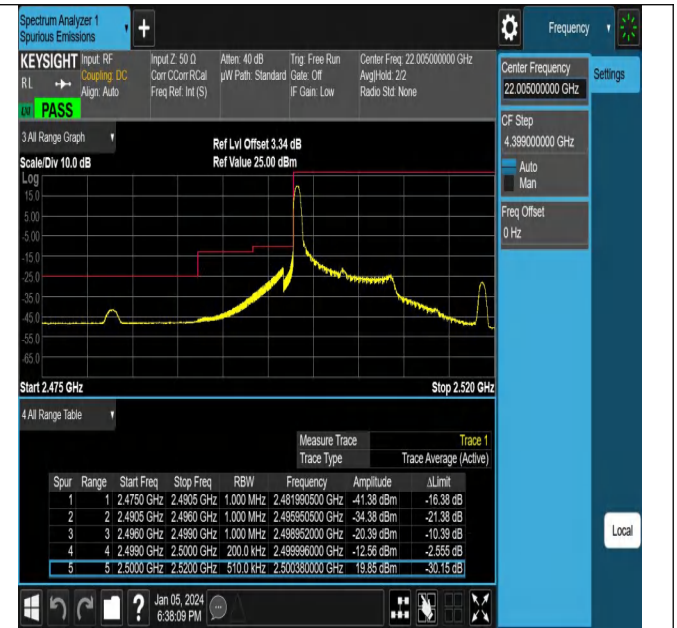
NTNV_N7_PC3_15_10_L_TID20_#1
