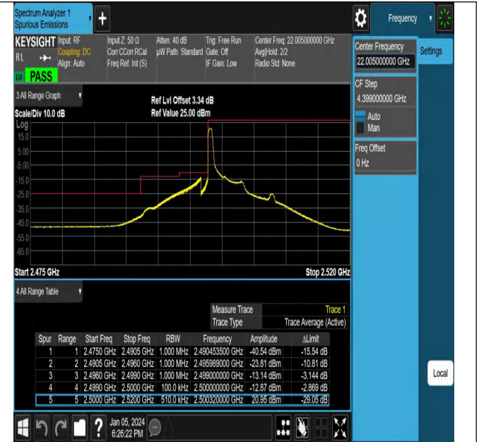
NTNV_N7_PC3_15_5_L_TID8_#1
