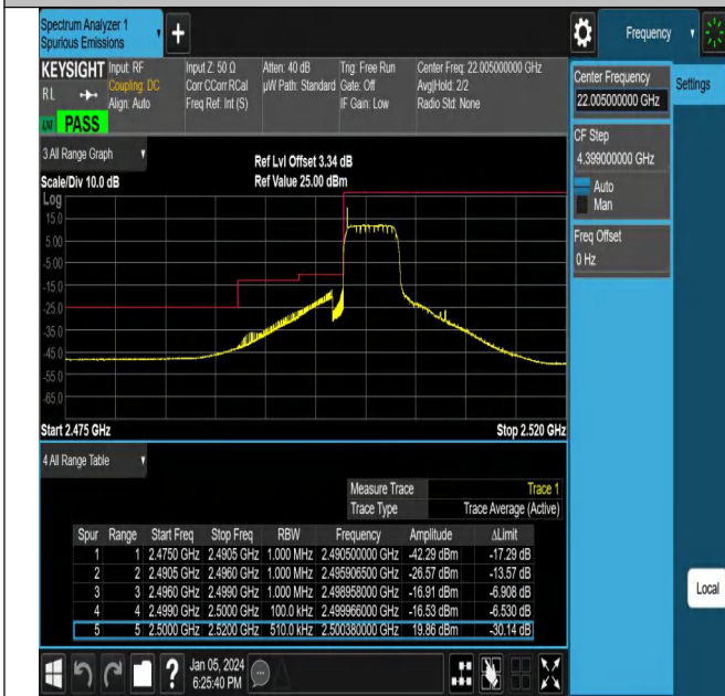
NTNV_N7_PC3_15_5_L_TID4_#1
