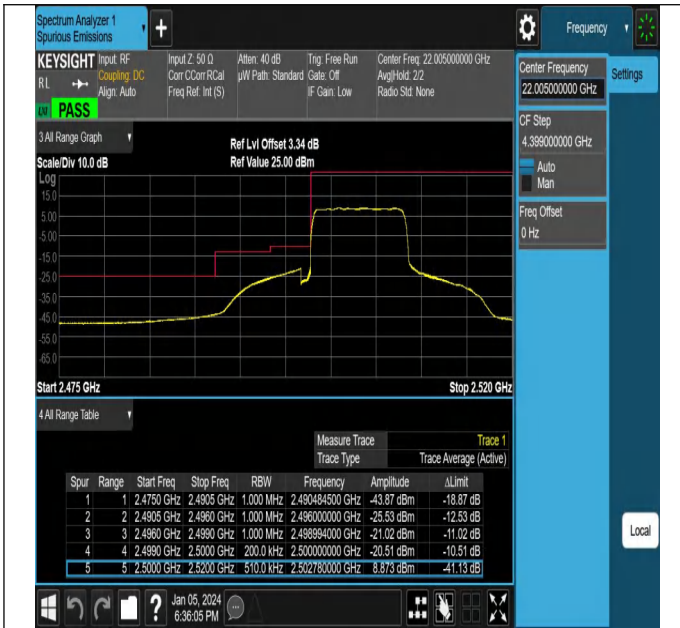
NTNV_N7_PC3_15_10_L_TID7_#1
