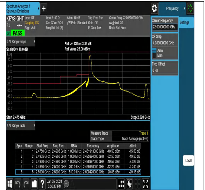
NTNV_N7_PC3_15_10_L_TID8_#1
