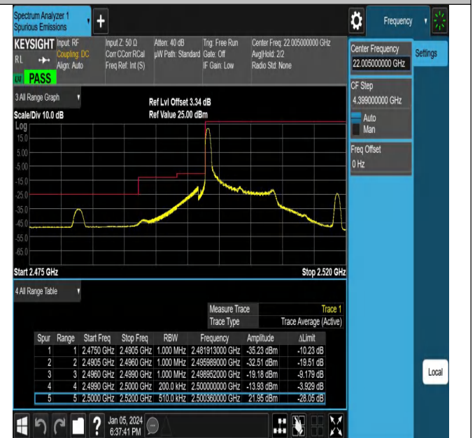
NTNV_N7_PC3_15_10_L_TID17_#1
