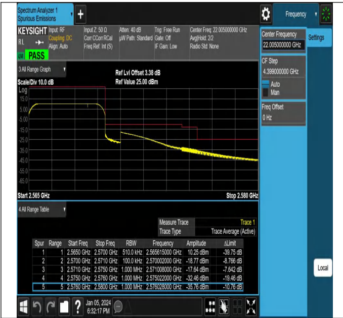
NTNV_N7_PC3_15_5_H_TID16_#1
