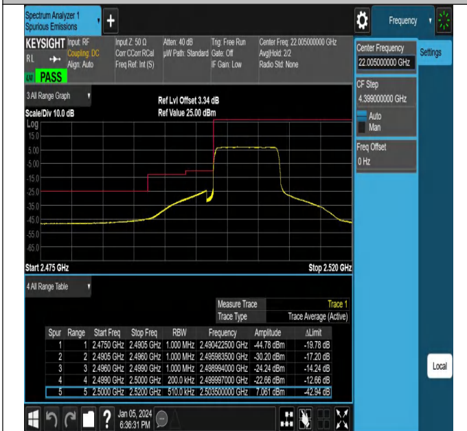
NTNV_N7_PC3_15_10_L_TID10_#1
