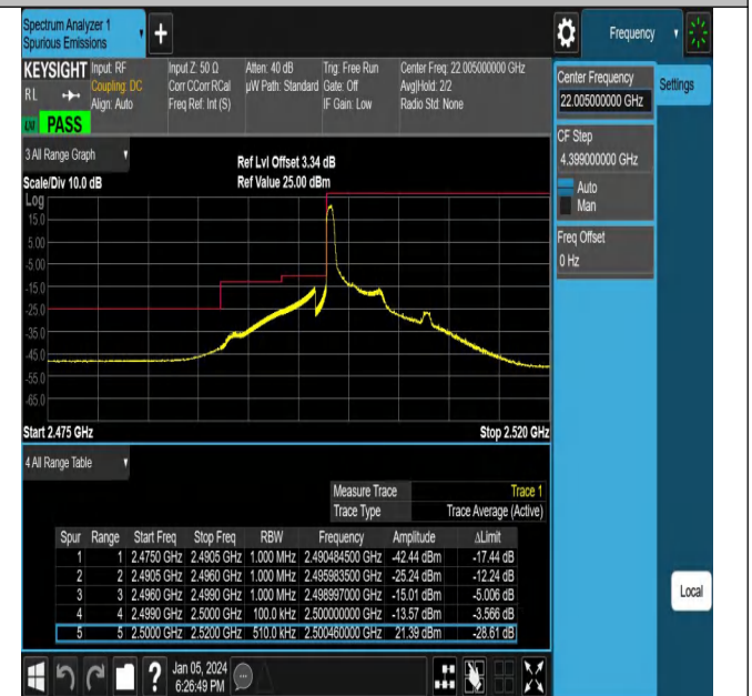
NTNV_N7_PC3_15_5_L_TID11_#1
