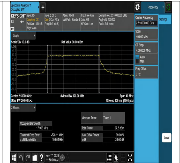
NTNV_N7_PC3_15_20_L_TID2_Ant1#1
