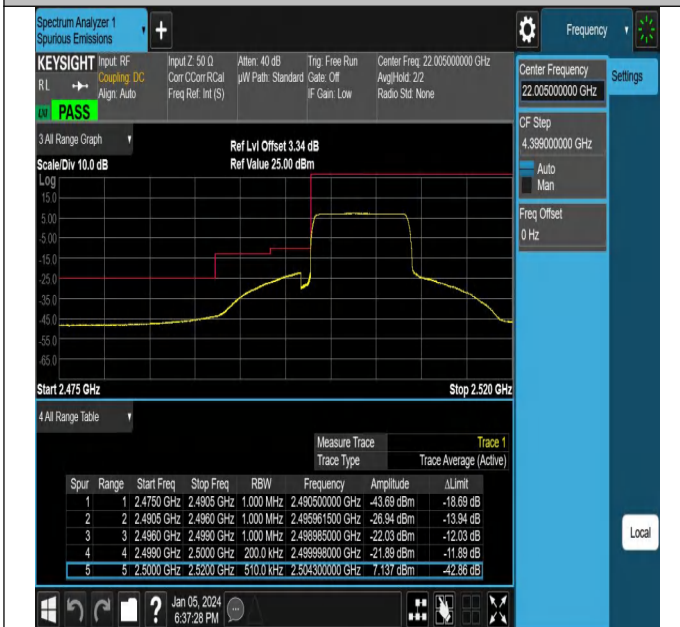
NTNV_N7_PC3_15_10_L_TID16_#1
