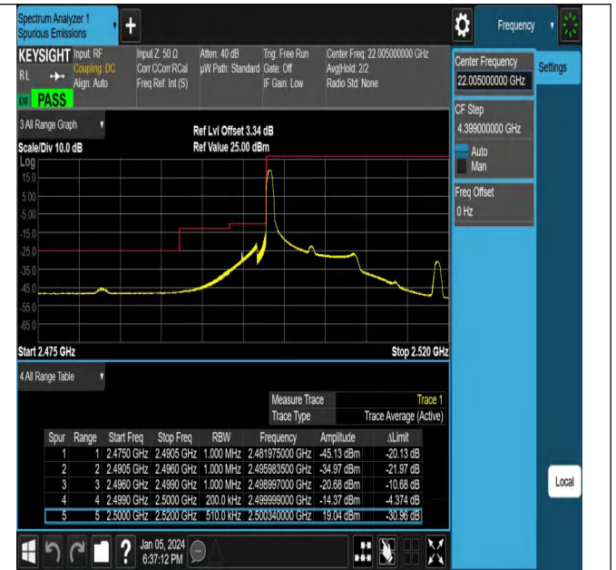
NTNV_N7_PC3_15_10_L_TID14_#1
