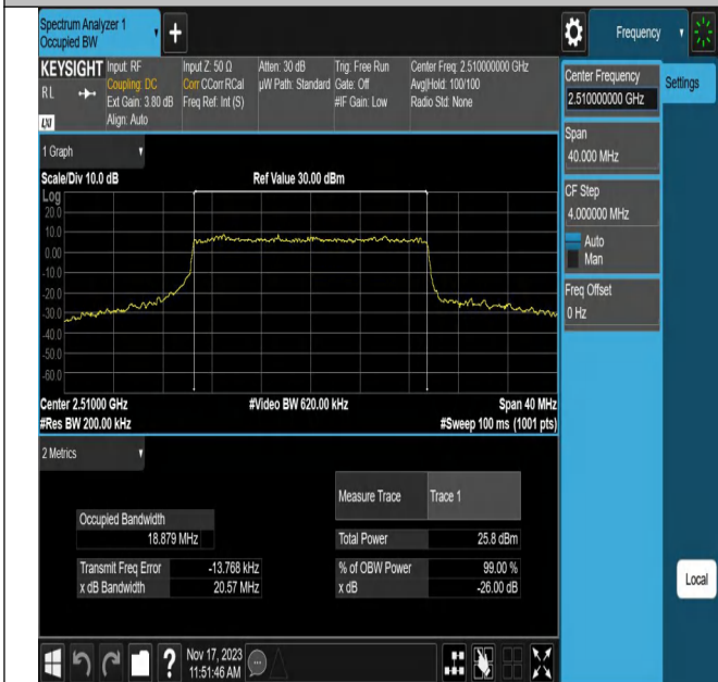
NTNV_N7_PC3_15_20_L_TID7_Ant1#1
