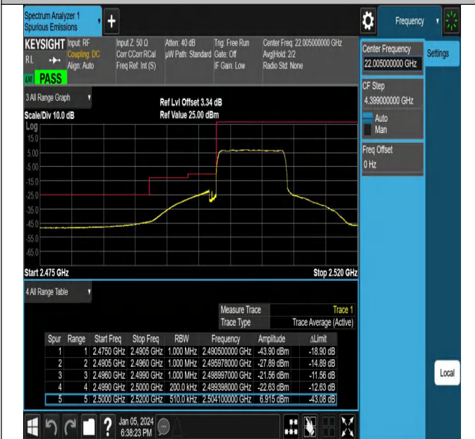
NTNV_N7_PC3_15_10_L_TID22_#1
