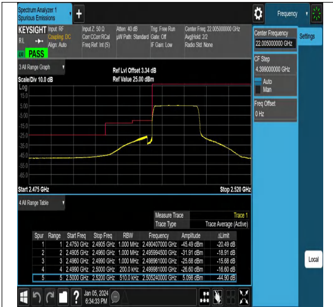
NTNV_N7_PC3_15_10_L_TID1_#1
