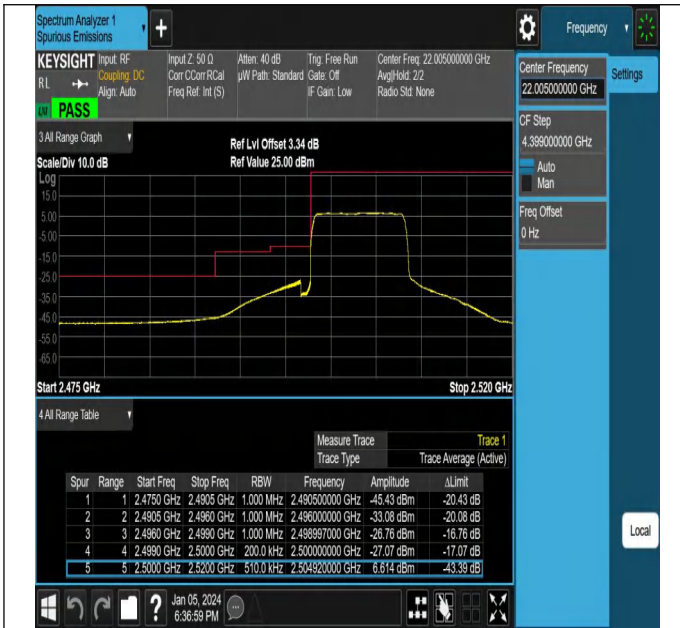
NTNV_N7_PC3_15_10_L_TID13_#1
