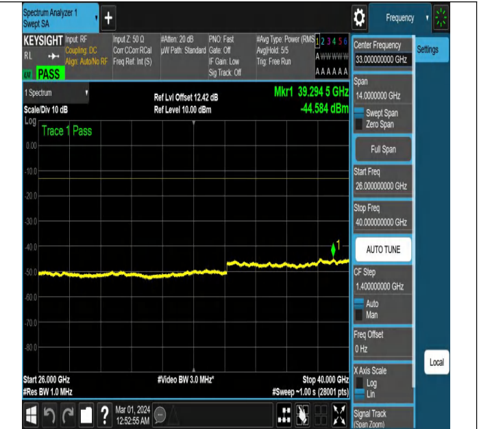
NTVN-N78-3450-3550-PC2-30-100-L-CP-QPSK-Edge_1RB_L
