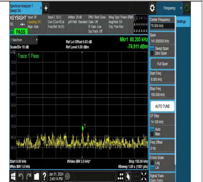
NTVN-N78-3450-3550-PC2-30-100-L-CP-QPSK-Edge_1RB_L eft-Ant2-PASS
