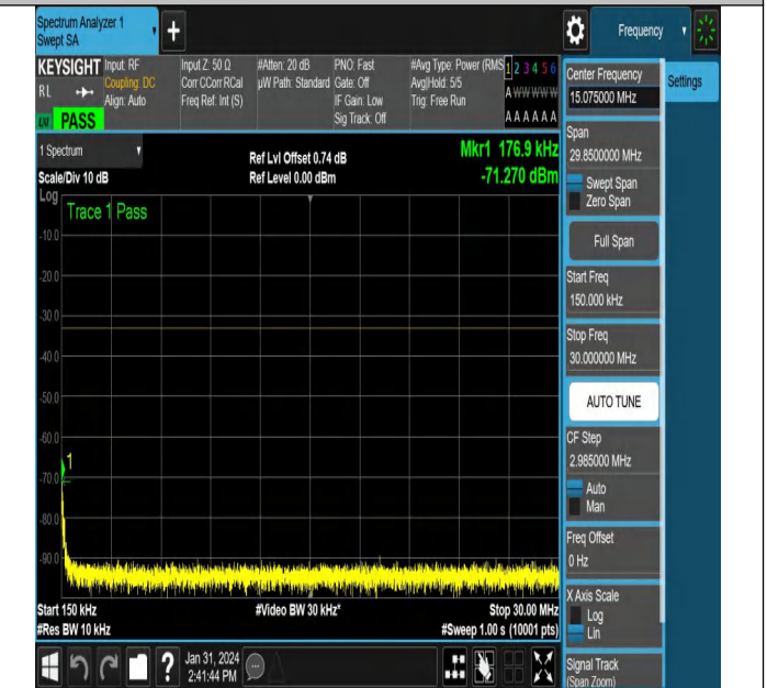
NTVN-N78-3450-3550-PC2-30-100-L-CP-QPSK-Edge_1RB_R
