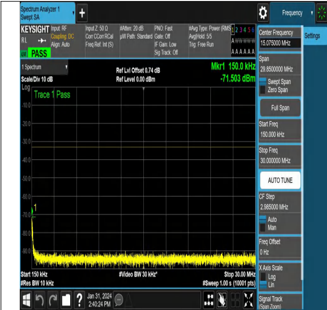
NTNV-N78-3450-3550-PC2-30-100-L-CP-QPSK-Edge_1RB_L
