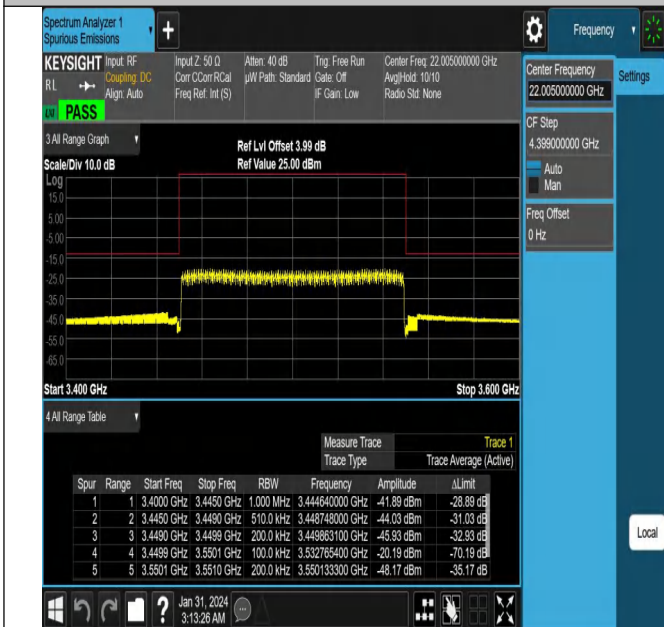
NTNV_N78-3450-3550_PC2_30_100_L_TID10_#1
