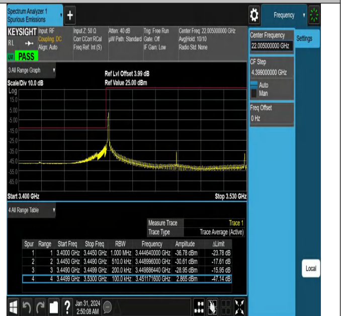
NTNV_N78-3450-3550_PC2_30_80_L_TID5_#1
