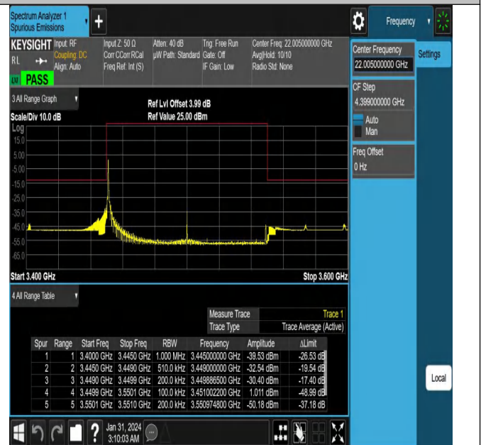
NTNV_N78-3450-3550_PC2_30_100_L_TID5_#1
