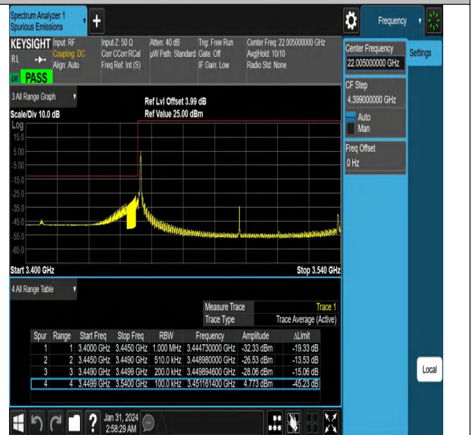
NTNV_N78-3450-3550_PC2_30_90_L_TID5_#1
