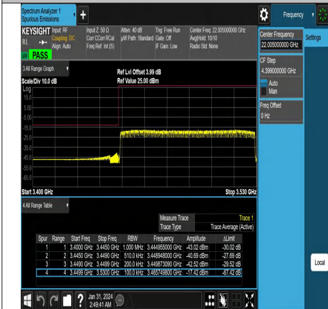
NTNV_N78-3450-3550_PC2_30_80_L_TID4_#1
