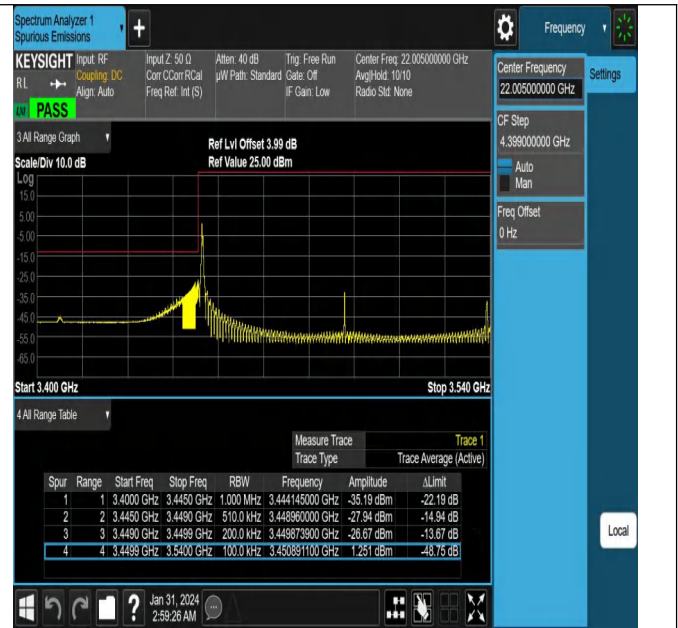
NTNV_N78-3450-3550_PC2_30_90_L_TID8_#1
