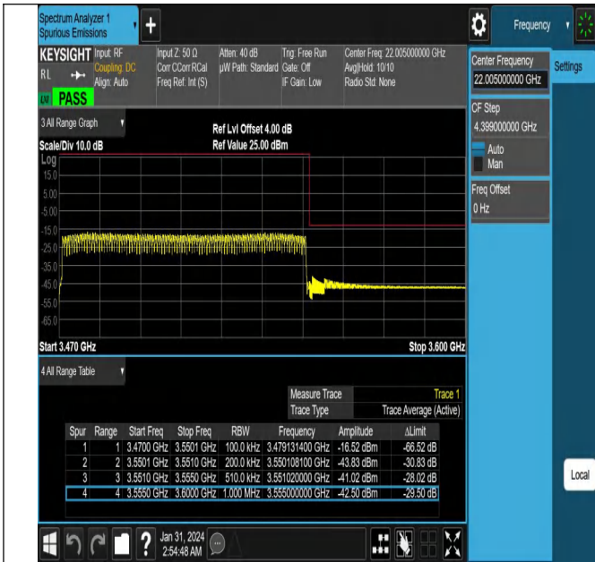
NTNV_N78-3450-3550_PC2_30_80_H_TID7_#1
