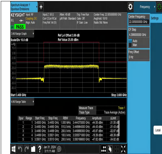
NTNV_N78-3450-3550_PC2_30_100_L_TID7_#1
