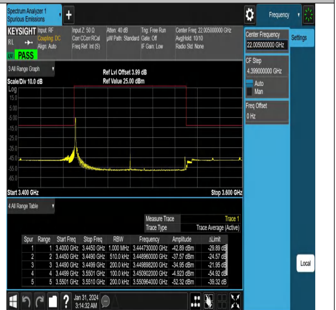
NTNV_N78-3450-3550_PC2_30_100_L_TID11_#1
