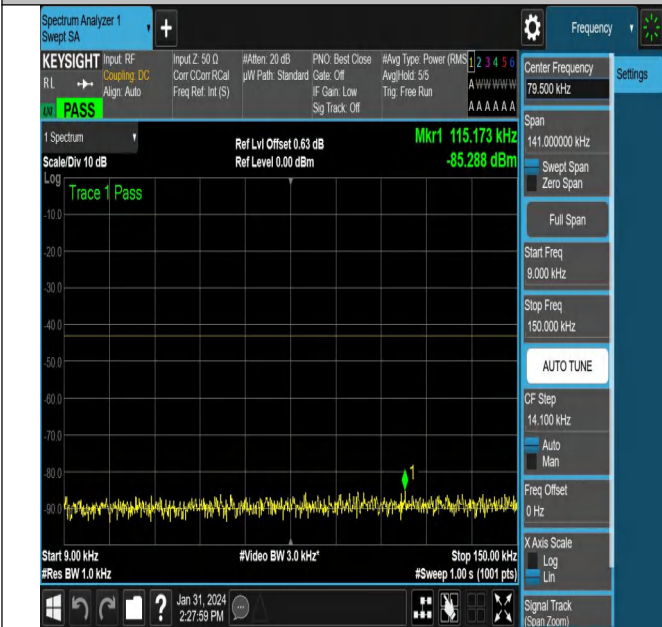
NTVN-N78-3450-3550-PC2-30-100-L-CP-QPSK-Edge_1RB_R
