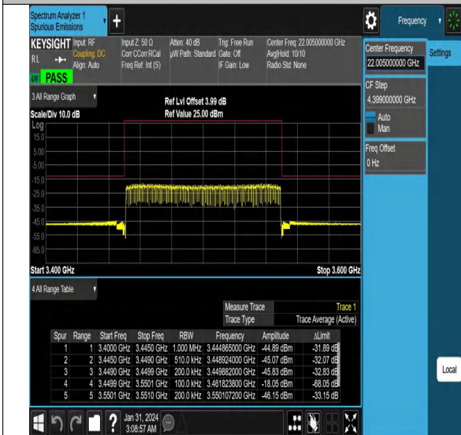
NTNV_N78-3450-3550_PC2_30_100_L_TID4_#1
