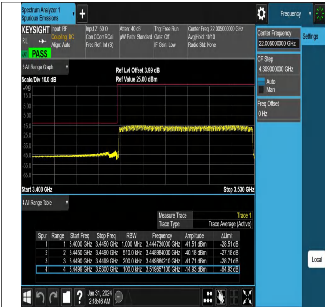
NTNV_N78-3450-3550_PC2_30_80_L_TID1_#1
