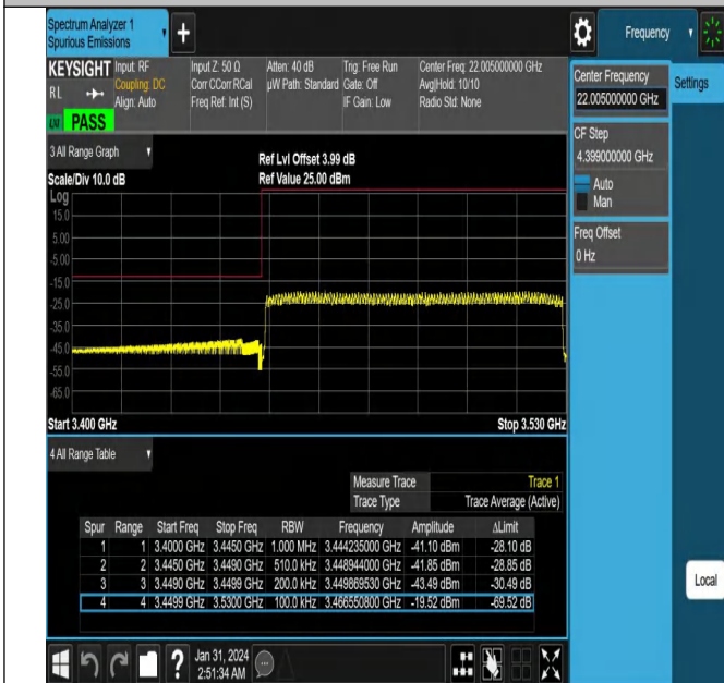
NTNV_N78-3450-3550_PC2_30_80_L_TID10_#1
