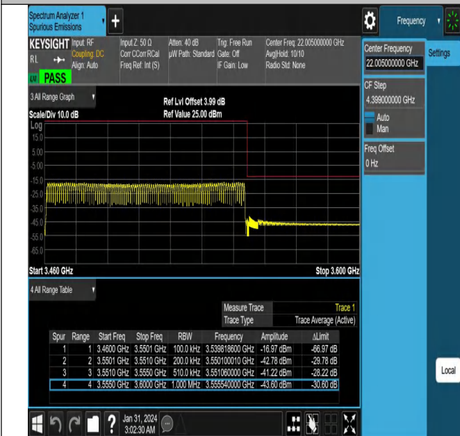
NTNV_N78-3450-3550_PC2_30_90_H_TID4_#1
