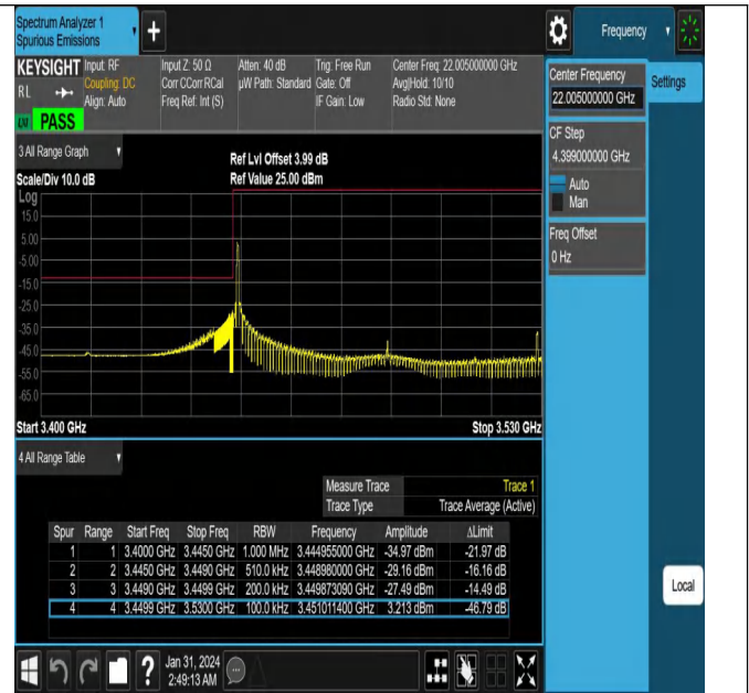
NTNV_N78-3450-3550_PC2_30_80_L_TID2_#1
