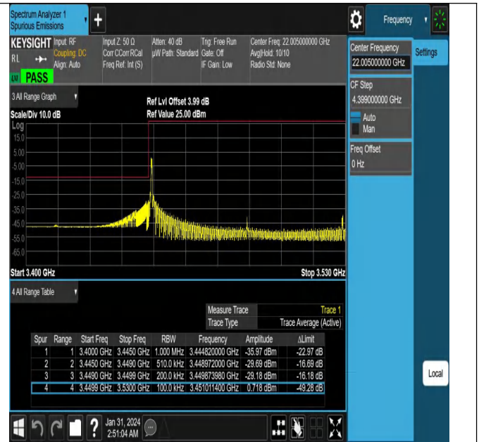
NTNV_N78-3450-3550_PC2_30_80_L_TID8_#1
