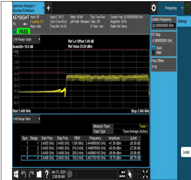
NTNV_N78-3450-3550_PC2_30_90_L_TID7_#1
