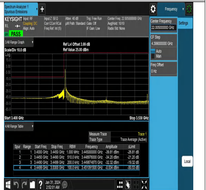
NTNV_N78-3450-3550_PC2_30_80_L_TID11_#1
