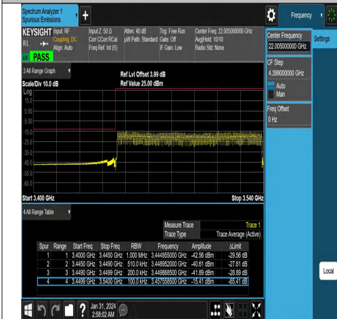
NTNV_N78-3450-3550_PC2_30_90_L_TID4_#1
