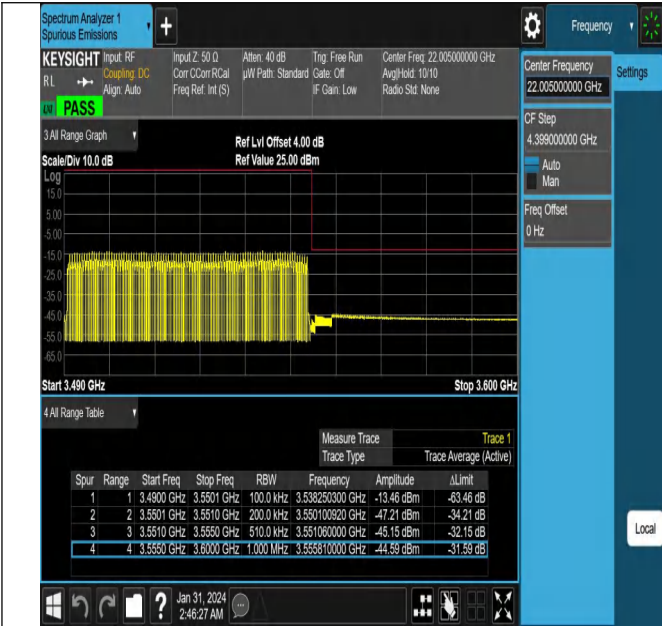
NTNV_N78-3450-3550_PC2_30_60_H_TID7_#1
