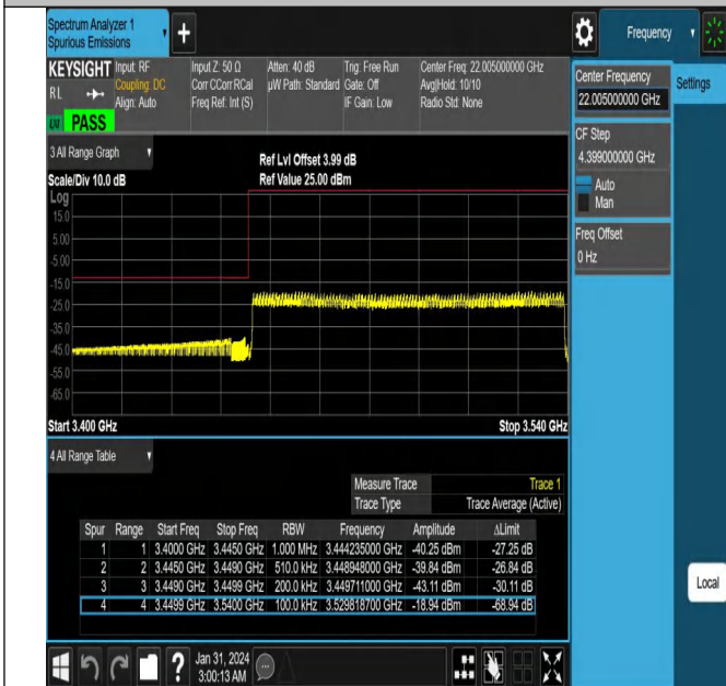
NTNV_N78-3450-3550_PC2_30_90_L_TID10_#1
