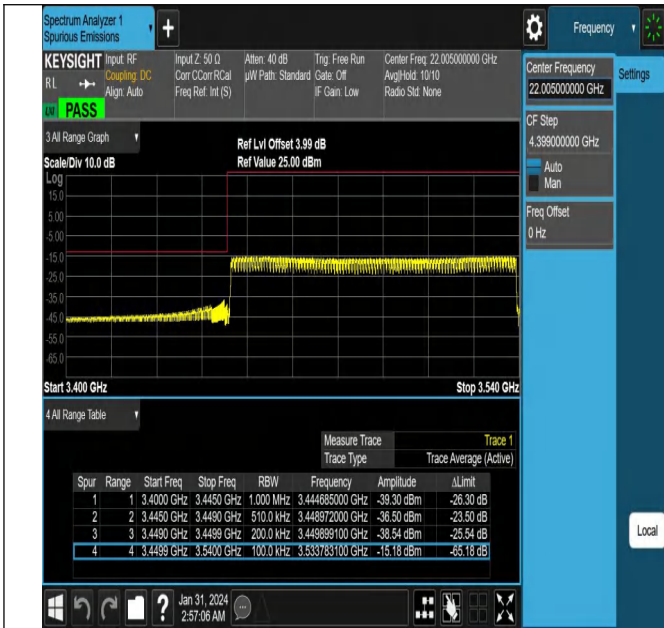
NTNV_N78-3450-3550_PC2_30_90_L_TID1_#1
