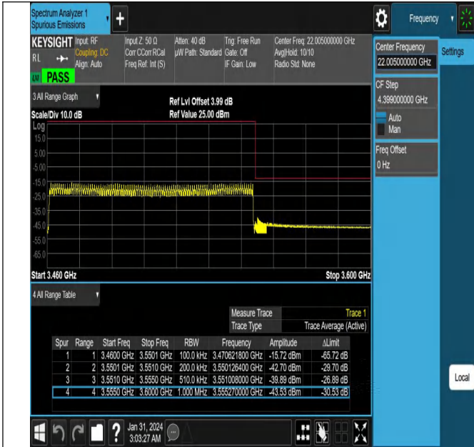
NTNV_N78-3450-3550_PC2_30_90_H_TID7_#1
