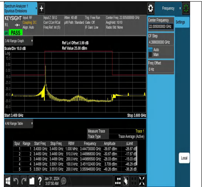
NTNV_N78-3450-3550_PC2_30_100_L_TID2_#1
