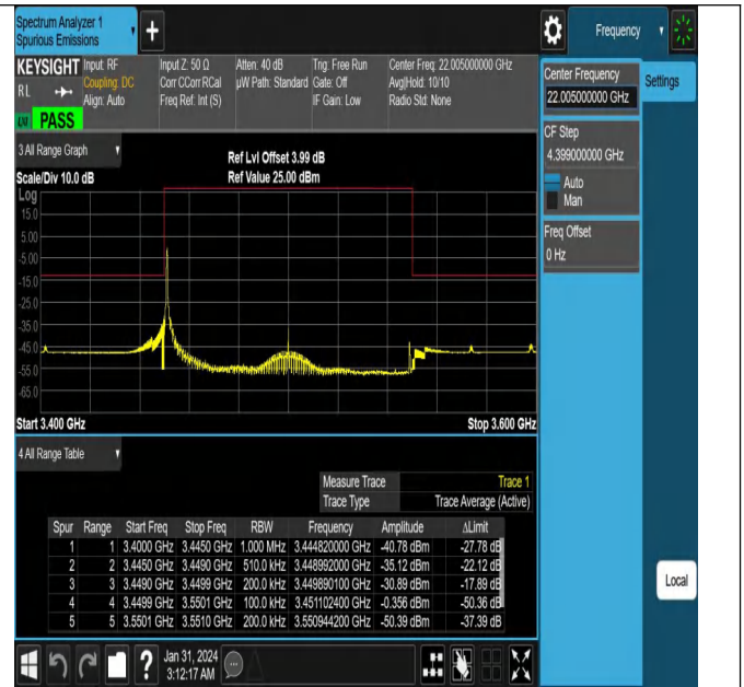
NTNV_N78-3450-3550_PC2_30_100_L_TID8_#1
