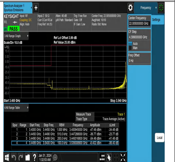
NTNV_N78-3450-3550_PC2_30_90_L_TID12_#1
