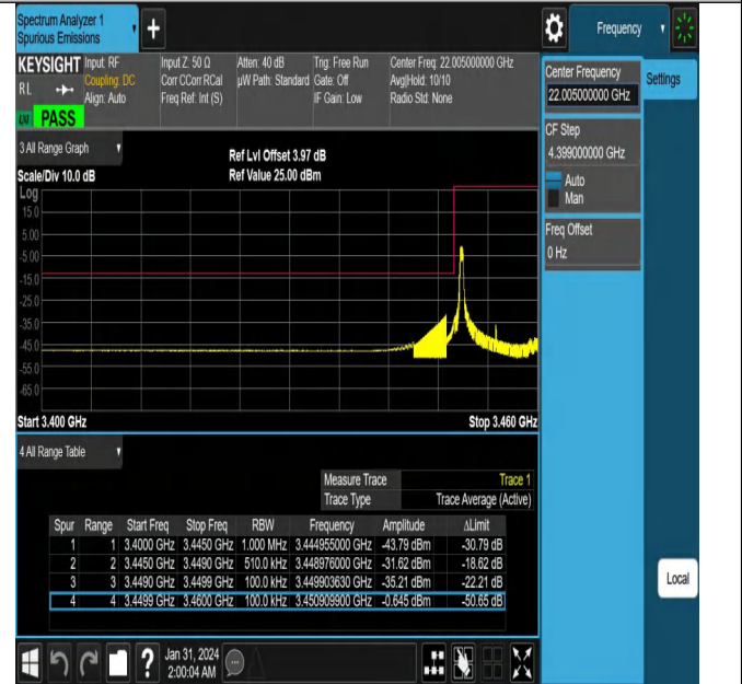
NTNV_N78-3450-3550_PC2_30_10_L_TID11_#1
