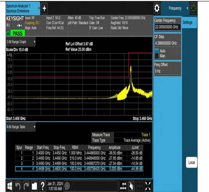
NTNV_N78-3450-3550_PC2_30_10_L_TID2_#1
