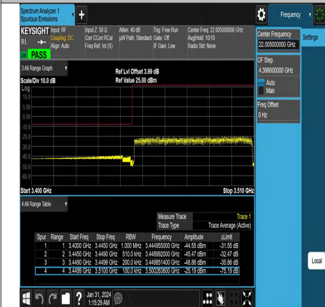
NTNV_N78-3450-3550_PC2_30_60_L_TID10_#1
