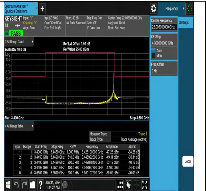
NTNV_N78-3450-3550_PC2_30_100_L_TID9_#1
