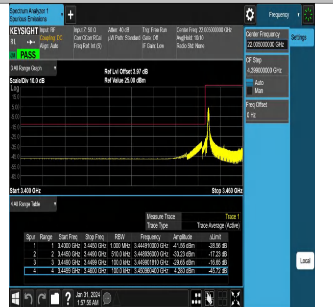
NTNV_N78-3450-3550_PC2_30_10_L_TID5_#1
