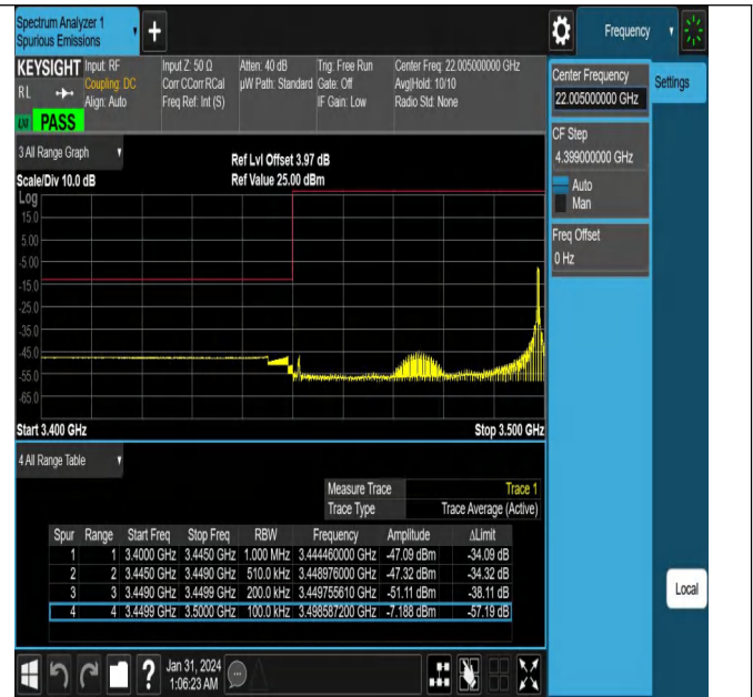
NTNV_N78-3450-3550_PC2_30_50_L_TID9_#1
