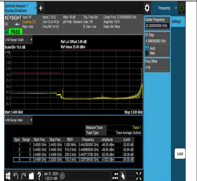
NTNV_N78-3450-3550_PC2_30_80_L_TID6_#1
