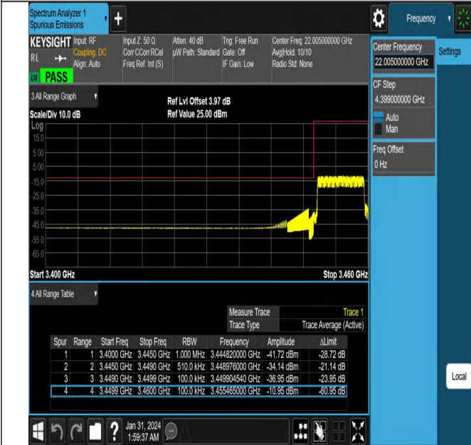
NTNV_N78-3450-3550_PC2_30_10_L_TID10_#1
