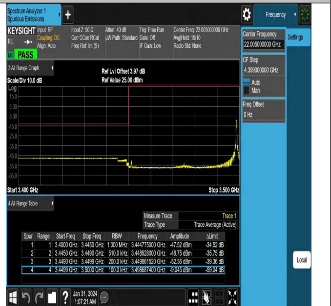
NTNV_N78-3450-3550_PC2_30_50_L_TID12_#1
