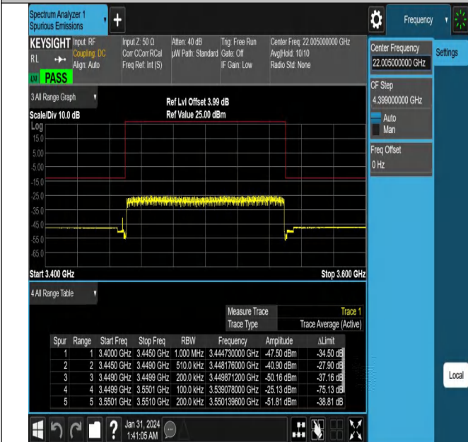
NTNV_N78-3450-3550_PC2_30_100_L_TID4_#1
