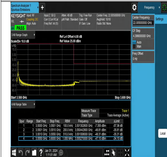
NTNV_N78-3450-3550_PC2_30_50_H_TID11_#1
