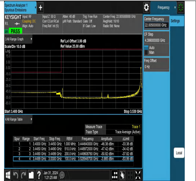
NTNV_N78-3450-3550_PC2_30_80_L_TID3_#1
