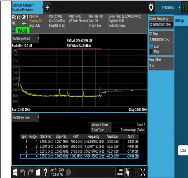
NTNV_N78-3450-3550_PC2_30_90_H_TID2_#1
