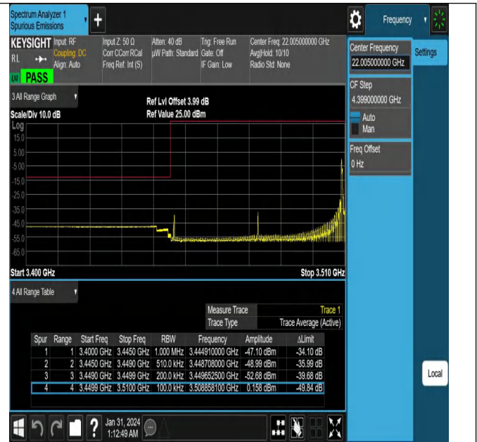
NTNV_N78-3450-3550_PC2_30_60_L_TID3_#1
