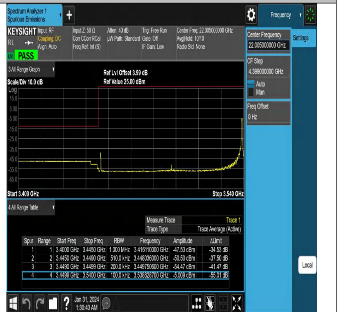
NTNV_N78-3450-3550_PC2_30_90_L_TID6_#1
