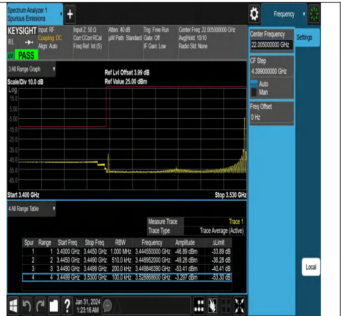
NTNV_N78-3450-3550_PC2_30_80_L_TID9_#1
