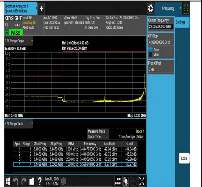
NTNV_N78-3450-3550_PC2_30_80_L_TID12_#1
