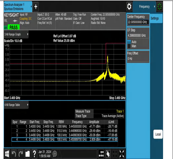
NTNV_N78-3450-3550_PC2_30_10_L_TID8_#1
