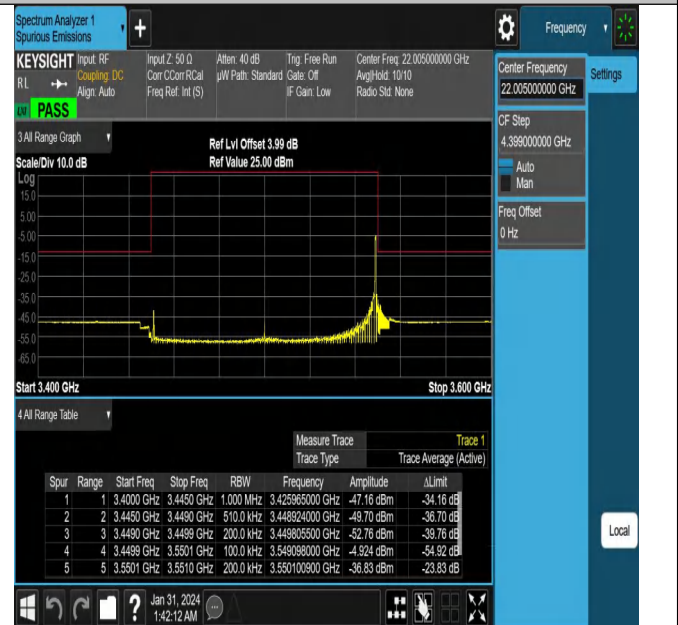
NTNV_N78-3450-3550_PC2_30_100_L_TID6_#1
