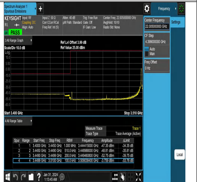
NTNV_N78-3450-3550_PC2_30_60_L_TID6_#1
