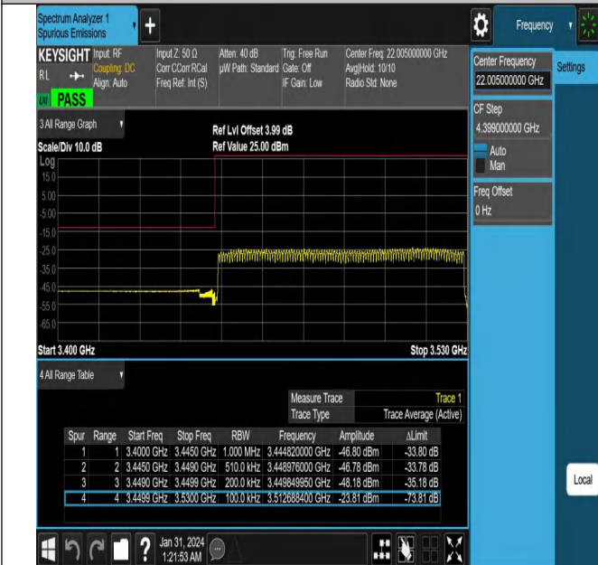
NTNV_N78-3450-3550_PC2_30_80_L_TID4_#1
