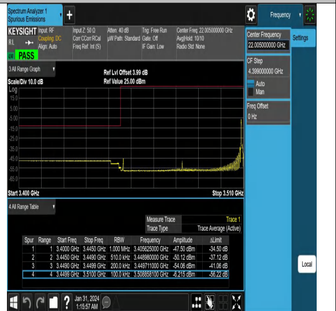
NTNV_N78-3450-3550_PC2_30_60_L_TID12_#1
