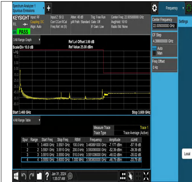
NTNV_N78-3450-3550_PC2_30_90_H_TID8_#1
