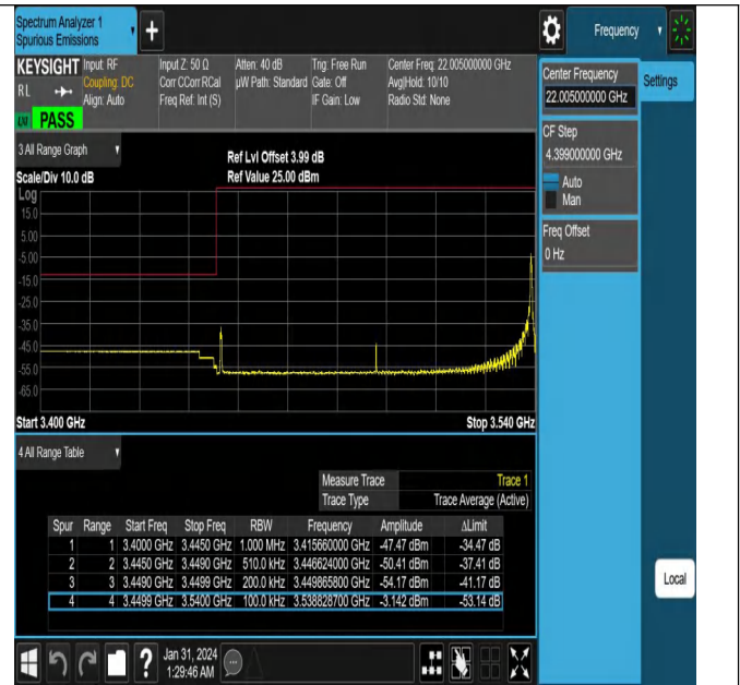
NTNV_N78-3450-3550_PC2_30_90_L_TID3_#1
