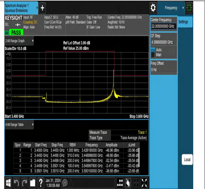
NTNV_N78-3450-3550_PC2_30_100_L_TID3_#1
