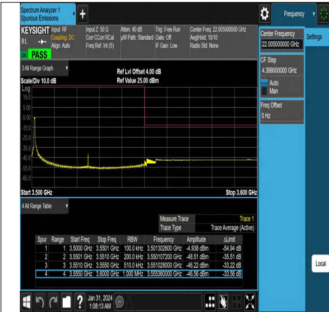
NTNV_N78-3450-3550_PC2_30_50_H_TID2_#1
