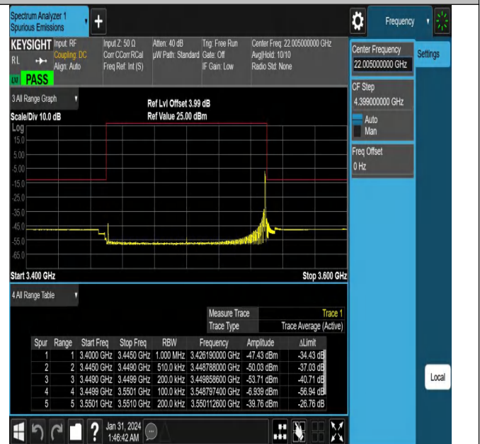
NTNV_N78-3450-3550_PC2_30_100_L_TID12_#1
