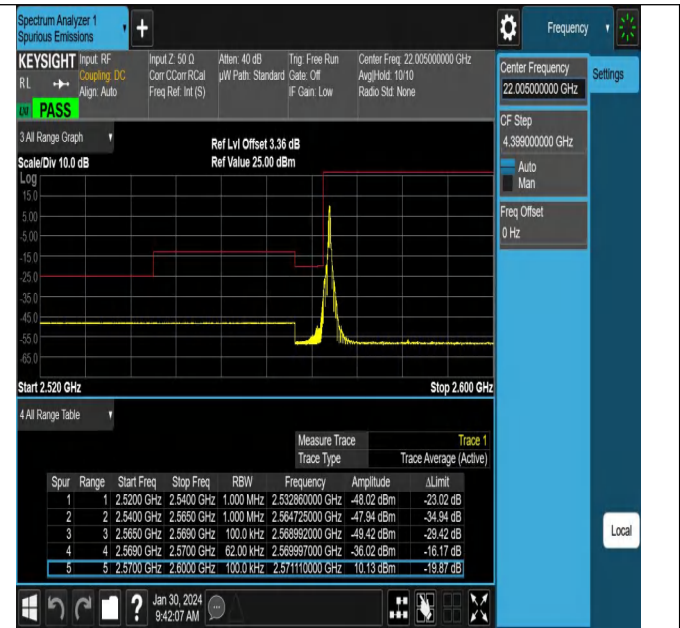
NTNV_N38_PC3_30_30_L_TID2_#1
