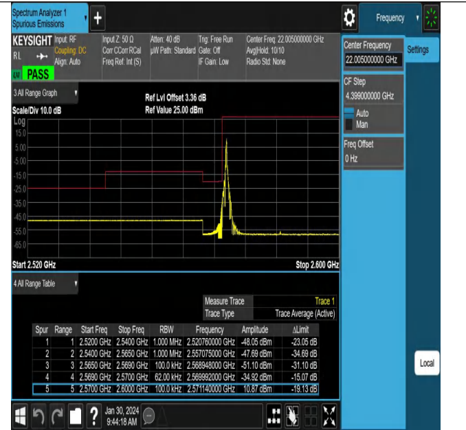
NTNV_N38_PC3_30_30_L_TID8_#1
