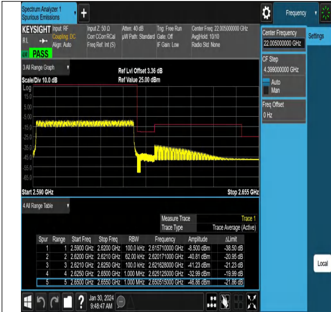
NTNV_N38_PC3_30_30_H_TID7_#1
