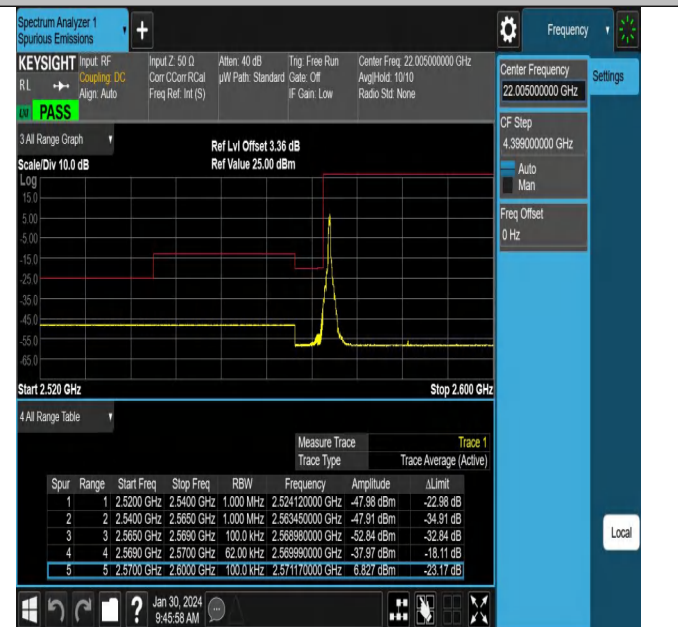
NTNV_N38_PC3_30_30_L_TID11_#1
