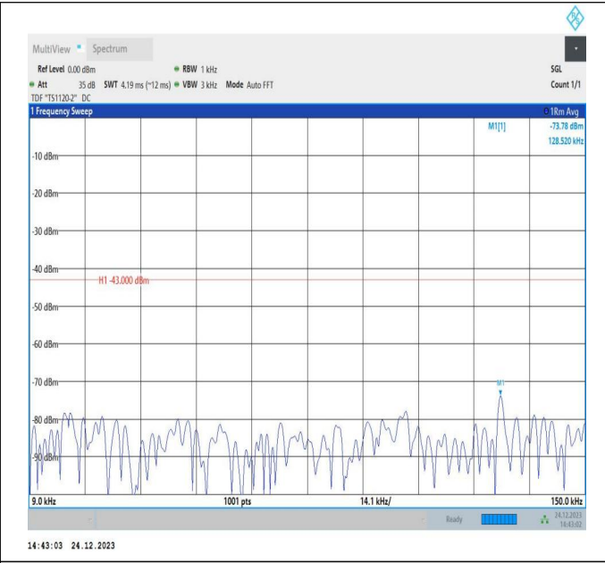
66-66-20MHz-20MHz-QPSK-QPSK-132323-132521-1RB#0-1RB#99-0.009~0.15MHz-PASS
