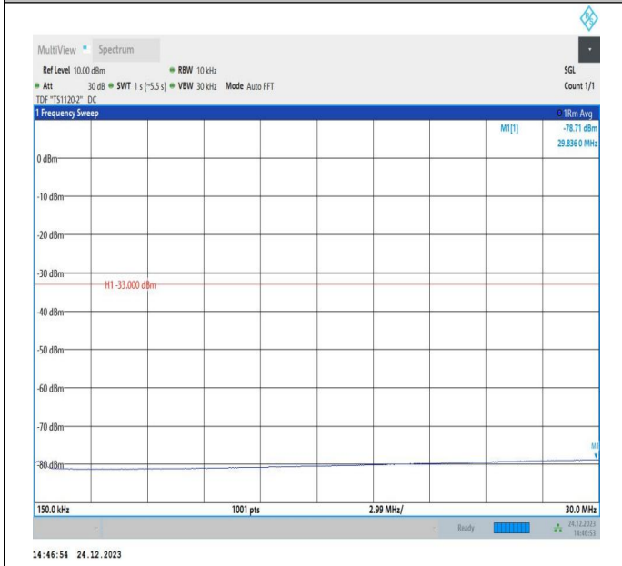
66-66-20MHz-20MHz-QPSK-QPSK-132374-132572-1RB#0-1RB#99-0.15~30MHz-PASS
