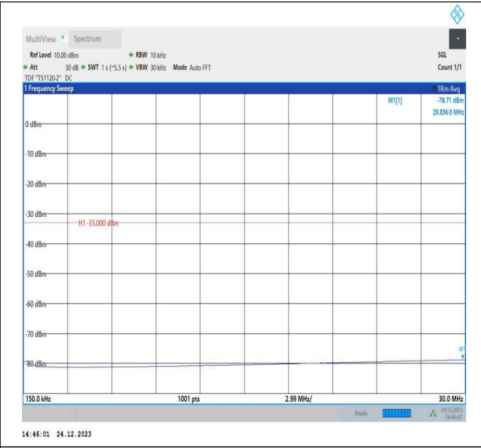
66-66-20MHz-20MHz-QPSK-QPSK-132374-132572-1RB#99 -ORB#0-0.15~30MHz-PASS
