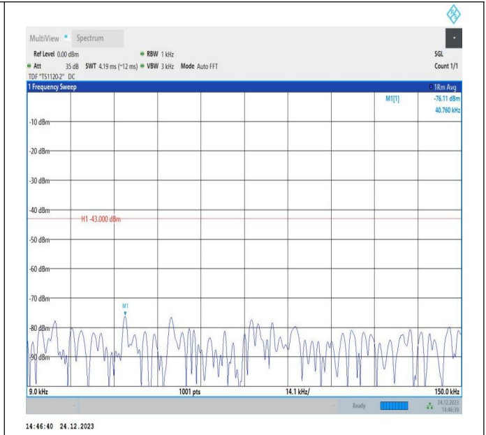
66-66-20MHz-20MHz-QPSK-QPSK-132374-132572-1RB#0-1RB#99-0.009~0.15MHz-PASS
