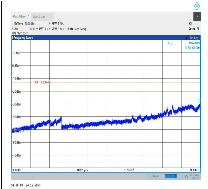
66-66-20MHz-20MHz-QPSK-QPSK-132374-132572-1RB#99-0RB#0-3000~20000MHz-PASS
