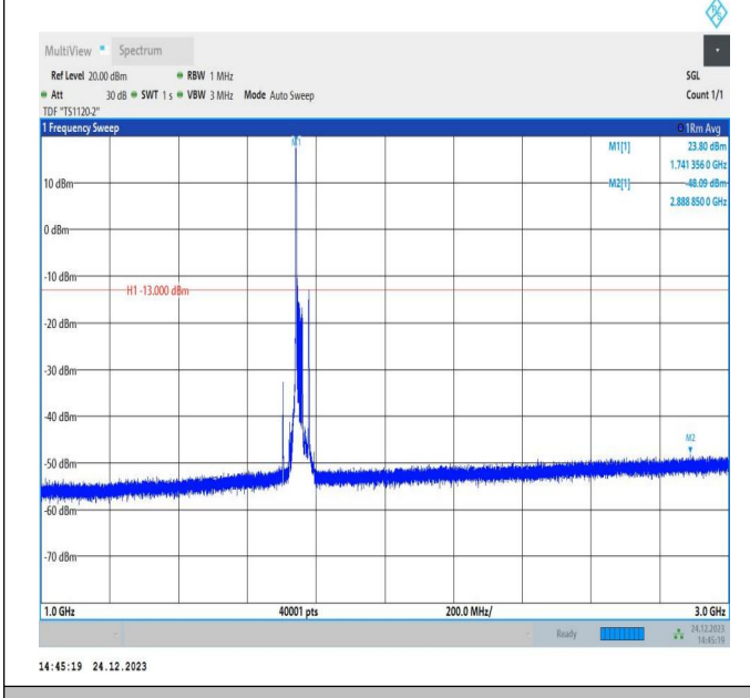
66-66-20MHz-20MHz-QPSK-QPSK-132374-132572-1RB#0-ORB#0-1000~3000MHz-PASS
