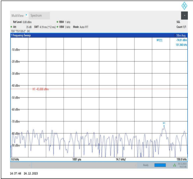
66-66-20MHz-20MHz-QPSK-QPSK-132072-132270-1RB#99 -ORB#0-0.009~0.15MHz-PASS
