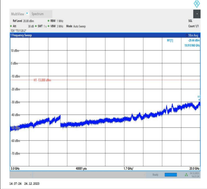
66-66-20MHz-20MHz-QPSK-QPSK-132072-132270-1RB#0-ORB#0-3000~20000MHz-PASS
