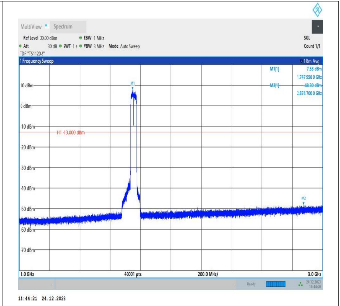
66-66-20MHz-20MHz-QPSK-QPSK-132323-132521-100RB# 0-100RB#0-1000~3000MHz-PASS
