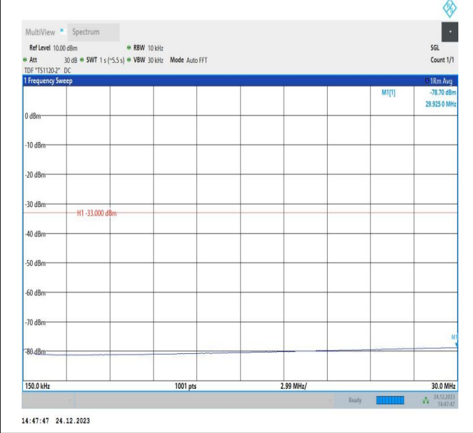
66-66-20MHz-20MHz-QPSK-QPSK-132374-132572-100RB#0-100RB#0-0.15~30MHz-PASS
