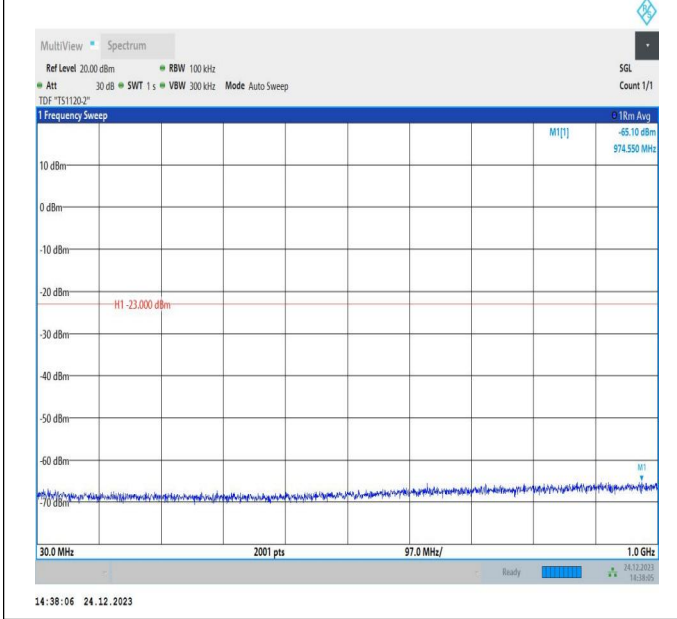
66-66-20MHz-20MHz-QPSK-QPSK-132072-132270-1RB#99 -ORB#0-30~1000MHz-PASS
