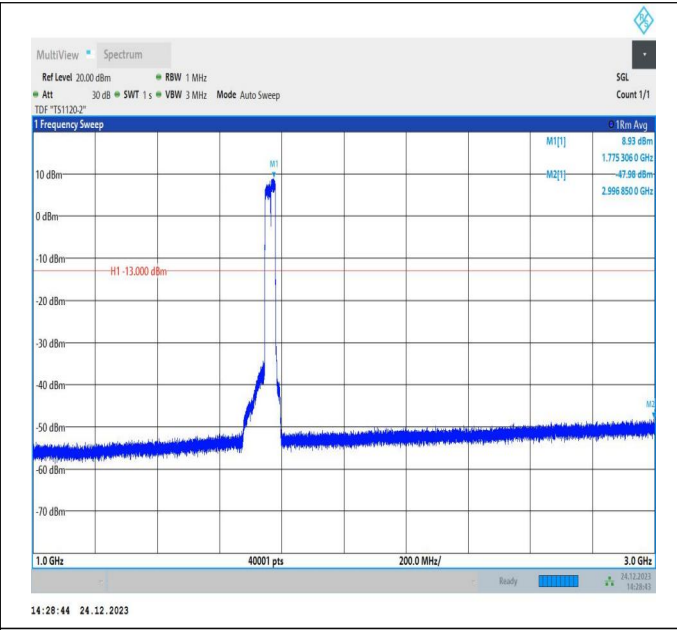
66-66-20MHz-15MHz-QPSK-QPSK-132423-132594-100RB# 0-75RB#0-1000~3000MHz-PASS
