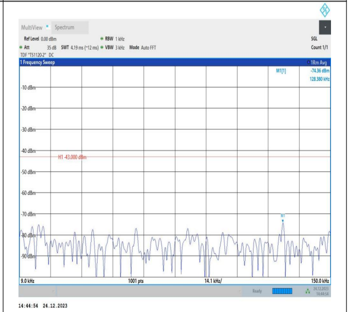
66-66-20MHz-20MHz-QPSK-QPSK-132374-132572-1RB#0- 0RB#0-0.009~0.15MHz-PASS
