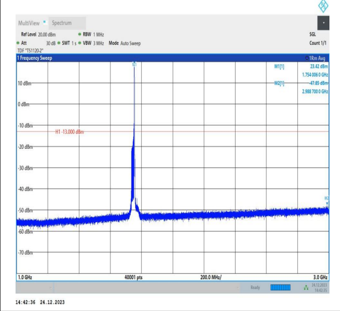
66-66-20MHz-20MHz-QPSK-QPSK-132323-132521-1RB#99 -ORB#0-1000~3000MHz-PASS
