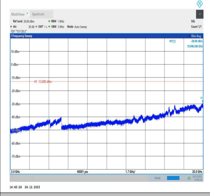
66-66-20MHz-20MHz-QPSK-QPSK-132374-132572-1RB#0-ORB#0-3000~20000MHz-PASS
