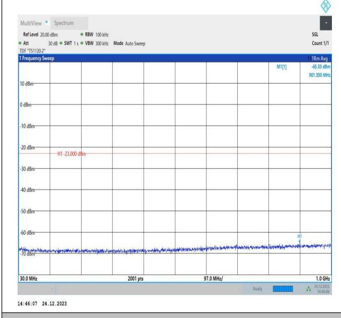
66-66-20MHz-20MHz-QPSK-QPSK-132374-132572-1RB#99 -ORB#0-30~1000MHz-PASS
