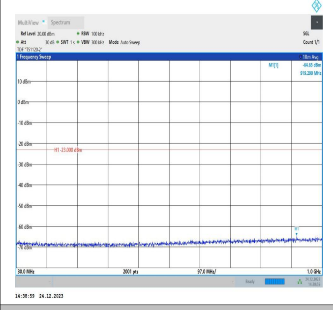
66-66-20MHz-20MHz-QPSK-QPSK-132072-132270-1RB#0-1RB#99-30~1000MHz-PASS
