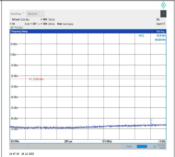
66-66-20MHz-20MHz-QPSK-QPSK-132374-132572-1RB#0-1RB#99-30~1000MHz-PASS
