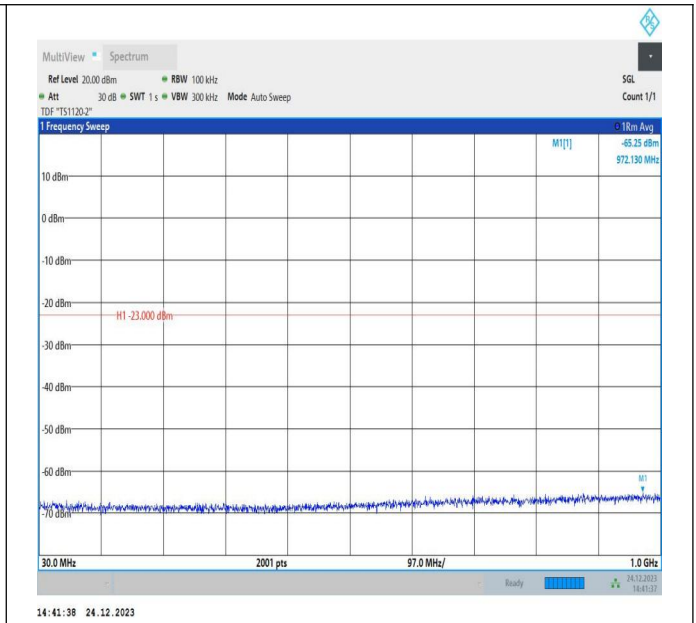
66-66-20MHz-20MHz-QPSK-QPSK-132323-132521-1RB#0-ORB#0-30~1000MHz-PASS
