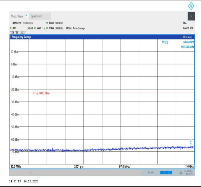
66-66-20MHz-20MHz-QPSK-QPSK-132072-132270-1RB#0-ORB#0-30~1000MHz-PASS
