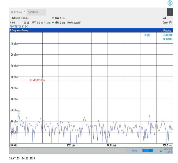
66-66-20MHz-20MHz-QPSK-QPSK-132374-132572-100RB#0-100RB#0-0.009~0.15MHz-PASS
