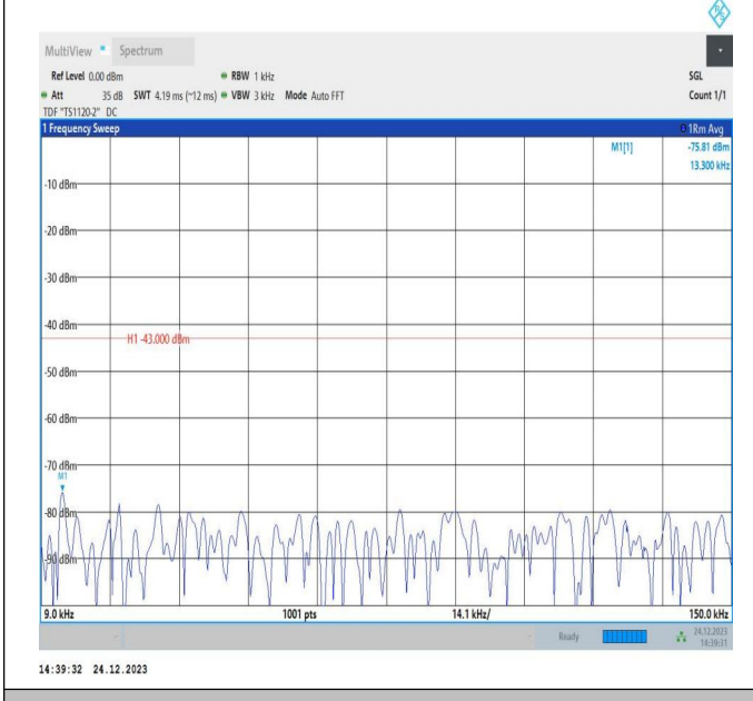
66-66-20MHz-20MHz-QPSK-QPSK-132072-132270-100RB#0-100RB#0-0.009~0.15MHz-PASS
