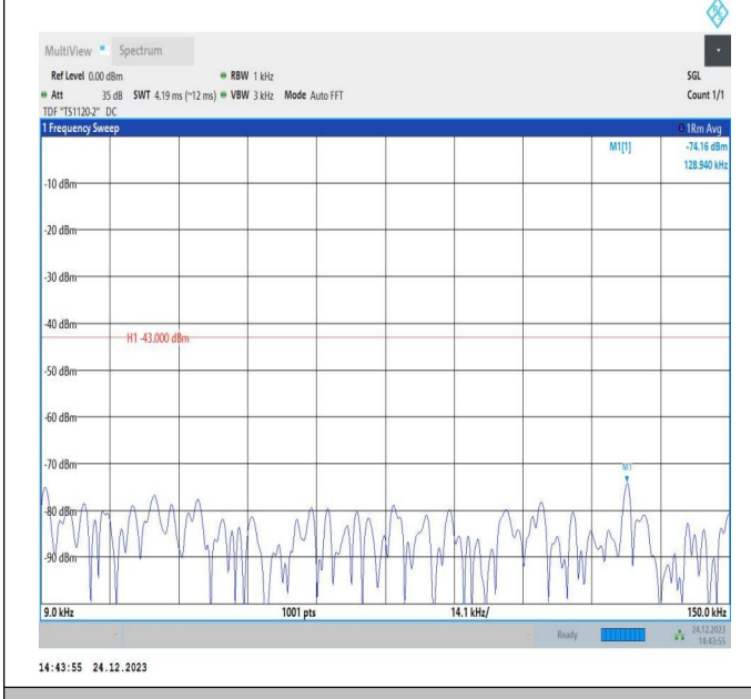
66-66-20MHz-20MHz-QPSK-QPSK-132323-132521-100RB#0-100RB#0-0.009~0.15MHz-PASS
