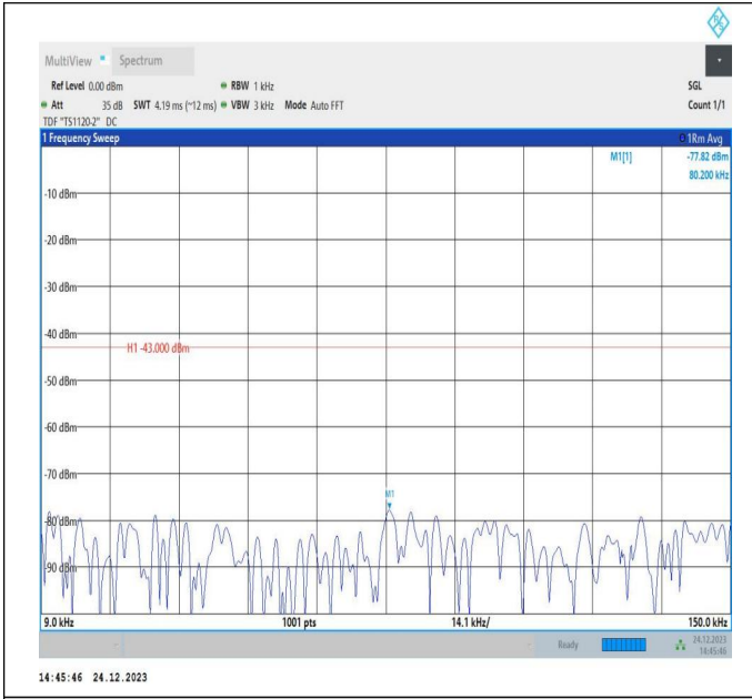
66-66-20MHz-20MHz-QPSK-QPSK-132374-132572-1RB#99 -ORB#0-0.009~0.15MHz-PASS
