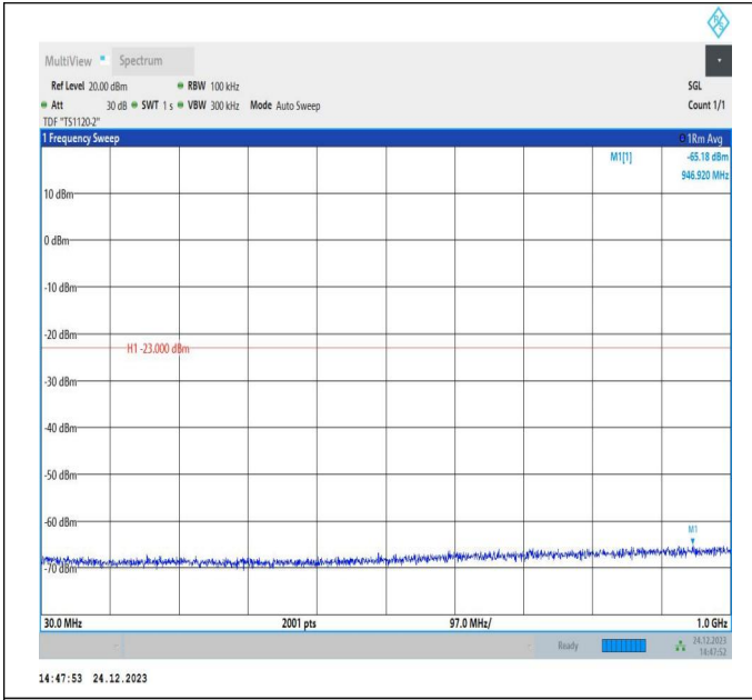
66-66-20MHz-20MHz-QPSK-QPSK-132374-132572-100RB# 0-100RB#0-30~1000MHz-PASS
