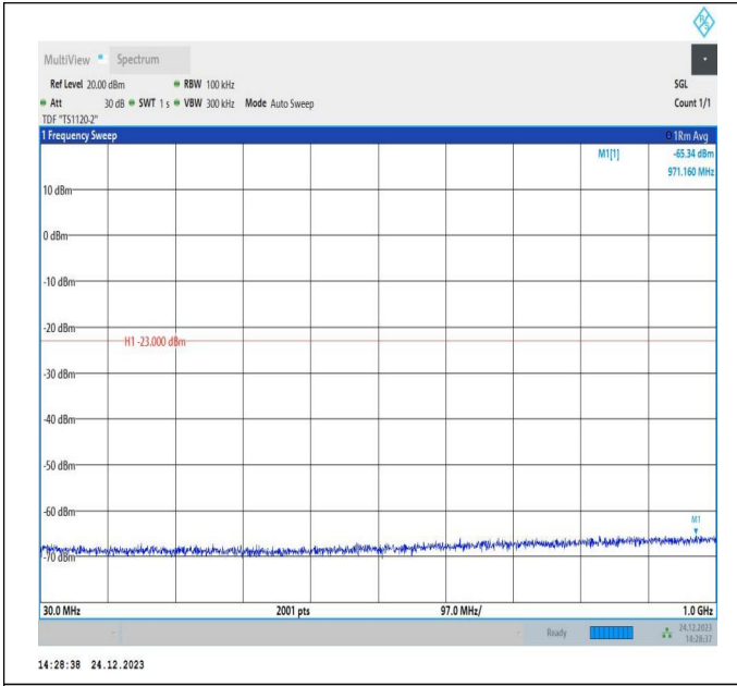
66-66-20MHz-15MHz-QPSK-QPSK-132423-132594-100RB# 0-75RB#0-30~1000MHz-PASS
