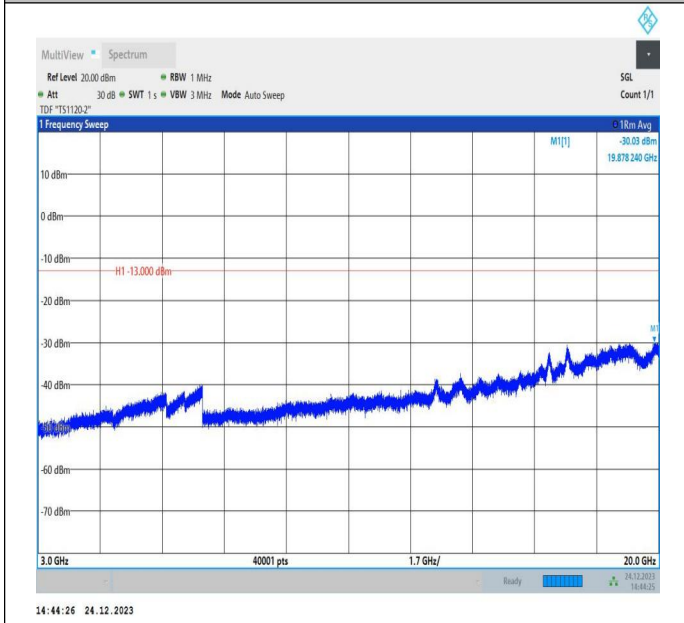
66-66-20MHz-20MHz-QPSK-QPSK-132323-132521-100RB# 0-100RB#0-3000~20000MHz-PASS
