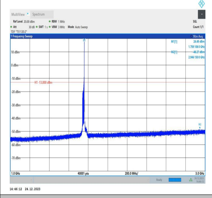
66-66-20MHz-20MHz-QPSK-QPSK-132374-132572-1RB#99 -ORB#0-1000~3000MHz-PASS
