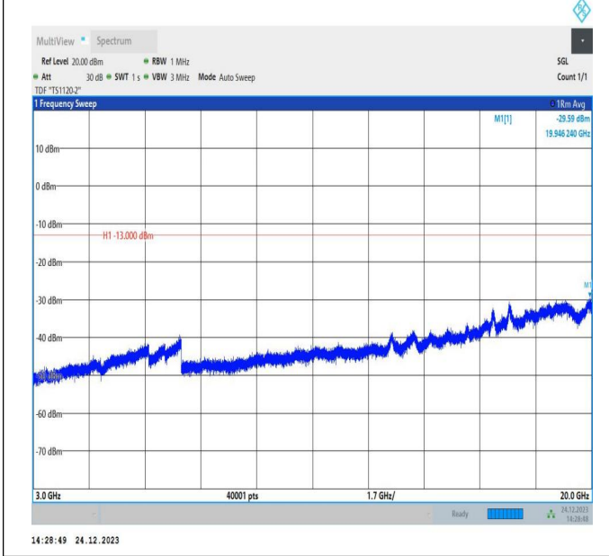
66-66-20MHz-15MHz-QPSK-QPSK-132423-132594-100RB# 0-75RB#0-3000~20000MHz-PASS
