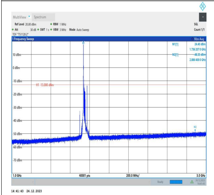
66-66-20MHz-20MHz-QPSK-QPSK-132323-132521-1RB#0-ORB#0-1000~3000MHz-PASS
