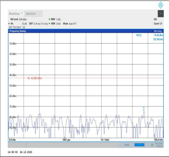
66-66-20MHz-20MHz-QPSK-QPSK-132072-132270-1RB#0-1RB#99-0.009~0.15MHz-PASS
