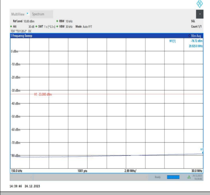
66-66-20MHz-20MHz-QPSK-QPSK-132072-132270-100RB#0-100RB#0-0.15~30MHz-PASS
