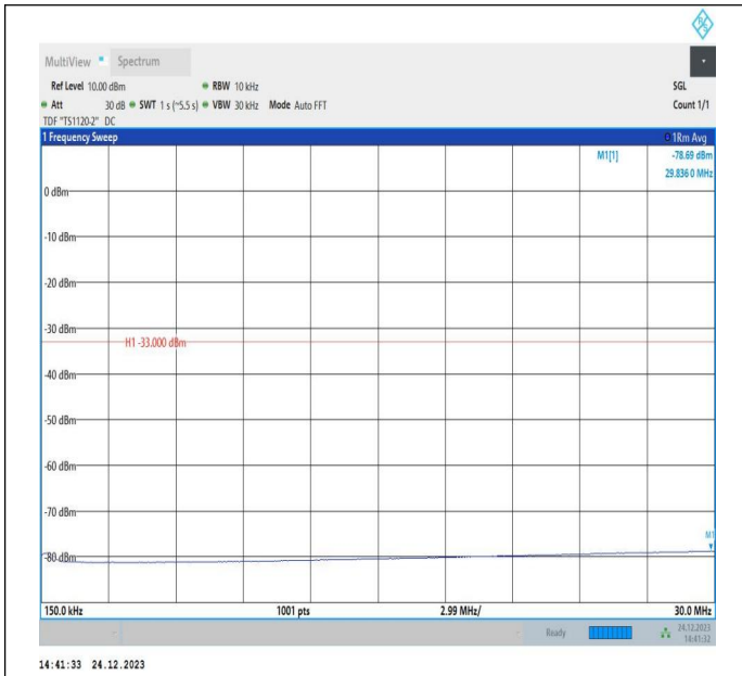
66-66-20MHz-20MHz-QPSK-QPSK-132323-132521-1RB#0-ORB#0-0.15~30MHz-PASS
