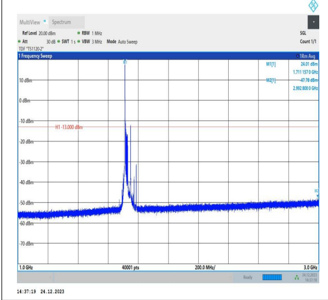
66-66-20MHz-20MHz-QPSK-QPSK-132072-132270-1RB#0-ORB#0-1000~3000MHz-PASS
