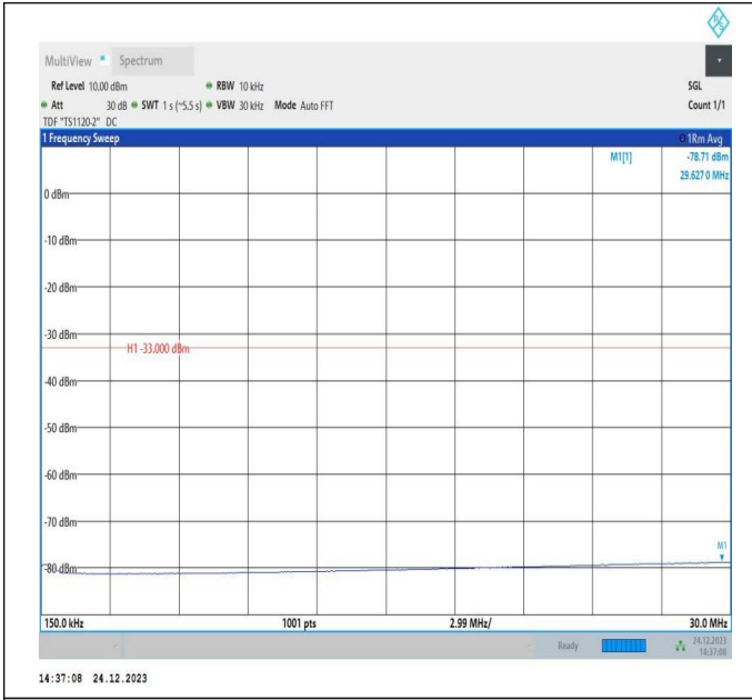
66-66-20MHz-20MHz-QPSK-QPSK-132072-132270-1RB#0-ORB#0-0.15~30MHz-PASS
