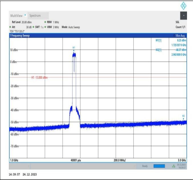
66-66-20MHz-20MHz-QPSK-QPSK-132072-132270-100RB# 0-100RB#0-1000~3000MHz-PASS
