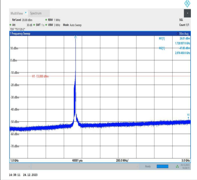
66-66-20MHz-20MHz-QPSK-QPSK-132072-132270-1RB#99 -ORB#0-1000~3000MHz-PASS
