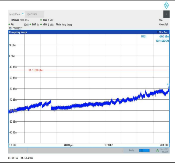
66-66-20MHz-20MHz-QPSK-QPSK-132072-132270-1RB#0-1RB#99-3000~20000MHz-PASS
