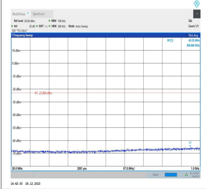
66-66-20MHz-20MHz-QPSK-QPSK-132323-132521-1RB#99 -ORB#0-30~1000MHz-PASS
