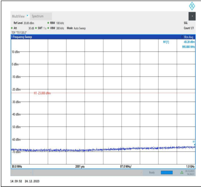
66-66-20MHz-20MHz-QPSK-QPSK-132072-132270-100RB# 0-100RB#0-30~1000MHz-PASS
