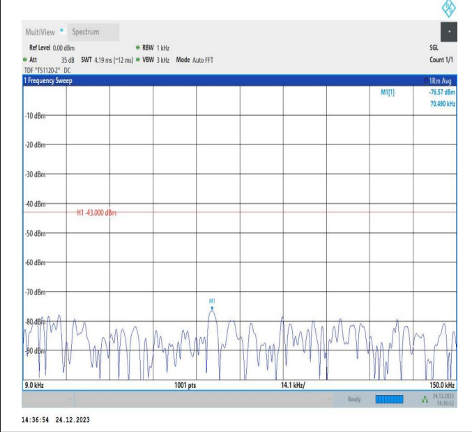
66-66-20MHz-20MHz-QPSK-QPSK-132072-132270-1RB#0- 0RB#0-0.009~0.15MHz-PASS
