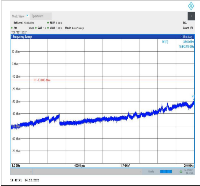
66-66-20MHz-20MHz-QPSK-QPSK-132323-132521-1RB#99-0RB#0-3000~20000MHz-PASS
