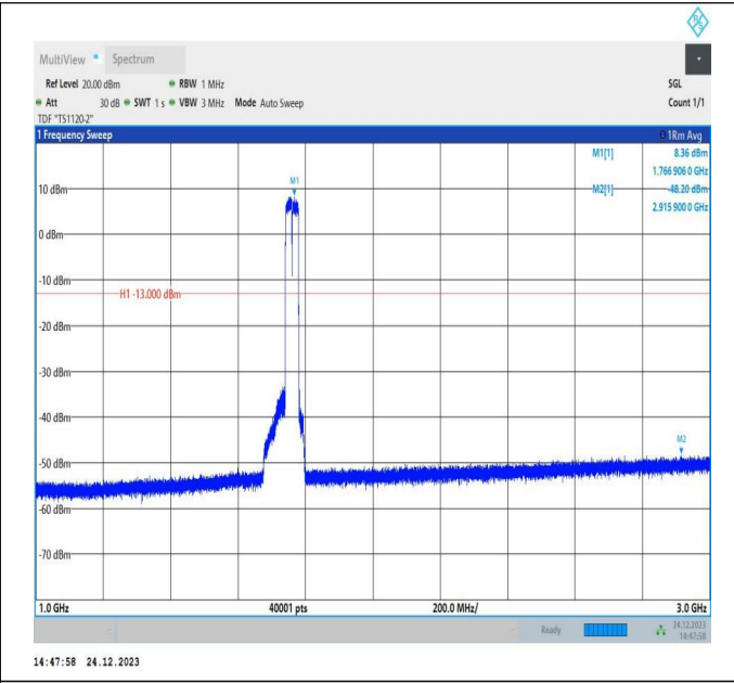
66-66-20MHz-20MHz-QPSK-QPSK-132374-132572-100RB# 0-100RB#0-1000~3000MHz-PASS
