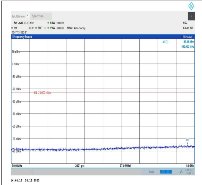
66-66-20MHz-20MHz-QPSK-QPSK-132323-132521-100RB# 0-100RB#0-30~1000MHz-PASS
