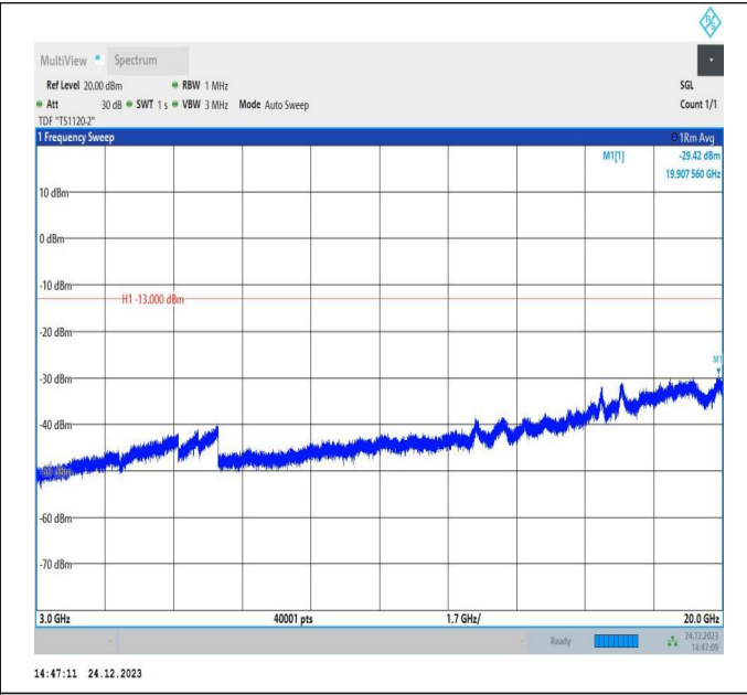
66-66-20MHz-20MHz-QPSK-QPSK-132374-132572-1RB#0-1RB#99-3000~20000MHz-PASS
