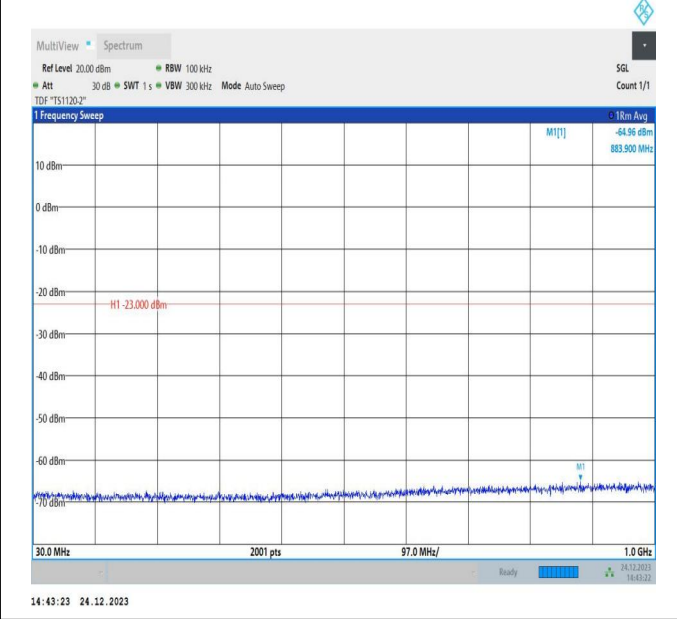
66-66-20MHz-20MHz-QPSK-QPSK-132323-132521-1RB#0-1RB#99-30~1000MHz-PASS
