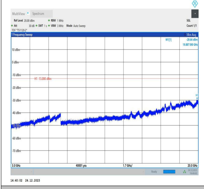
66-66-20MHz-20MHz-QPSK-QPSK-132072-132270-100RB# 0-100RB#0-3000~20000MHz-PASS
