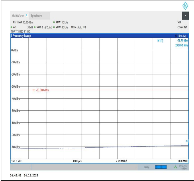
66-66-20MHz-20MHz-QPSK-QPSK-132374-132572-1RB#0-ORB#0-0.15~30MHz-PASS
