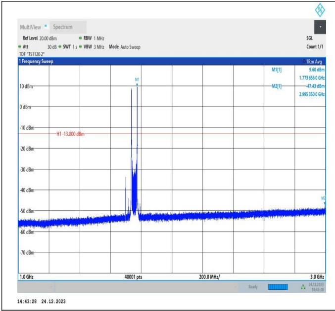
66-66-20MHz-20MHz-QPSK-QPSK-132323-132521-1RB#0-1RB#99-1000~3000MHz-PASS
