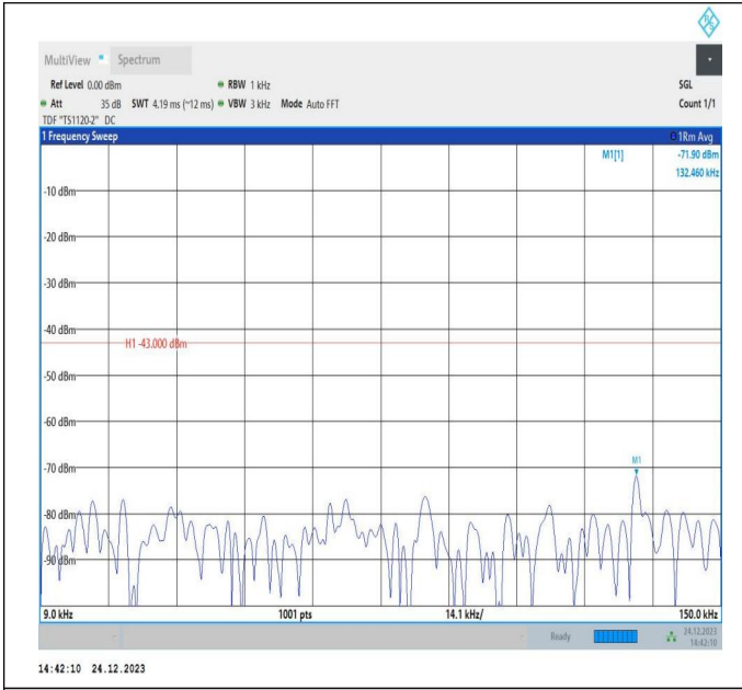
66-66-20MHz-20MHz-QPSK-QPSK-132323-132521-1RB#99 -ORB#0-0.009~0.15MHz-PASS
