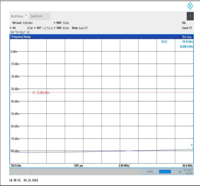
66-66-20MHz-20MHz-QPSK-QPSK-132072-132270-1RB#99 -ORB#0-0.15~30MHz-PASS
