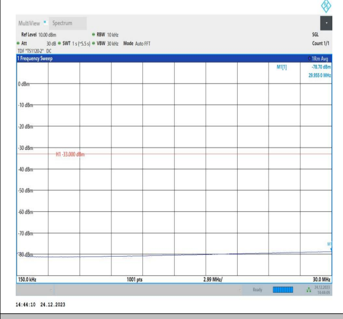
66-66-20MHz-20MHz-QPSK-QPSK-132323-132521-100RB#0-100RB#0-0.15~30MHz-PASS
