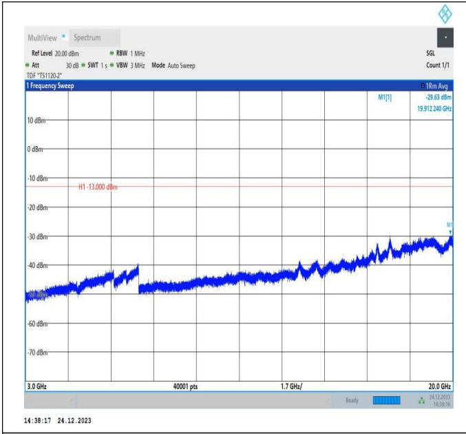
66-66-20MHz-20MHz-QPSK-QPSK-132072-132270-1RB#99-0RB#0-3000~20000MHz-PASS
