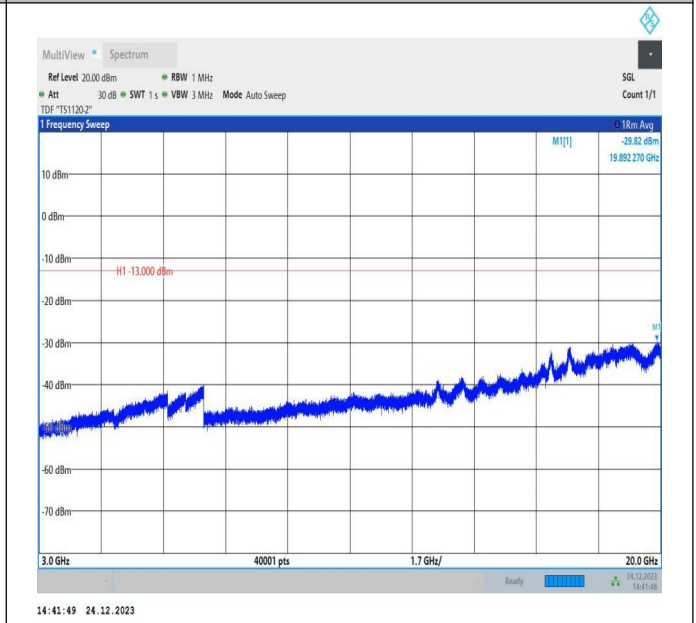
66-66-20MHz-20MHz-QPSK-QPSK-132323-132521-1RB#0-ORB#0-3000~20000MHz-PASS
