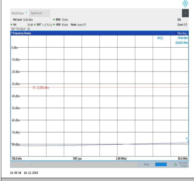
66-66-20MHz-20MHz-QPSK-QPSK-132072-132270-1RB#0-1RB#99-0.15~30MHz-PASS
