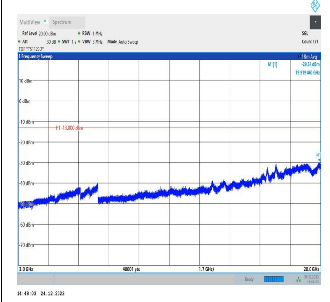
66-66-20MHz-20MHz-QPSK-QPSK-132374-132572-100RB# 0-100RB#0-3000~20000MHz-PASS
