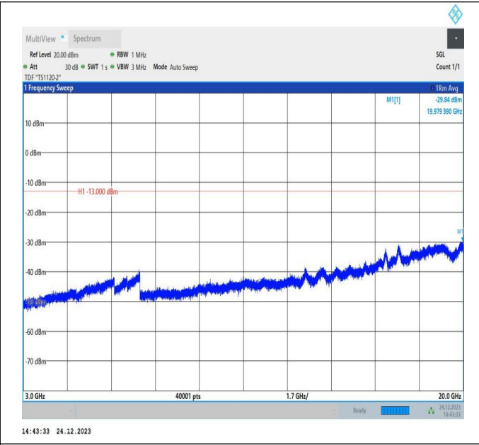
66-66-20MHz-20MHz-QPSK-QPSK-132323-132521-1RB#0-1RB#99-3000~20000MHz-PASS
