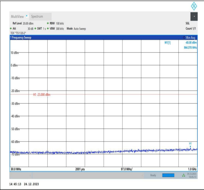
66-66-20MHz-20MHz-QPSK-QPSK-132374-132572-1RB#0-ORB#0-30~1000MHz-PASS
