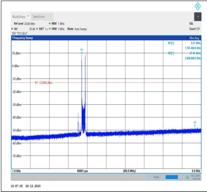
66-66-20MHz-20MHz-QPSK-QPSK-132374-132572-1RB#0-1RB#99-1000~3000MHz-PASS
