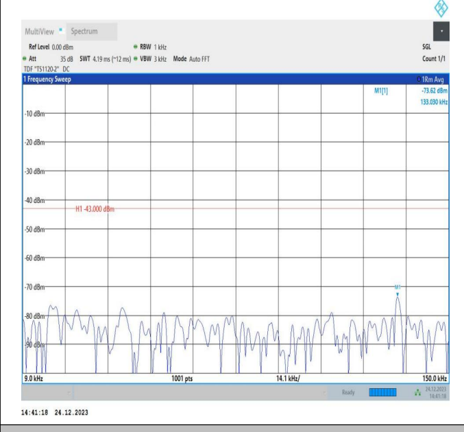
66-66-20MHz-20MHz-QPSK-QPSK-132323-132521-1RB#0- 0RB#0-0.009~0.15MHz-PASS
