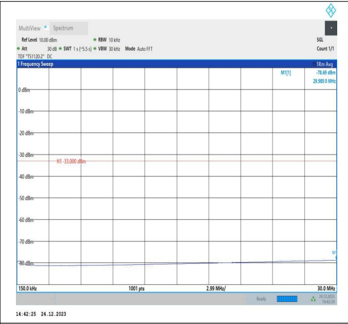
66-66-20MHz-20MHz-QPSK-QPSK-132323-132521-1RB#99 -ORB#0-0.15~30MHz-PASS
