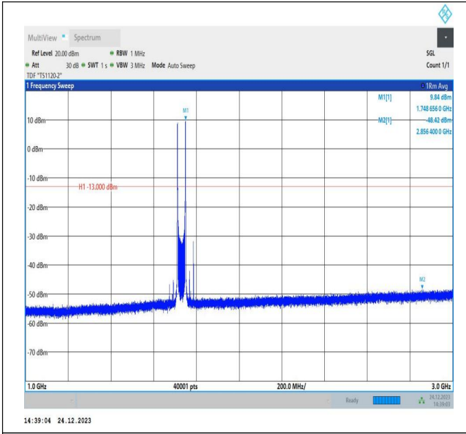
66-66-20MHz-20MHz-QPSK-QPSK-132072-132270-1RB#0-1RB#99-1000~3000MHz-PASS
