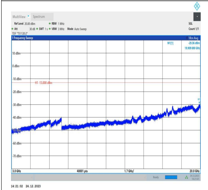
66-66-20MHz-15MHz-QPSK-QPSK-132072-132243-100RB# 0-75RB#0-3000~20000MHz-PASS
