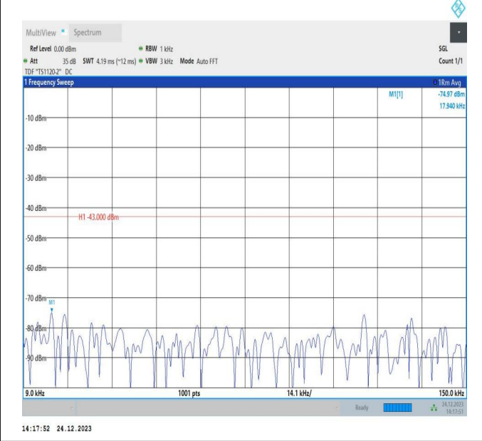
66-66-20MHz-15MHz-QPSK-QPSK-132072-132243-1RB#0- 0RB#0-0.009~0.15MHz-PASS
