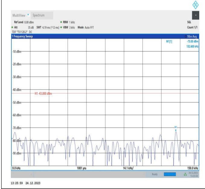
66-66-20MHz-10MHz-QPSK-QPSK-132473-132617-100RB#0-50RB#0-0.009~0.15MHz-PASS
