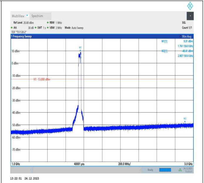
66-66-20MHz-10MHz-QPSK-QPSK-132373-132517-100RB# 0-50RB#0-1000~3000MHz-PASS
