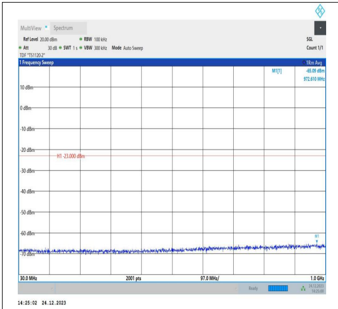
66-66-20MHz-15MHz-QPSK-QPSK-132348-132519-100RB# 0-75RB#0-30~1000MHz-PASS
