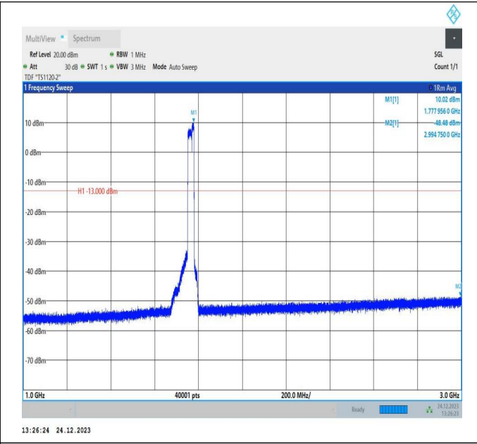
66-66-20MHz-10MHz-QPSK-QPSK-132473-132617-100RB# 0-50RB#0-1000~3000MHz-PASS
