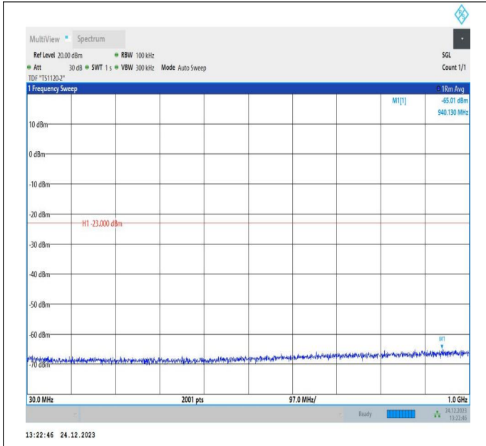
66-66-20MHz-10MHz-QPSK-QPSK-132373-132517-100RB# 0-50RB#0-30~1000MHz-PASS
