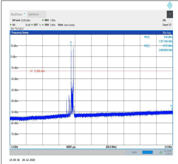
66-66-20MHz-10MHz-QPSK-QPSK-132473-132617-1RB#0-1RB#49-1000~3000MHz-PASS
