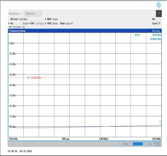
66-66-20MHz-10MHz-QPSK-QPSK-132473-132617-1RB#99 -ORB#0-0.15~30MHz-PASS
