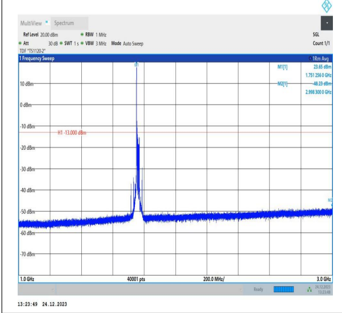
66-66-20MHz-10MHz-QPSK-QPSK-132473-132617-1RB#0-ORB#0-1000~3000MHz-PASS
