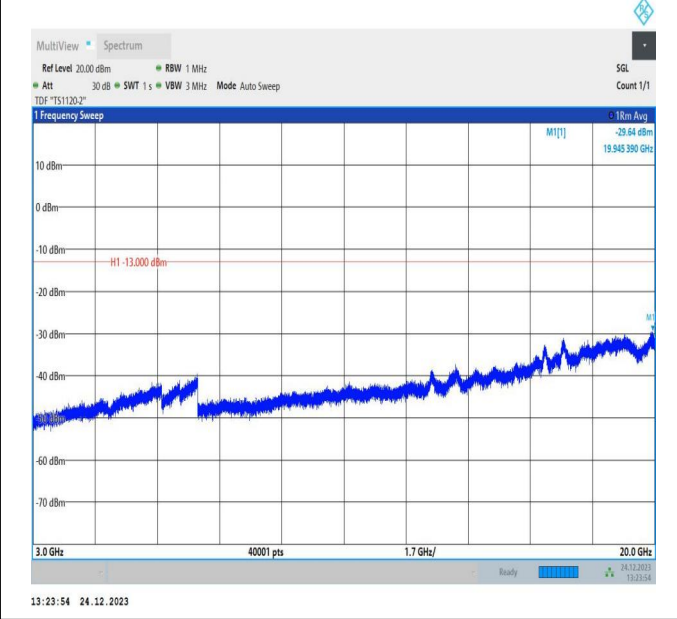
66-66-20MHz-10MHz-QPSK-QPSK-132473-132617-1RB#0-ORB#0-3000~20000MHz-PASS
