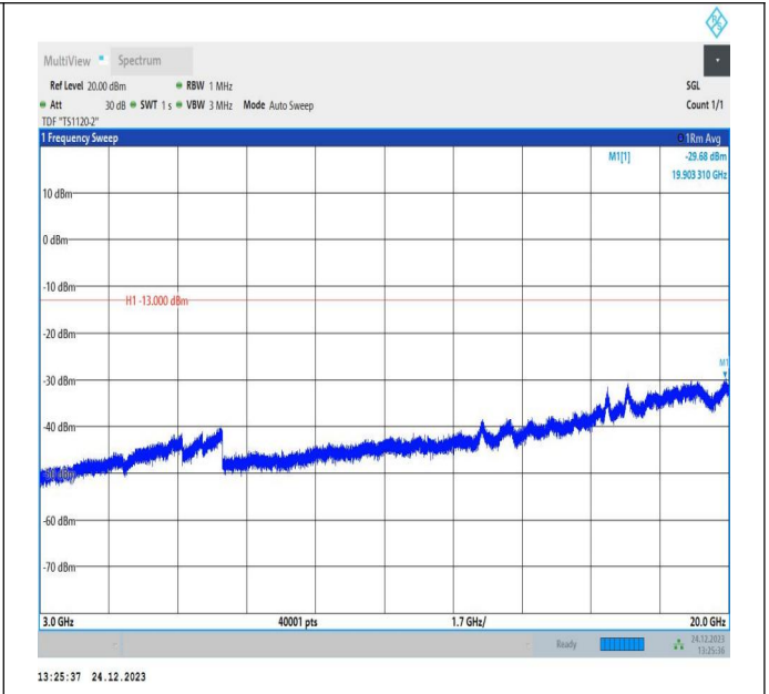
66-66-20MHz-10MHz-QPSK-QPSK-132473-132617-1RB#0-1RB#49-3000~20000MHz-PASS
