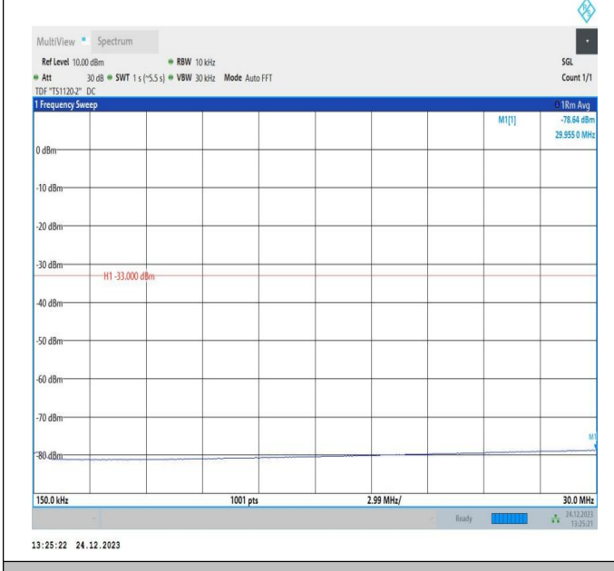
66-66-20MHz-10MHz-QPSK-QPSK-132473-132617-1RB#0- 1RB#49-0.15~30MHz-PASS
