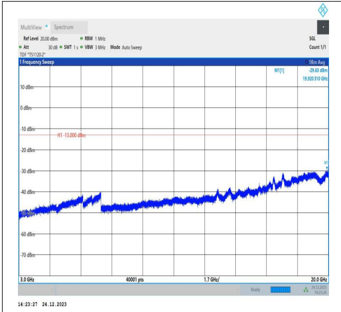
66-66-20MHz-15MHz-QPSK-QPSK-132348-132519-1RB#99 -0RB#0-3000~20000MHz-PASS
