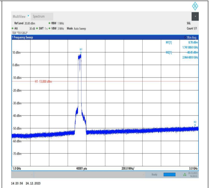
66-66-20MHz-15MHz-QPSK-QPSK-132072-132243-100RB# 0-75RB#0-1000~3000MHz-PASS
