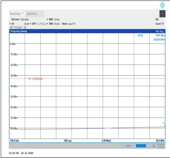
66-66-20MHz-10MHz-QPSK-QPSK-132473-132617-1RB#0-ORB#0-0.15~30MHz-PASS
