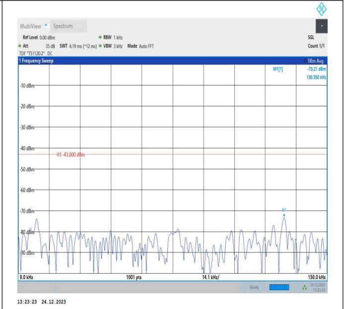
66-66-20MHz-10MHz-QPSK-QPSK-132473-132617-1RB#0- 0RB#0-0.009~0.15MHz-PASS
