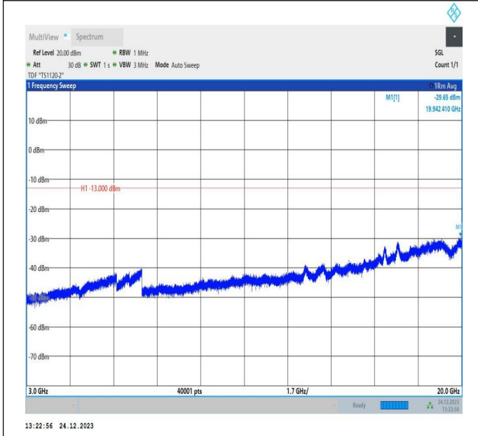
66-66-20MHz-10MHz-QPSK-QPSK-132373-132517-100RB# 0-50RB#0-3000~20000MHz-PASS
