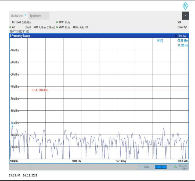
66-66-20MHz-10MHz-QPSK-QPSK-132473-132617-1RB#0- 1RB#49-0.009~0.15MHz-PASS
