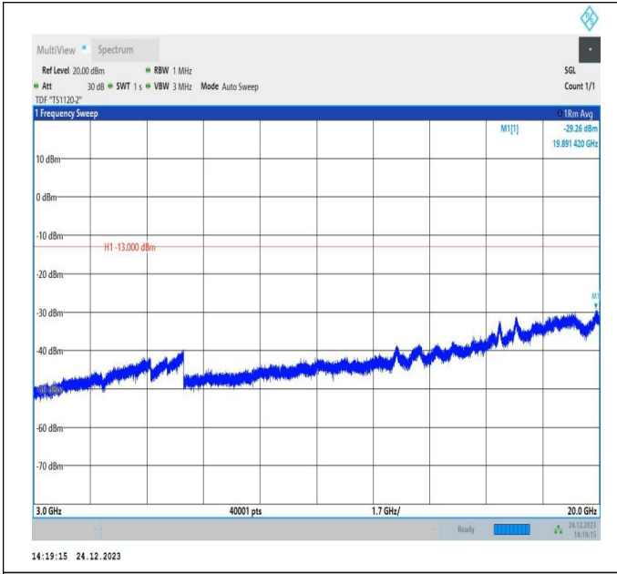
66-66-20MHz-15MHz-QPSK-QPSK-132072-132243-1RB#99-0RB#0-3000~20000MHz-PASS
