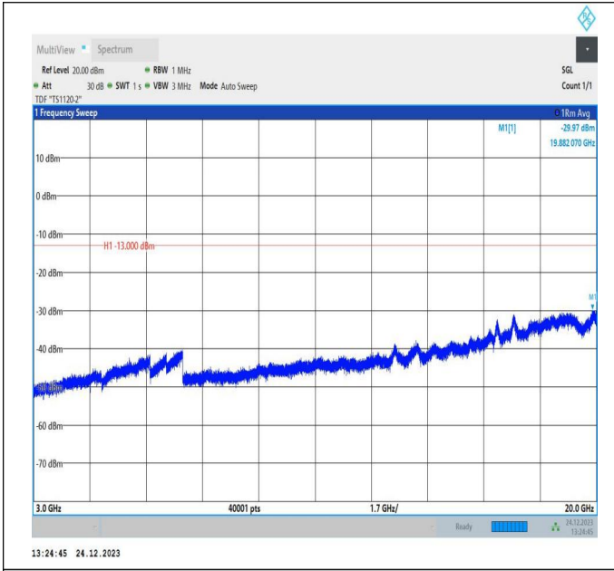
66-66-20MHz-10MHz-QPSK-QPSK-132473-132617-1RB#99 -0RB#0-3000~20000MHz-PASS
