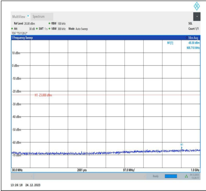
66-66-20MHz-10MHz-QPSK-QPSK-132473-132617-100RB# 0-50RB#0-30~1000MHz-PASS
