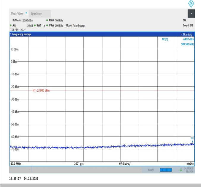
66-66-20MHz-10MHz-QPSK-QPSK-132473-132617-1RB#0- 1RB#49-30~1000MHz-PASS
