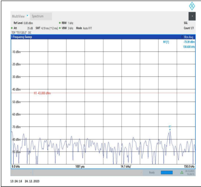
66-66-20MHz-10MHz-QPSK-QPSK-132473-132617-1RB#99 -ORB#0-0.009~0.15MHz-PASS
