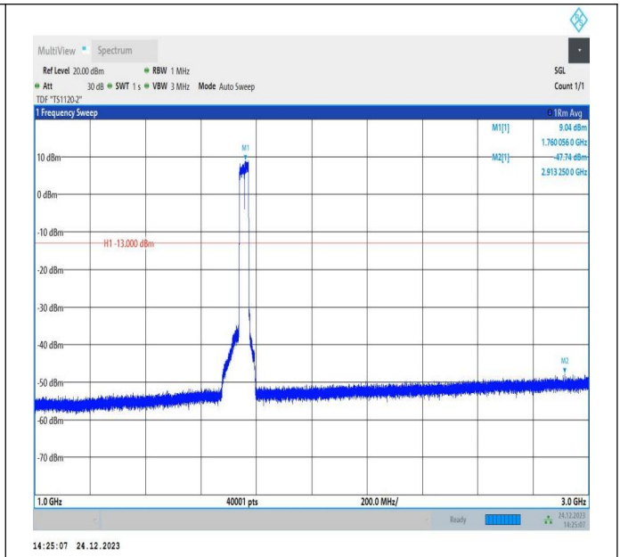
66-66-20MHz-15MHz-QPSK-QPSK-132348-132519-100RB# 0-75RB#0-1000~3000MHz-PASS
