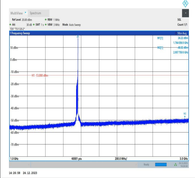
66-66-20MHz-15MHz-QPSK-QPSK-132423-132594-1RB#99 -ORB#0-1000~3000MHz-PASS
