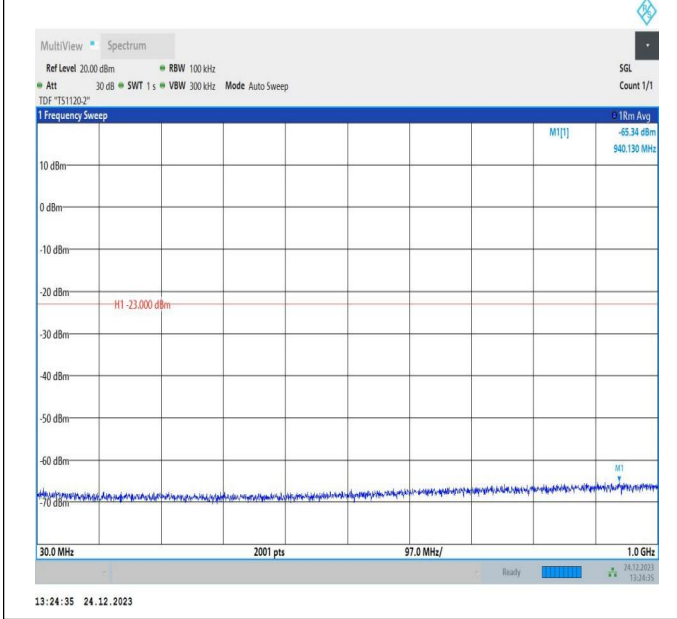
66-66-20MHz-10MHz-QPSK-QPSK-132473-132617-1RB#99 -ORB#0-30~1000MHz-PASS
