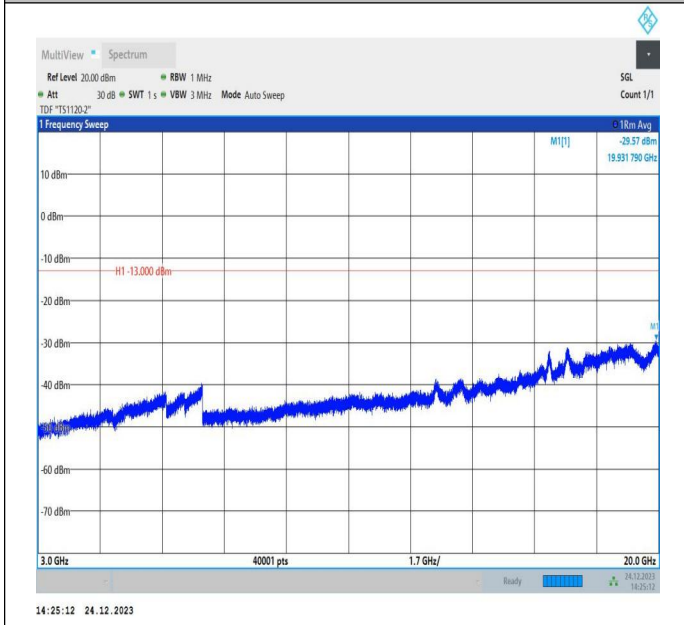
66-66-20MHz-15MHz-QPSK-QPSK-132348-132519-100RB# 0-75RB#0-3000~20000MHz-PASS
