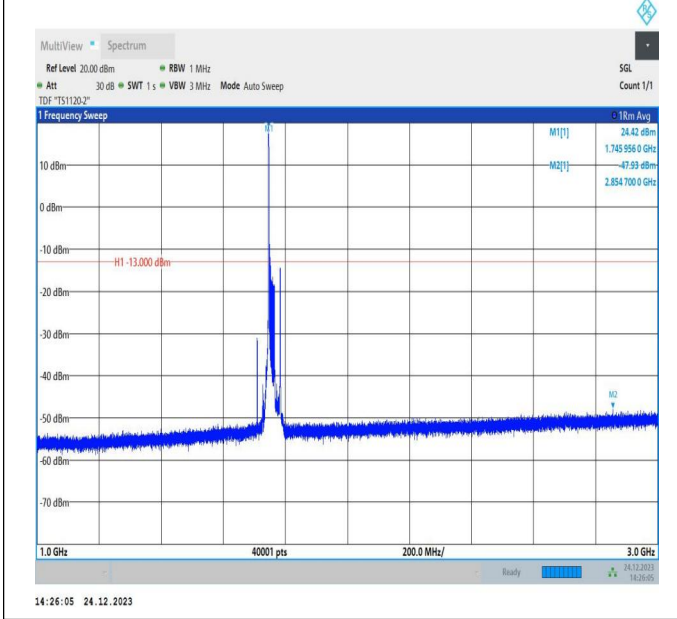
66-66-20MHz-15MHz-QPSK-QPSK-132423-132594-1RB#0-ORB#0-1000~3000MHz-PASS
