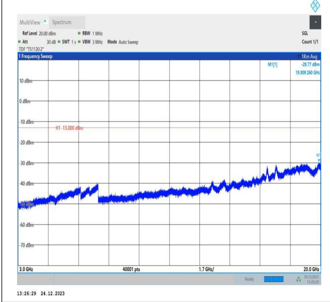
66-66-20MHz-10MHz-QPSK-QPSK-132473-132617-100RB# 0-50RB#0-3000~20000MHz-PASS
