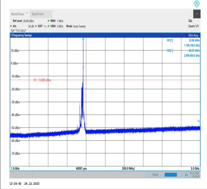
66-66-20MHz-10MHz-QPSK-QPSK-132473-132617-1RB#99 -ORB#0-1000~3000MHz-PASS
