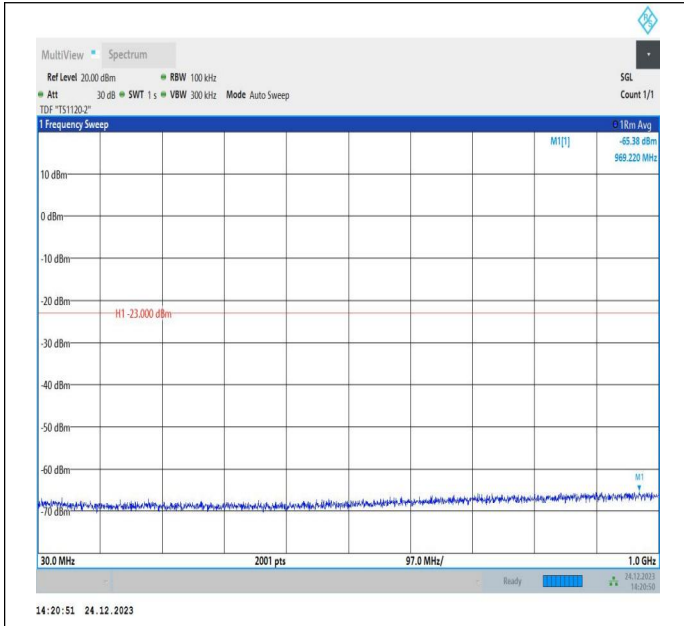
66-66-20MHz-15MHz-QPSK-QPSK-132072-132243-100RB# 0-75RB#0-30~1000MHz-PASS
