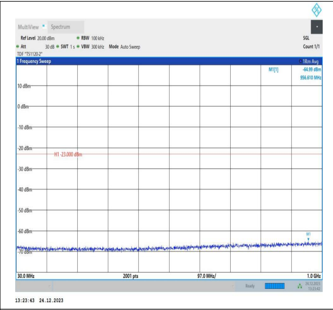
66-66-20MHz-10MHz-QPSK-QPSK-132473-132617-1RB#0-ORB#0-30~1000MHz-PASS
