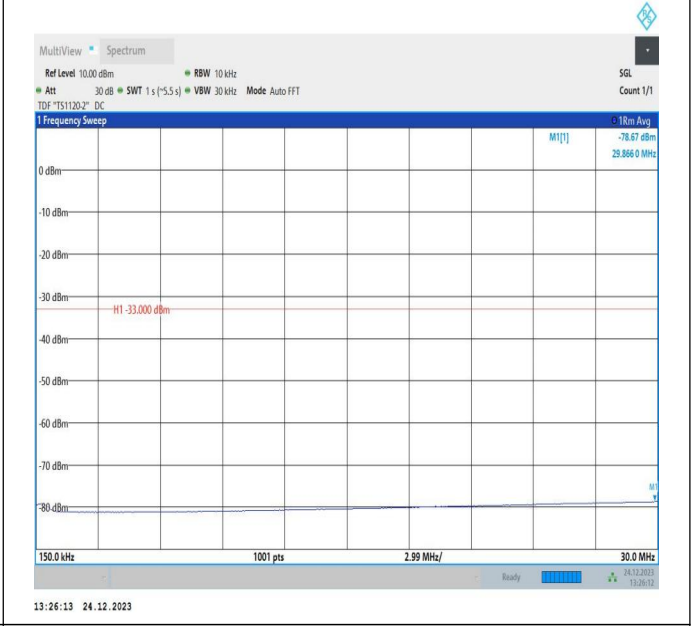
66-66-20MHz-10MHz-QPSK-QPSK-132473-132617-100RB#0-50RB#0-0.15~30MHz-PASS
