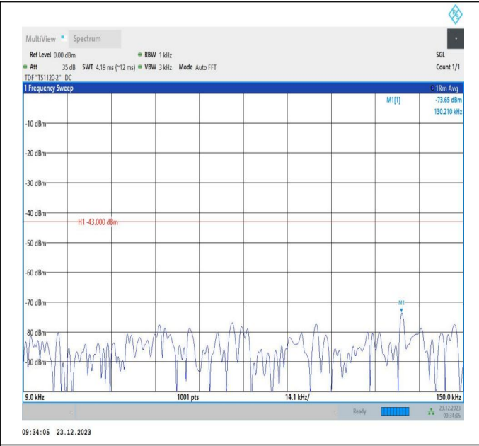
66-66-20MHz-5MHz-QPSK-QPSK-132522-132639-100RB#0 -25RB#0-0.009~0.15MHz-PASS
