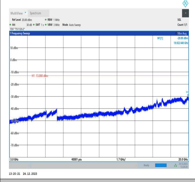
66-66-20MHz-10MHz-QPSK-QPSK-132373-132517-1RB#0-ORB#0-3000~20000MHz-PASS
