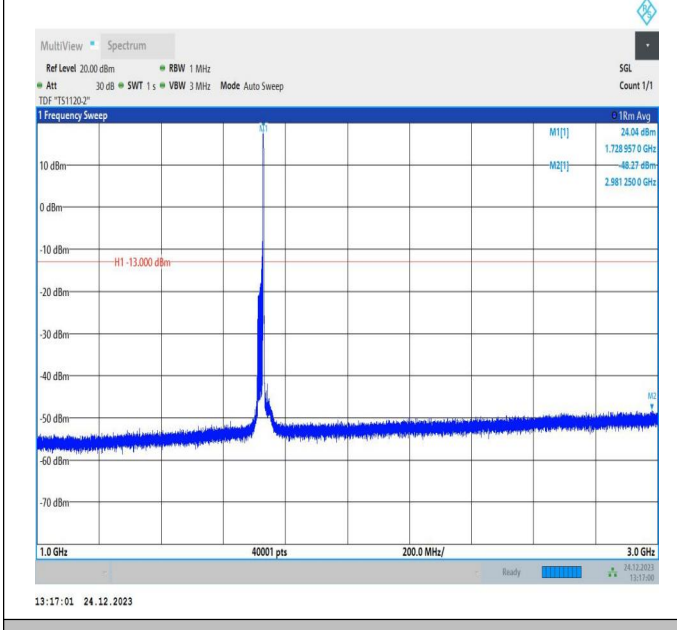
66-66-20MHz-10MHz-QPSK-QPSK-132072-132216-1RB#99 -ORB#0-1000~3000MHz-PASS
