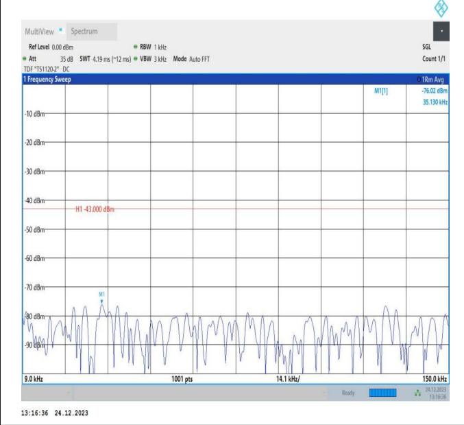
66-66-20MHz-10MHz-QPSK-QPSK-132072-132216-1RB#99 -ORB#0-0.009~0.15MHz-PASS
