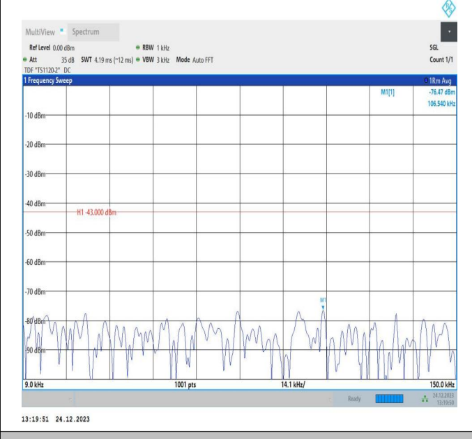
66-66-20MHz-10MHz-QPSK-QPSK-132373-132517-1RB#0- 0RB#0-0.009~0.15MHz-PASS
