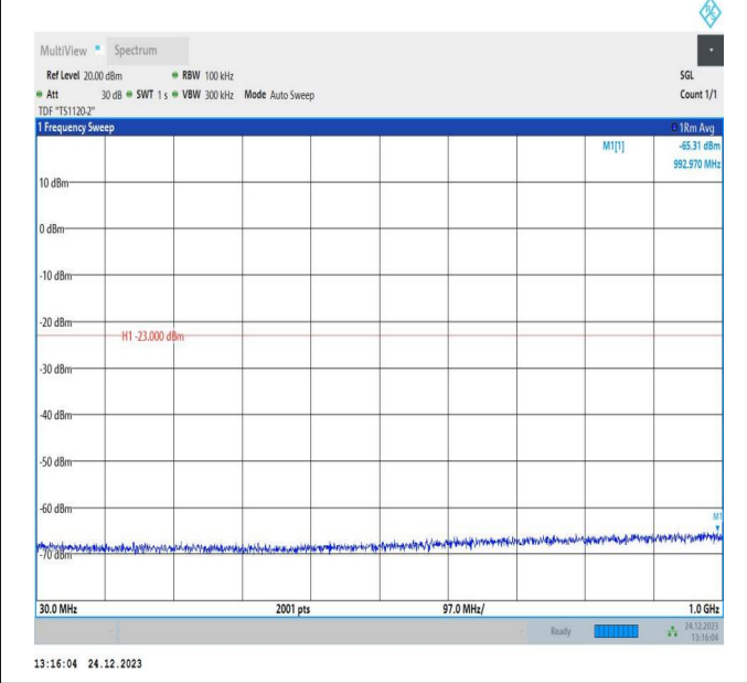
66-66-20MHz-10MHz-QPSK-QPSK-132072-132216-1RB#0-0RB#0-30~1000MHz-PASS
