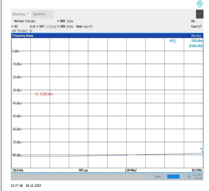
66-66-20MHz-10MHz-QPSK-QPSK-132072-132216-1RB#0- 1RB#49-0.15~30MHz-PASS
