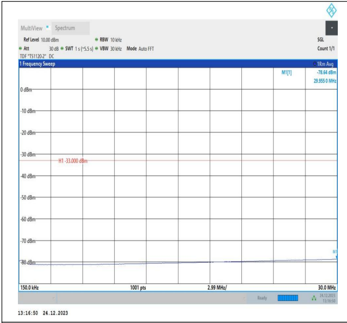
66-66-20MHz-10MHz-QPSK-QPSK-132072-132216-1RB#99 -ORB#0-0.15~30MHz-PASS
