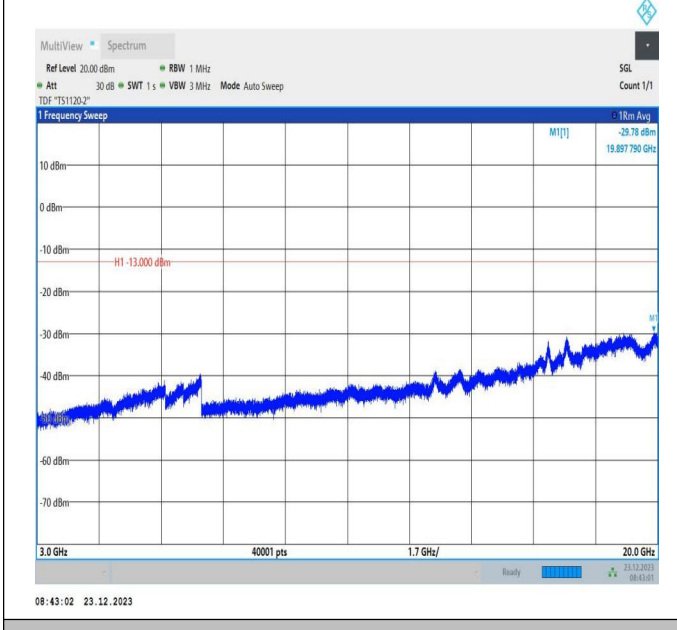
66-66-20MHz-5MHz-QPSK-QPSK-132522-132639-1RB#0-1 RB#24-3000~20000MHz-PASS
