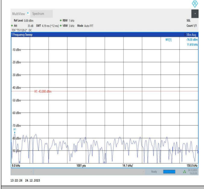
66-66-20MHz-10MHz-QPSK-QPSK-132373-132517-100RB#0-50RB#0-0.009~0.15MHz-PASS
