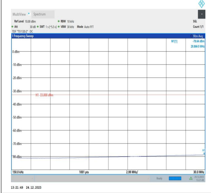
66-66-20MHz-10MHz-QPSK-QPSK-132373-132517-1RB#0- 1RB#49-0.15~30MHz-PASS
