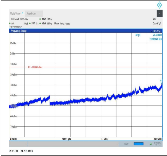
66-66-20MHz-10MHz-QPSK-QPSK-132373-132517-1RB#99 -0RB#0-3000~20000MHz-PASS
