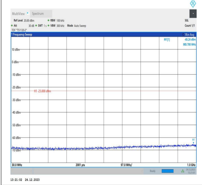
66-66-20MHz-10MHz-QPSK-QPSK-132373-132517-1RB#99 -ORB#0-30~1000MHz-PASS
