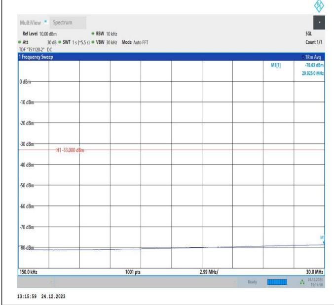
66-66-20MHz-10MHz-QPSK-QPSK-132072-132216-1RB#0-0RB#0-0.15~30MHz-PASS
