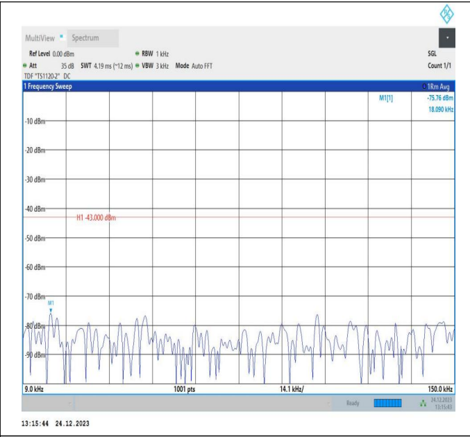
66-66-20MHz-10MHz-QPSK-QPSK-132072-132216-1RB#0-0RB#0-0.009~0.15MHz-PASS
