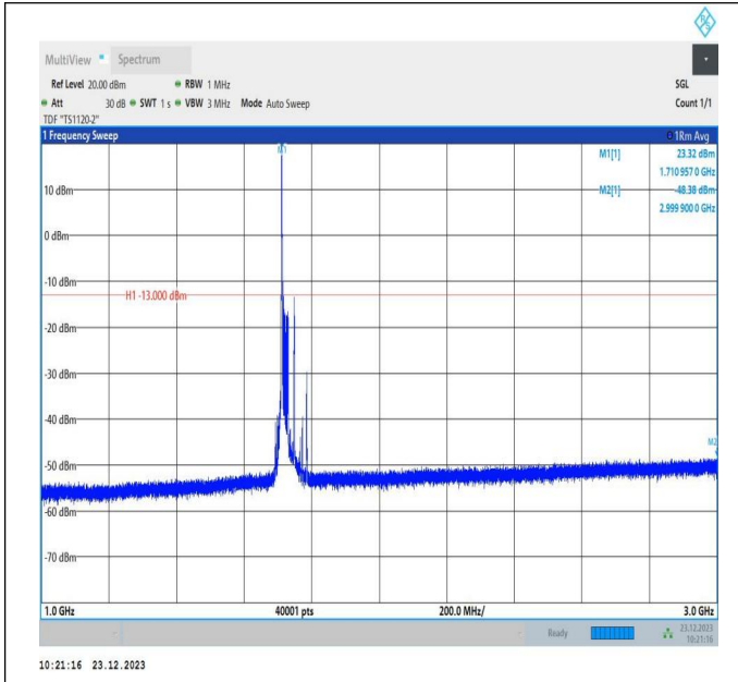
66-66-20MHz-10MHz-16QAM-16QAM-132072-132216-1RB# 0-ORB#0-1000~3000MHz-PASS
