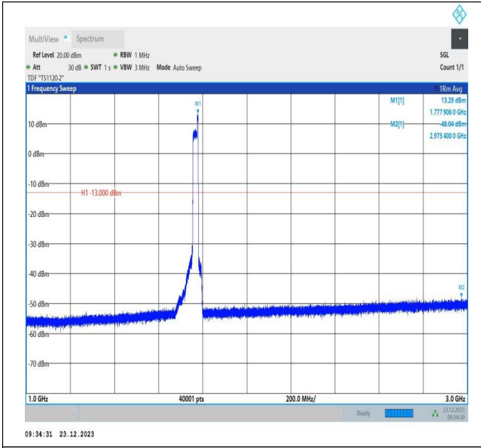
66-66-20MHz-5MHz-QPSK-QPSK-132522-132639-100RB#0 -25RB#0-1000~3000MHz-PASS
