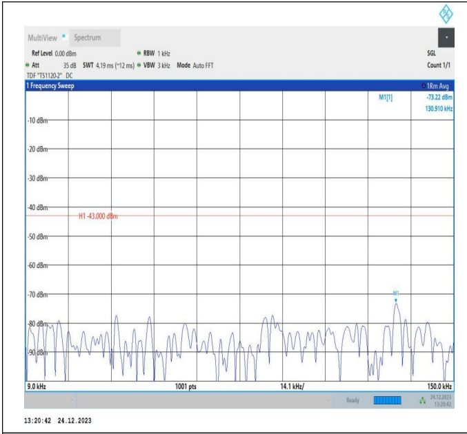
66-66-20MHz-10MHz-QPSK-QPSK-132373-132517-1RB#99 -ORB#0-0.009~0.15MHz-PASS
