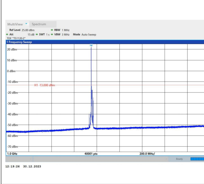
66-66-20MHz-5MHz-64QAM-64QAM-132522-132639-100RB #0-25RB#0-1000~3000MHz-PASS
