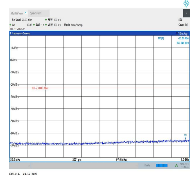
66-66-20MHz-10MHz-QPSK-QPSK-132072-132216-1RB#0- 1RB#49-30~1000MHz-PASS
