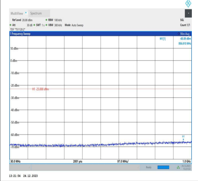
66-66-20MHz-10MHz-QPSK-QPSK-132373-132517-1RB#0- 1RB#49-30~1000MHz-PASS
