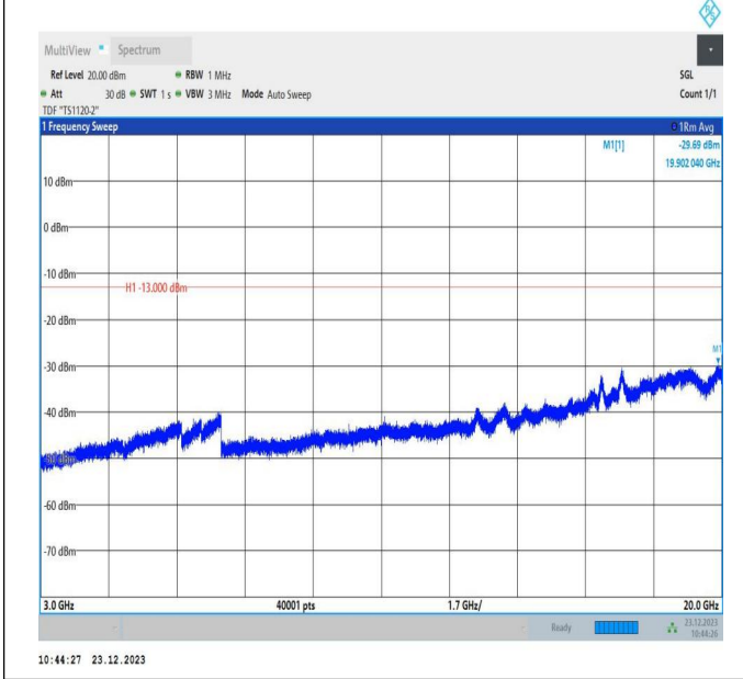
66-66-20MHz-10MHz-64QAM-64QAM-132072-132216-1RB# 0-ORB#0-3000~20000MHz-PASS
