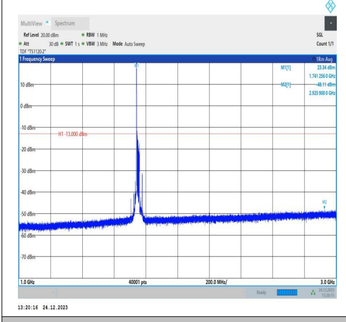
66-66-20MHz-10MHz-QPSK-QPSK-132373-132517-1RB#0-ORB#0-1000~3000MHz-PASS
