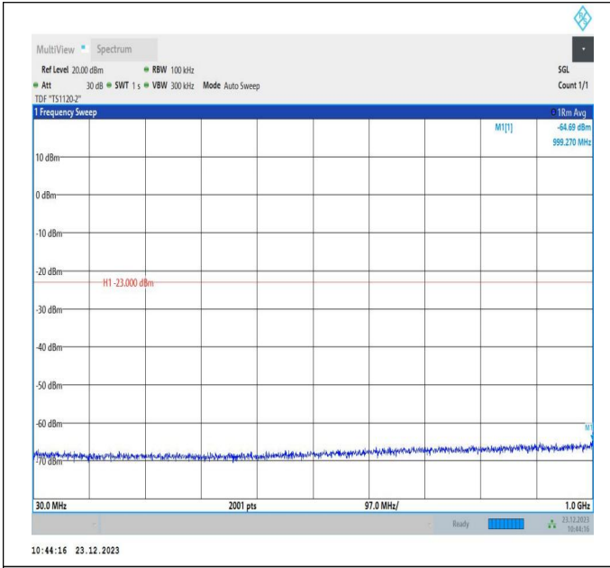
66-66-20MHz-10MHz-64QAM-64QAM-132072-132216-1RB# 0-ORB#0-30~1000MHz-PASS
