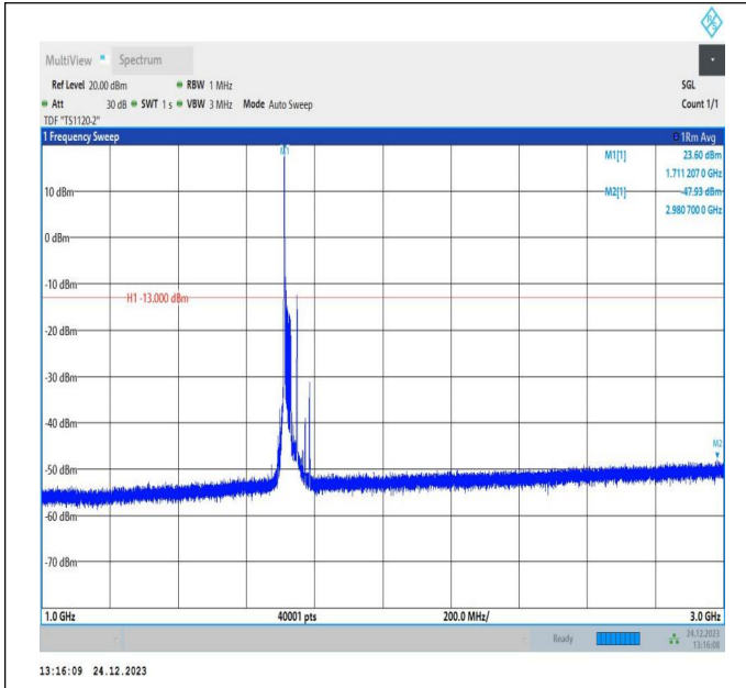
66-66-20MHz-10MHz-QPSK-QPSK-132072-132216-1RB#0-ORB#0-1000~3000MHz-PASS
