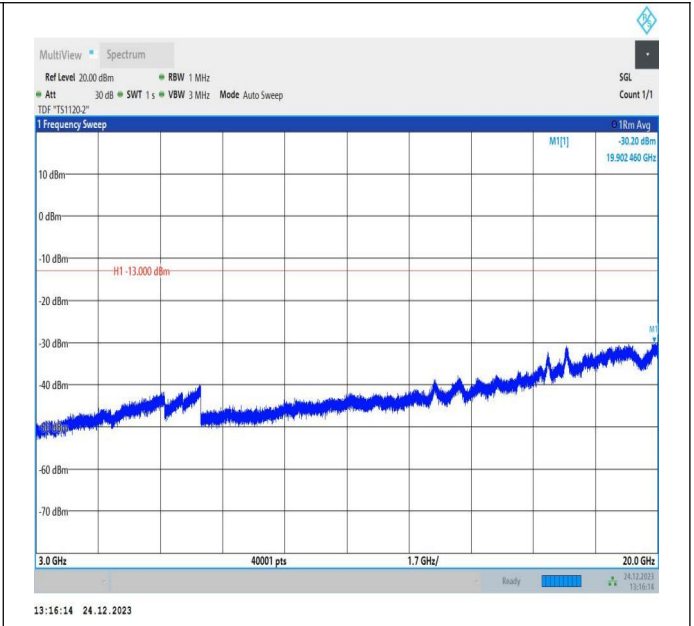
66-66-20MHz-10MHz-QPSK-QPSK-132072-132216-1RB#0-ORB#0-3000~20000MHz-PASS
