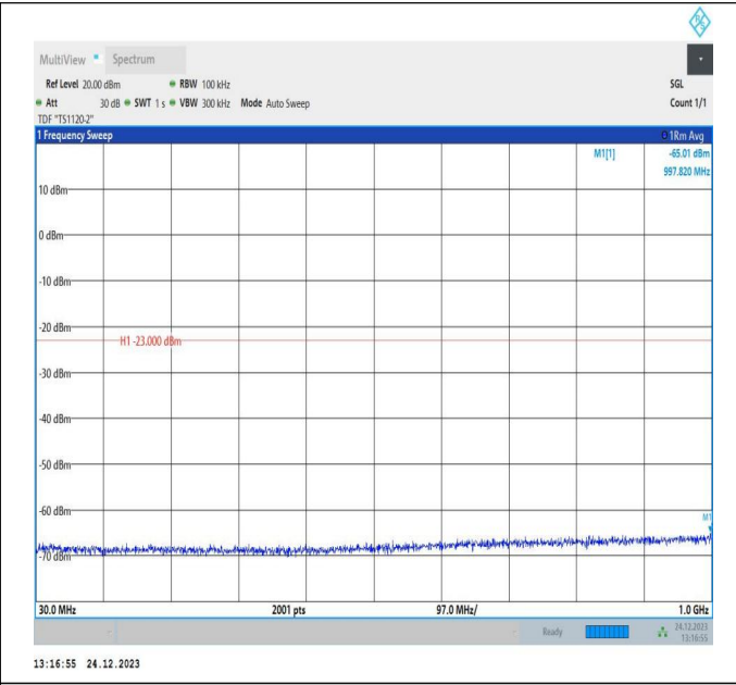
66-66-20MHz-10MHz-QPSK-QPSK-132072-132216-1RB#99 -ORB#0-30~1000MHz-PASS
