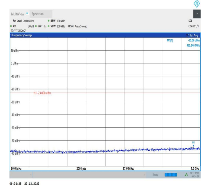
66-66-20MHz-5MHz-QPSK-QPSK-132522-132639-100RB#0 -25RB#0-30~1000MHz-PASS
