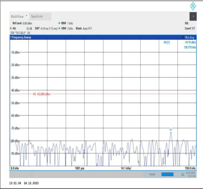
66-66-20MHz-10MHz-QPSK-QPSK-132373-132517-1RB#0- 1RB#49-0.009~0.15MHz-PASS
