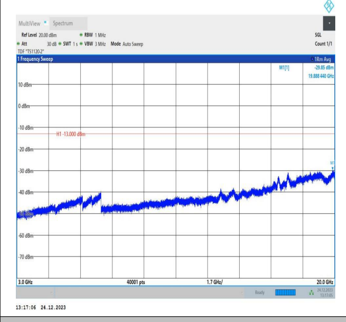
66-66-20MHz-10MHz-QPSK-QPSK-132072-132216-1RB#99 -ORB#0-3000~20000MHz-PASS
