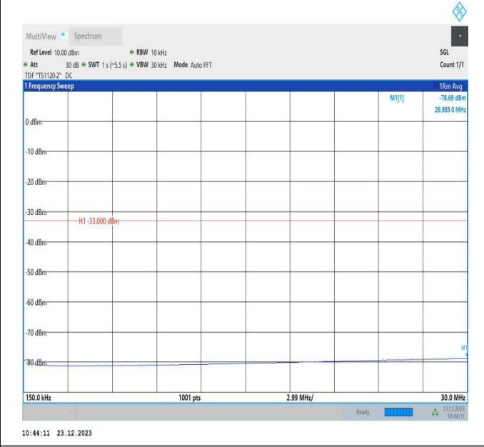
66-66-20MHz-10MHz-64QAM-64QAM-132072-132216-1RB# 0-ORB#0-0.15~30MHz-PASS
