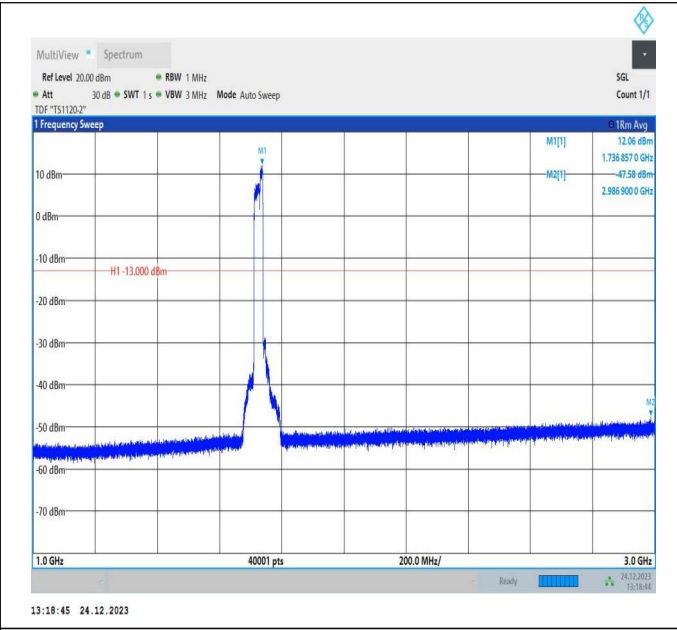
66-66-20MHz-10MHz-QPSK-QPSK-132072-132216-100RB# 0-50RB#0-1000~3000MHz-PASS
