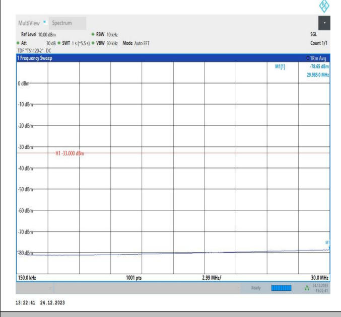
66-66-20MHz-10MHz-QPSK-QPSK-132373-132517-100RB#0-50RB#0-0.15~30MHz-PASS
