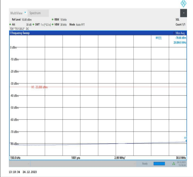
66-66-20MHz-10MHz-QPSK-QPSK-132072-132216-100RB#0-50RB#0-0.15~30MHz-PASS
