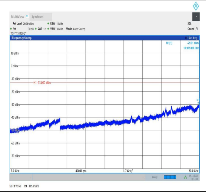
66-66-20MHz-10MHz-QPSK-QPSK-132072-132216-1RB#0-1RB#49-3000~20000MHz-PASS
