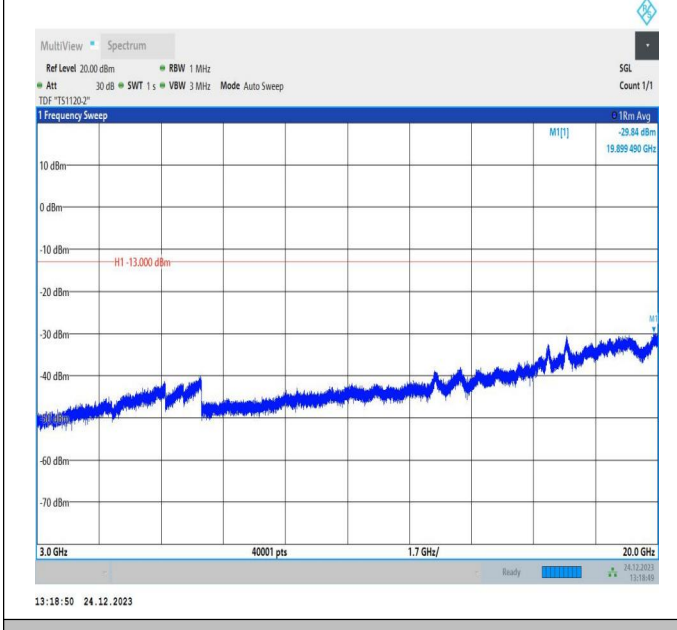
66-66-20MHz-10MHz-QPSK-QPSK-132072-132216-100RB# 0-50RB#0-3000~20000MHz-PASS
