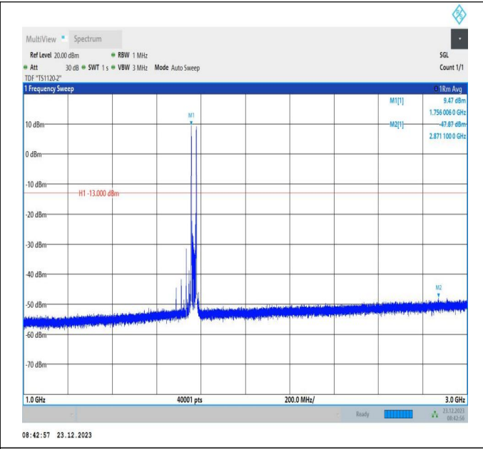
66-66-20MHz-5MHz-QPSK-QPSK-132522-132639-1RB#0-1 RB#24-1000~3000MHz-PASS
