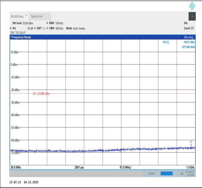
66-66-20MHz-10MHz-QPSK-QPSK-132373-132517-1RB#0-ORB#0-30~1000MHz-PASS
