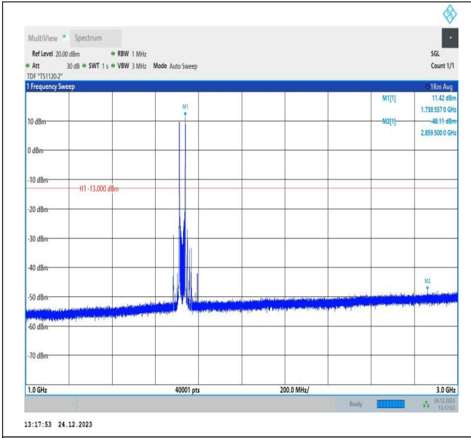
66-66-20MHz-10MHz-QPSK-QPSK-132072-132216-1RB#0-1RB#49-1000~3000MHz-PASS
