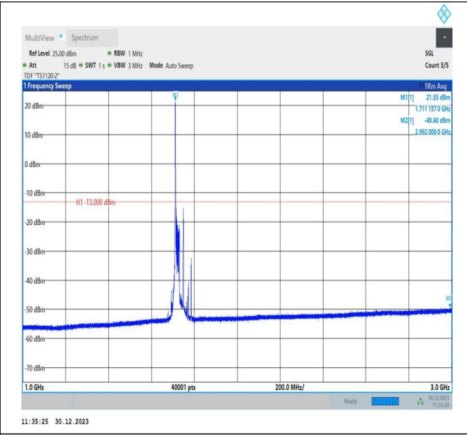
66-66-20MHz-10MHz-64QAM-64QAM-132072-132216-1RB# 0-ORB#0-1000~3000MHz-PASS
