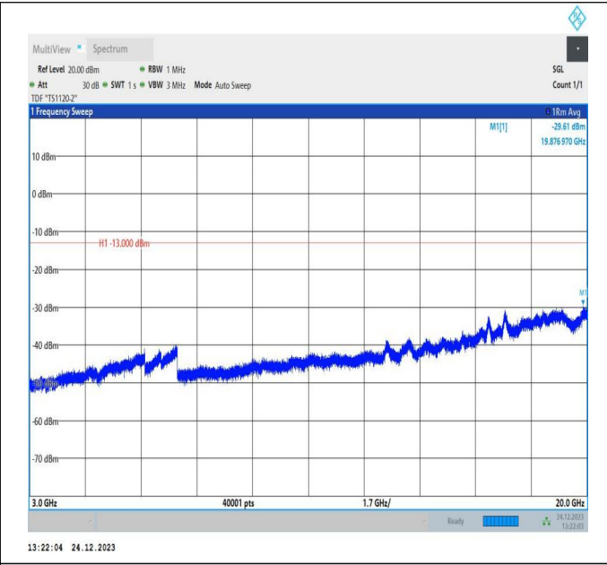
66-66-20MHz-10MHz-QPSK-QPSK-132373-132517-1RB#0-1RB#49-3000~20000MHz-PASS
