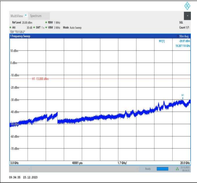
66-66-20MHz-5MHz-QPSK-QPSK-132522-132639-100RB#0 -25RB#0-3000~20000MHz-PASS
