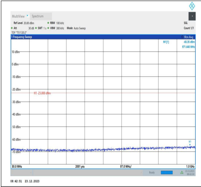
66-66-20MHz-5MHz-QPSK-QPSK-132522-132639-1RB#0-1 RB#24-30~1000MHz-PASS
