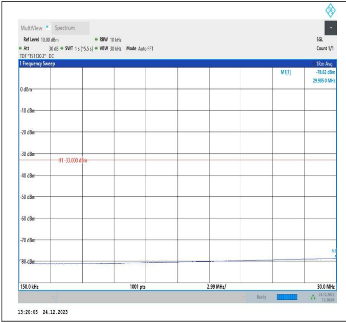
66-66-20MHz-10MHz-QPSK-QPSK-132373-132517-1RB#0-ORB#0-0.15~30MHz-PASS
