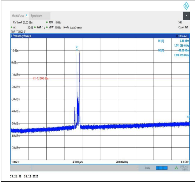
66-66-20MHz-10MHz-QPSK-QPSK-132373-132517-1RB#0-1RB#49-1000~3000MHz-PASS
