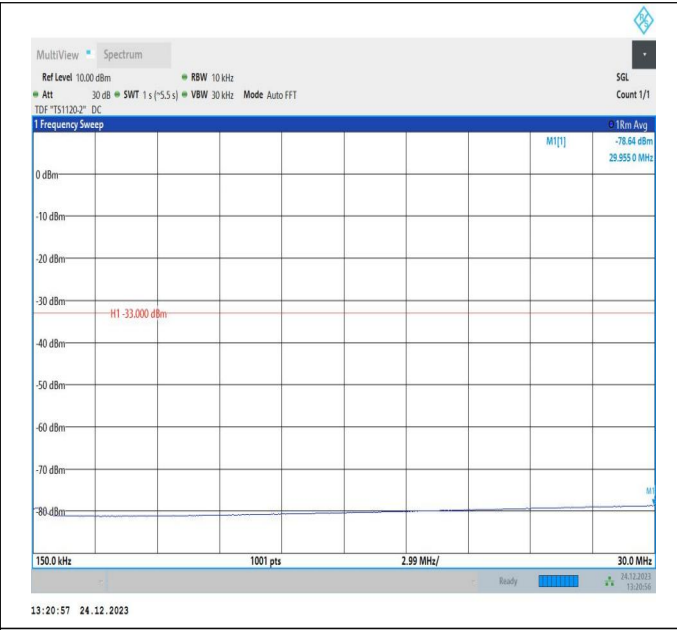
66-66-20MHz-10MHz-QPSK-QPSK-132373-132517-1RB#99 -ORB#0-0.15~30MHz-PASS
