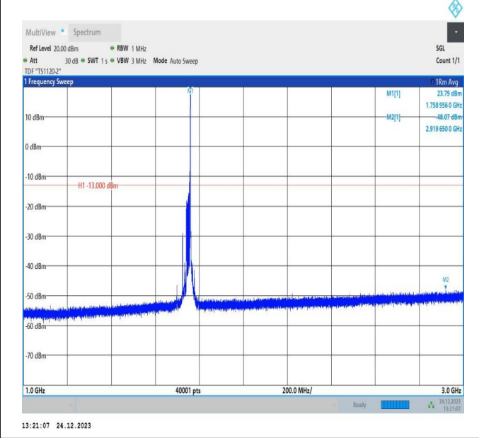
66-66-20MHz-10MHz-QPSK-QPSK-132373-132517-1RB#99 -ORB#0-1000~3000MHz-PASS
