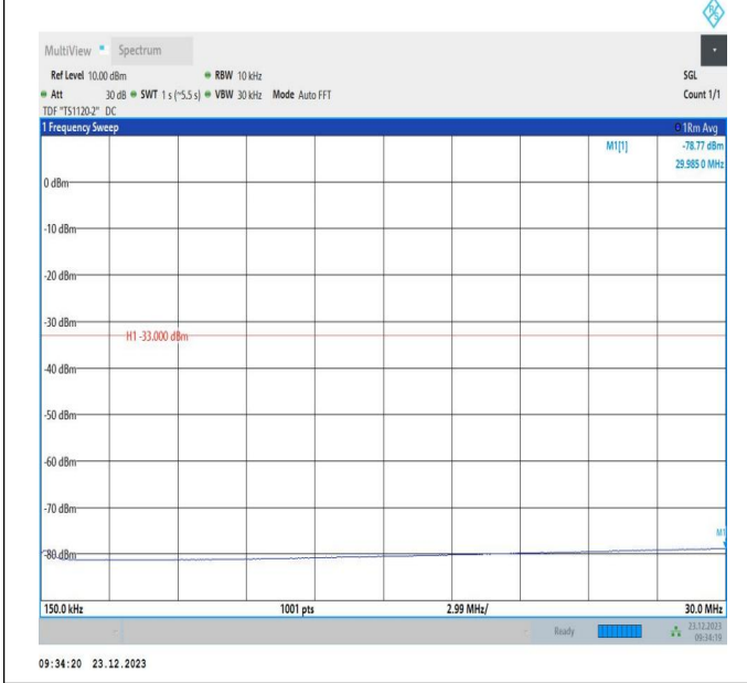
66-66-20MHz-5MHz-QPSK-QPSK-132522-132639-100RB#0 -25RB#0-0.15~30MHz-PASS
