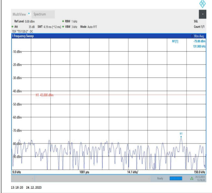
66-66-20MHz-10MHz-QPSK-QPSK-132072-132216-100RB#0-50RB#0-0.009~0.15MHz-PASS
