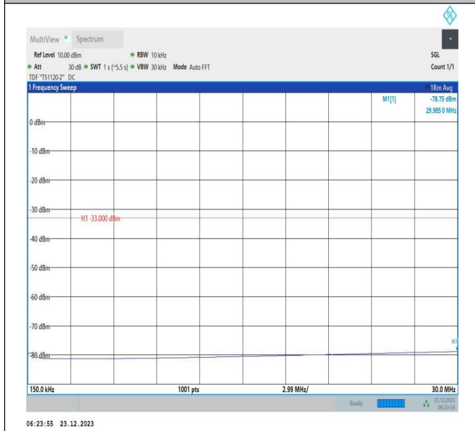
66-66-20MHz-5MHz-QPSK-QPSK-132397-132514-100RB#0 -25RB#0-0.15~30MHz-PASS
