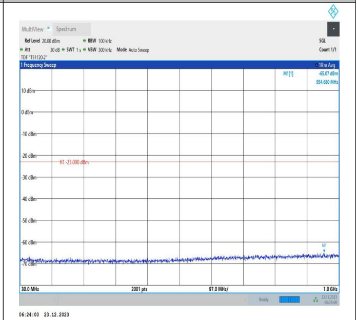
66-66-20MHz-5MHz-QPSK-QPSK-132397-132514-100RB#0 -25RB#0-30~1000MHz-PASS
