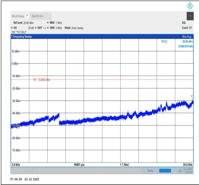
66-66-20MHz-5MHz-QPSK-QPSK-132522-132639-1RB#0-0-RB#0-3000~20000MHz-PASS
