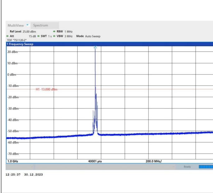
66-66-20MHz-5MHz-64QAM-64QAM-132397-132514-100RB #0-25RB#0-1000~3000MHz-PASS
