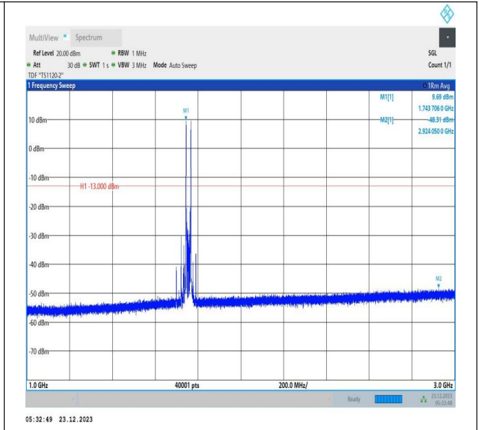
66-66-20MHz-5MHz-QPSK-QPSK-132397-132514-1RB#0-1 RB#24-1000~3000MHz-PASS
