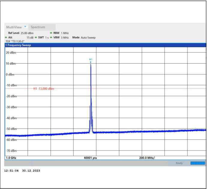
66-66-20MHz-5MHz-64QAM-64QAM-132397-132514-1RB#0 -ORB#0-1000~3000MHz-PASS
