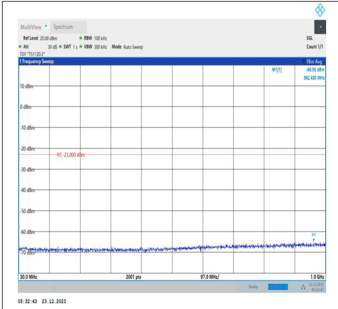
66-66-20MHz-5MHz-QPSK-QPSK-132397-132514-1RB#0-1 RB#24-30~1000MHz-PASS
