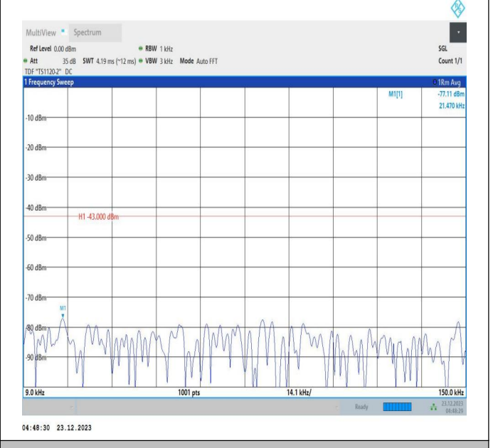
66-66-20MHz-5MHz-QPSK-QPSK-132397-132514-1RB#99- ORB#0-0.009~0.15MHz-PASS
