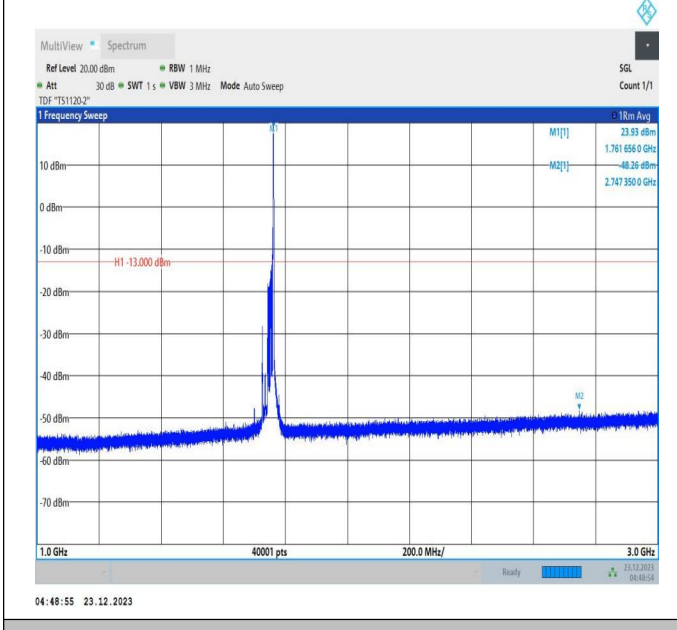
66-66-20MHz-5MHz-QPSK-QPSK-132397-132514-1RB#99-ORB#0-1000~3000MHz-PASS
