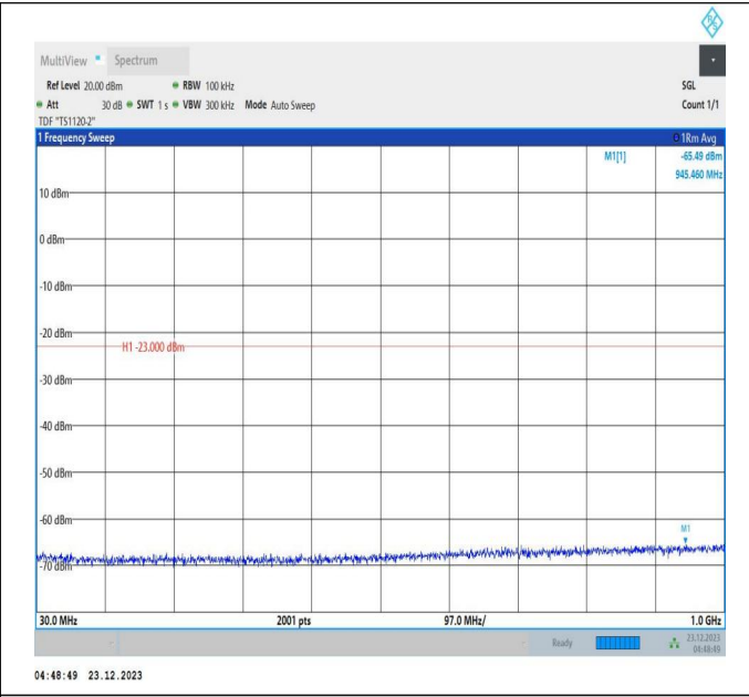
66-66-20MHz-5MHz-QPSK-QPSK-132397-132514-1RB#99-ORB#0-30~1000MHz-PASS
