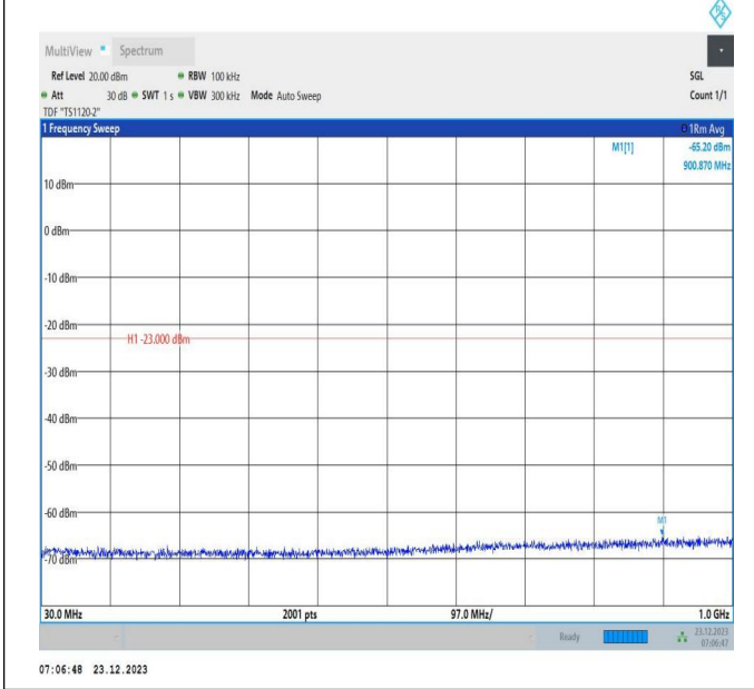
66-66-20MHz-5MHz-QPSK-QPSK-132522-132639-1RB#0-0 RB#0-30~1000MHz-PASS
