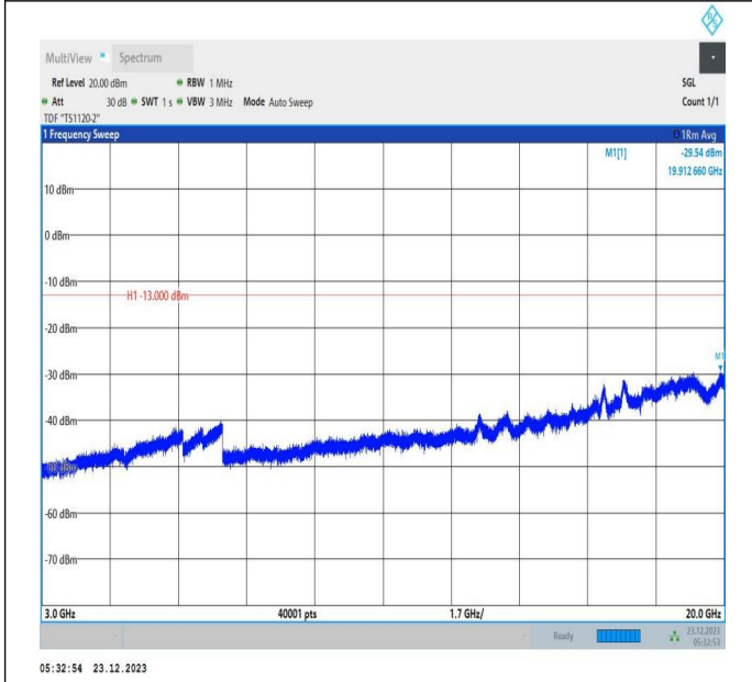
66-66-20MHz-5MHz-QPSK-QPSK-132397-132514-1RB#0-1 RB#24-3000~20000MHz-PASS
