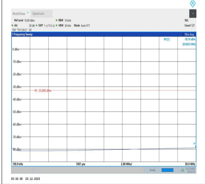
66-66-20MHz-5MHz-QPSK-QPSK-132397-132514-1RB#0-1 RB#24-0.15~30MHz-PASS
