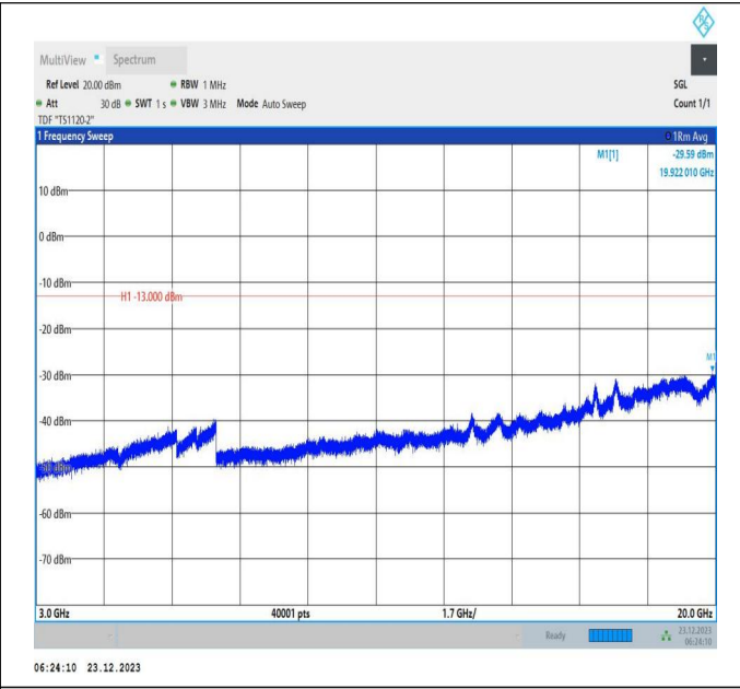
66-66-20MHz-5MHz-QPSK-QPSK-132397-132514-100RB#0 -25RB#0-3000~20000MHz-PASS
