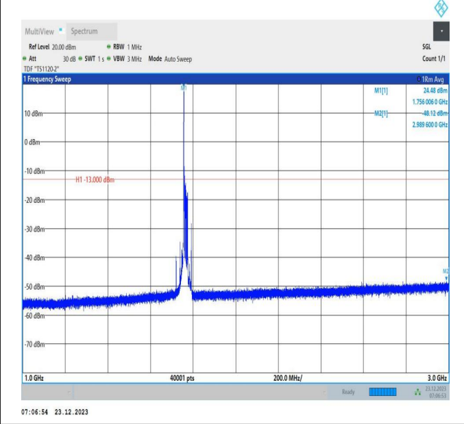
66-66-20MHz-5MHz-QPSK-QPSK-132522-132639-1RB#0-0 RB#0-1000~3000MHz-PASS
