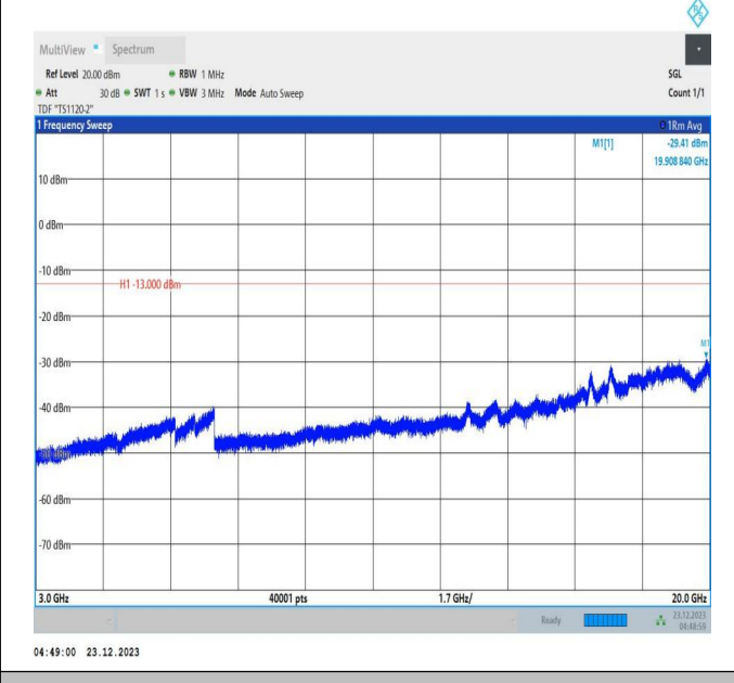
66-66-20MHz-5MHz-QPSK-QPSK-132397-132514-1RB#99-ORB#0-3000~20000MHz-PASS
