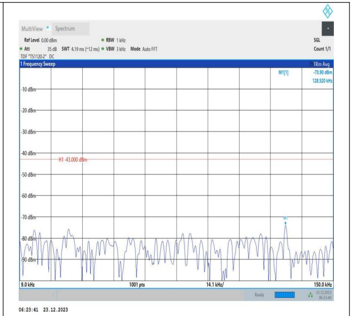
66-66-20MHz-5MHz-QPSK-QPSK-132397-132514-100RB#0 -25RB#0-0.009~0.15MHz-PASS
