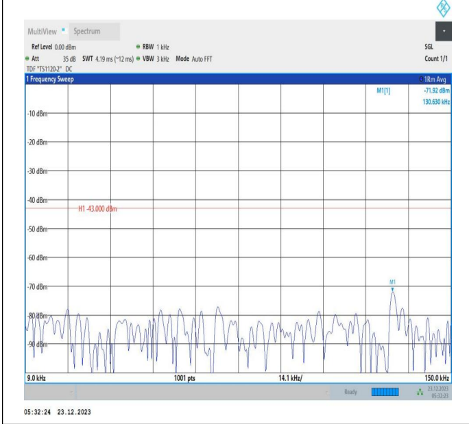
66-66-20MHz-5MHz-QPSK-QPSK-132397-132514-1RB#0-1 RB#24-0.009~0.15MHz-PASS
