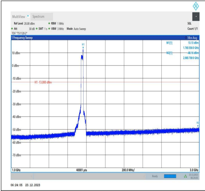
66-66-20MHz-5MHz-QPSK-QPSK-132397-132514-100RB#0 -25RB#0-1000~3000MHz-PASS
