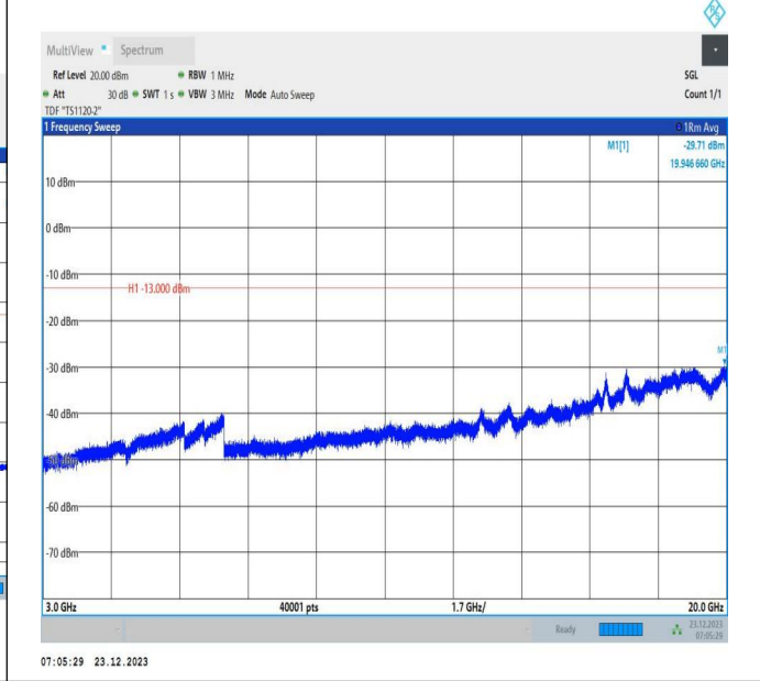
66-66-20MHz-5MHz-64QAM-64QAM-132397-132514-100RB #0-25RB#0-3000~20000MHz-PASS
