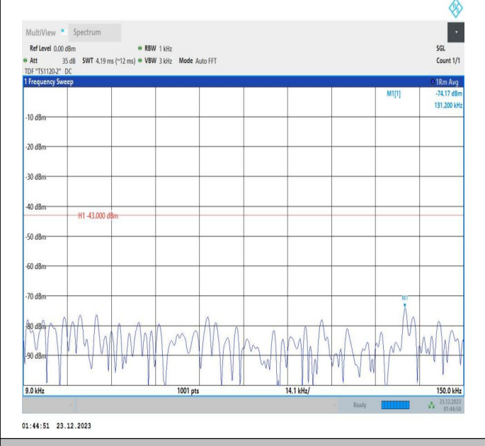
66-66-20MHz-5MHz-QPSK-QPSK-132072-132189-1RB#99- ORB#0-0.009~0.15MHz-PASS
