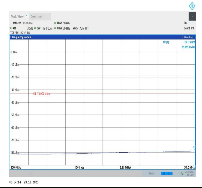
66-66-20MHz-5MHz-QPSK-QPSK-132072-132189-1RB#0-0 RB#0-0.15~30MHz-PASS
