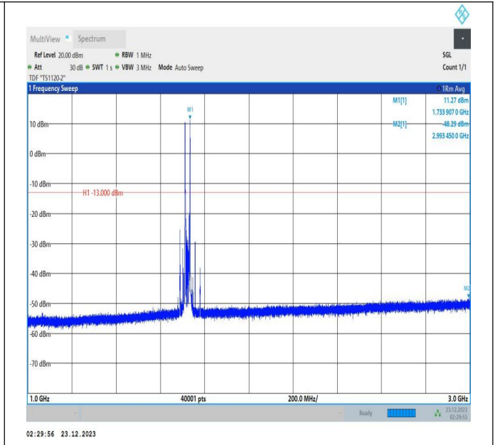
66-66-20MHz-5MHz-QPSK-QPSK-132072-132189-1RB#0-1 RB#24-1000~3000MHz-PASS
