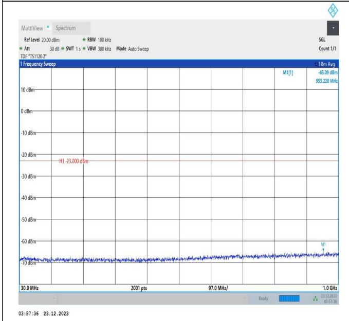
66-66-20MHz-5MHz-QPSK-QPSK-132397-132514-1RB#0-0 RB#0-30~1000MHz-PASS
