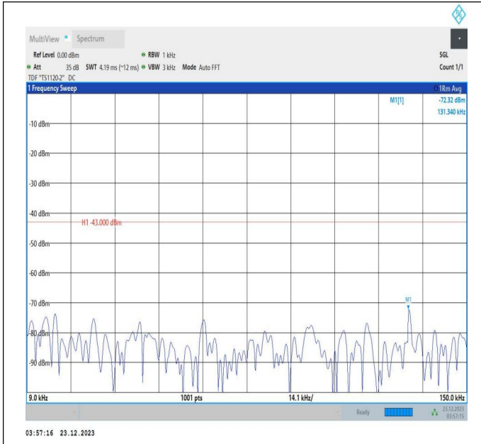
66-66-20MHz-5MHz-QPSK-QPSK-132397-132514-1RB#0-0 RB#0-0.009~0.15MHz-PASS
