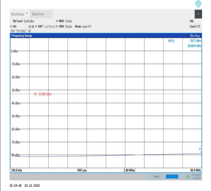
66-66-20MHz-5MHz-QPSK-QPSK-132072-132189-1RB#0-1 RB#24-0.15~30MHz-PASS
