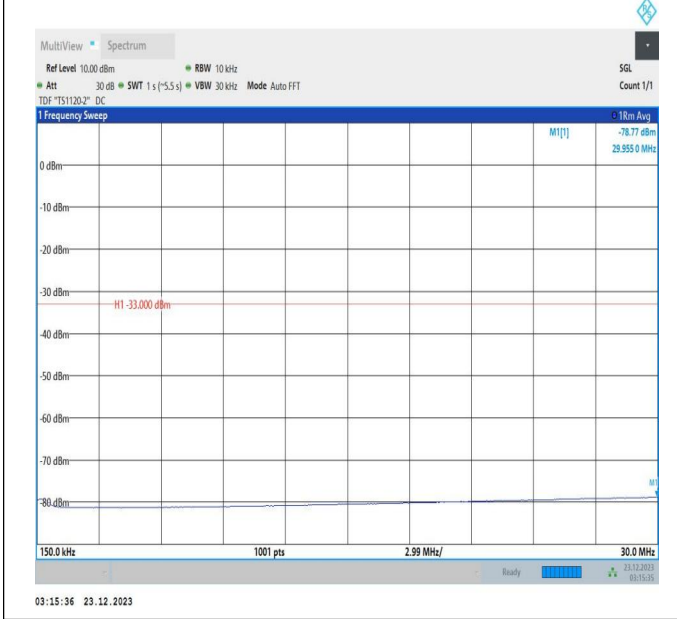
66-66-20MHz-5MHz-QPSK-QPSK-132072-132189-100RB#0 -25RB#0-0.15~30MHz-PASS
