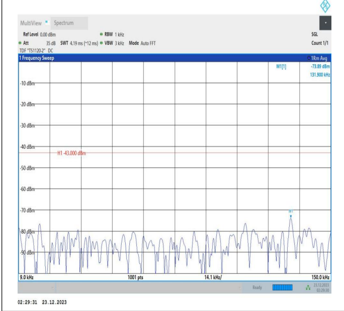
66-66-20MHz-5MHz-QPSK-QPSK-132072-132189-1RB#0-1 RB#24-0.009~0.15MHz-PASS
