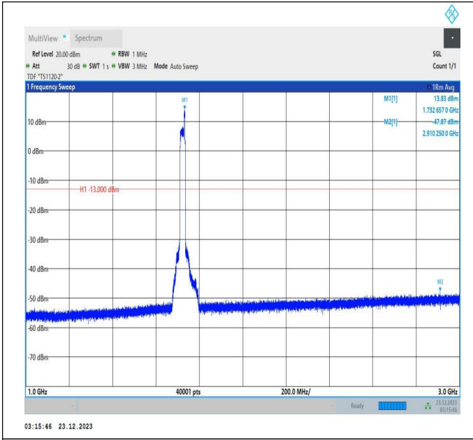
66-66-20MHz-5MHz-QPSK-QPSK-132072-132189-100RB#0 -25RB#0-1000~3000MHz-PASS
