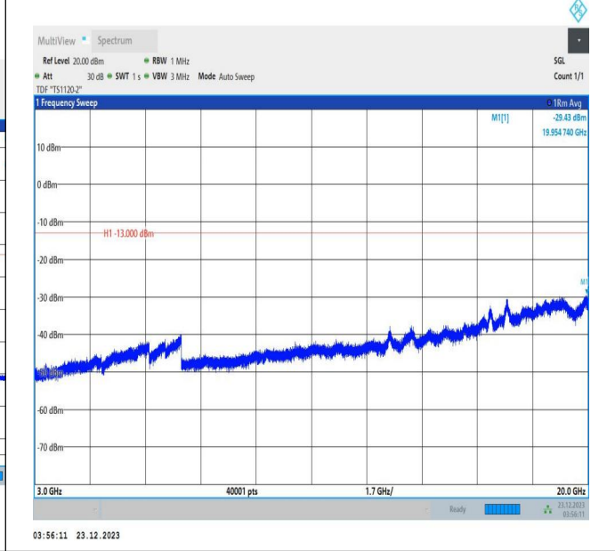
66-66-20MHz-5MHz-64QAM-64QAM-132072-132189-100RB #0-25RB#0-3000~20000MHz-PASS
