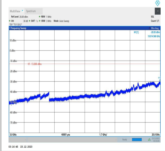
66-66-20MHz-5MHz-16QAM-16QAM-132072-132189-100RB #0-25RB#0-3000~20000MHz-PASS
