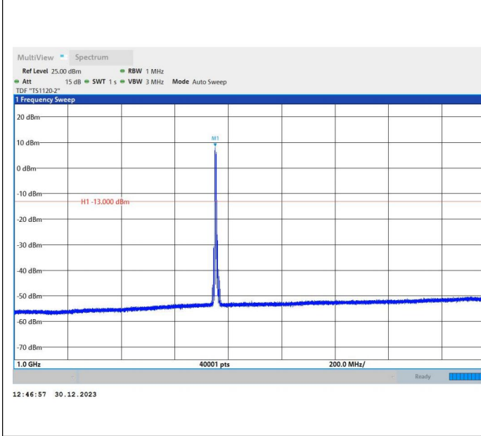
66-66-20MHz-5MHz-64QAM-64QAM-132072-132189-100RB #0-25RB#0-1000~3000MHz-PASS
