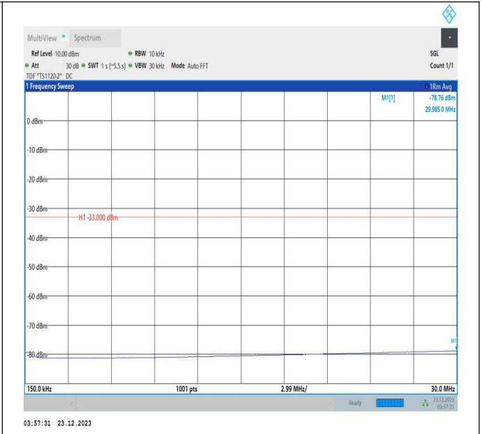
66-66-20MHz-5MHz-QPSK-QPSK-132397-132514-1RB#0-0 RB#0-0.15~30MHz-PASS
