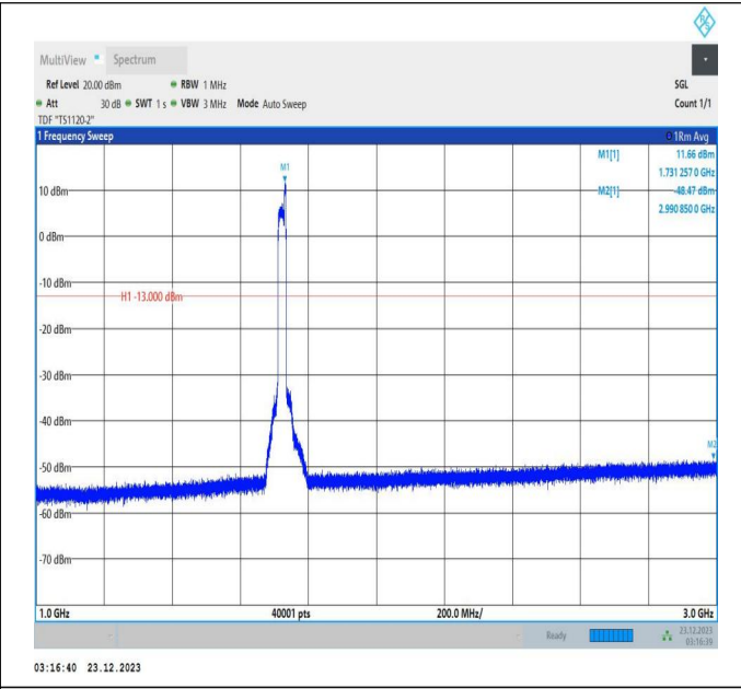
66-66-20MHz-5MHz-16QAM-16QAM-132072-132189-100RB #0-25RB#0-1000~3000MHz-PASS
