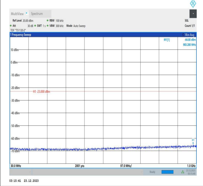
66-66-20MHz-5MHz-QPSK-QPSK-132072-132189-100RB#0 -25RB#0-30~1000MHz-PASS
