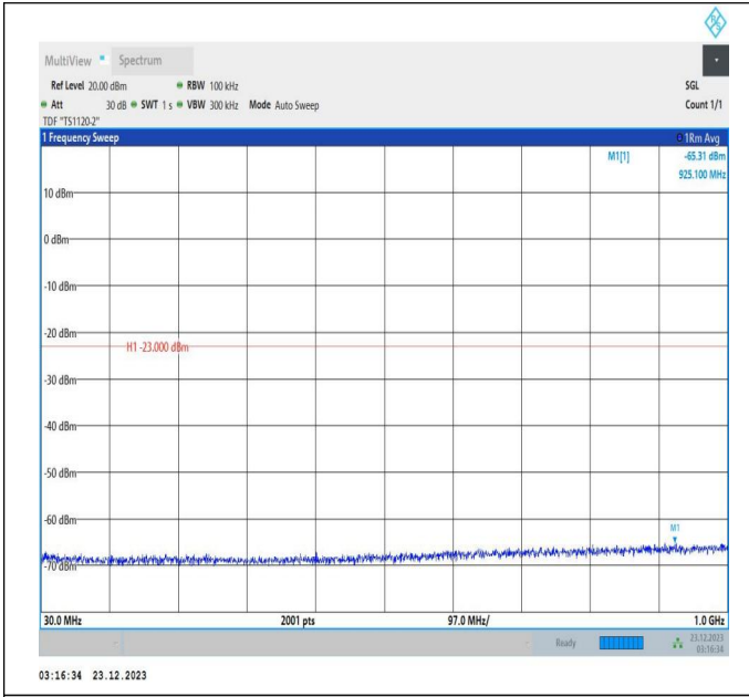
66-66-20MHz-5MHz-16QAM-16QAM-132072-132189-100RB #0-25RB#0-30~1000MHz-PASS
