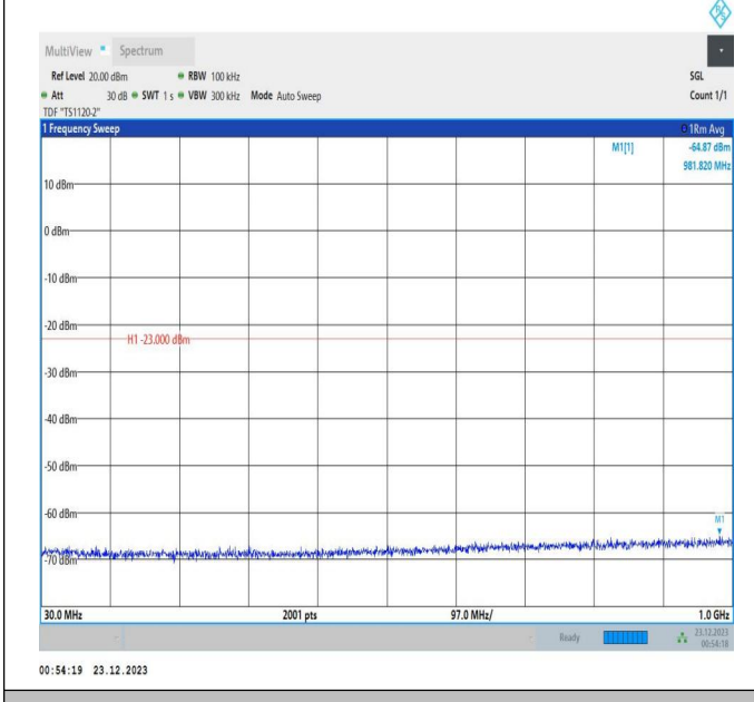
66-66-20MHz-5MHz-QPSK-QPSK-132072-132189-1RB#0-0 RB#0-30~1000MHz-PASS
