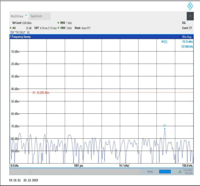
66-66-20MHz-5MHz-QPSK-QPSK-132072-132189-100RB#0 -25RB#0-0.009~0.15MHz-PASS
