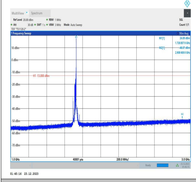
66-66-20MHz-5MHz-QPSK-QPSK-132072-132189-1RB#99-ORB#0-1000~3000MHz-PASS
