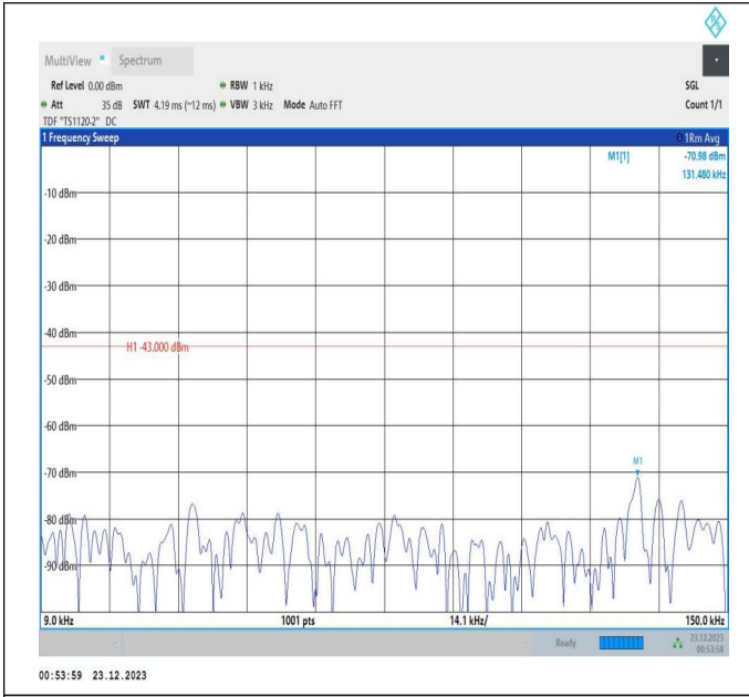
66-66-20MHz-5MHz-QPSK-QPSK-132072-132189-1RB#0-0 RB#0-0.009~0.15MHz-PASS
