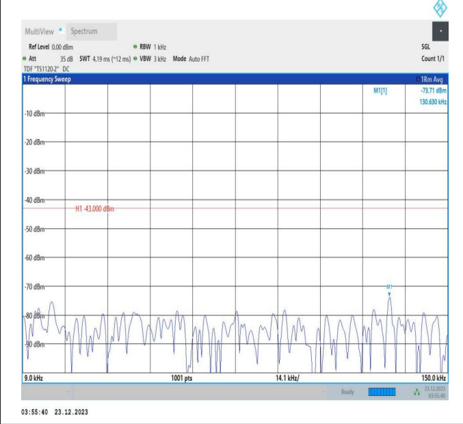
66-66-20MHz-5MHz-64QAM-64QAM-132072-132189-100RB #0-25RB#0-0.009~0.15MHz-PASS
