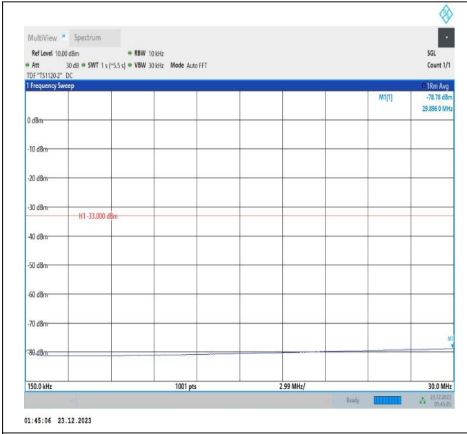
66-66-20MHz-5MHz-QPSK-QPSK-132072-132189-1RB#99-ORB#0-0.15~30MHz-PASS
