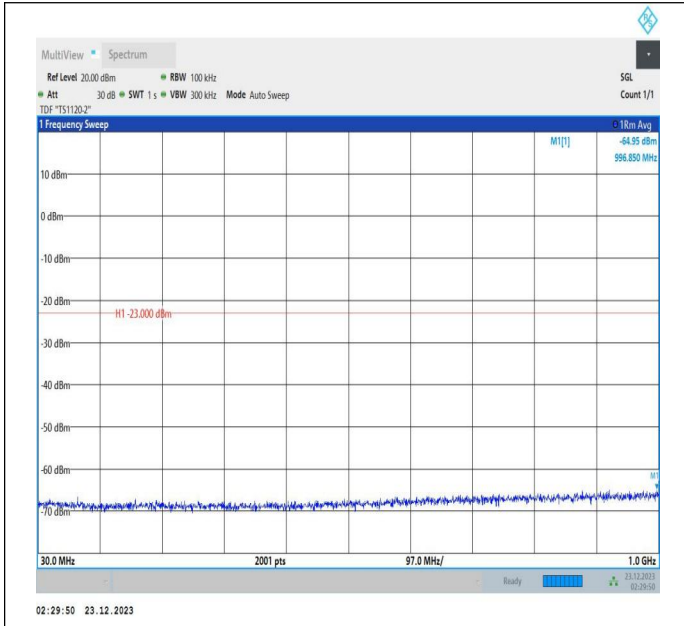
66-66-20MHz-5MHz-QPSK-QPSK-132072-132189-1RB#0-1 RB#24-30~1000MHz-PASS
