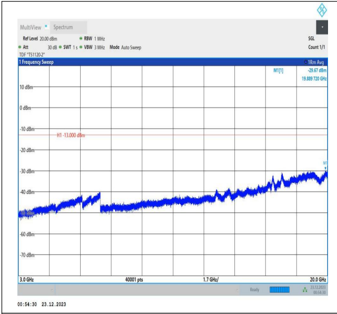
66-66-20MHz-5MHz-QPSK-QPSK-132072-132189-1RB#0-0 RB#0-3000~20000MHz-PASS
