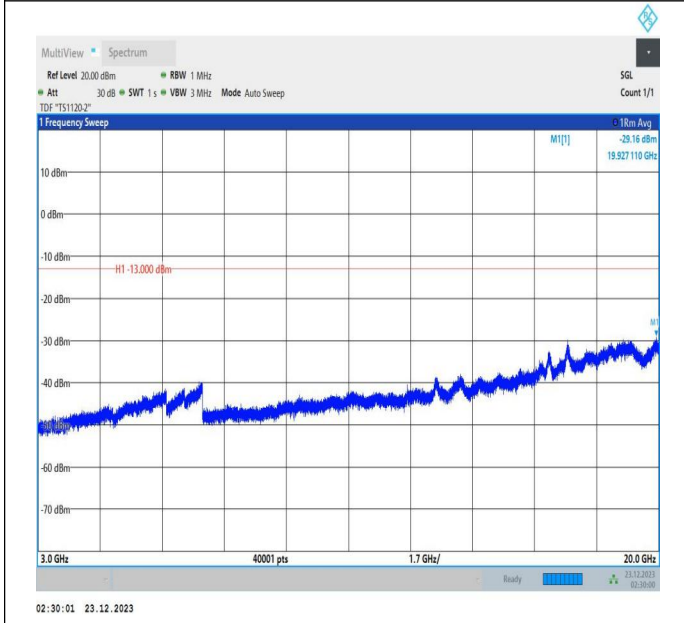
66-66-20MHz-5MHz-QPSK-QPSK-132072-132189-1RB#0-1 RB#24-3000~20000MHz-PASS
