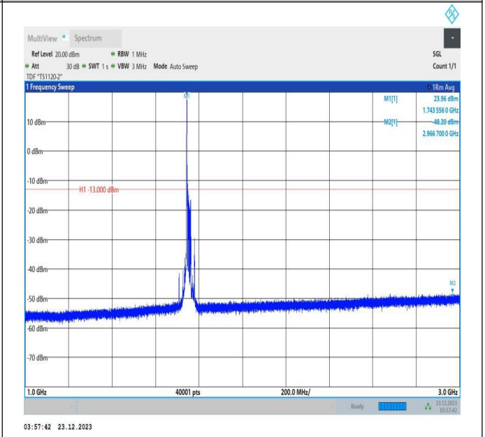
66-66-20MHz-5MHz-QPSK-QPSK-132397-132514-1RB#0-0 RB#0-1000~3000MHz-PASS
