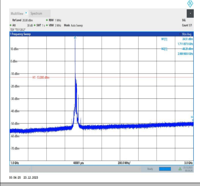
66-66-20MHz-5MHz-QPSK-QPSK-132072-132189-1RB#0-0 RB#0-1000~3000MHz-PASS
