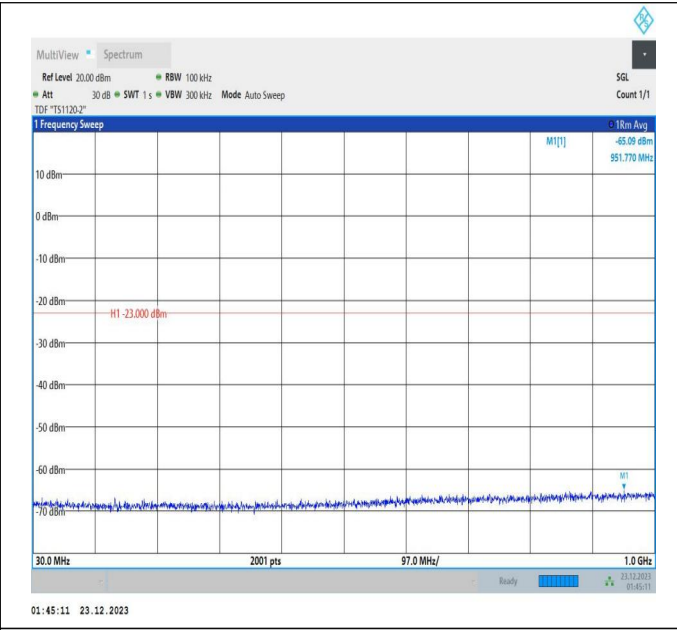
66-66-20MHz-5MHz-QPSK-QPSK-132072-132189-1RB#99-ORB#0-30~1000MHz-PASS
