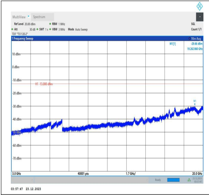
66-66-20MHz-5MHz-QPSK-QPSK-132397-132514-1RB#0-0 RB#0-3000~20000MHz-PASS
