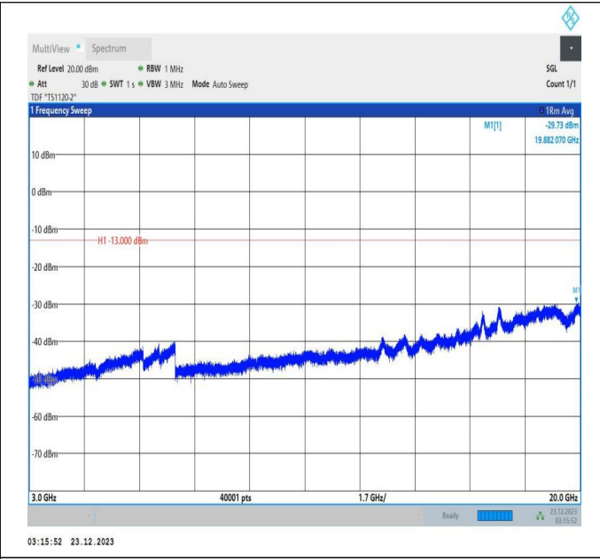
66-66-20MHz-5MHz-QPSK-QPSK-132072-132189-100RB#0 -25RB#0-3000~20000MHz-PASS
