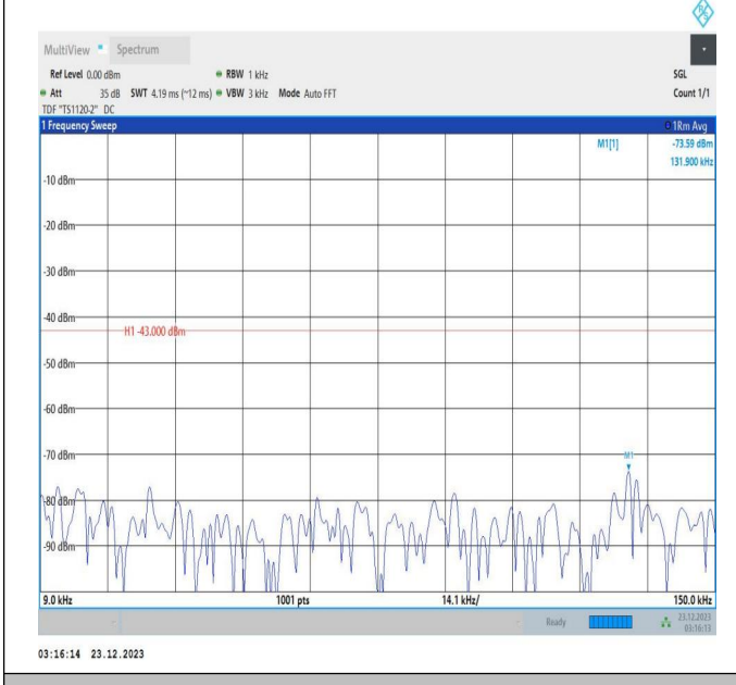
66-66-20MHz-5MHz-16QAM-16QAM-132072-132189-100RB #0-25RB#0-0.009~0.15MHz-PASS
