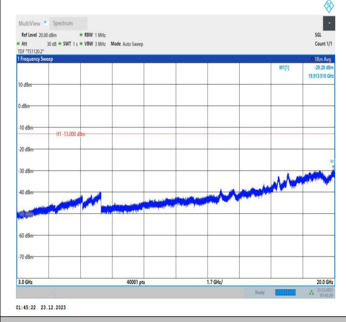
66-66-20MHz-5MHz-QPSK-QPSK-132072-132189-1RB#99-ORB#0-3000~20000MHz-PASS
