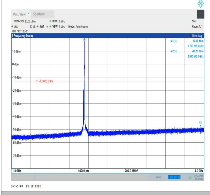
66-66-15MHz-20MHz-QPSK-QPSK-132401-132572-1RB#74 -ORB#0-1000~3000MHz-PASS
