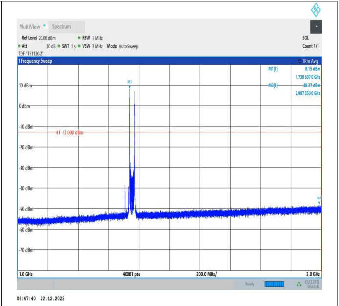
66-66-15MHz-20MHz-QPSK-QPSK-132325-132496-1RB#0-1RB#99-1000~3000MHz-PASS
