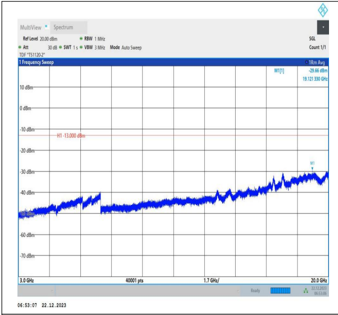
66-66-15MHz-20MHz-QPSK-QPSK-132401-132572-1RB#0-ORB#0-3000~20000MHz-PASS
