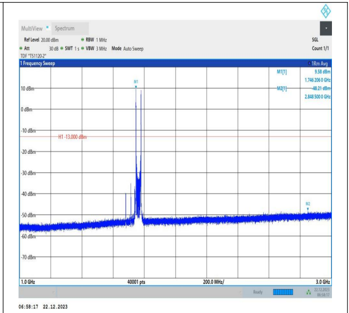
66-66-15MHz-20MHz-QPSK-QPSK-132401-132572-1RB#0-1RB#99-1000~3000MHz-PASS
