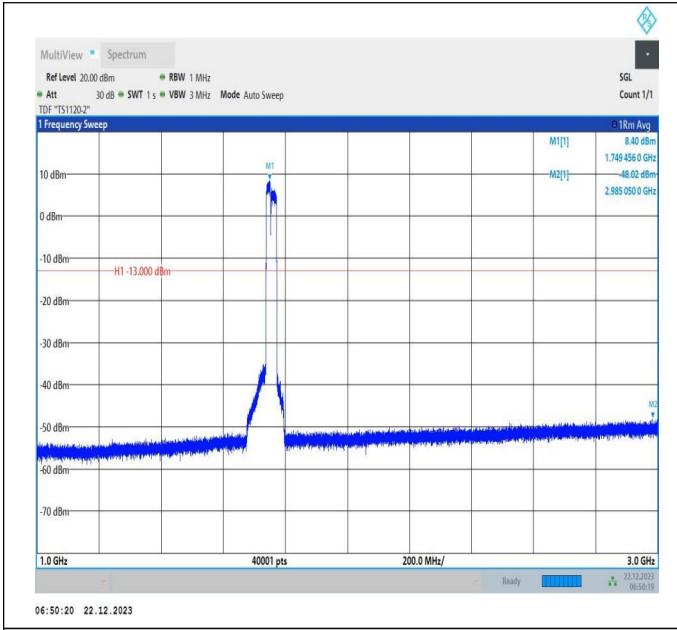
66-66-15MHz-20MHz-QPSK-QPSK-132325-132496-75RB#0 -100RB#0-1000~3000MHz-PASS
