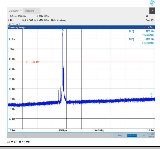
66-66-15MHz-20MHz-QPSK-QPSK-132401-132572-1RB#0-ORB#0-1000~3000MHz-PASS
