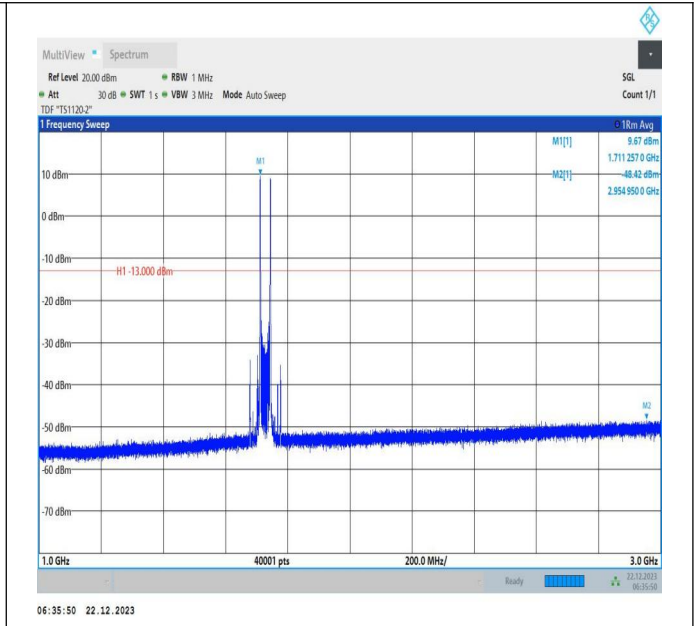
66-66-15MHz-20MHz-QPSK-QPSK-132050-132221-1RB#0-1RB#99-1000~3000MHz-PASS
