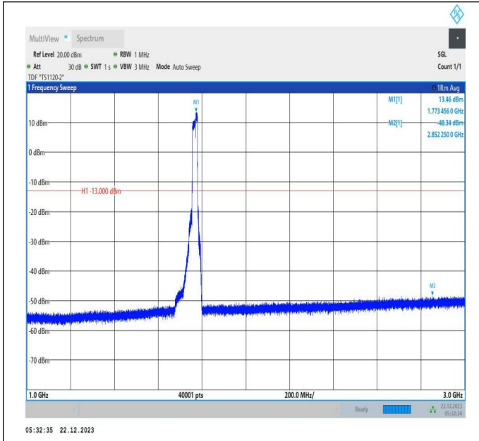
66-66-15MHz-10MHz-QPSK-QPSK-132499-132619-75RB#0 -50RB#0-1000~3000MHz-PASS
