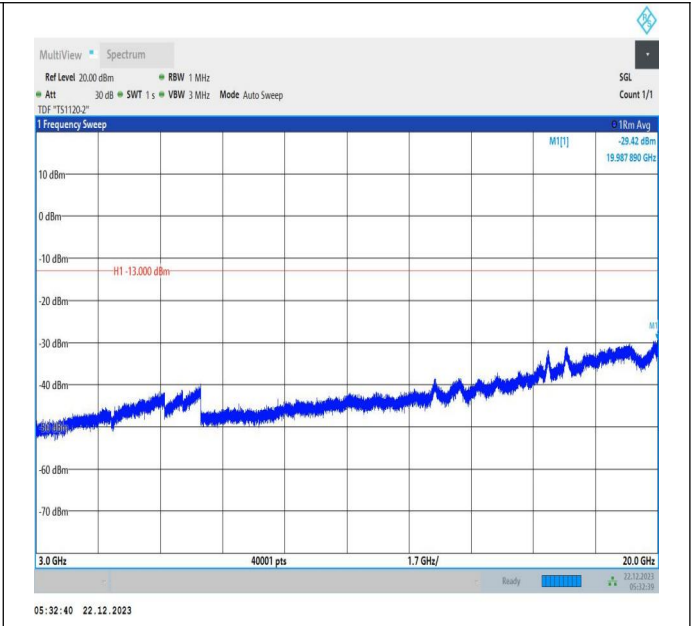
66-66-15MHz-10MHz-QPSK-QPSK-132499-132619-75RB#0 -50RB#0-3000~20000MHz-PASS
