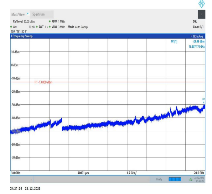
66-66-15MHz-10MHz-QPSK-QPSK-132499-132619-1RB#74 -ORB#0-3000~20000MHz-PASS
