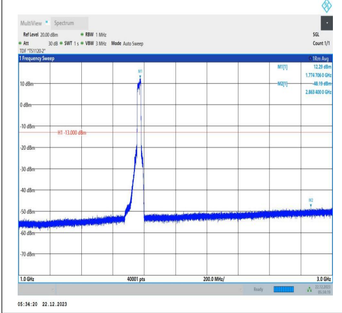
66-66-15MHz-10MHz-64QAM-64QAM-132499-132619-75RB #0-50RB#0-1000~3000MHz-PASS
