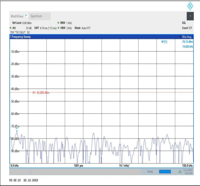
66-66-15MHz-10MHz-QPSK-QPSK-132499-132619-75RB#0 -50RB#0-0.009~0.15MHz-PASS
