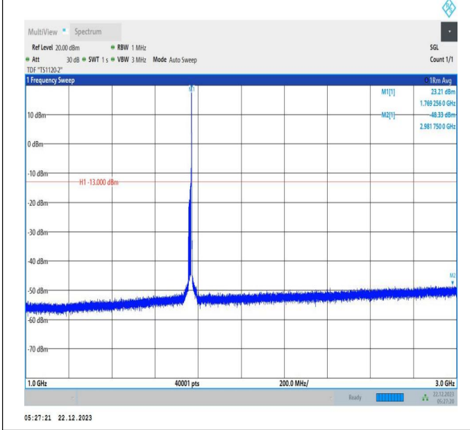
66-66-15MHz-10MHz-QPSK-QPSK-132499-132619-1RB#74 -ORB#0-1000~3000MHz-PASS
