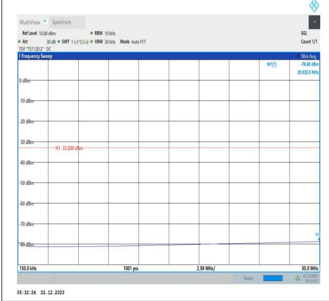
66-66-15MHz-10MHz-QPSK-QPSK-132499-132619-75RB#0 -50RB#0-0.15~30MHz-PASS
