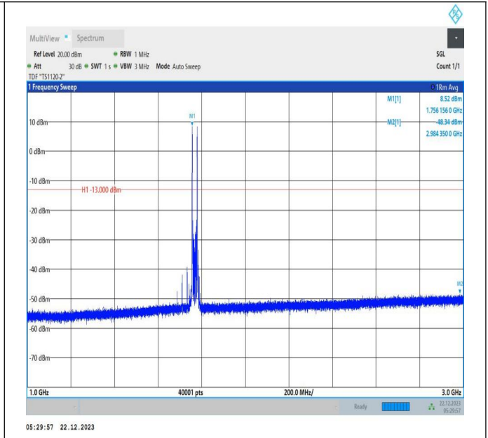
66-66-15MHz-10MHz-QPSK-QPSK-132499-132619-1RB#0-1RB#49-1000~3000MHz-PASS
