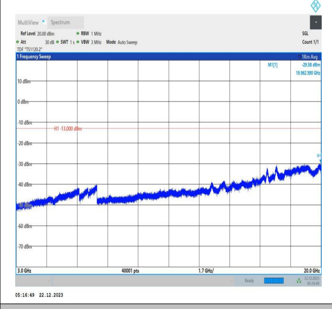
66-66-15MHz-10MHz-QPSK-QPSK-132373-132493-1RB#74 -ORB#0-3000~20000MHz-PASS
