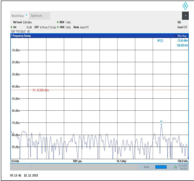
66-66-15MHz-10MHz-QPSK-QPSK-132373-132493-1RB#0-ORB#0-0.009~0.15MHz-PASS
