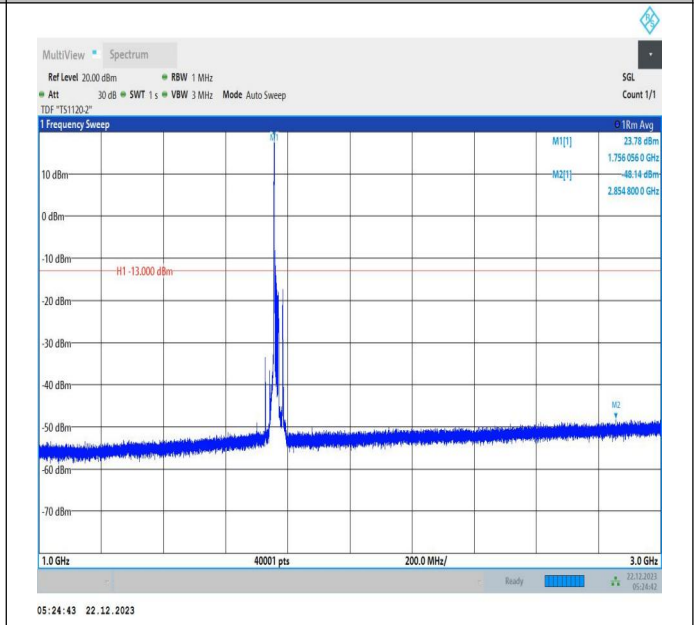
66-66-15MHz-10MHz-QPSK-QPSK-132499-132619-1RB#0-ORB#0-1000~3000MHz-PASS
