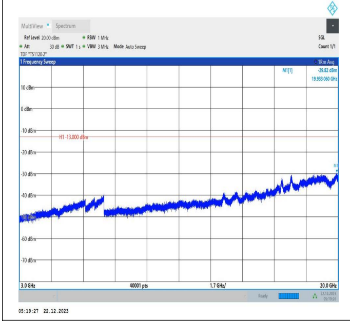
66-66-15MHz-10MHz-QPSK-QPSK-132373-132493-1RB#0-1RB#49-3000~20000MHz-PASS
