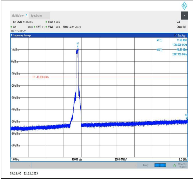
66-66-15MHz-10MHz-QPSK-QPSK-132373-132493-75RB#0 -50RB#0-1000~3000MHz-PASS
