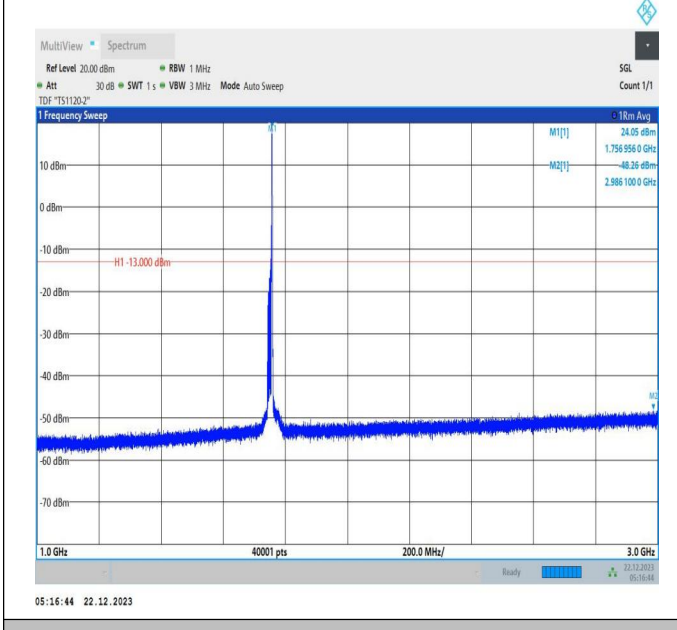
66-66-15MHz-10MHz-QPSK-QPSK-132373-132493-1RB#74 -ORB#0-1000~3000MHz-PASS
