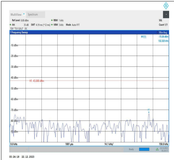
66-66-15MHz-10MHz-QPSK-QPSK-132499-132619-1RB#0-ORB#0-0.009~0.15MHz-PASS
