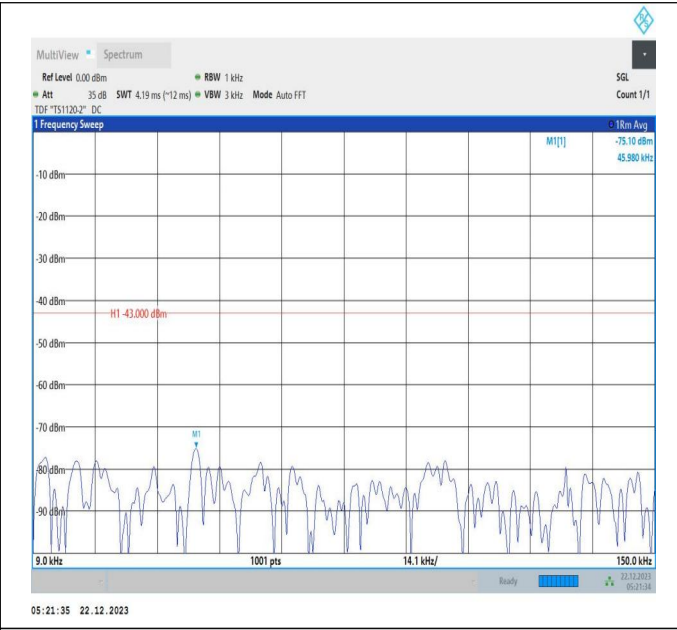
66-66-15MHz-10MHz-QPSK-QPSK-132373-132493-75RB#0-50RB#0-0.009~0.15MHz-PASS
