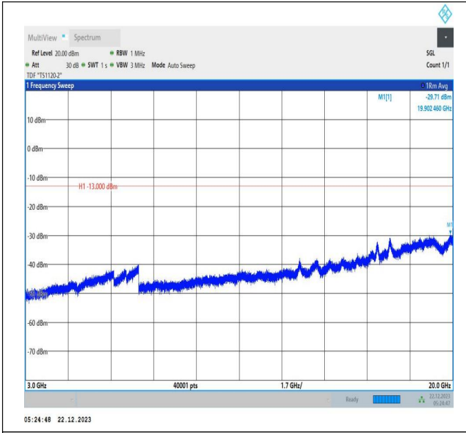
66-66-15MHz-10MHz-QPSK-QPSK-132499-132619-1RB#0-ORB#0-3000~20000MHz-PASS
