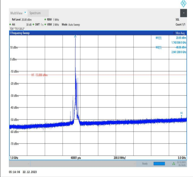
66-66-15MHz-10MHz-QPSK-QPSK-132373-132493-1RB#0-ORB#0-1000~3000MHz-PASS
