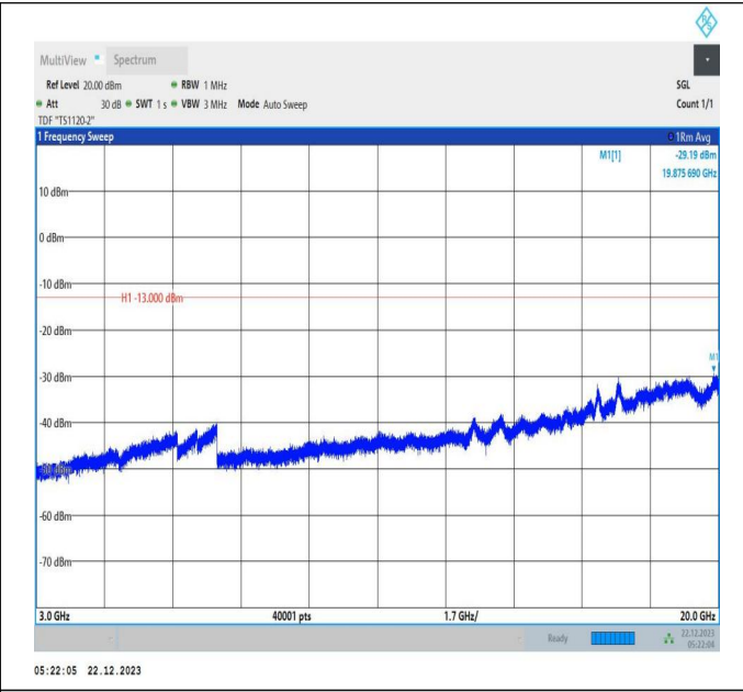
66-66-15MHz-10MHz-QPSK-QPSK-132373-132493-75RB#0 -50RB#0-3000~20000MHz-PASS
