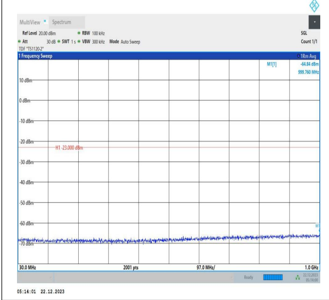
66-66-15MHz-10MHz-QPSK-QPSK-132373-132493-1RB#0-ORB#0-30~1000MHz-PASS
