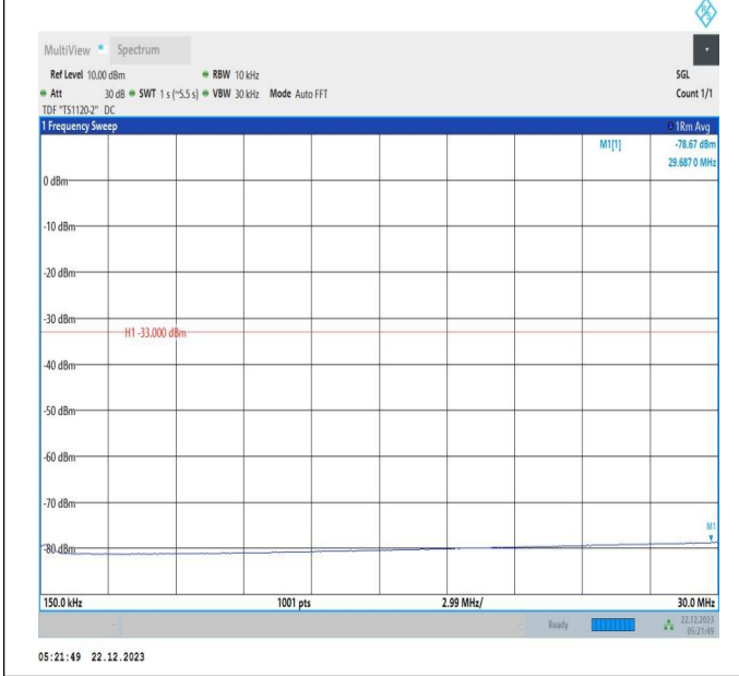
66-66-15MHz-10MHz-QPSK-QPSK-132373-132493-75RB#0-50RB#0-0.15~30MHz-PASS
