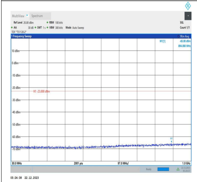
66-66-15MHz-10MHz-QPSK-QPSK-132499-132619-1RB#0-ORB#0-30~1000MHz-PASS
