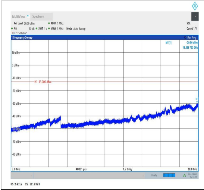
66-66-15MHz-10MHz-QPSK-QPSK-132373-132493-1RB#0-ORB#0-3000~20000MHz-PASS
