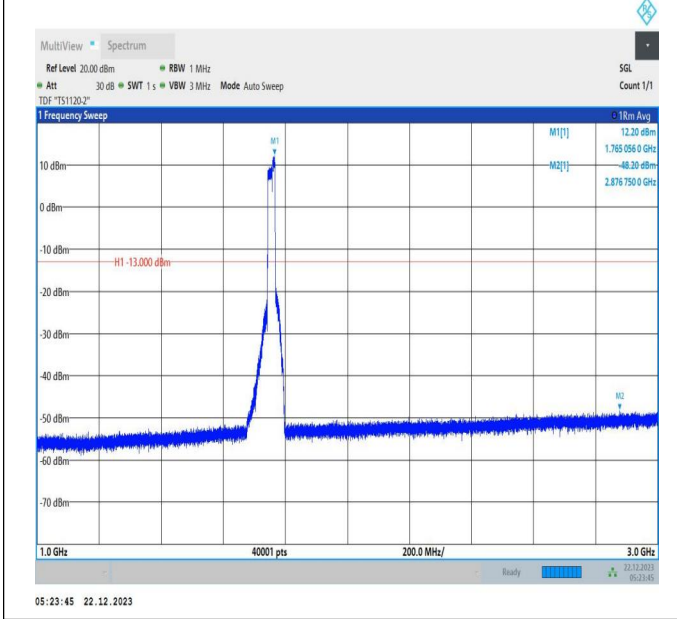
66-66-15MHz-10MHz-64QAM-64QAM-132373-132493-75RB #0-50RB#0-1000~3000MHz-PASS
