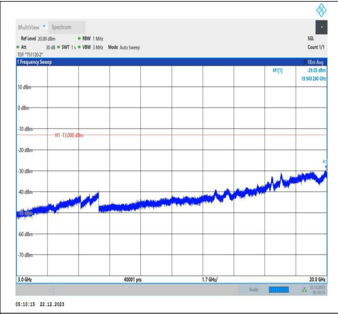
66-66-15MHz-10MHz-QPSK-QPSK-132047-132167-75RB#0 -50RB#0-3000~20000MHz-PASS
