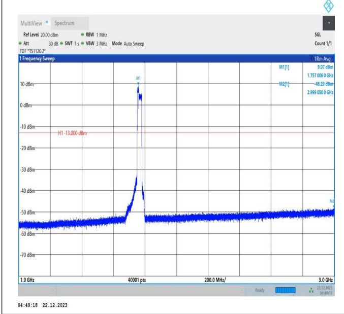
66-66-10MHz-20MHz-64QAM-64QAM-132428-132572-50RB #0-100RB#0-1000~3000MHz-PASS
