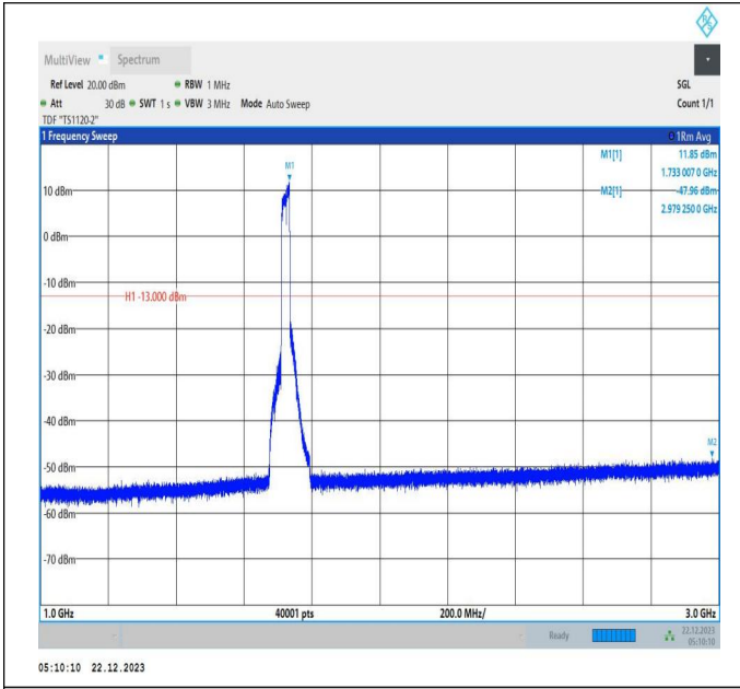
66-66-15MHz-10MHz-QPSK-QPSK-132047-132167-75RB#0 -50RB#0-1000~3000MHz-PASS
