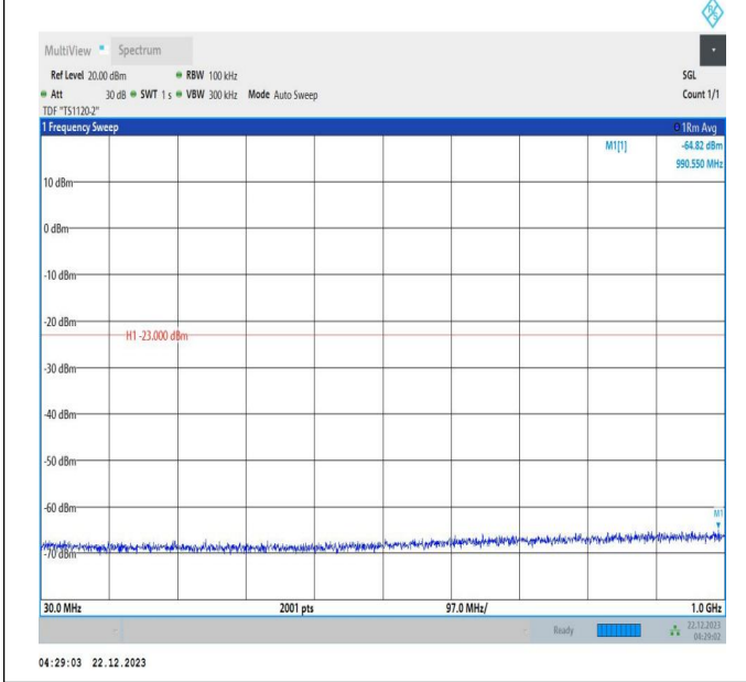
66-66-10MHz-20MHz-QPSK-QPSK-132328-132472-1RB#0-ORB#0-30~1000MHz-PASS
