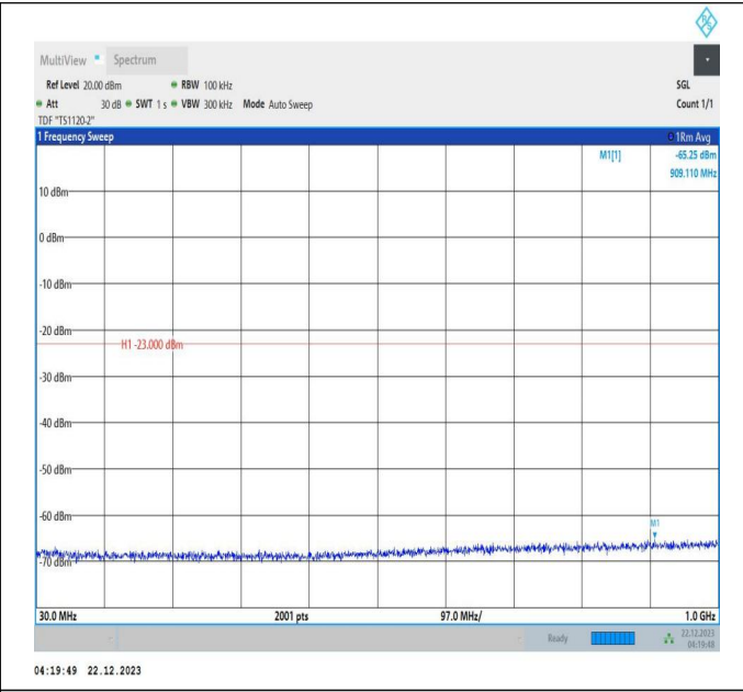
66-66-10MHz-20MHz-QPSK-QPSK-132027-132171-1RB#49 -ORB#0-30~1000MHz-PASS
