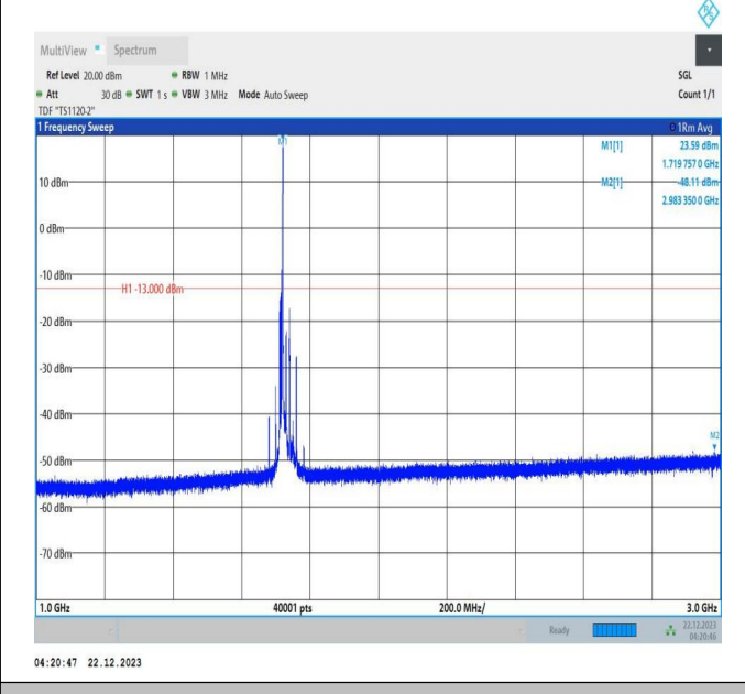
66-66-10MHz-20MHz-16QAM-16QAM-132027-132171-1RB# 49-ORB#0-1000~3000MHz-PASS
