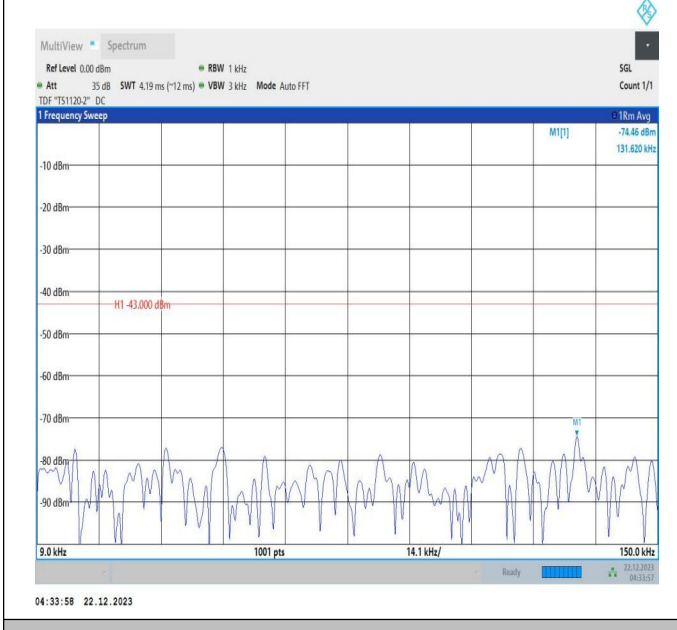
66-66-10MHz-20MHz-QPSK-QPSK-132328-132472-1RB#0- 1RB#99-0.009~0.15MHz-PASS
