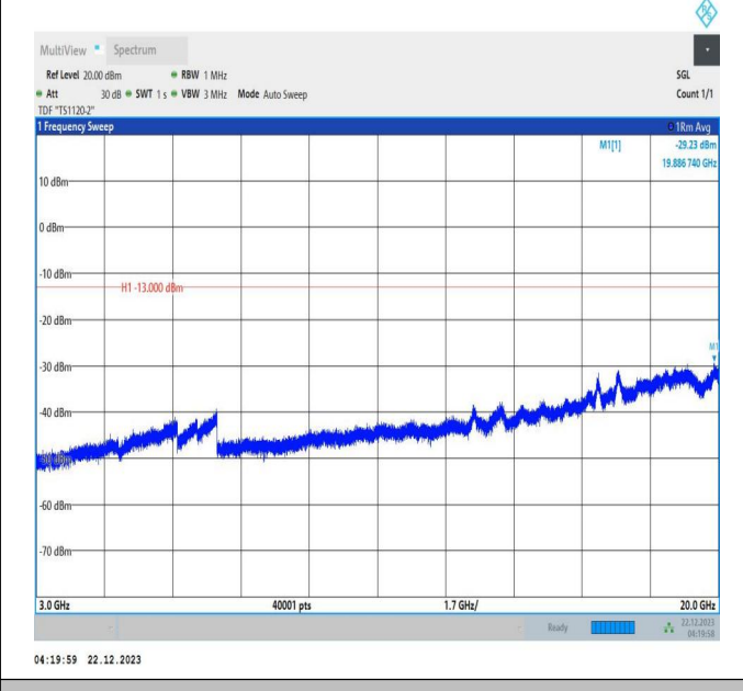
66-66-10MHz-20MHz-QPSK-QPSK-132027-132171-1RB#49 -ORB#0-3000~20000MHz-PASS
