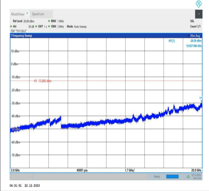
66-66-10MHz-20MHz-QPSK-QPSK-132328-132472-1RB#49 -ORB#0-3000~20000MHz-PASS
