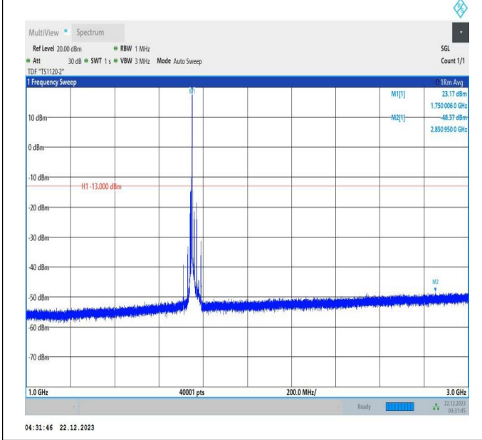
66-66-10MHz-20MHz-QPSK-QPSK-132328-132472-1RB#49 -ORB#0-1000~3000MHz-PASS
