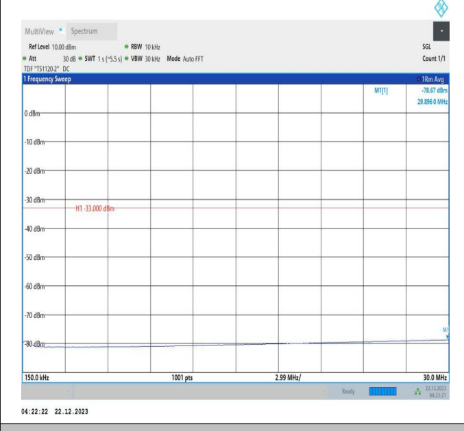
66-66-10MHz-20MHz-QPSK-QPSK-132027-132171-1RB#0- 1RB#99-0.15~30MHz-PASS
