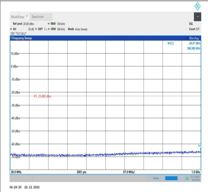
66-66-10MHz-20MHz-64QAM-64QAM-132027-132171-50RB #0-100RB#0-30~1000MHz-PASS
