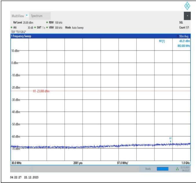
66-66-10MHz-20MHz-QPSK-QPSK-132027-132171-1RB#0-1RB#99-30~1000MHz-PASS
