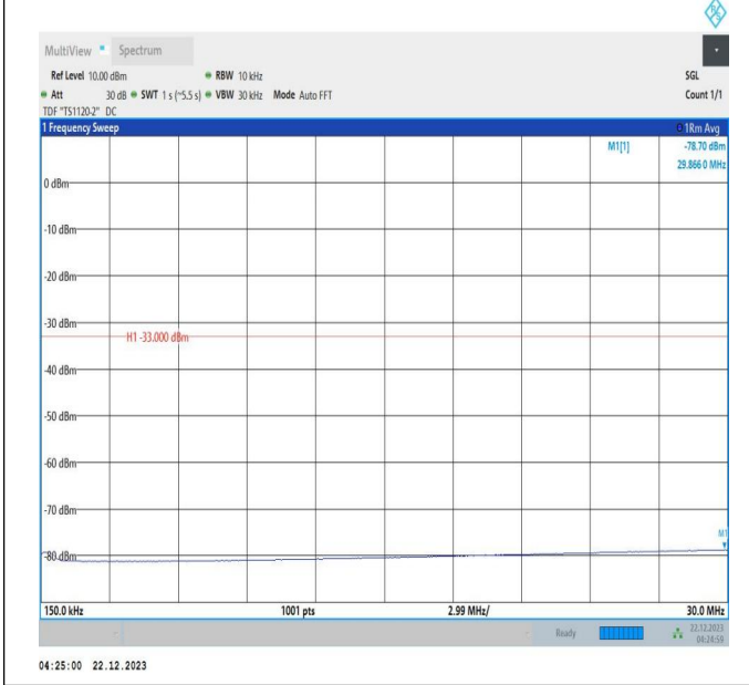
66-66-10MHz-20MHz-QPSK-QPSK-132027-132171-50RB#0-100RB#0-0.15~30MHz-PASS
