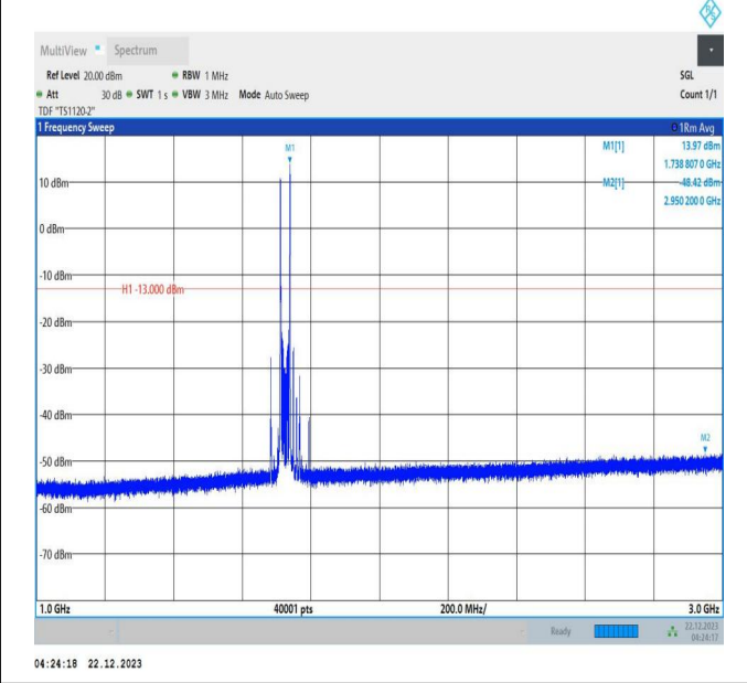
66-66-10MHz-20MHz-64QAM-64QAM-132027-132171-1RB# 0-1RB#99-1000~3000MHz-PASS
