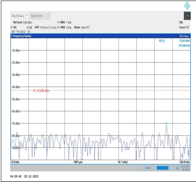
66-66-10MHz-20MHz-QPSK-QPSK-132328-132472-1RB#0-ORB#0-0.009~0.15MHz-PASS
