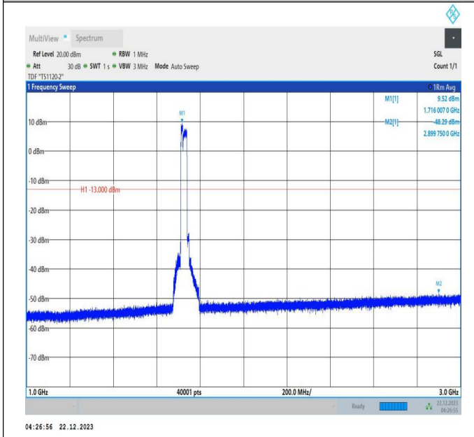
66-66-10MHz-20MHz-64QAM-64QAM-132027-132171-50RB #0-100RB#0-1000~3000MHz-PASS
