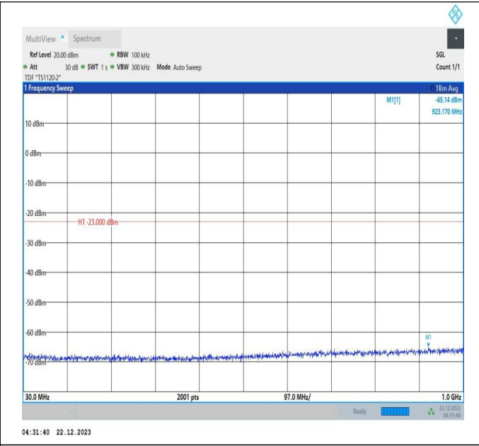
66-66-10MHz-20MHz-QPSK-QPSK-132328-132472-1RB#49 -ORB#0-30~1000MHz-PASS
