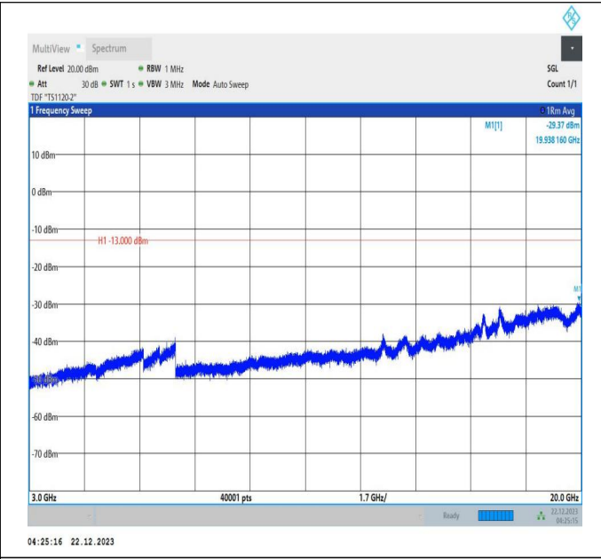
66-66-10MHz-20MHz-QPSK-QPSK-132027-132171-50RB#0 -100RB#0-3000~20000MHz-PASS
