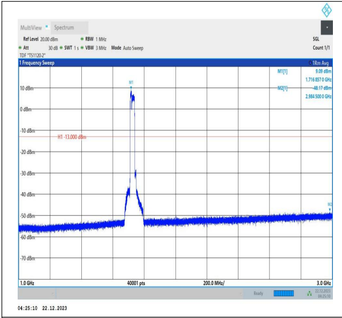
66-66-10MHz-20MHz-QPSK-QPSK-132027-132171-50RB#0 -100RB#0-1000~3000MHz-PASS
