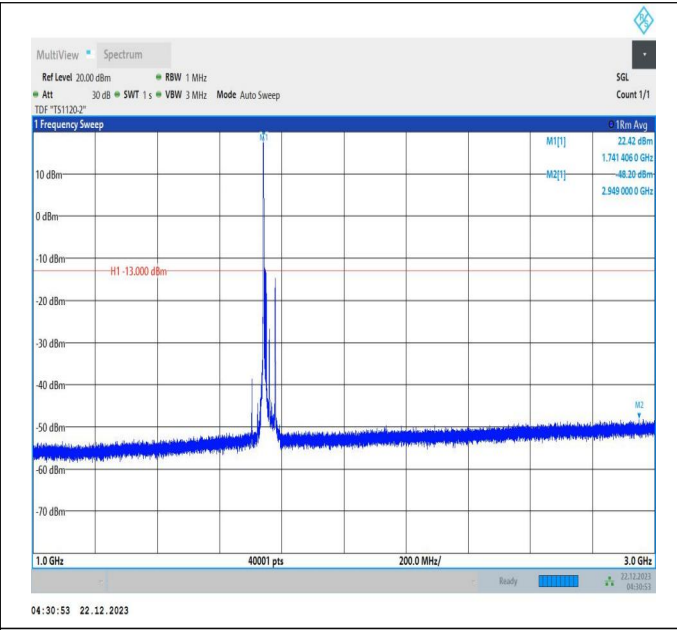
66-66-10MHz-20MHz-64QAM-64QAM-132328-132472-1RB# 0-ORB#0-1000~3000MHz-PASS
