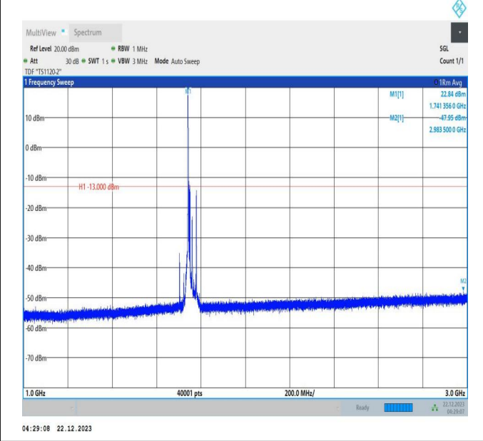
66-66-10MHz-20MHz-QPSK-QPSK-132328-132472-1RB#0-ORB#0-1000~3000MHz-PASS
