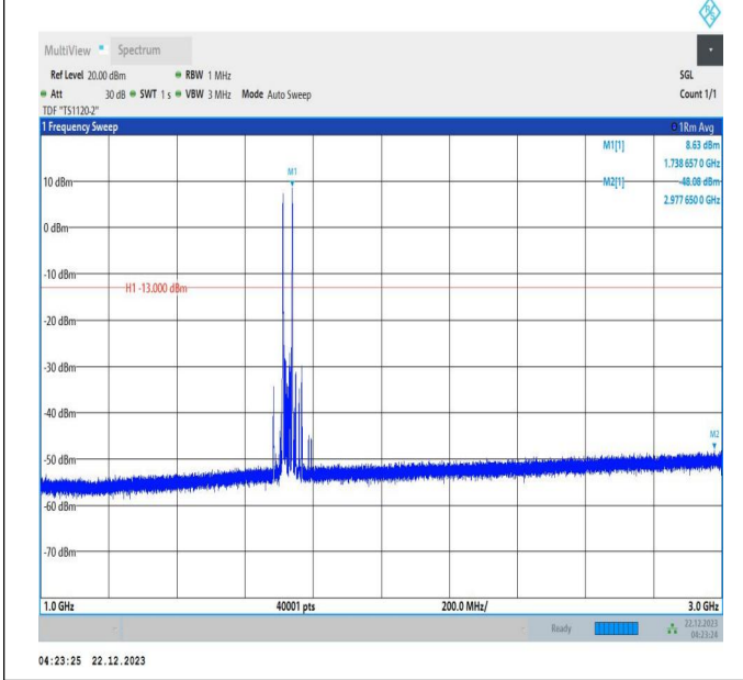
66-66-10MHz-20MHz-16QAM-16QAM-132027-132171-1RB# 0-1RB#99-1000~3000MHz-PASS
