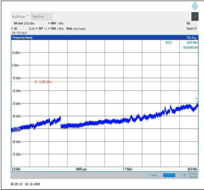
66-66-10MHz-20MHz-QPSK-QPSK-132328-132472-1RB#0-ORB#0-3000~20000MHz-PASS
