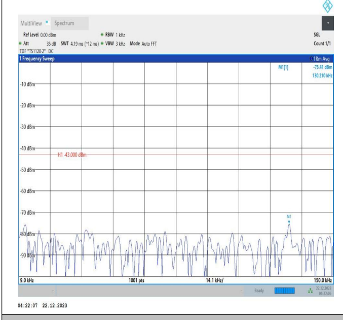
66-66-10MHz-20MHz-QPSK-QPSK-132027-132171-1RB#0- 1RB#99-0.009~0.15MHz-PASS
