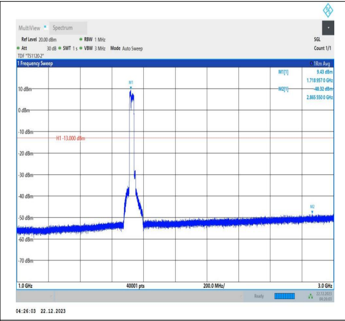
66-66-10MHz-20MHz-16QAM-16QAM-132027-132171-50RB #0-100RB#0-1000~3000MHz-PASS
