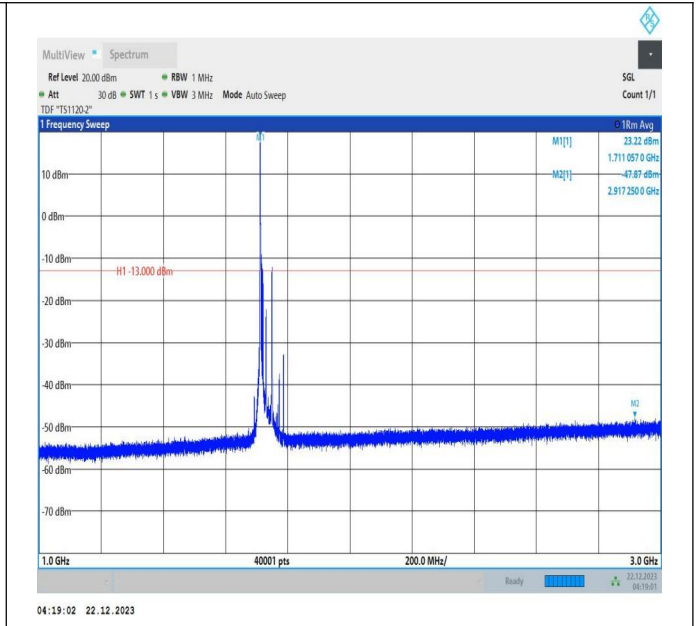
66-66-10MHz-20MHz-64QAM-64QAM-132027-132171-1RB# 0-ORB#0-1000~3000MHz-PASS
