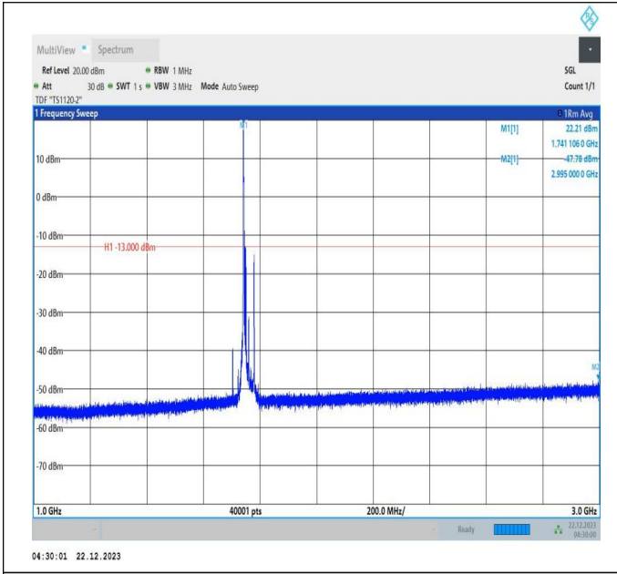
66-66-10MHz-20MHz-16QAM-16QAM-132328-132472-1RB# 0-ORB#0-1000~3000MHz-PASS
