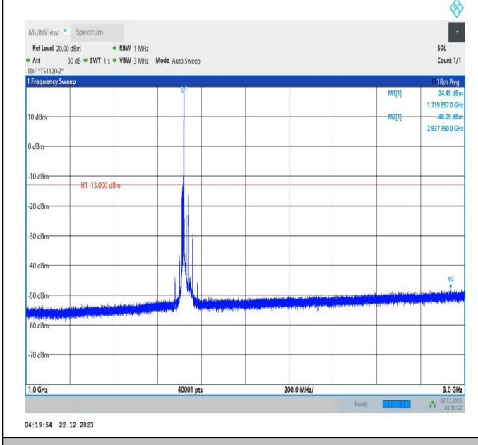
66-66-10MHz-20MHz-QPSK-QPSK-132027-132171-1RB#49 -ORB#0-1000~3000MHz-PASS
