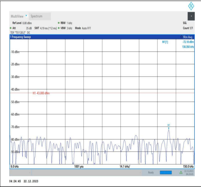
66-66-10MHz-20MHz-QPSK-QPSK-132027-132171-50RB#0-100RB#0-0.009~0.15MHz-PASS
