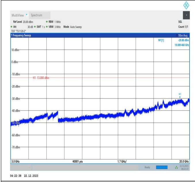
66-66-10MHz-20MHz-QPSK-QPSK-132027-132171-1RB#0-1RB#99-3000~20000MHz-PASS
