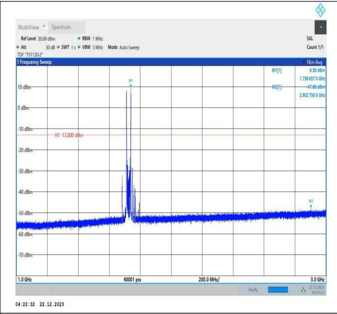
66-66-10MHz-20MHz-QPSK-QPSK-132027-132171-1RB#0-1RB#99-1000~3000MHz-PASS
