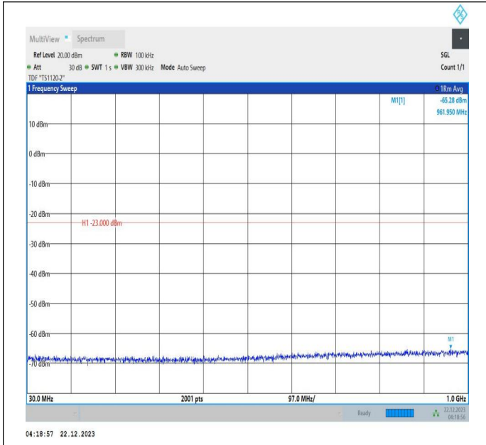
66-66-10MHz-20MHz-64QAM-64QAM-132027-132171-1RB# 0-ORB#0-30~1000MHz-PASS
