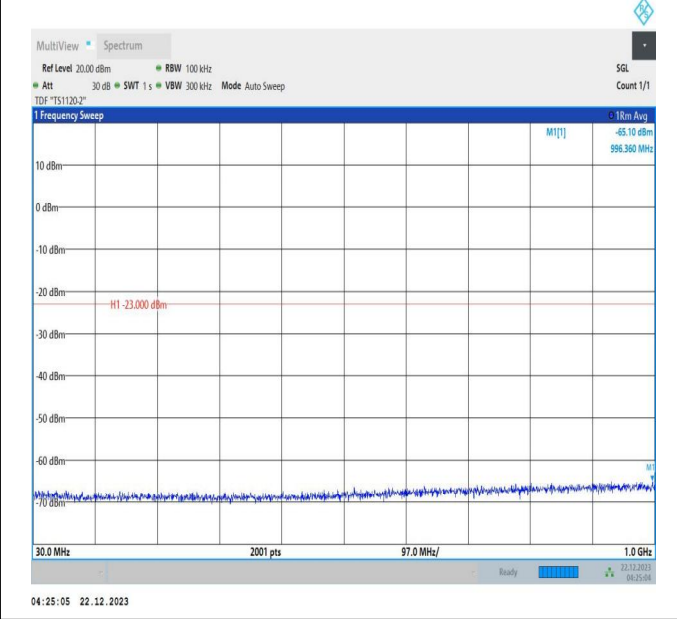
66-66-10MHz-20MHz-QPSK-QPSK-132027-132171-50RB#0-100RB#0-30~1000MHz-PASS
