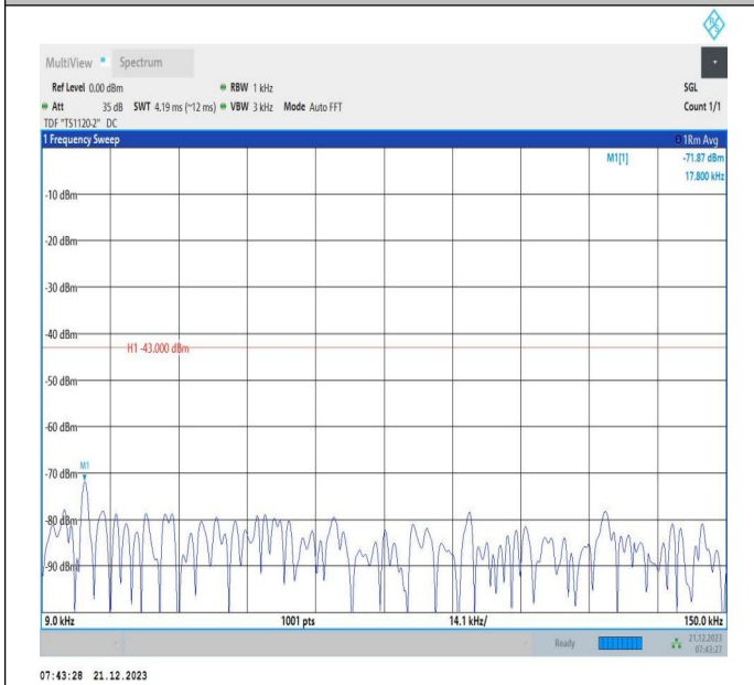
66-66-10MHz-15MHz-QPSK-QPSK-132477-132597-1RB#0- 1RB#74-0.009~0.15MHz-PASS
