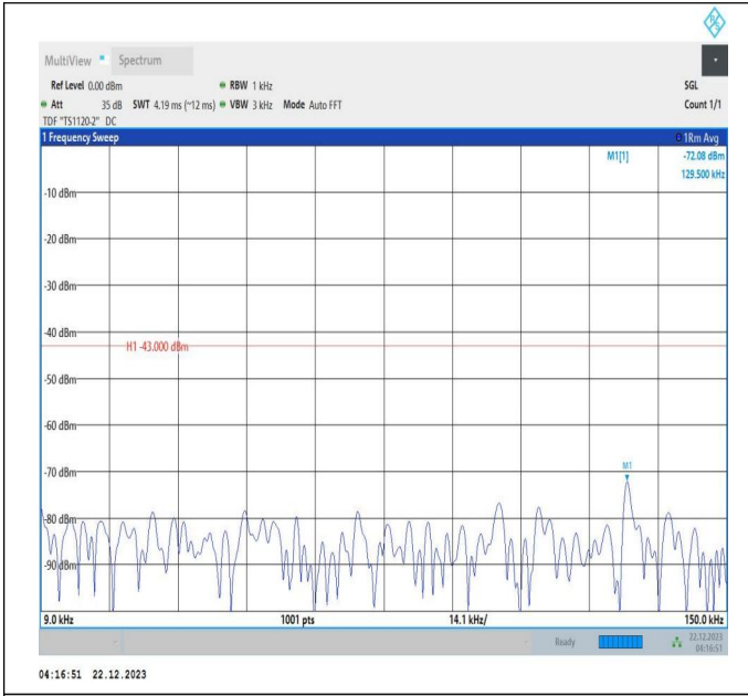
66-66-10MHz-20MHz-QPSK-QPSK-132027-132171-1RB#0-ORB#0-0.009~0.15MHz-PASS
