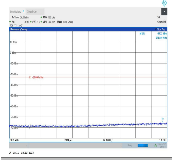
66-66-10MHz-20MHz-QPSK-QPSK-132027-132171-1RB#0-ORB#0-30~1000MHz-PASS
