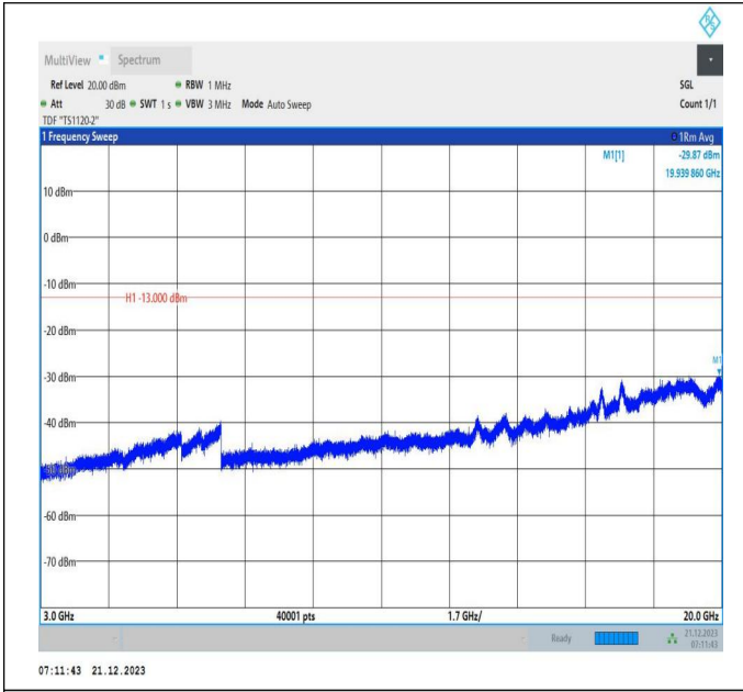
66-66-10MHz-15MHz-QPSK-QPSK-132477-132597-1RB#-ORB#0-3000~20000MHz-PASS
