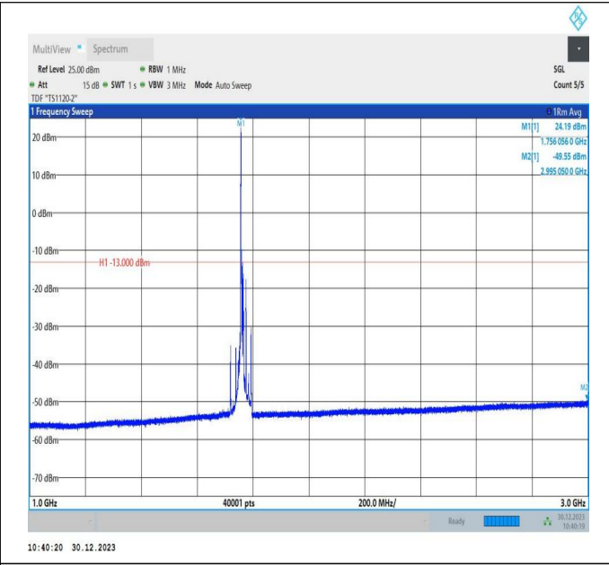
66-66-10MHz-15MHz-64QAM-64QAM-132477-132597-1RB# 0-ORB#0-1000~3000MHz-PASS
