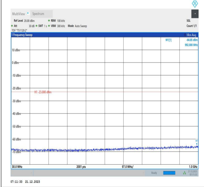
66-66-10MHz-15MHz-QPSK-QPSK-132477-132597-1RB#0-ORB#0-30~1000MHz-PASS
