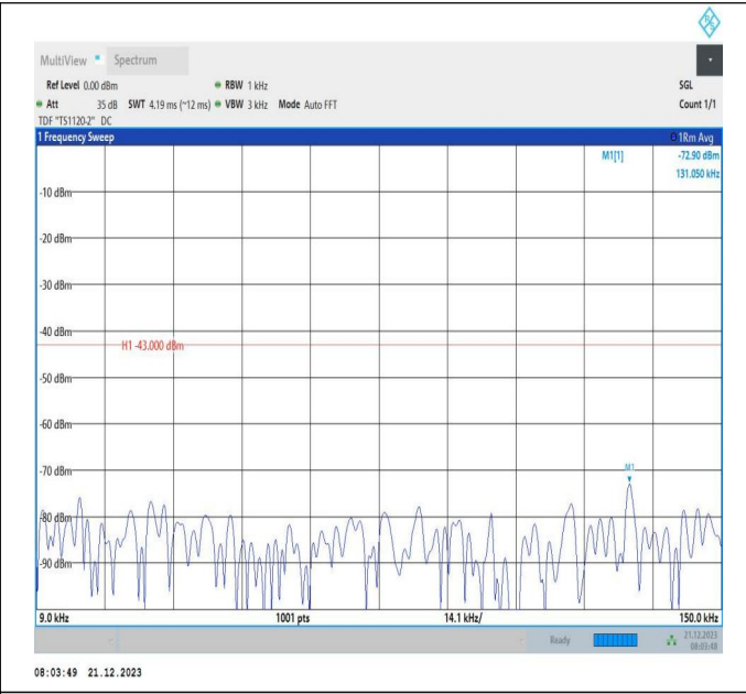
66-66-10MHz-15MHz-QPSK-QPSK-132477-132597-50RB#0 -75RB#0-0.009~0.15MHz-PASS
