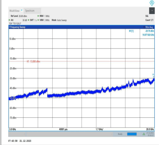
66-66-10MHz-15MHz-QPSK-QPSK-132477-132597-1RB#0-1RB#74-3000~20000MHz-PASS
