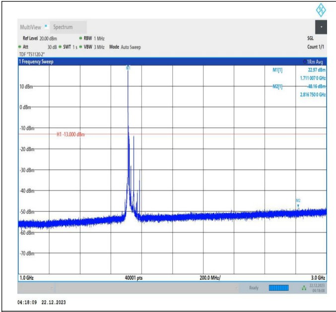
66-66-10MHz-20MHz-16QAM-16QAM-132027-132171-1RB# 0-ORB#0-1000~3000MHz-PASS
