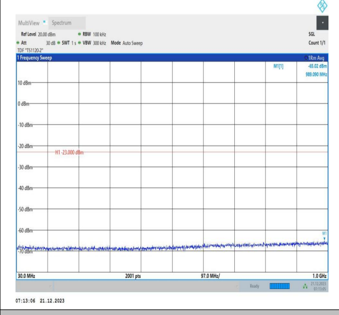
66-66-10MHz-15MHz-16QAM-16QAM-132477-132597-1RB#-0-ORB#0-30~1000MHz-PASS
