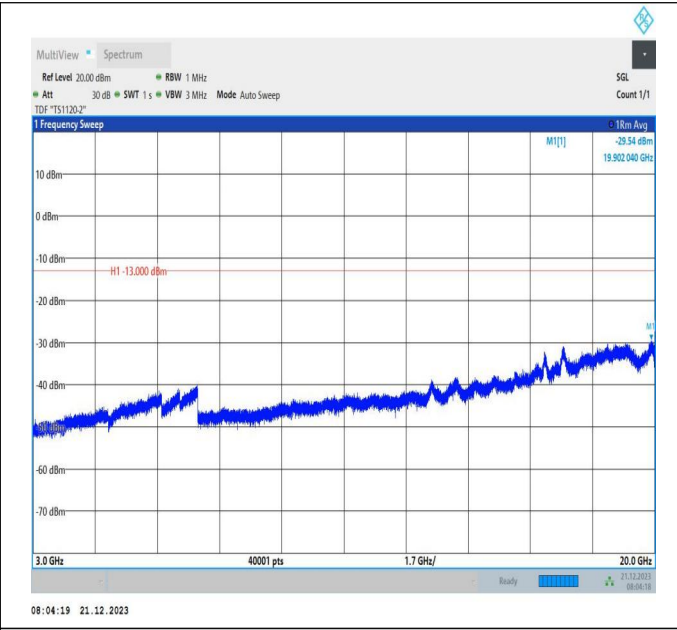
66-66-10MHz-15MHz-QPSK-QPSK-132477-132597-50RB#0 -75RB#0-3000~20000MHz-PASS
