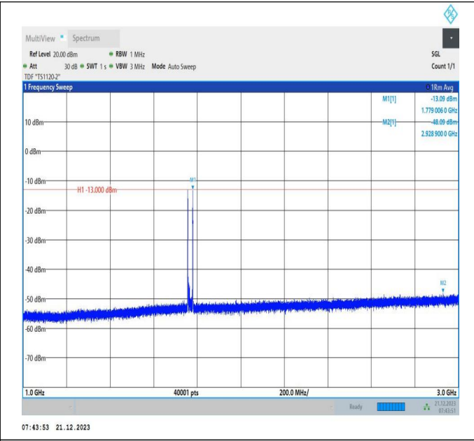
66-66-10MHz-15MHz-QPSK-QPSK-132477-132597-1RB#0-1RB#74-1000~3000MHz-PASS
