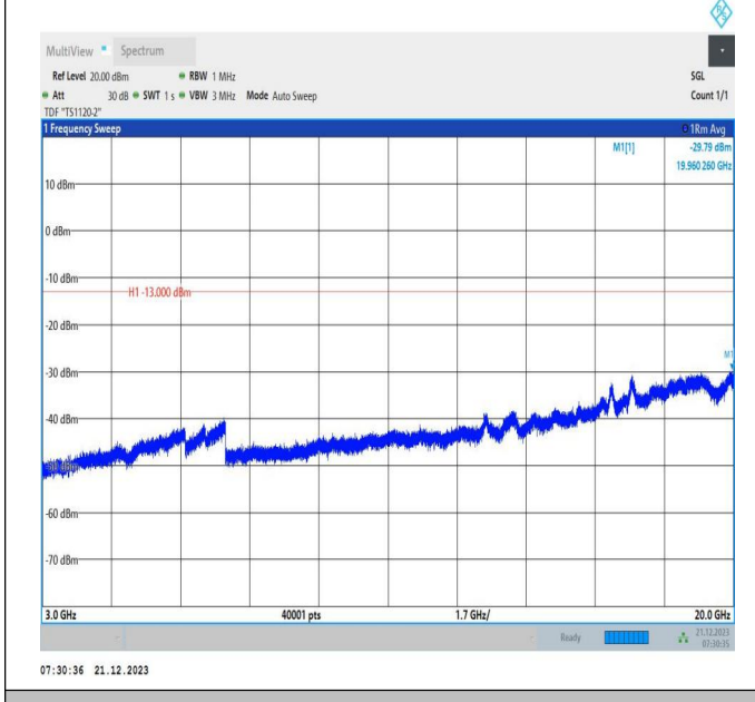
66-66-10MHz-15MHz-64QAM-64QAM-132477-132597-1RB# 0-ORB#0-3000~20000MHz-PASS
