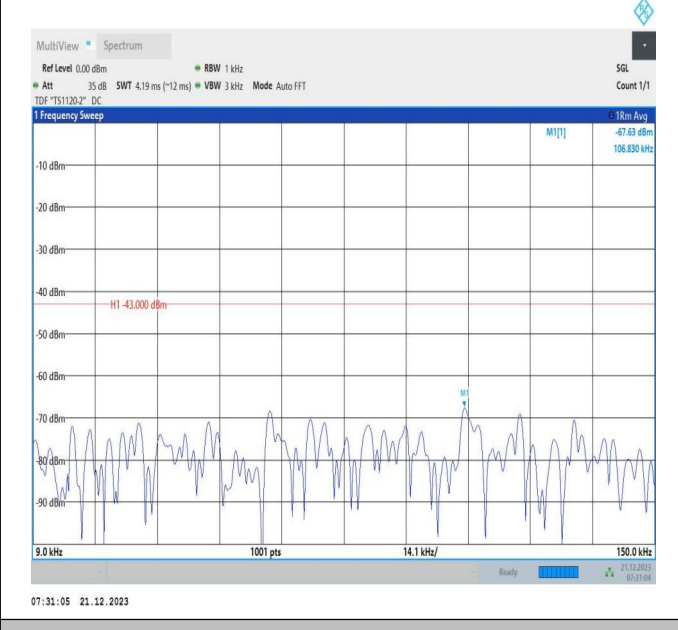
66-66-10MHz-15MHz-QPSK-QPSK-132477-132597-1RB#49 -ORB#0-0.009~0.15MHz-PASS
