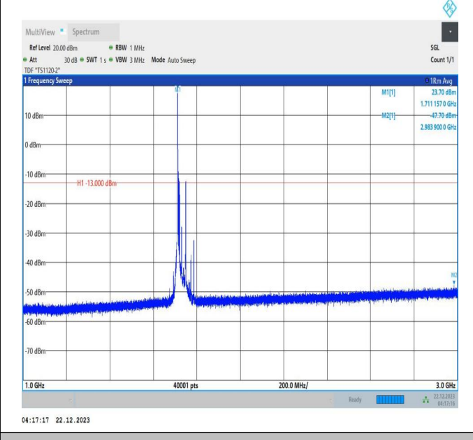
66-66-10MHz-20MHz-QPSK-QPSK-132027-132171-1RB#0-ORB#0-1000~3000MHz-PASS
