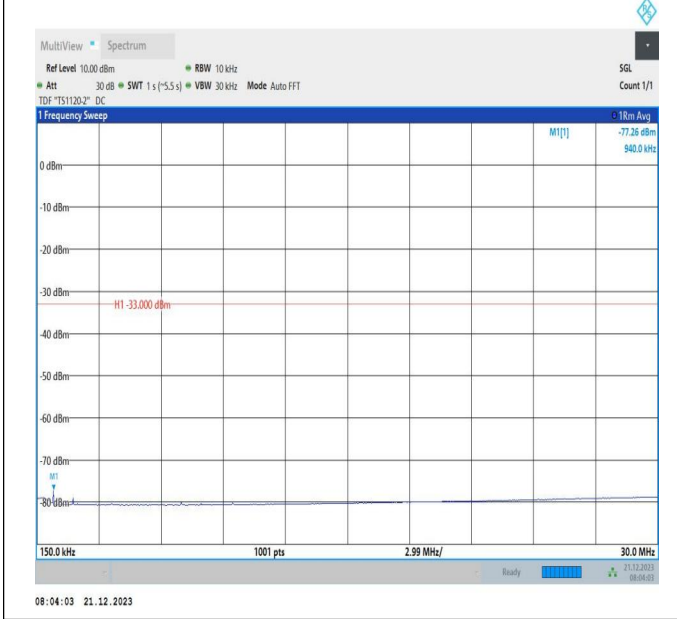
66-66-10MHz-15MHz-QPSK-QPSK-132477-132597-50RB#0 -75RB#0-0.15~30MHz-PASS
