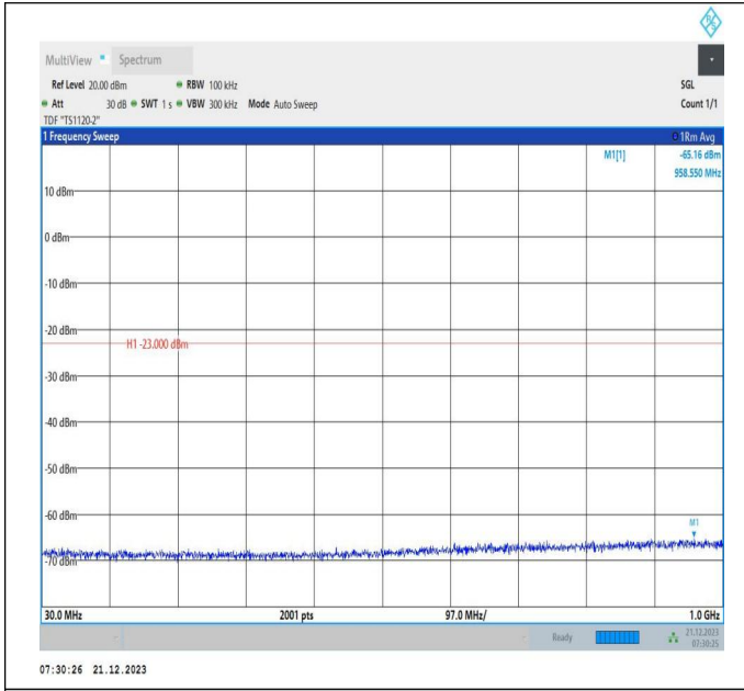
66-66-10MHz-15MHz-64QAM-64QAM-132477-132597-1RB# 0-ORB#0-30~1000MHz-PASS
