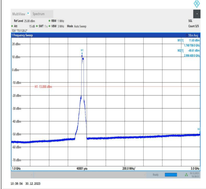
66-66-10MHz-15MHz-64QAM-64QAM-132351-132471-50RB #0-75RB#0-1000~3000MHz-PASS
