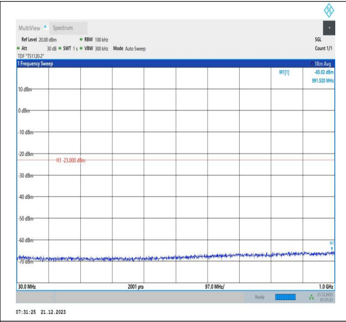
66-66-10MHz-15MHz-QPSK-QPSK-132477-132597-1RB#49 -ORB#0-30~1000MHz-PASS
