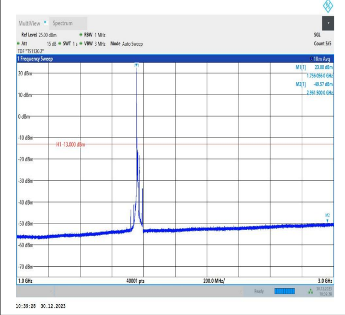
66-66-10MHz-15MHz-QPSK-QPSK-132477-132597-1RB#0-ORB#0-1000~3000MHz-PASS
