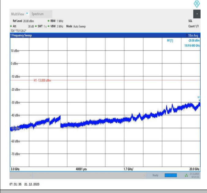
66-66-10MHz-15MHz-QPSK-QPSK-132477-132597-1RB#49 -ORB#0-3000~20000MHz-PASS
