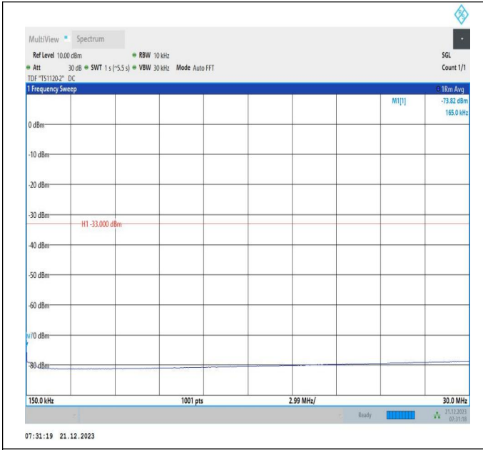
66-66-10MHz-15MHz-QPSK-QPSK-132477-132597-1RB#49 -ORB#0-0.15~30MHz-PASS
