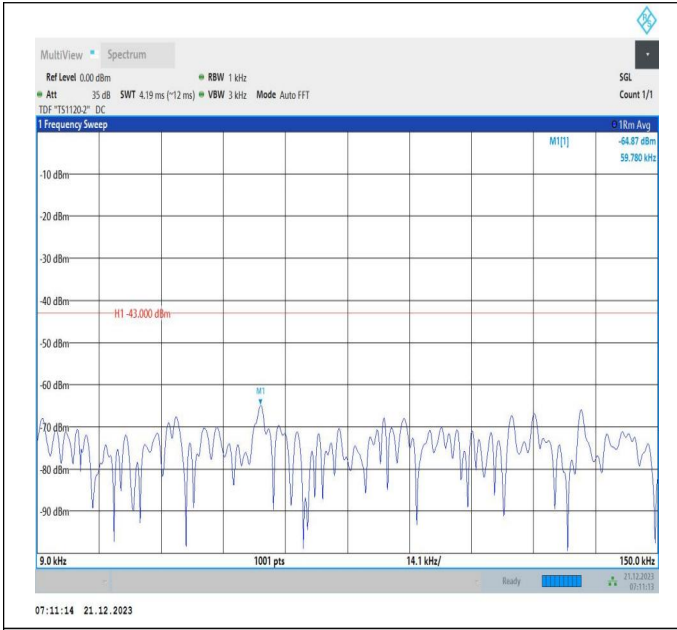
66-66-10MHz-15MHz-QPSK-QPSK-132477-132597-1RB#0-ORB#0-0.009~0.15MHz-PASS
