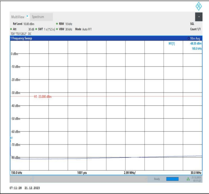
66-66-10MHz-15MHz-QPSK-QPSK-132477-132597-1RB#0-ORB#0-0.15~30MHz-PASS
