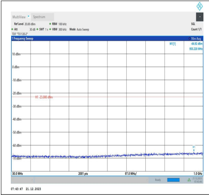
66-66-10MHz-15MHz-QPSK-QPSK-132477-132597-1RB#0-1RB#74-30~1000MHz-PASS
