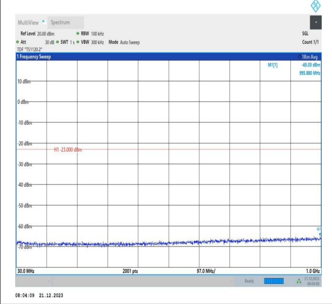
66-66-10MHz-15MHz-QPSK-QPSK-132477-132597-50RB#0 -75RB#0-30~1000MHz-PASS
