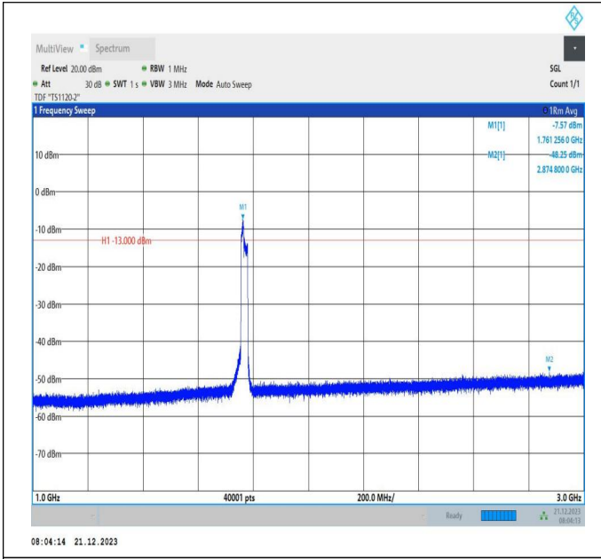
66-66-10MHz-15MHz-QPSK-QPSK-132477-132597-50RB#0 -75RB#0-1000~3000MHz-PASS
