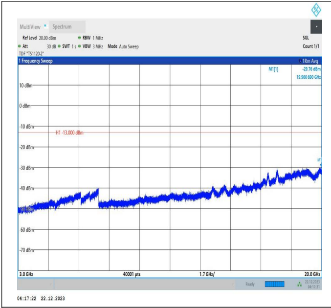
66-66-10MHz-20MHz-QPSK-QPSK-132027-132171-1RB#0-ORB#0-3000~20000MHz-PASS
