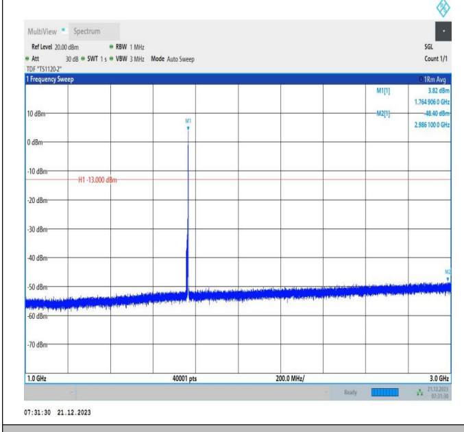
66-66-10MHz-15MHz-QPSK-QPSK-132477-132597-1RB#49 -ORB#0-1000~3000MHz-PASS
