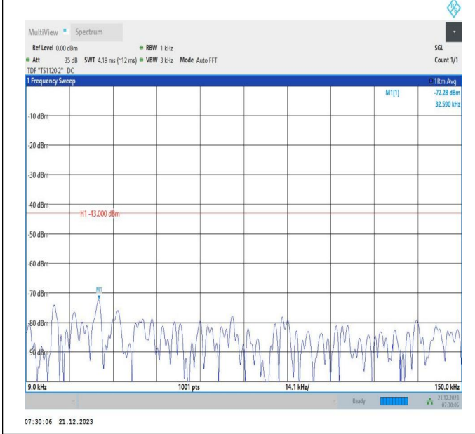
66-66-10MHz-15MHz-64QAM-64QAM-132477-132597-1RB# 0-ORB#0-0.009~0.15MHz-PASS
