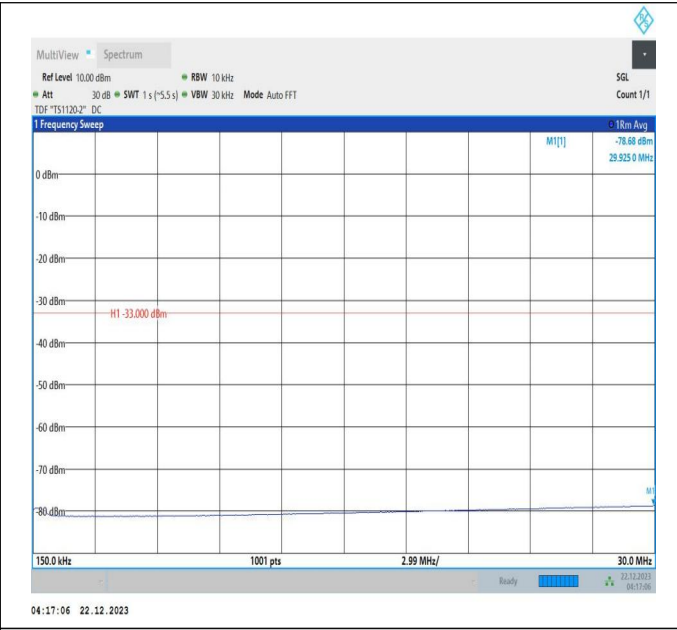
66-66-10MHz-20MHz-QPSK-QPSK-132027-132171-1RB#0-ORB#0-0.15~30MHz-PASS
