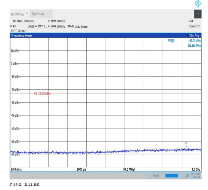
66-66-10MHz-15MHz-QPSK-QPSK-132351-132471-50RB#0-75RB#0-30~1000MHz-PASS
