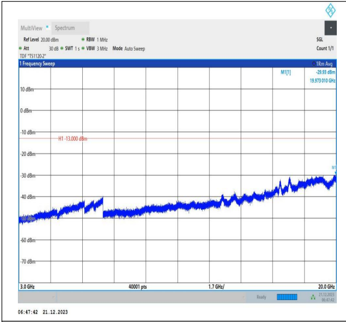
66-66-10MHz-15MHz-QPSK-QPSK-132351-132471-1RB#-0RB#0-3000~20000MHz-PASS
