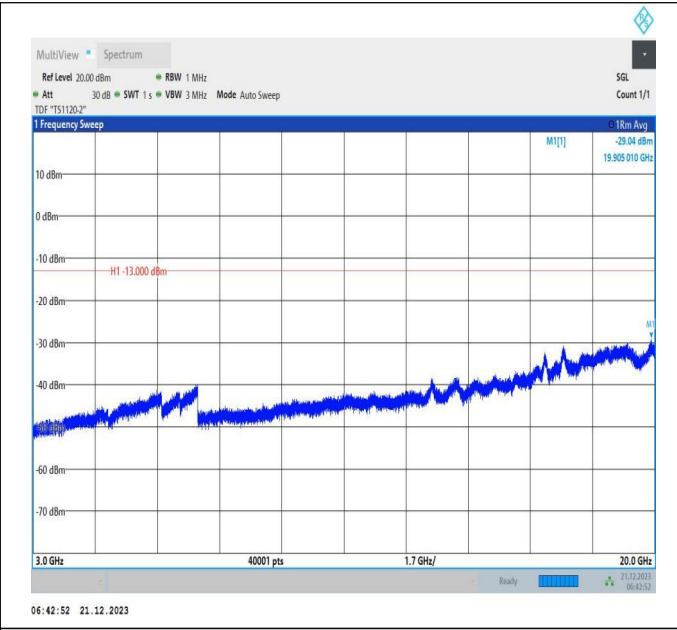
66-66-10MHz-15MHz-QPSK-QPSK-132025-132145-50RB#0 -75RB#0-3000~20000MHz-PASS
