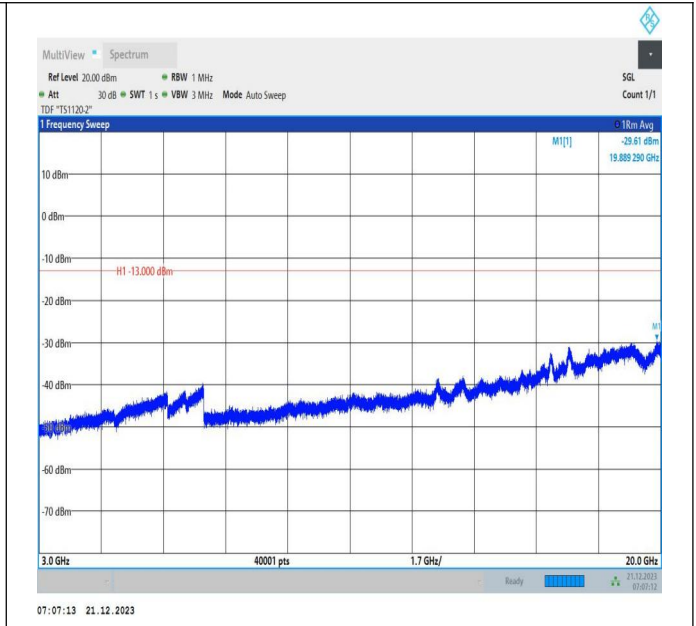
66-66-10MHz-15MHz-QPSK-QPSK-132351-132471-50RB#0 -75RB#0-3000~20000MHz-PASS
