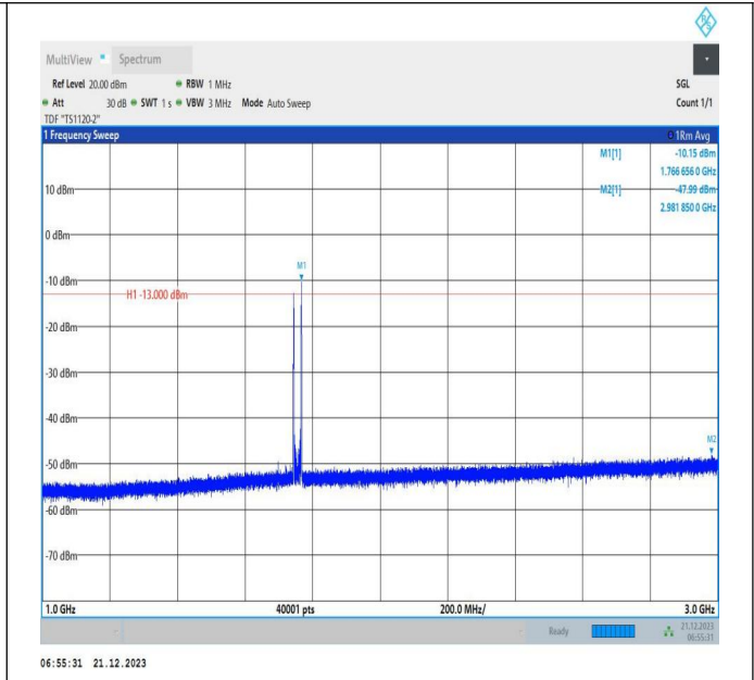
66-66-10MHz-15MHz-QPSK-QPSK-132351-132471-1RB#0-1RB#74-1000~3000MHz-PASS
