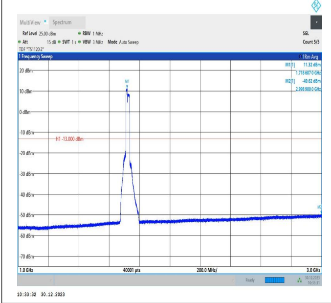
66-66-10MHz-15MHz-64QAM-64QAM-132025-132145-50RB #0-75RB#0-1000~3000MHz-PASS
