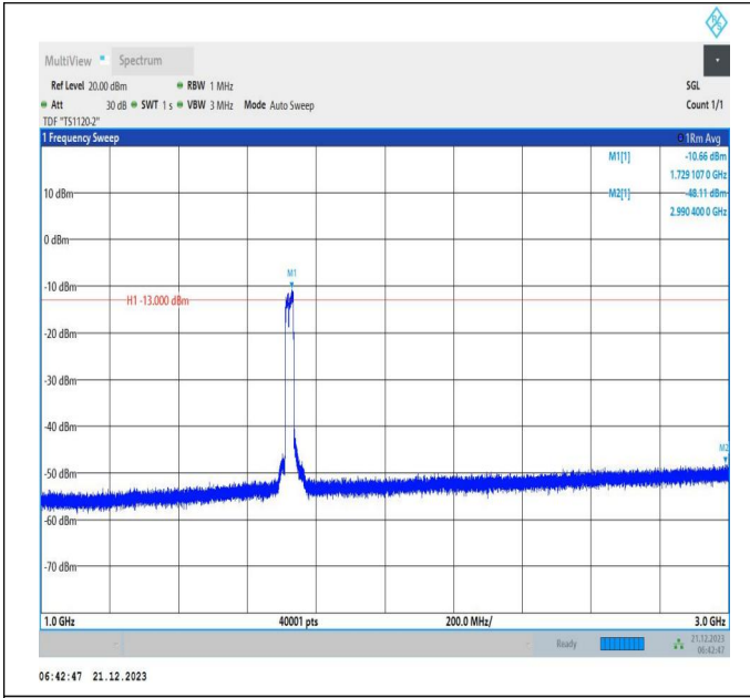
66-66-10MHz-15MHz-QPSK-QPSK-132025-132145-50RB#0 -75RB#0-1000~3000MHz-PASS
