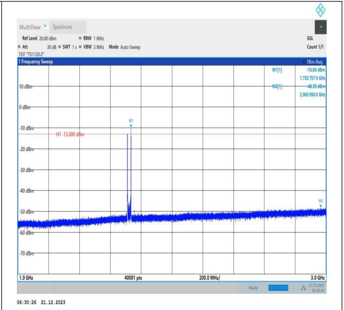
66-66-10MHz-15MHz-QPSK-QPSK-132025-132145-1RB#0-1RB#74-1000~3000MHz-PASS
