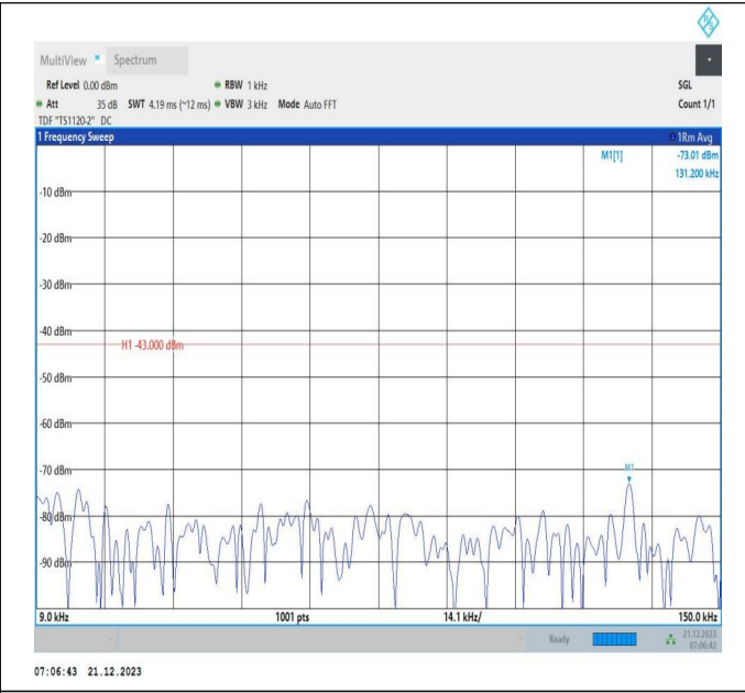
66-66-10MHz-15MHz-QPSK-QPSK-132351-132471-50RB#0-75RB#0-0.009~0.15MHz-PASS
