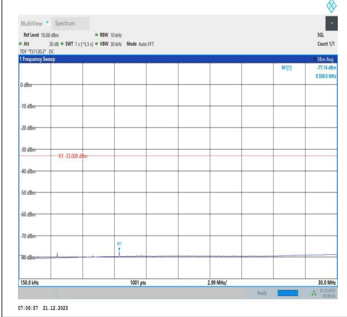
66-66-10MHz-15MHz-QPSK-QPSK-132351-132471-50RB#0-75RB#0-0.15~30MHz-PASS
