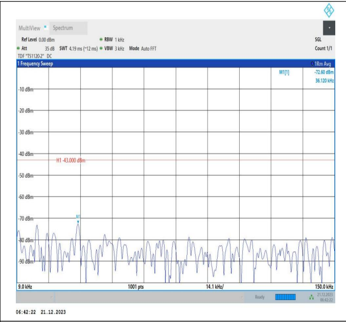
66-66-10MHz-15MHz-QPSK-QPSK-132025-132145-50RB#0-75RB#0-0.009~0.15MHz-PASS
