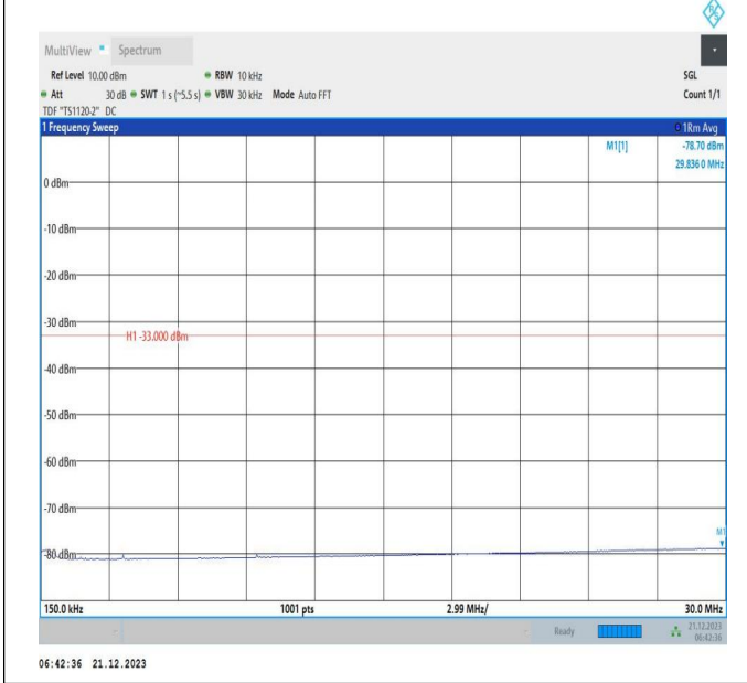
66-66-10MHz-15MHz-QPSK-QPSK-132025-132145-50RB#0-75RB#0-0.15~30MHz-PASS
