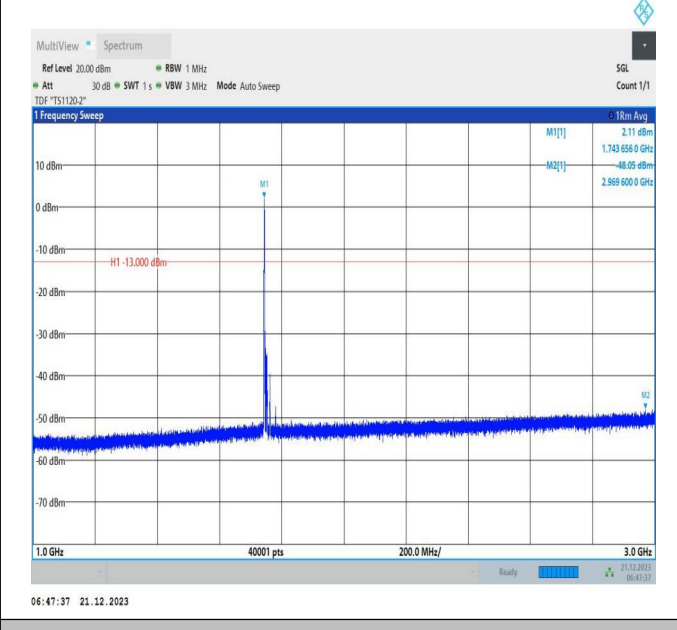
66-66-10MHz-15MHz-QPSK-QPSK-132351-132471-1RB#0-ORB#0-1000~3000MHz-PASS
