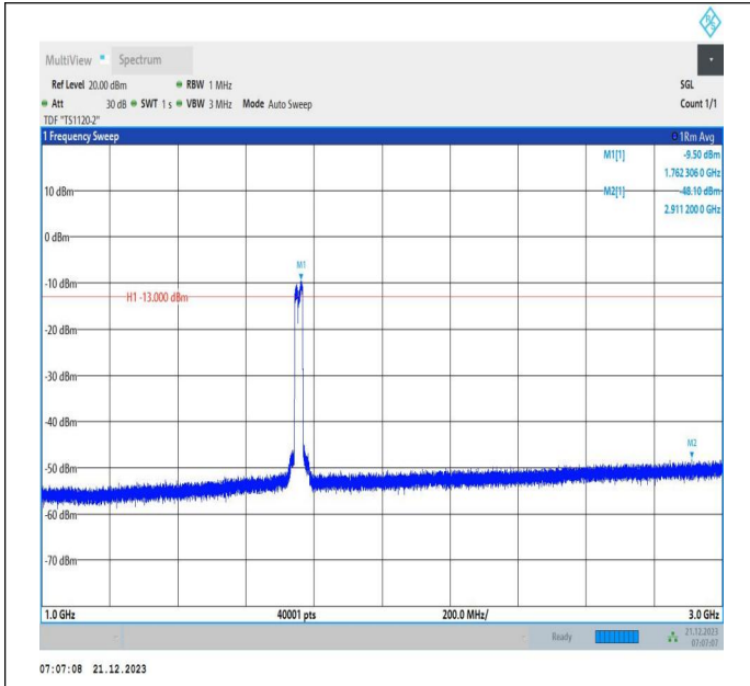
66-66-10MHz-15MHz-QPSK-QPSK-132351-132471-50RB#0 -75RB#0-1000~3000MHz-PASS
