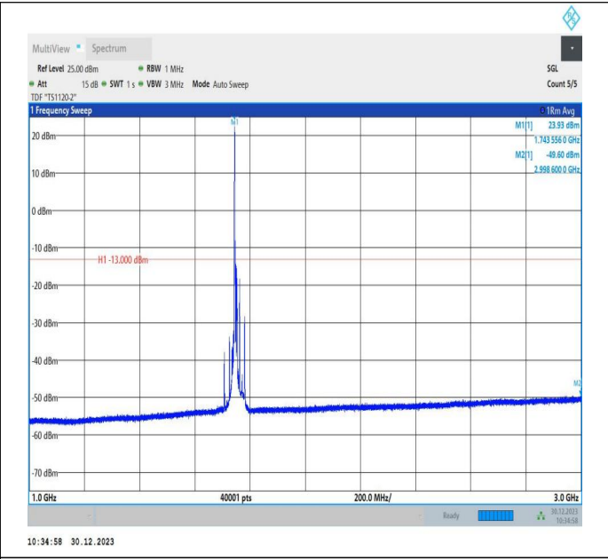
66-66-10MHz-15MHz-64QAM-64QAM-132351-132471-1RB# 0-ORB#0-1000~3000MHz-PASS
