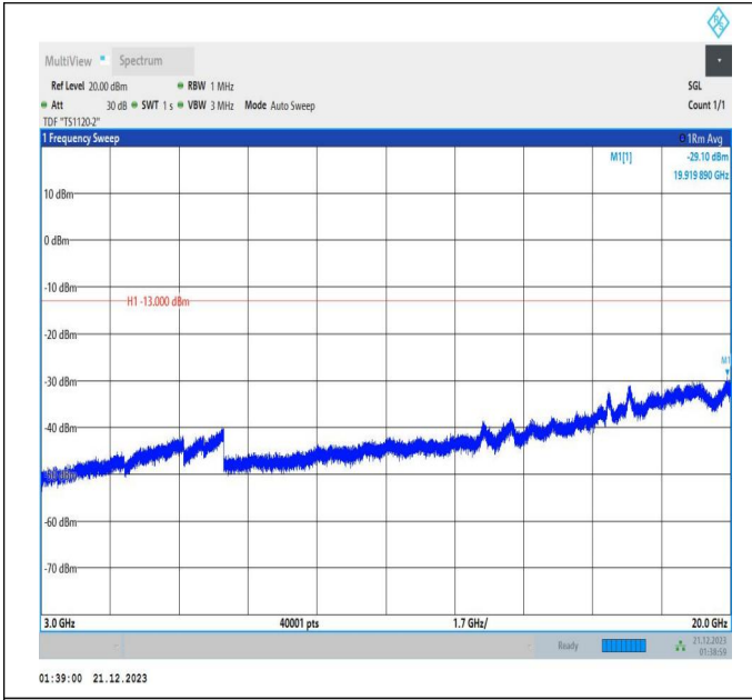
66-66-5MHz-20MHz-QPSK-QPSK-132328-132472-1RB#0-0 RB#0-3000~20000MHz-PASS
