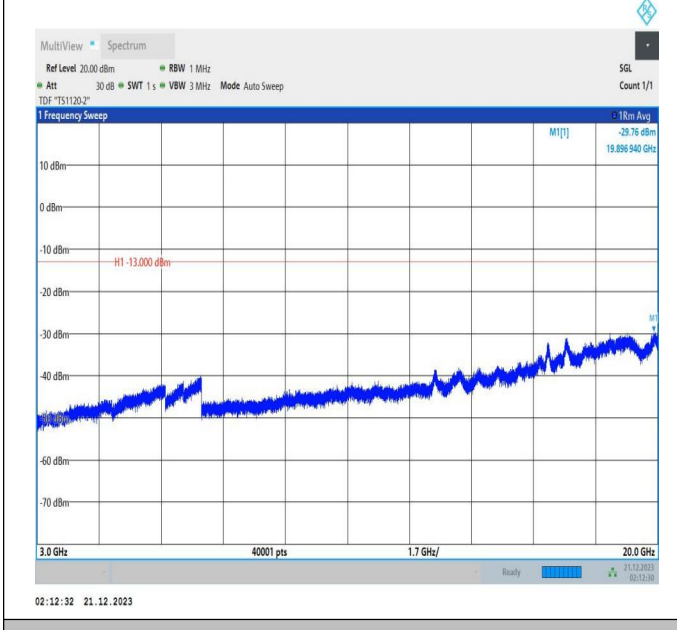
66-66-5MHz-20MHz-QPSK-QPSK-132328-132472-1RB#0-1 RB#99-3000~20000MHz-PASS
