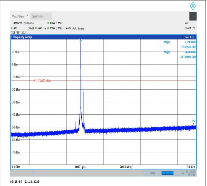
66-66-5MHz-20MHz-QPSK-QPSK-132428-132572-1RB#0-0 RB#0-1000~3000MHz-PASS
