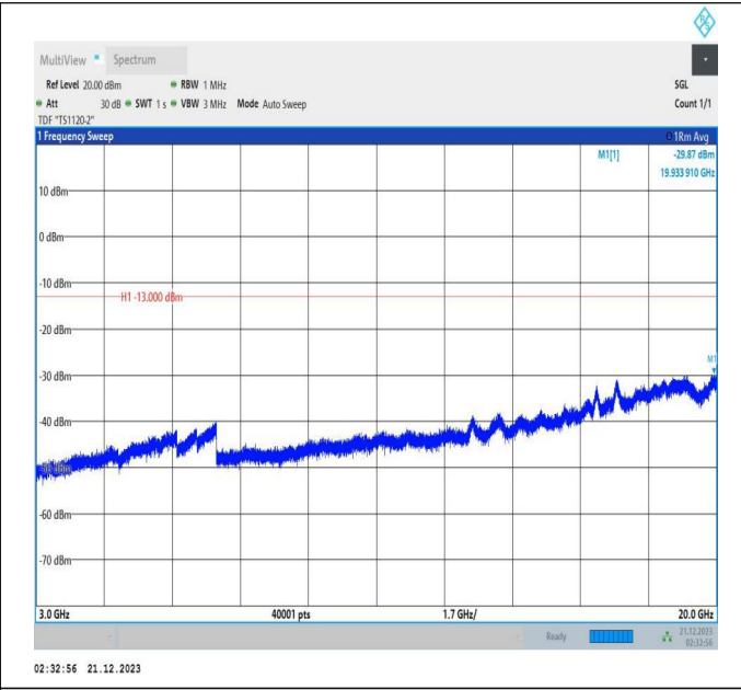
66-66-5MHz-20MHz-QPSK-QPSK-132328-132472-25RB#0-100RB#0-3000~20000MHz-PASS
