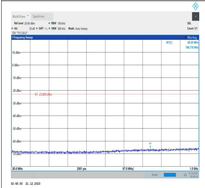
66-66-5MHz-20MHz-QPSK-QPSK-132428-132572-1RB#0-0 RB#0-30~1000MHz-PASS
