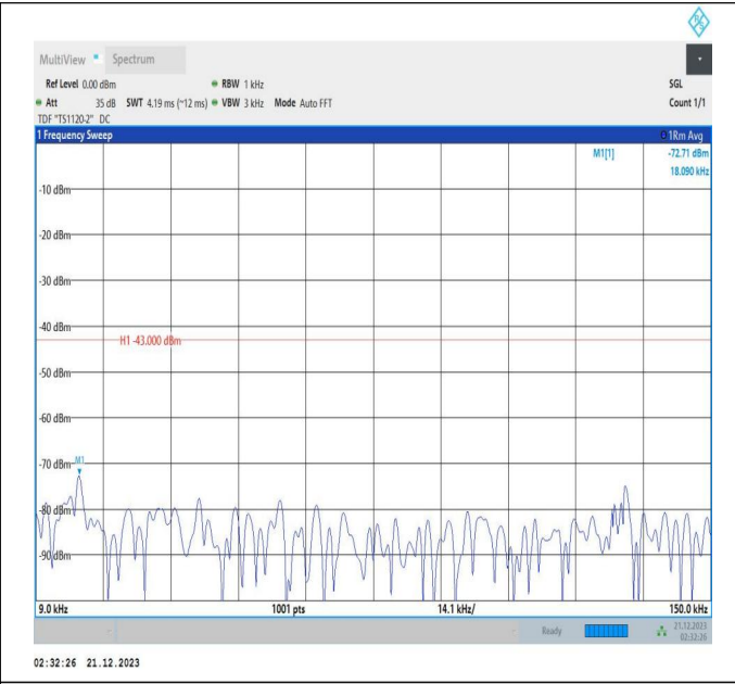
66-66-5MHz-20MHz-QPSK-QPSK-132328-132472-25RB#0-100RB#0-0.009~0.15MHz-PASS
