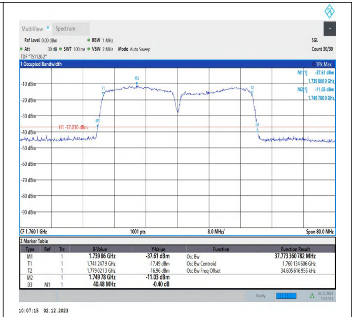
66-66-20MHz-20MHz-QPSK-QPSK-132374-132572-100RB# 0-100RB#0-PASS
