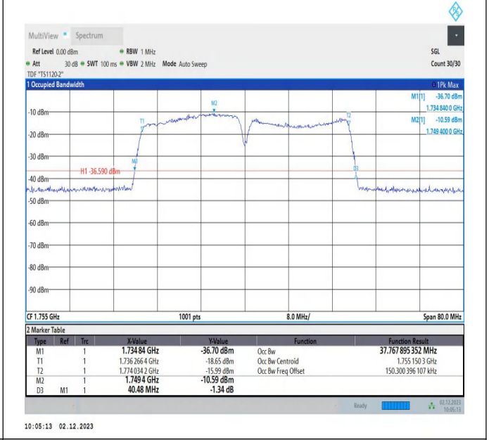
66-66-20MHz-20MHz-QPSK-QPSK-132323-132521-100RB# 0-100RB#0-PASS
