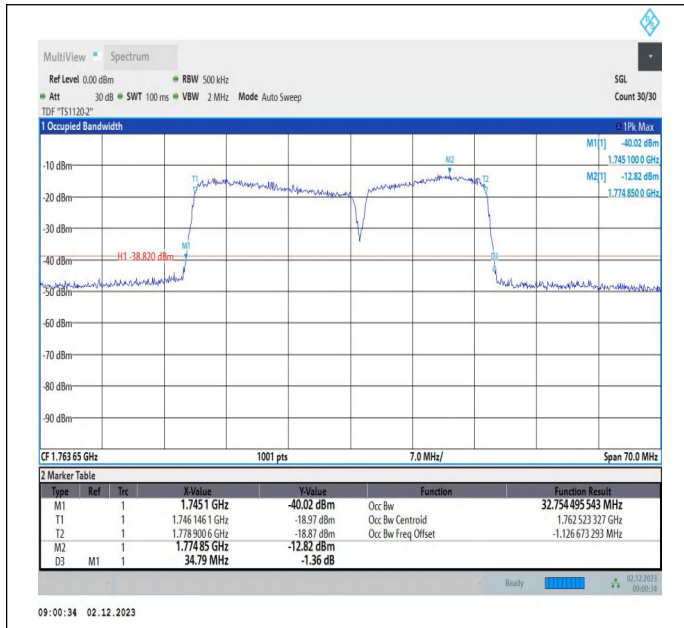
66-66-20MHz-15MHz-QPSK-QPSK-132423-132594-100RB#0-75RB#0-PASS
