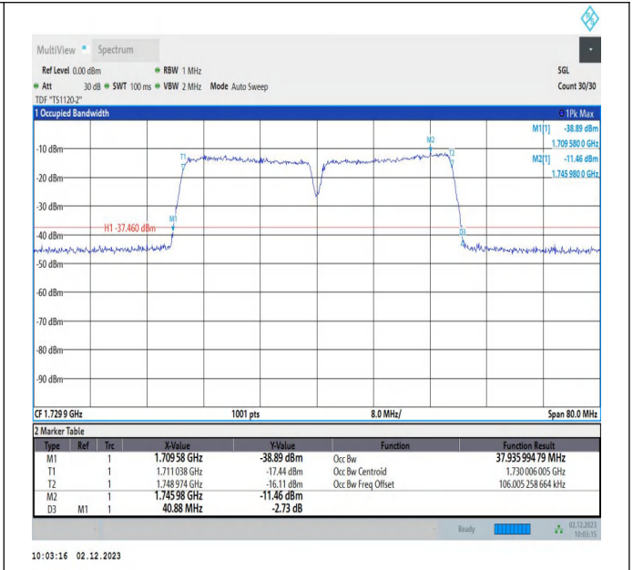
66-66-20MHz-20MHz-QPSK-QPSK-132072-132270-100RB# 0-100RB#0-PASS
