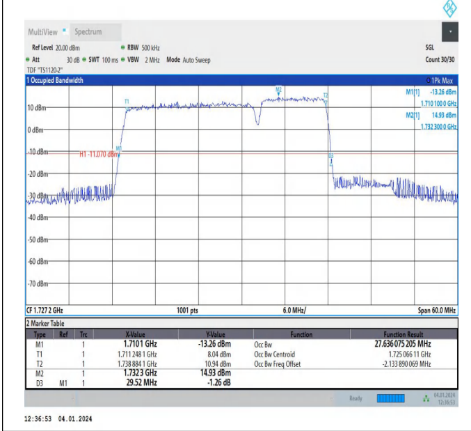
66-66-20MHz-10MHz-64QAM-64QAM-132072-132216-100R B#0-50RB#0-PASS
