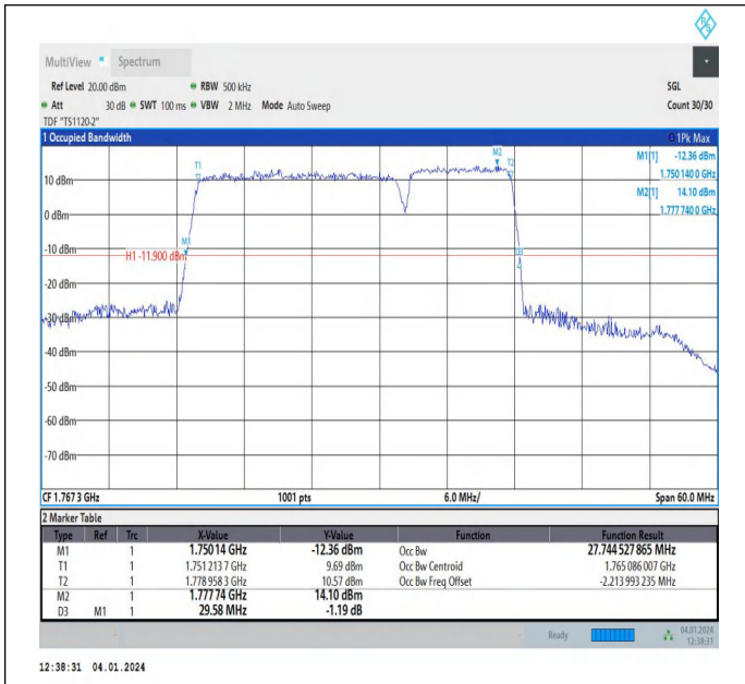
66-66-20MHz-10MHz-64QAM-64QAM-132473-132617-100R B#0-50RB#0-PASS
