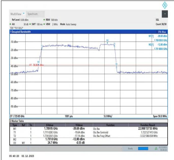
66-66-20MHz-5MHz-QPSK-QPSK-132072-132189-100RB#0-25RB#0-PASS
