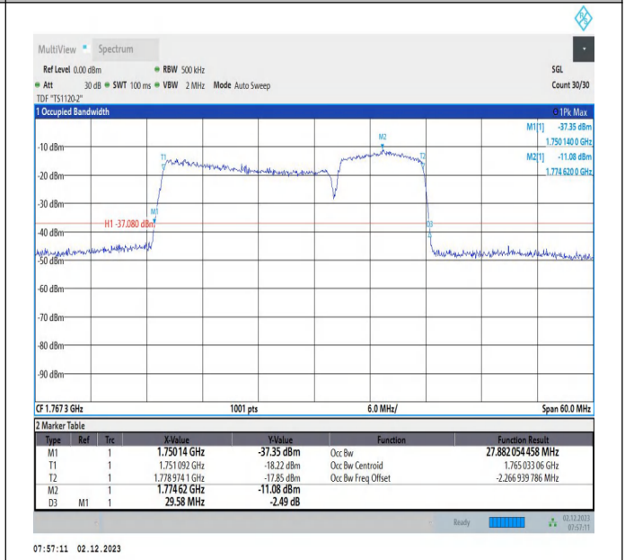
66-66-20MHz-10MHz-QPSK-QPSK-132473-132617-100RB# 0-50RB#0-PASS
