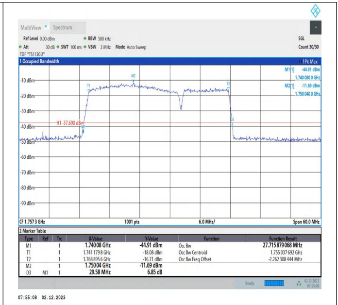
66-66-20MHz-10MHz-QPSK-QPSK-132373-132517-100RB# 0-50RB#0-PASS
