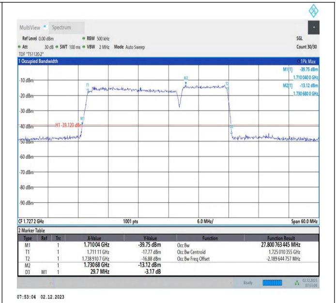
66-66-20MHz-10MHz-QPSK-QPSK-132072-132216-100RB# 0-50RB#0-PASS
