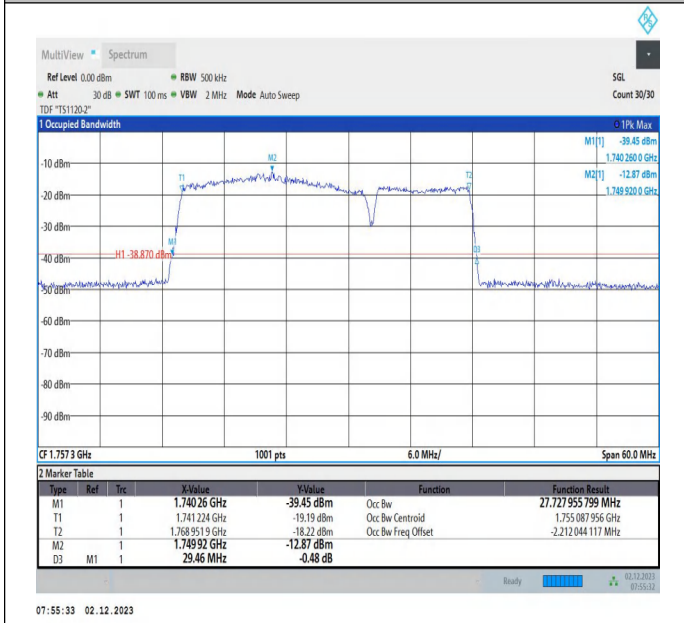
66-66-20MHz-10MHz-16QAM-16QAM-132373-132517-100RB#0-50RB#0-PASS
