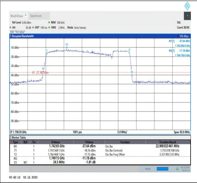
66-66-20MHz-5MHz-QPSK-QPSK-132397-132514-100RB#0-25RB#0-PASS
