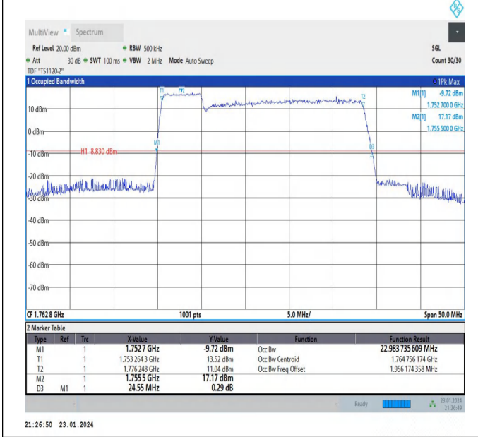
66-66-5MHz-20MHz-QPSK-QPSK-132428-132572-25RB#0- 100RB#0-PASS
