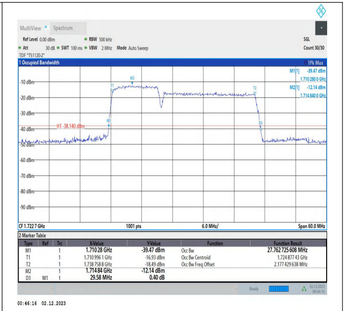
66-66-10MHz-20MHz-QPSK-QPSK-132027-132171-50RB#0-100RB#0-PASS
