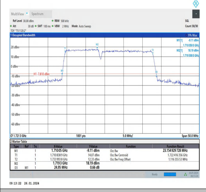
66-66-10MHz-15MHz-QPSK-QPSK-132025-132145-50RB#0-75RB#0-PASS
