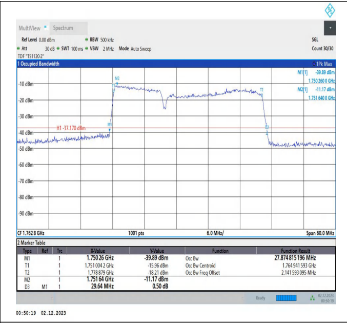
66-66-10MHz-20MHz-QPSK-QPSK-132428-132572-50RB#0-100RB#0-PASS
