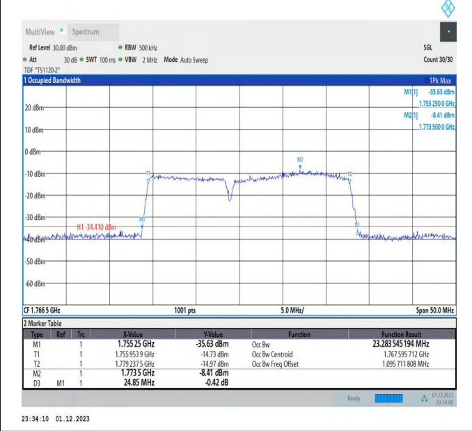
66-66-10MHz-15MHz-QPSK-QPSK-132477-132597-50RB#0-75RB#0-PASS
