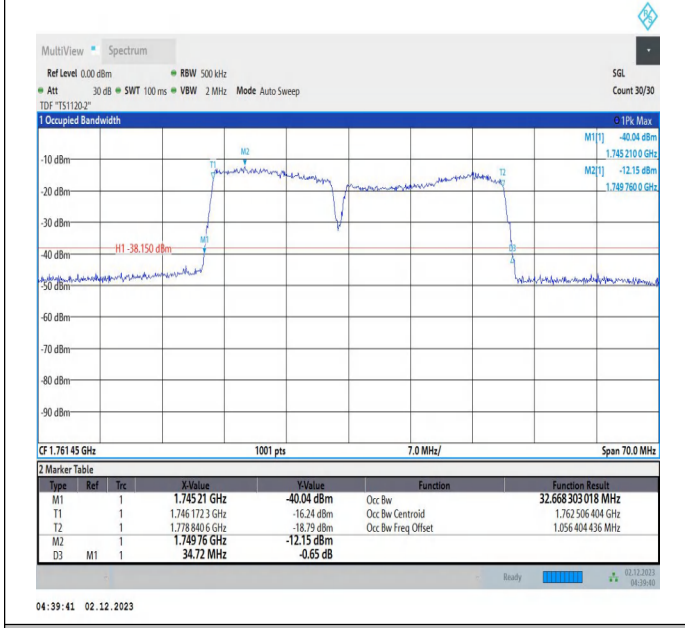
66-66-15MHz-20MHz-QPSK-QPSK-132401-132572-75RB#0 -100RB#0-PASS
