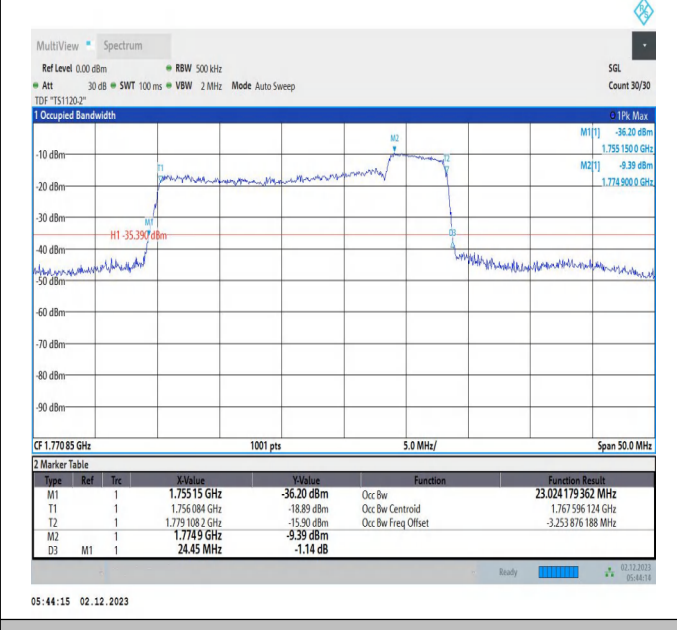
66-66-20MHz-5MHz-QPSK-QPSK-132522-132639-100RB#0-25RB#0-PASS
