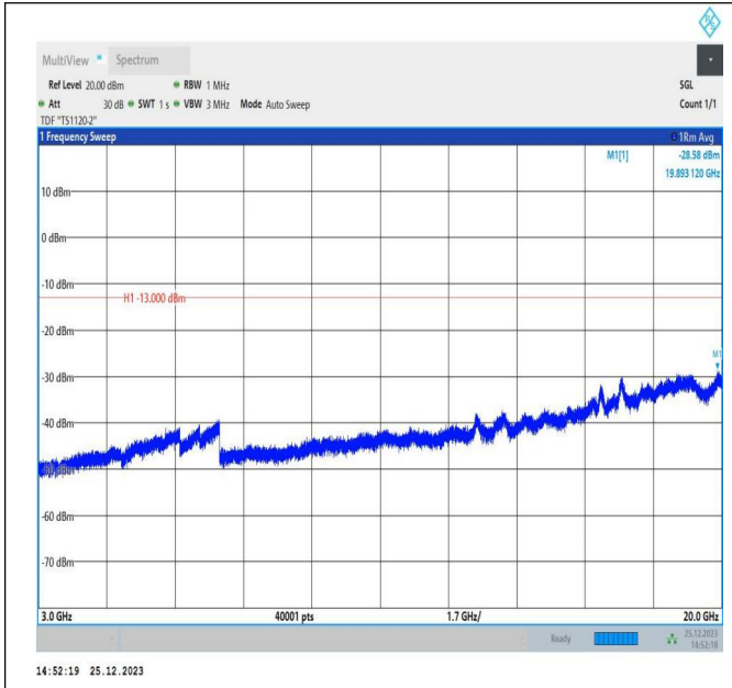
66-66-5MHz-15MHz-QPSK-QPSK-132504-132597-1RB#0-1 RB#74-3000~20000MHz-PASS
