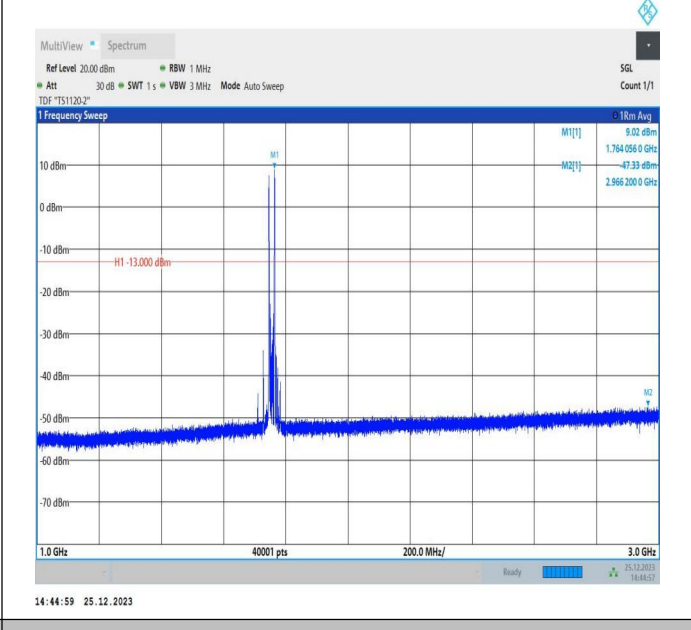
66-66-5MHz-15MHz-QPSK-QPSK-132353-132446-1RB#0-1R B#74-1000~3000MHz-PASS
