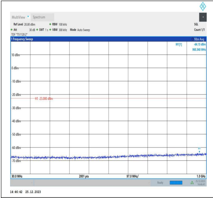
66-66-5MHz-15MHz-QPSK-QPSK-132353-132446-25RB#0-75RB#0-30~1000MHz-PASS
