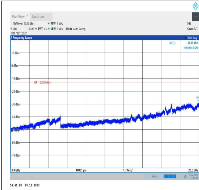
66-66-5MHz-15MHz-QPSK-QPSK-132353-132446-1RB#0-0RB#0-3000~20000MHz-PASS
