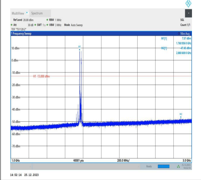
66-66-5MHz-15MHz-QPSK-QPSK-132504-132597-1RB#0-1R B#74-1000~3000MHz-PASS
