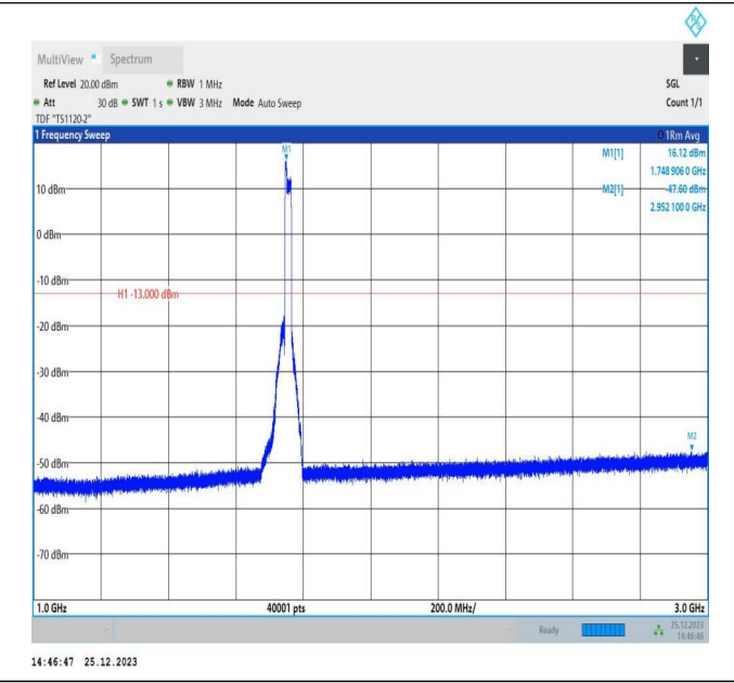
66-66-5MHz-15MHz-QPSK-QPSK-132353-132446-25RB#0-75RB#0-1000~3000MHz-PASS
