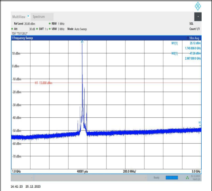
66-66-5MHz-15MHz-QPSK-QPSK-132353-132446-1RB#0-0R B#0-1000~3000MHz-PASS
