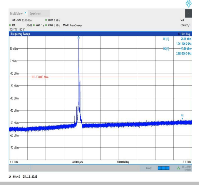
66-66-5MHz-15MHz-QPSK-QPSK-132504-132597-1RB#0-0R B#0-1000~3000MHz-PASS
