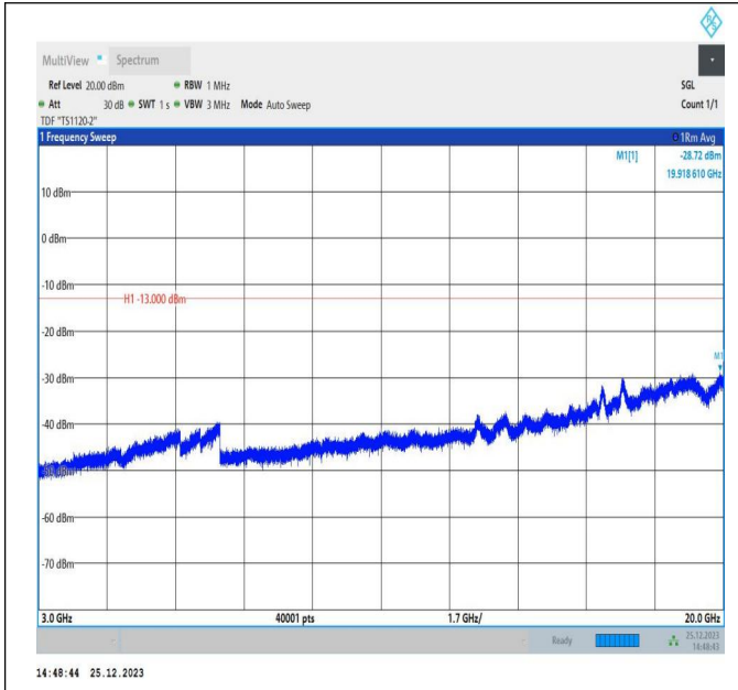
66-66-5MHz-15MHz-QPSK-QPSK-132504-132597-1RB#0-0RB#0-3000~20000MHz-PASS
