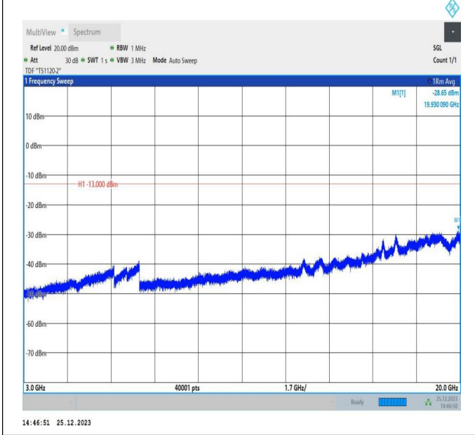
66-66-5MHz-15MHz-QPSK-QPSK-132353-132446-25RB#0-75RB#0-3000~20000MHz-PASS
