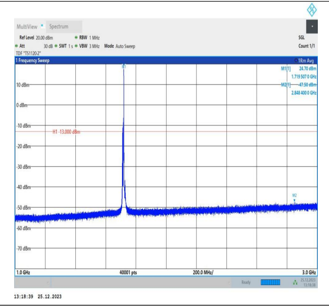
66-66-10MHz-10MHz-QPSK-QPSK-132022-132121-1RB#49- ORB#0-1000~3000MHz-PASS
