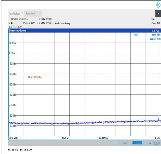
66-66-10MHz-5MHz-QPSK-QPSK-132572-132644-50RB#0-25RB#0-30~1000MHz-PASS
