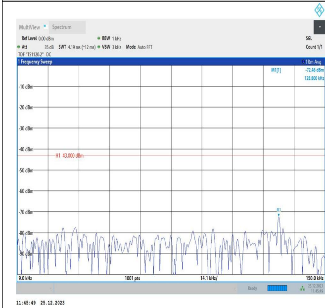
66-66-10MHz-5MHz-QPSK-QPSK-132022-132094-50RB#0-25RB#0-0.009~0.15MHz-PASS
