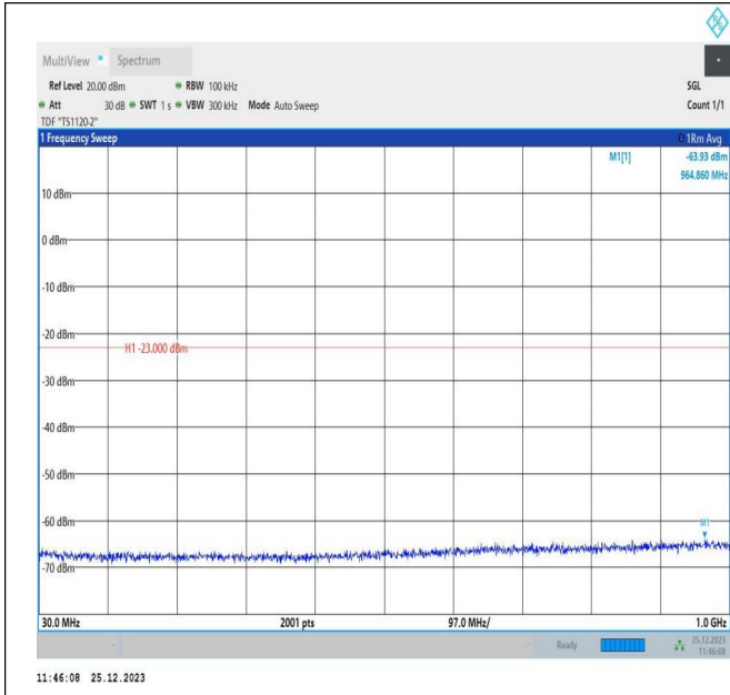
66-66-10MHz-5MHz-QPSK-QPSK-132022-132094-50RB#0-25RB#0-30~1000MHz-PASS
