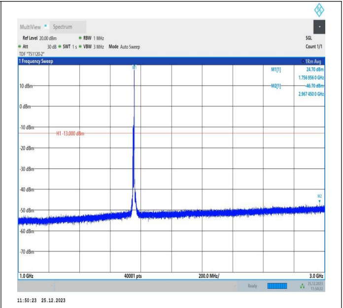
66-66-10MHz-5MHz-QPSK-QPSK-132397-132469-1RB#49-ORB#0-1000~3000MHz-PASS
