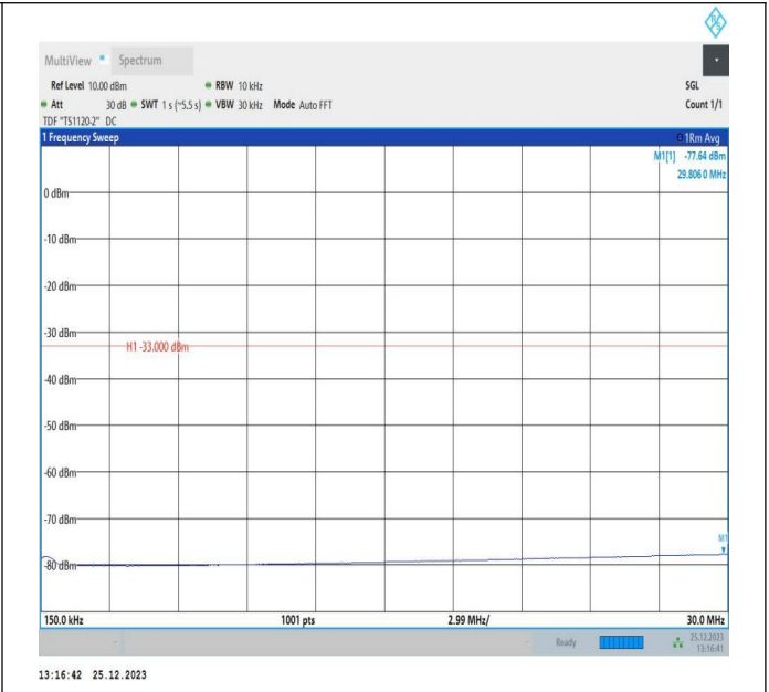
66-66-10MHz-10MHz-QPSK-QPSK-132022-132121-1RB#0-0RB#0-0.15~30MHz-PASS
