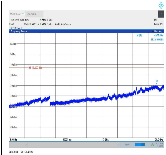
66-66-10MHz-5MHz-QPSK-QPSK-132572-132644-1RB#0-1 RB#24-3000~20000MHz-PASS
