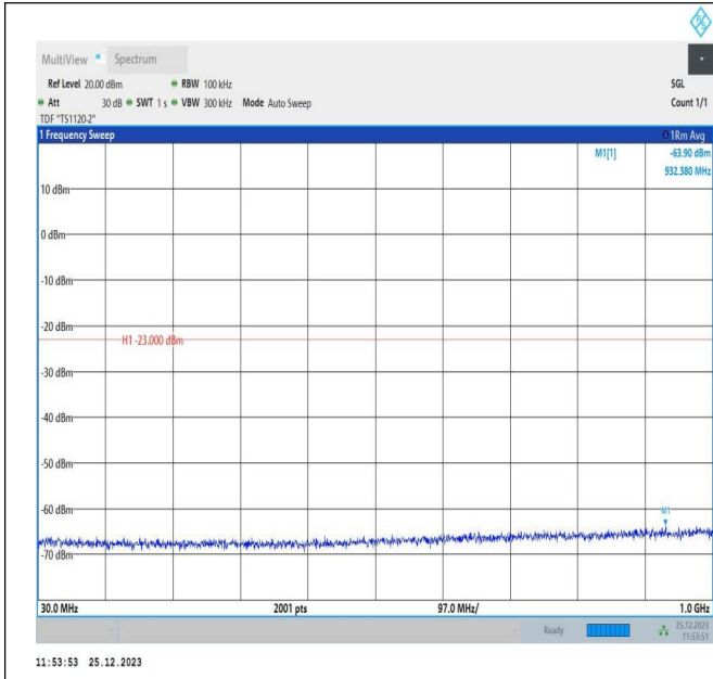
66-66-10MHz-5MHz-QPSK-QPSK-132397-132469-50RB#0-25RB#0-30~1000MHz-PASS
