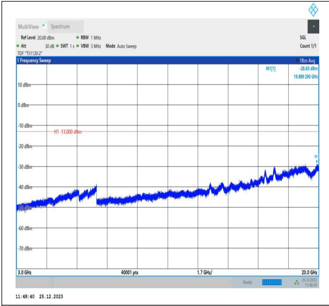
66-66-10MHz-5MHz-QPSK-QPSK-132397-132469-1RB#0-0RB#0-3000~20000MHz-PASS
