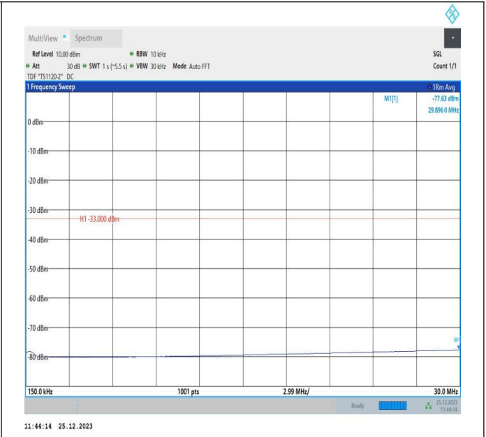
66-66-10MHz-5MHz-QPSK-QPSK-132022-132094-1RB#0-1R B#24-0.15~30MHz-PASS
