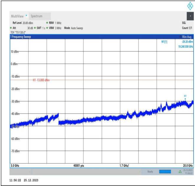
66-66-10MHz-5MHz-QPSK-QPSK-132572-132644-1RB#0-0 RB#0-3000~20000MHz-PASS
