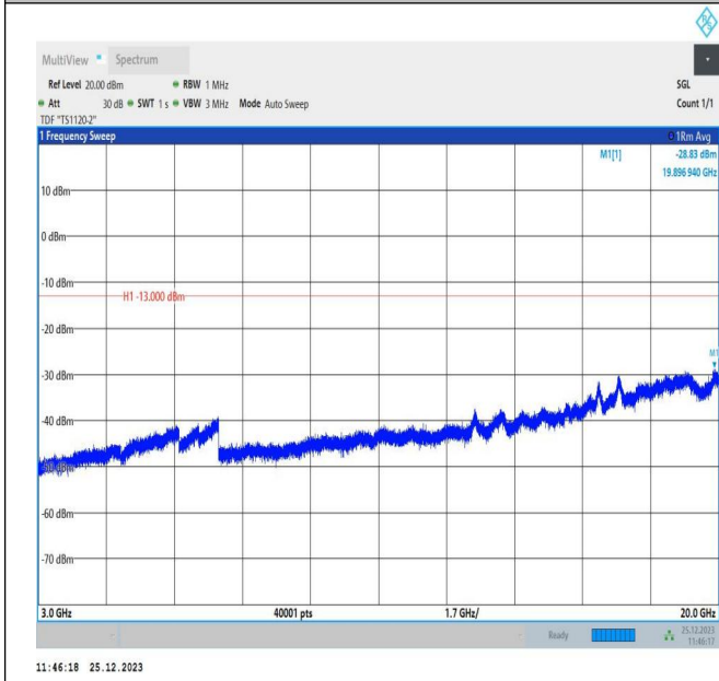
66-66-10MHz-5MHz-QPSK-QPSK-132022-132094-50RB#0-25RB#0-3000~20000MHz-PASS
