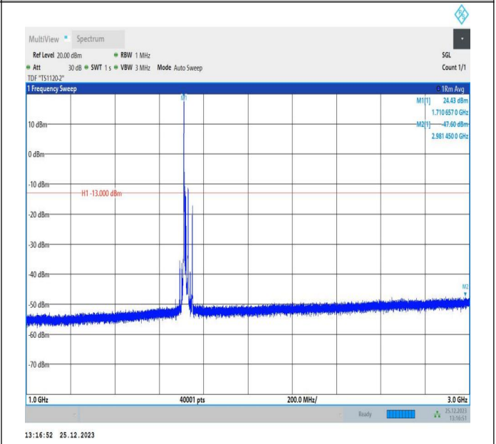
66-66-10MHz-10MHz-QPSK-QPSK-132022-132121-1RB#0-0RB#0-1000~3000MHz-PASS
