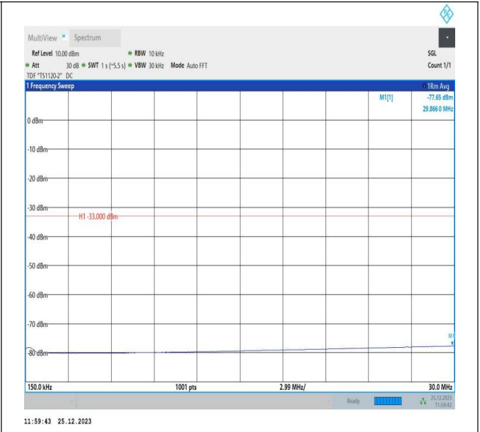
66-66-10MHz-5MHz-QPSK-QPSK-132572-132644-1RB#0-1R B#24-0.15~30MHz-PASS
