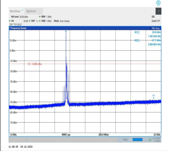
66-66-10MHz-5MHz-QPSK-QPSK-132397-132469-1RB#0-0R B#0-1000~3000MHz-PASS
