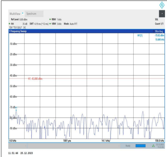
66-66-10MHz-5MHz-QPSK-QPSK-132397-132469-1RB#0-1 RB#24-0.009~0.15MHz-PASS
