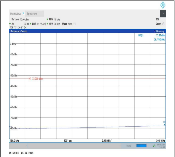
66-66-10MHz-5MHz-QPSK-QPSK-132397-132469-1RB#0-1R B#24-0.15~30MHz-PASS
