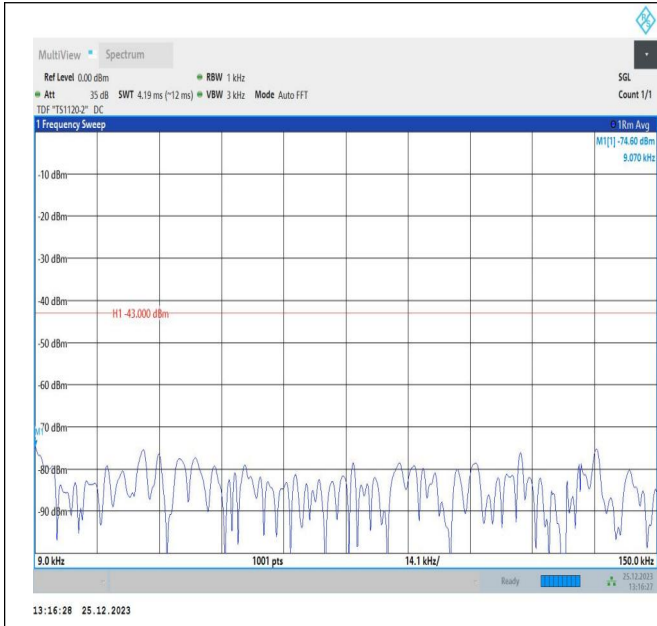
66-66-10MHz-10MHz-QPSK-QPSK-132022-132121-1RB#0-ORB#0-0.009~0.15MHz-PASS
