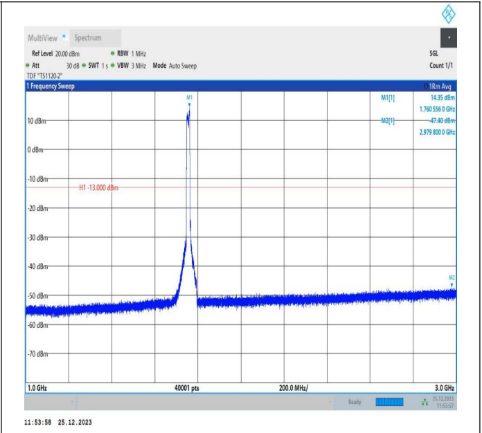
66-66-10MHz-5MHz-QPSK-QPSK-132397-132469-50RB#0-25RB#0-1000~3000MHz-PASS
