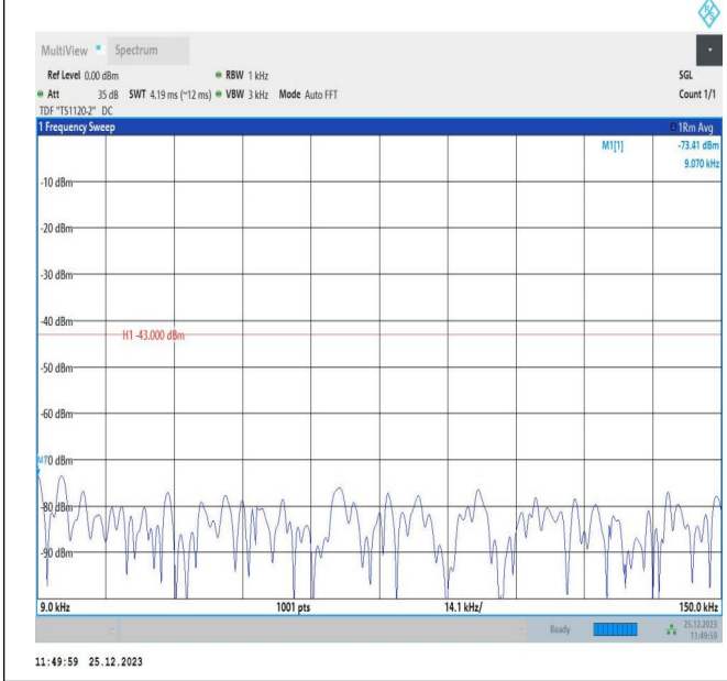
66-66-10MHz-5MHz-QPSK-QPSK-132397-132469-1RB#49-0RB#0-0.009~0.15MHz-PASS
