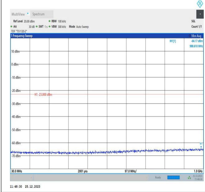
66-66-10MHz-5MHz-QPSK-QPSK-132397-132469-1RB#0-0 RB#0-30~1000MHz-PASS
