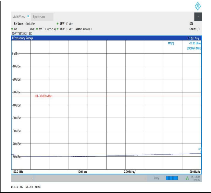
66-66-10MHz-5MHz-QPSK-QPSK-132397-132469-1RB#0-0R B#0-0.15~30MHz-PASS
