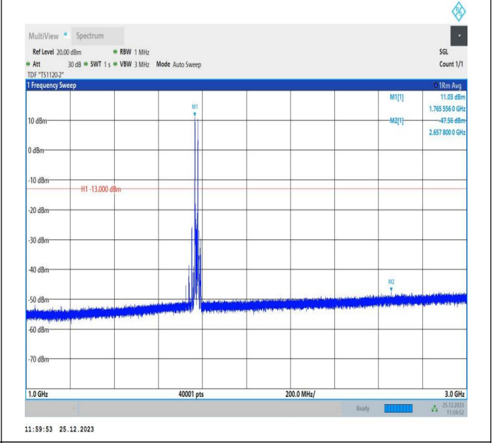
66-66-10MHz-5MHz-QPSK-QPSK-132572-132644-1RB#0-1R B#24-1000~3000MHz-PASS
