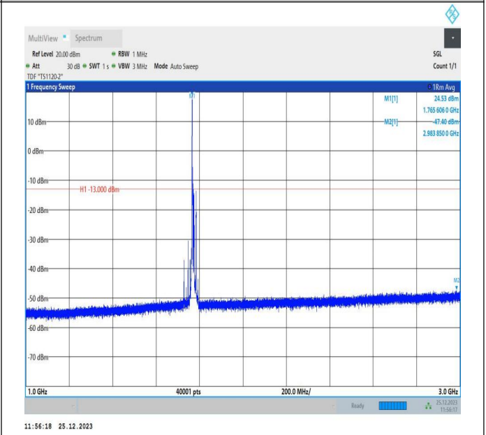
66-66-10MHz-5MHz-QPSK-QPSK-132572-132644-1RB#0-0R B#0-1000~3000MHz-PASS
