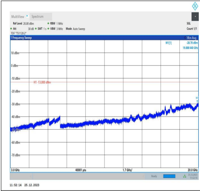
66-66-10MHz-5MHz-QPSK-QPSK-132397-132469-1RB#0-1 RB#24-3000~20000MHz-PASS
