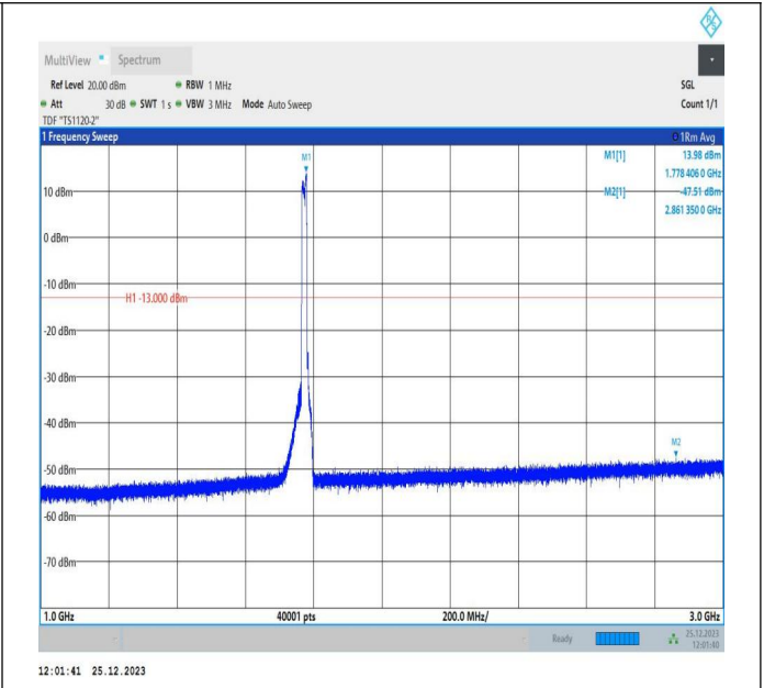
66-66-10MHz-5MHz-QPSK-QPSK-132572-132644-50RB#0-25RB#0-30~1000MHz-PASS 5RB#0-1000~3000MHz-PASS
