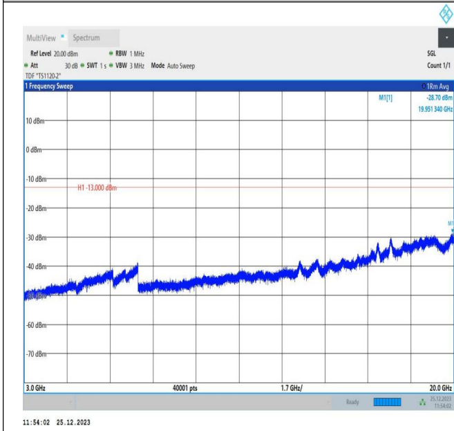
66-66-10MHz-5MHz-QPSK-QPSK-132397-132469-50RB#0-25RB#0-3000~20000MHz-PASS
