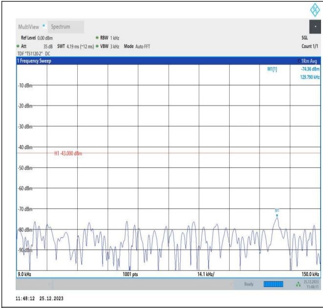
66-66-10MHz-5MHz-QPSK-QPSK-132397-132469-1RB#0-0 RB#0-0.009~0.15MHz-PASS
