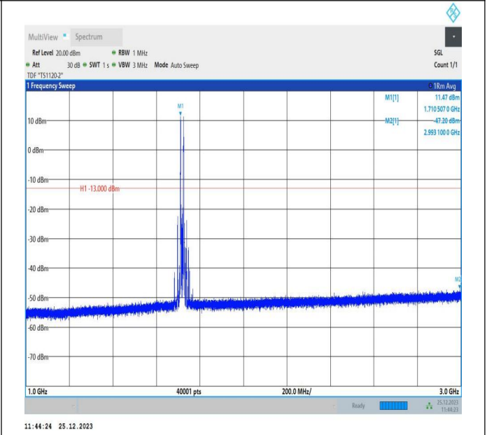
66-66-10MHz-5MHz-QPSK-QPSK-132022-132094-1RB#0-1R B#24-1000~3000MHz-PASS
