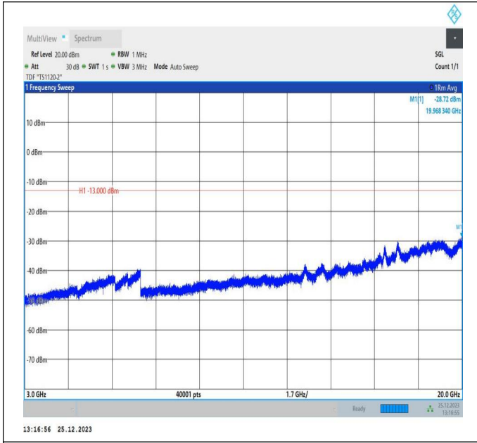
66-66-10MHz-10MHz-QPSK-QPSK-132022-132121-1RB#0-ORB#0-3000~20000MHz-PASS
