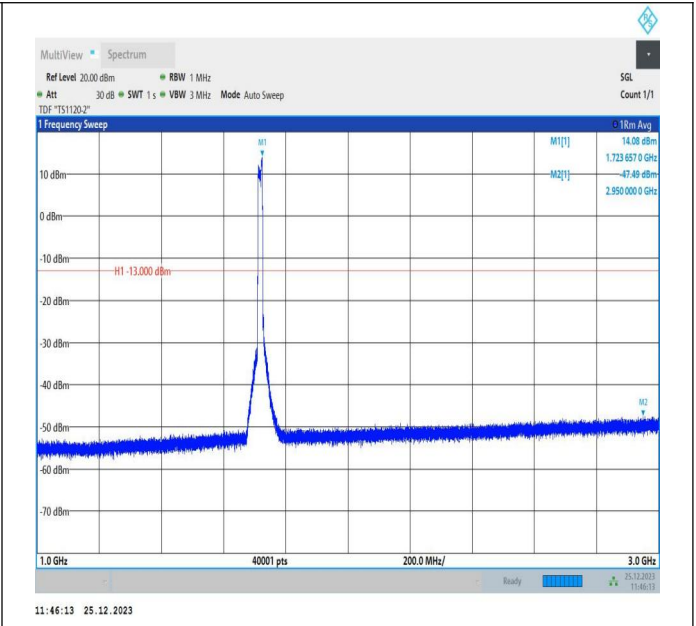
66-66-10MHz-5MHz-QPSK-QPSK-132022-132094-50RB#0-25RB#0-30~1000MHz-PASS 5RB#0-1000~3000MHz-PASS
