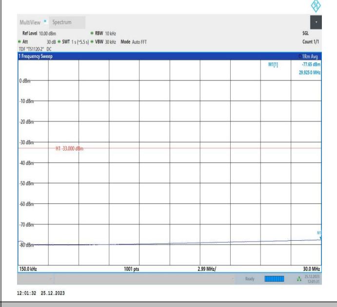
66-66-10MHz-5MHz-QPSK-QPSK-132572-132644-50RB#0-25RB#0-0.15~30MHz-PASS
