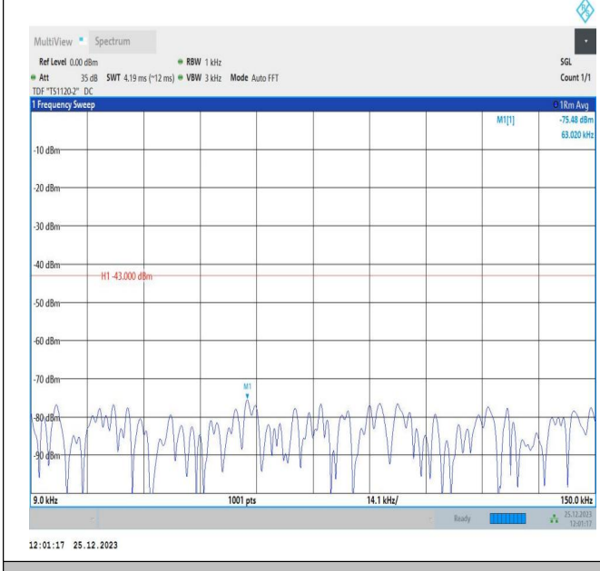
66-66-10MHz-5MHz-QPSK-QPSK-132572-132644-50RB#0-25RB#0-0.009~0.15MHz-PASS
