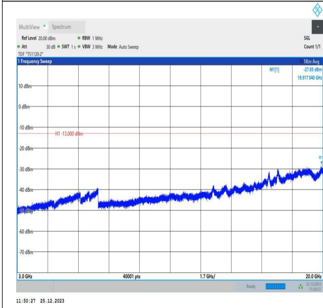
66-66-10MHz-5MHz-QPSK-QPSK-132397-132469-1RB#49-ORB#0-3000~20000MHz-PASS
