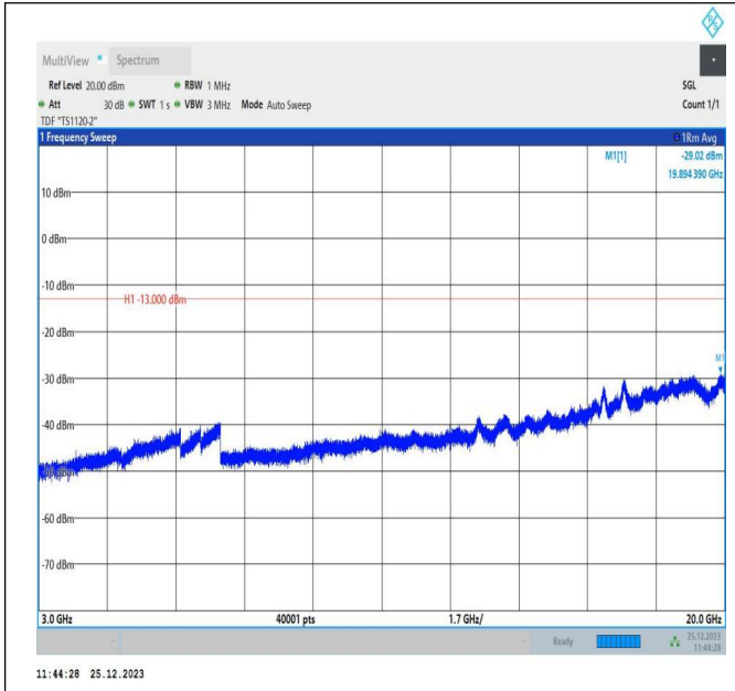
66-66-10MHz-5MHz-QPSK-QPSK-132022-132094-1RB#0-1 RB#24-3000~20000MHz-PASS
