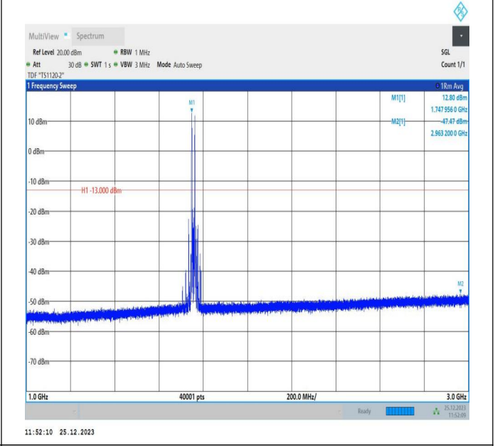
66-66-10MHz-5MHz-QPSK-QPSK-132397-132469-1RB#0-1R B#24-1000~3000MHz-PASS
