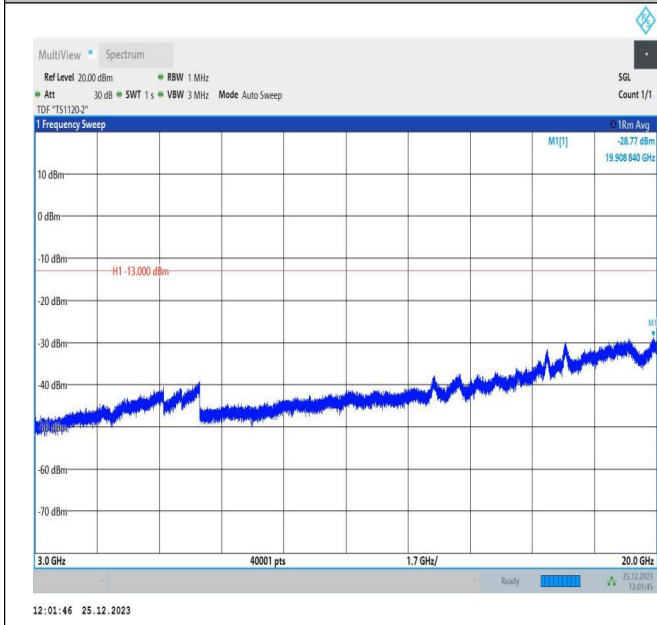
66-66-10MHz-5MHz-QPSK-QPSK-132572-132644-50RB#0-25RB#0-3000~20000MHz-PASS
