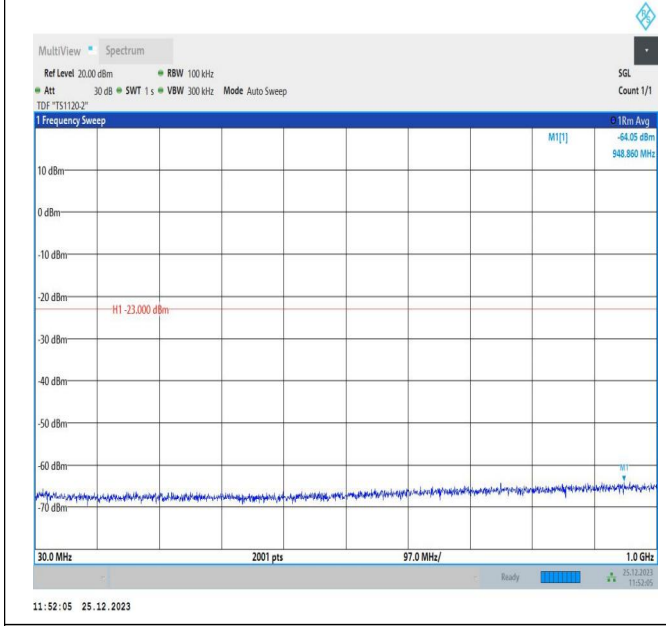
66-66-10MHz-5MHz-QPSK-QPSK-132397-132469-1RB#0-1 RB#24-30~1000MHz-PASS
