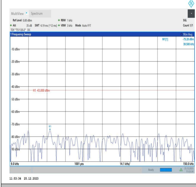
66-66-10MHz-5MHz-QPSK-QPSK-132397-132469-50RB#0-25RB#0-0.009~0.15MHz-PASS
