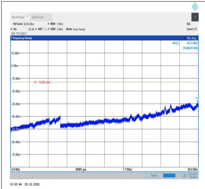
66-66-5MHz-10MHz-QPSK-QPSK-132375-132447-1RB#0-0RB#0-3000~20000MHz-PASS
