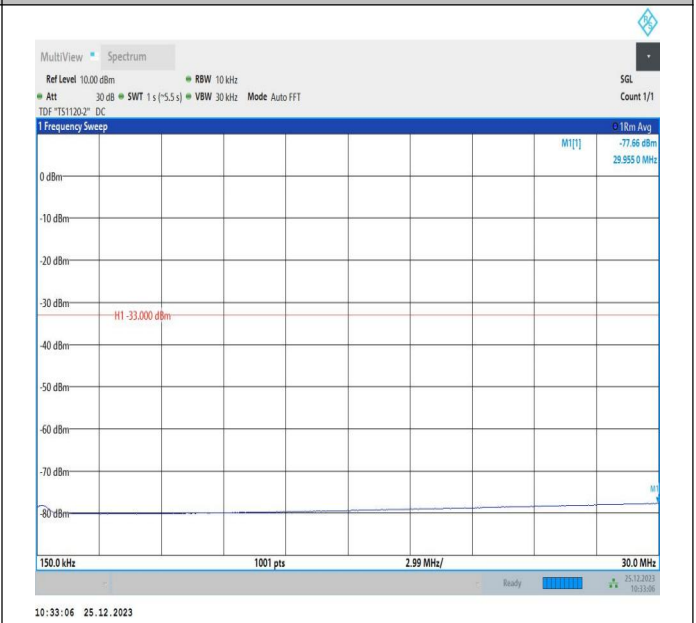
66-66-5MHz-10MHz-QPSK-QPSK-132550-132622-25RB#0-50RB#0-0.15~30MHz-PASS
