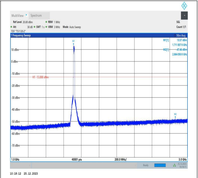
66-66-5MHz-10MHz-QPSK-QPSK-132000-132072-25RB#0-50RB#0-1000~3000MHz-PASS
