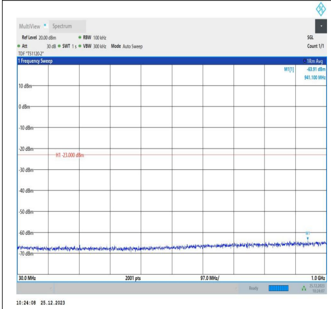
66-66-5MHz-10MHz-QPSK-QPSK-132375-132447-1RB#0-1 RB#49-30~1000MHz-PASS
