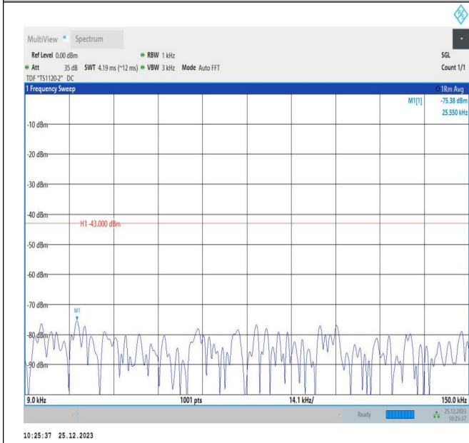
66-66-5MHz-10MHz-QPSK-QPSK-132375-132447-25RB#0-50RB#0-0.009~0.15MHz-PASS
