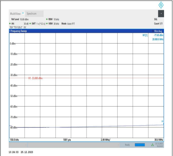
66-66-5MHz-10MHz-QPSK-QPSK-132375-132447-1RB#0-1R B#49-0.15~30MHz-PASS
