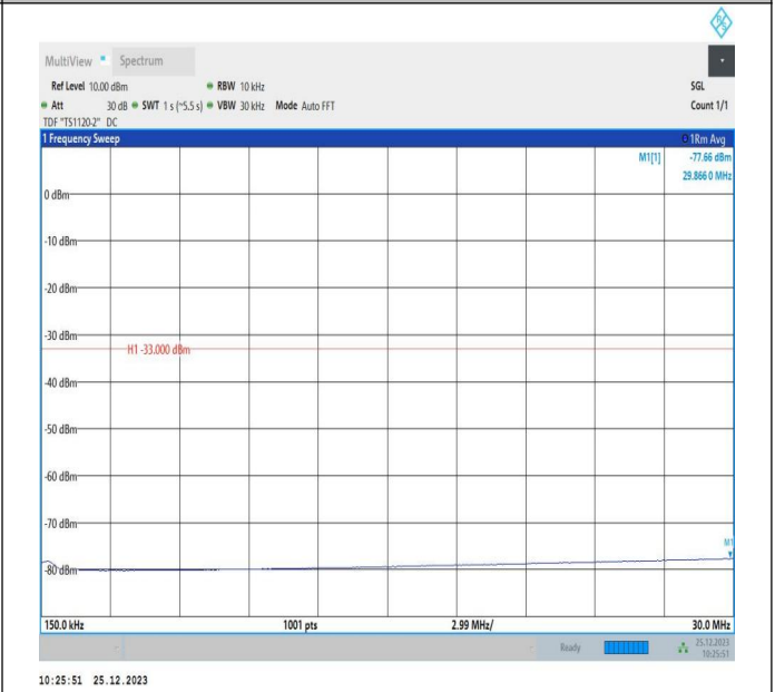
66-66-5MHz-10MHz-QPSK-QPSK-132375-132447-25RB#0-50RB#0-0.15~30MHz-PASS
