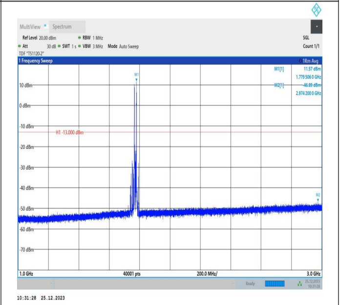
66-66-5MHz-10MHz-QPSK-QPSK-132550-132622-1RB#0-1R B#49-1000~3000MHz-PASS
