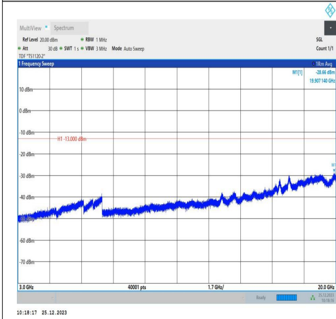
66-66-5MHz-10MHz-QPSK-QPSK-132000-132072-25RB#0-50RB#0-3000~20000MHz-PASS
