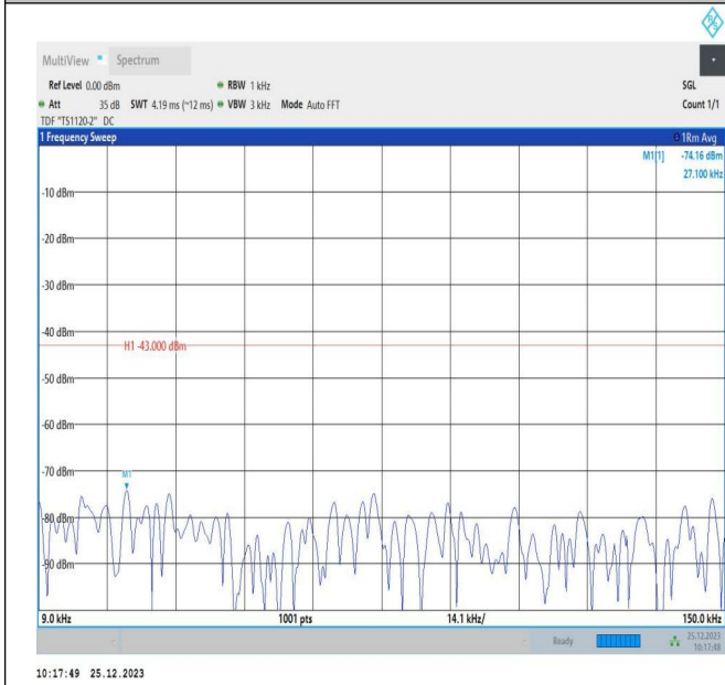
66-66-5MHz-10MHz-QPSK-QPSK-132000-132072-25RB#0-50RB#0-0.009~0.15MHz-PASS
