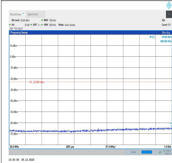
66-66-5MHz-10MHz-QPSK-QPSK-132375-132447-1RB#0-0 RB#0-30~1000MHz-PASS
