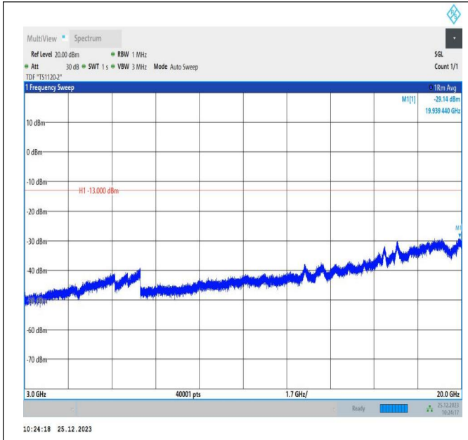
66-66-5MHz-10MHz-QPSK-QPSK-132375-132447-1RB#0-1 RB#49-3000~20000MHz-PASS
