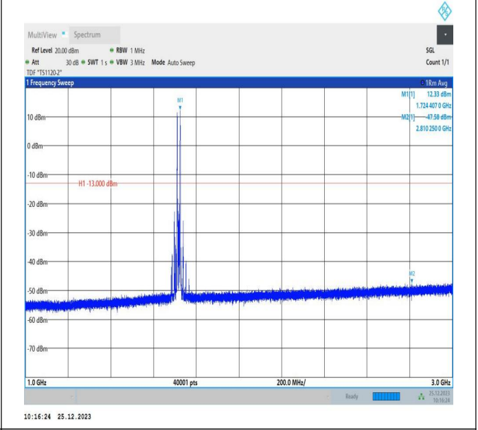
66-66-5MHz-10MHz-QPSK-QPSK-132000-132072-1RB#0-1R B#49-1000~3000MHz-PASS
