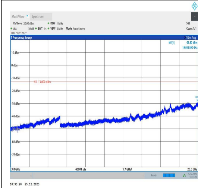
66-66-5MHz-10MHz-QPSK-QPSK-132550-132622-25RB#0-50RB#0-3000~20000MHz-PASS
