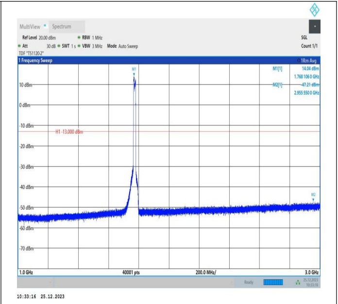
66-66-5MHz-10MHz-QPSK-QPSK-132550-132622-25RB#0-50RB#0-1000~3000MHz-PASS
