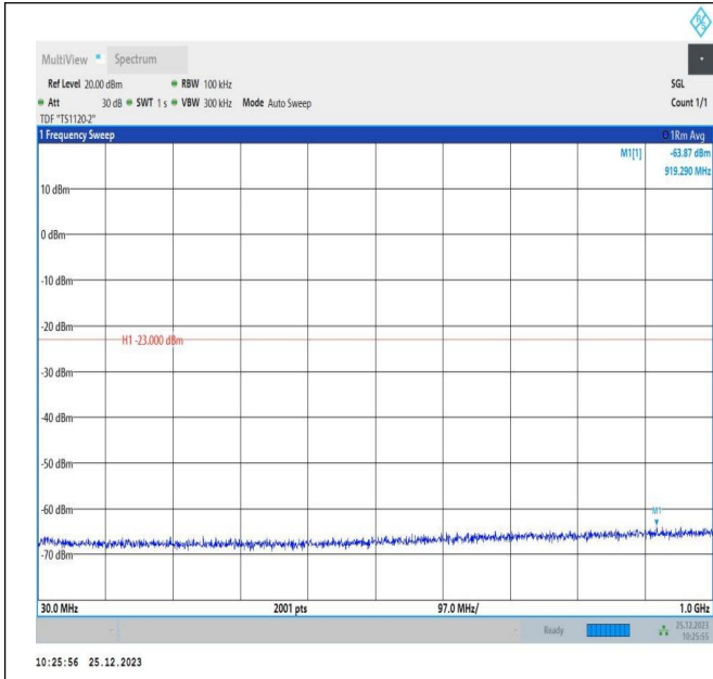
66-66-5MHz-10MHz-QPSK-QPSK-132375-132447-25RB#0-50RB#0-30~1000MHz-PASS
