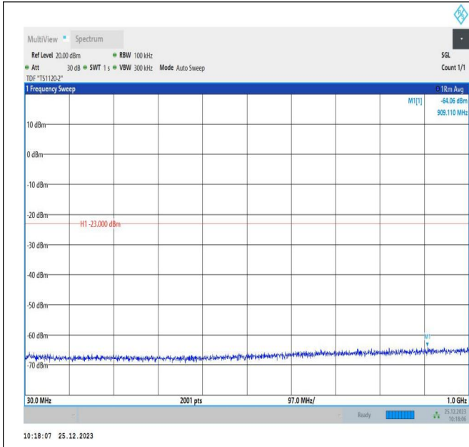
66-66-5MHz-10MHz-QPSK-QPSK-132000-132072-25RB#0-50RB#0-30~1000MHz-PASS
