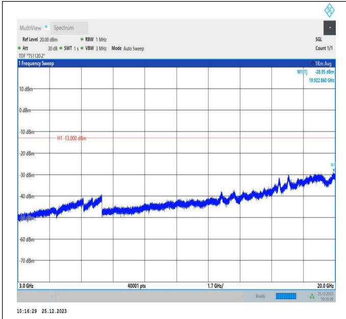
66-66-5MHz-10MHz-QPSK-QPSK-132000-132072-1RB#0-1 RB#49-3000~20000MHz-PASS
