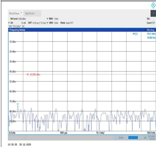
66-66-5MHz-10MHz-QPSK-QPSK-132550-132622-25RB#0-50RB#0-0.009~0.15MHz-PASS
