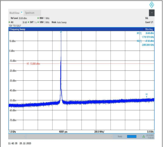
66-66-10MHz-5MHz-QPSK-QPSK-132022-132094-1RB#49-0RB#0-1000~3000MHz-PASS
