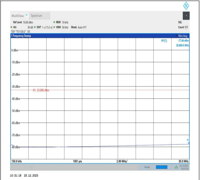
66-66-5MHz-10MHz-QPSK-QPSK-132550-132622-1RB#0-1R B#49-0.15~30MHz-PASS
