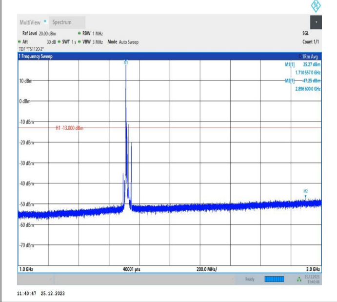
66-66-10MHz-5MHz-QPSK-QPSK-132022-132094-1RB#0-0R B#0-1000~3000MHz-PASS
