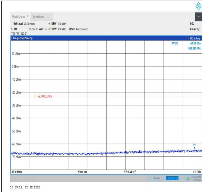
66-66-5MHz-10MHz-QPSK-QPSK-132550-132622-25RB#0-50RB#0-30~1000MHz-PASS
