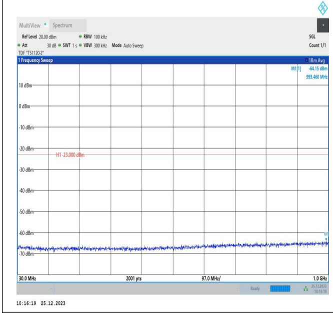
66-66-5MHz-10MHz-QPSK-QPSK-132000-132072-1RB#0-1 RB#49-30~1000MHz-PASS
