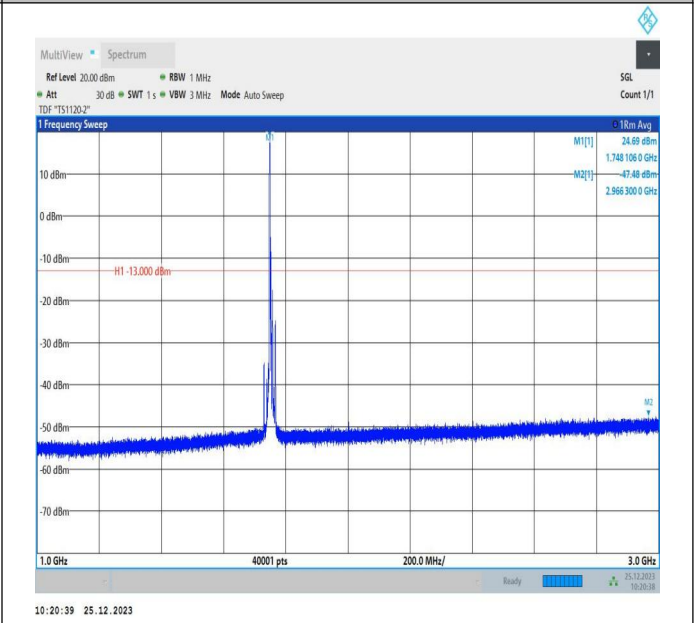
66-66-5MHz-10MHz-QPSK-QPSK-132375-132447-1RB#0-0R B#0-1000~3000MHz-PASS
