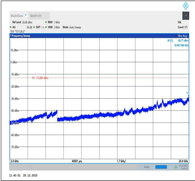
66-66-10MHz-5MHz-QPSK-QPSK-132022-132094-1RB#0-0RB#0-3000~20000MHz-PASS
