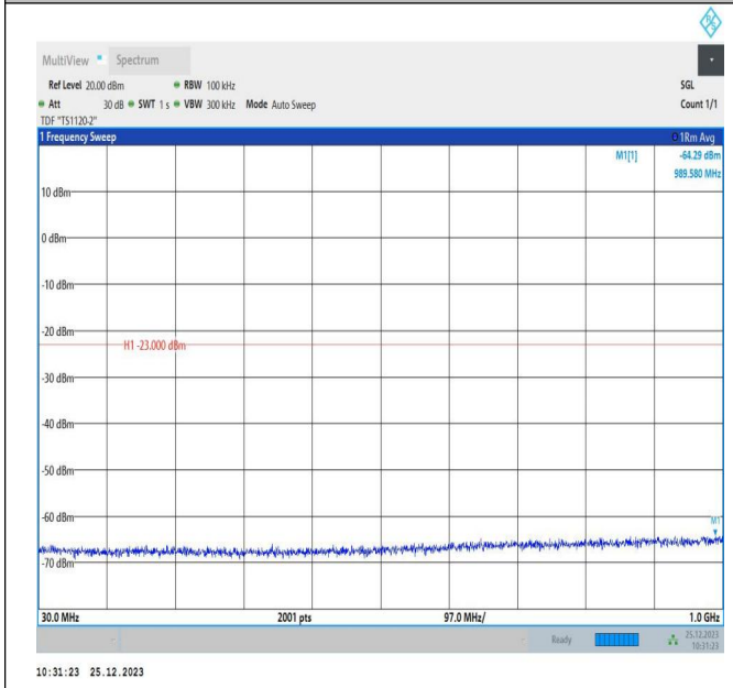
66-66-5MHz-10MHz-QPSK-QPSK-132550-132622-1RB#0-1 RB#49-30~1000MHz-PASS
