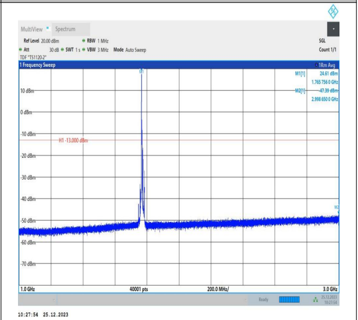
66-66-5MHz-10MHz-QPSK-QPSK-132550-132622-1RB#0-0R B#0-1000~3000MHz-PASS
