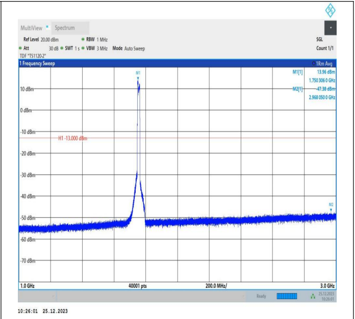
66-66-5MHz-10MHz-QPSK-QPSK-132375-132447-25RB#0-50RB#0-1000~3000MHz-PASS
