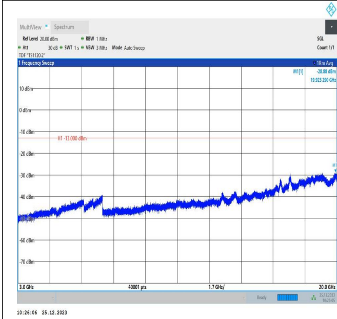
66-66-5MHz-10MHz-QPSK-QPSK-132375-132447-25RB#0-50RB#0-3000~20000MHz-PASS
