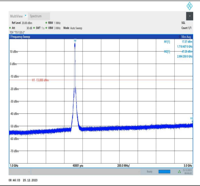
66-66-5MHz-5MHz-QPSK-QPSK-131997-132045-25RB#0-25 RB#0-1000~3000MHz-PASS
