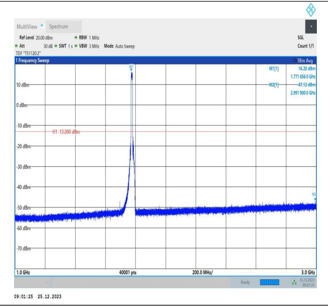
66-66-5MHz-5MHz-QPSK-QPSK-132599-132647-25RB#0-25 RB#0-1000~3000MHz-PASS
