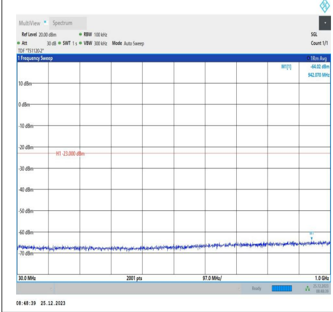
66-66-5MHz-5MHz-QPSK-QPSK-132398-132446-1RB#0-0R B#0-30~1000MHz-PASS
