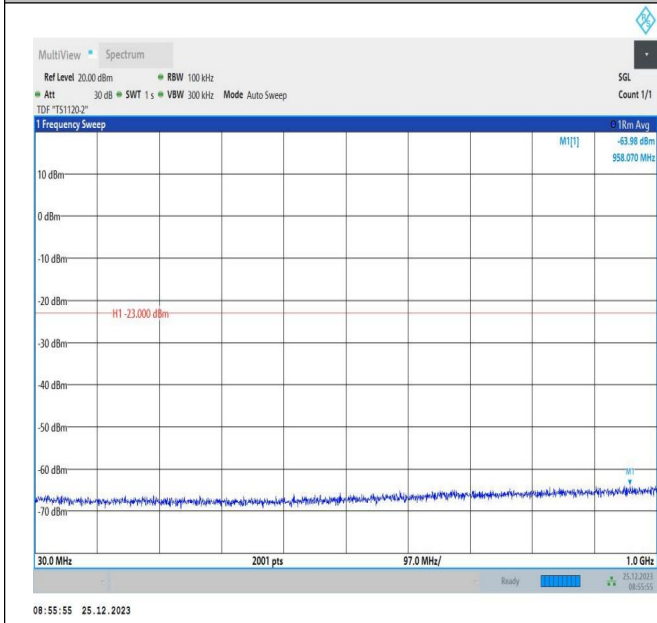
66-66-5MHz-5MHz-QPSK-QPSK-132599-132647-1RB#0-0R B#0-30~1000MHz-PASS
