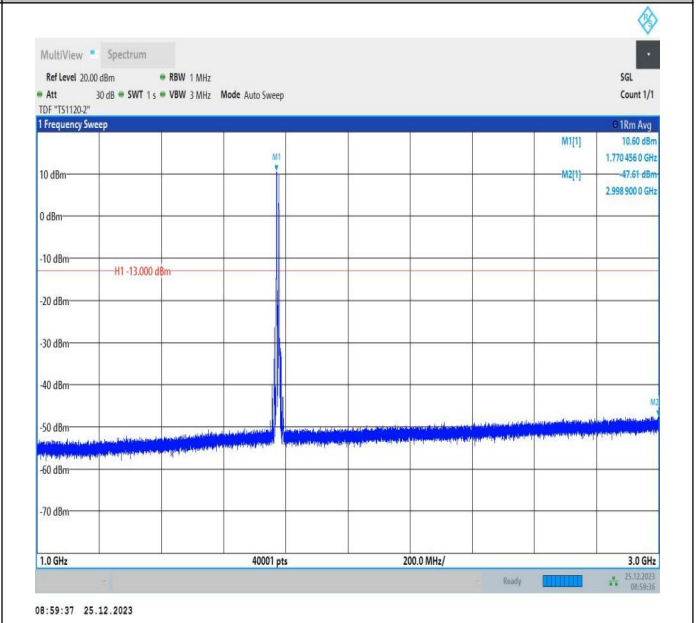
66-66-5MHz-5MHz-QPSK-QPSK-132599-132647-1RB#0-1R B#15-1000~3000MHz-PASS
