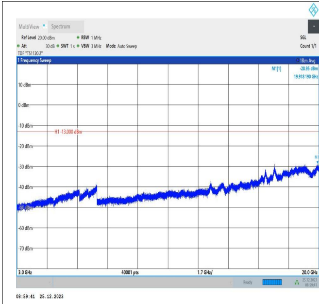
66-66-5MHz-5MHz-QPSK-QPSK-132599-132647-1RB#0-1R B#15-3000~20000MHz-PASS
