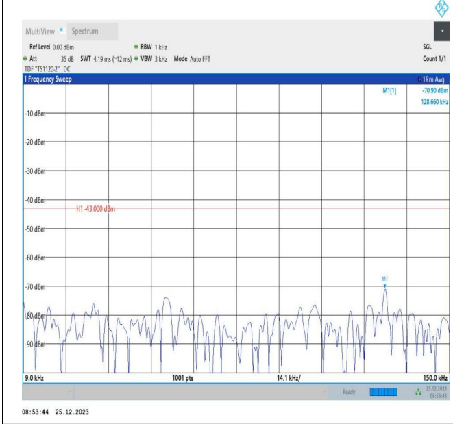
66-66-5MHz-5MHz-QPSK-QPSK-132398-132446-25RB#0-25RB#0-0.009~0.15MHz-PASS
