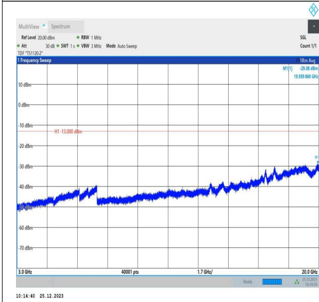
66-66-5MHz-10MHz-QPSK-QPSK-132000-132072-1RB#24-ORB#0-3000~20000MHz-PASS
