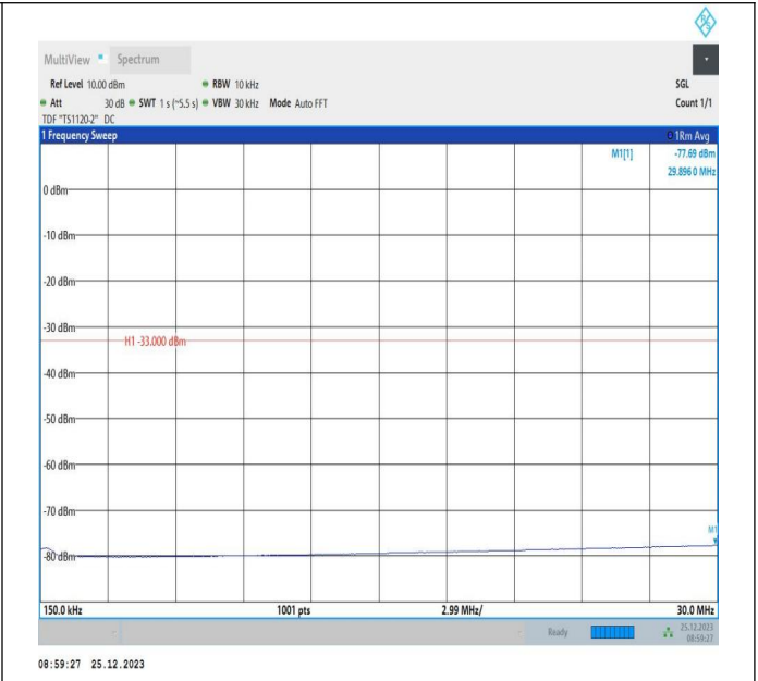
66-66-5MHz-5MHz-QPSK-QPSK-132599-132647-1RB#0-1R B#15-0.15~30MHz-PASS
