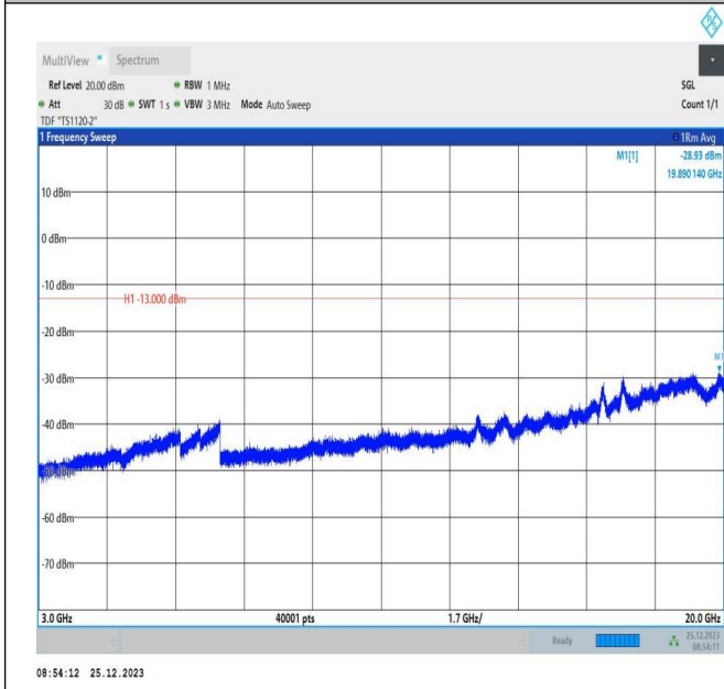
66-66-5MHz-5MHz-QPSK-QPSK-132398-132446-25RB#0-2 5RB#0-3000~20000MHz-PASS
