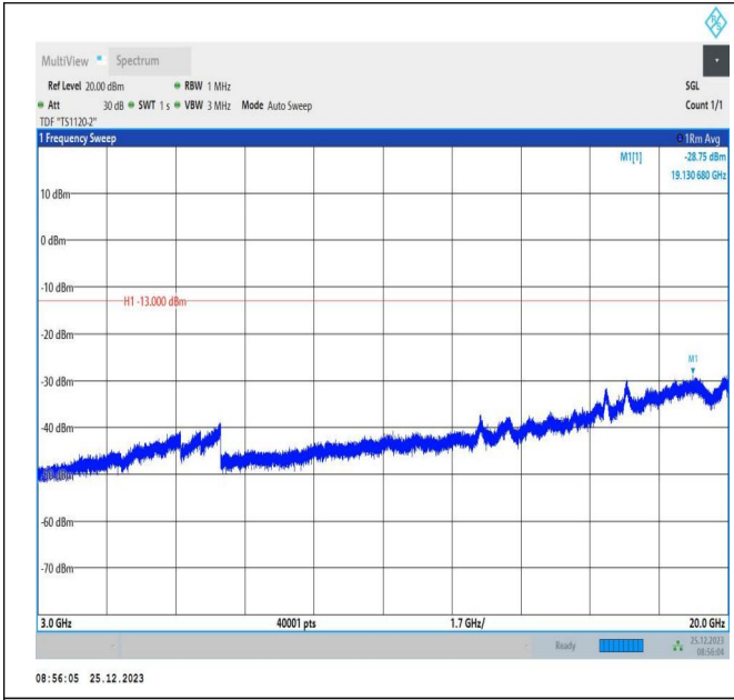
66-66-5MHz-5MHz-QPSK-QPSK-132599-132647-1RB#0-0R B#0-3000~20000MHz-PASS
