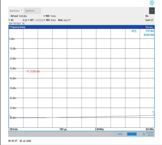
66-66-5MHz-5MHz-QPSK-QPSK-132398-132446-25RB#0-25RB#0-0.15~30MHz-PASS
