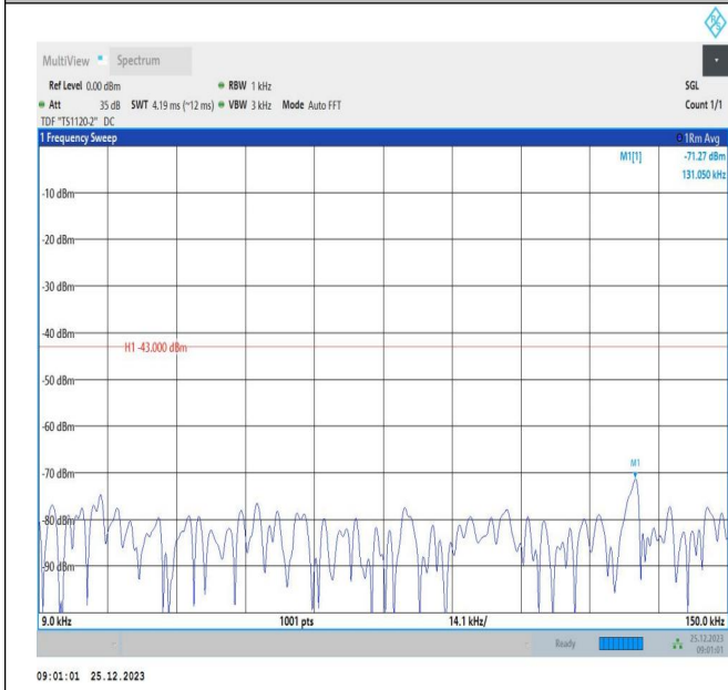
66-66-5MHz-5MHz-QPSK-QPSK-132599-132647-25RB#0-25RB#0-0.009~0.15MHz-PASS
