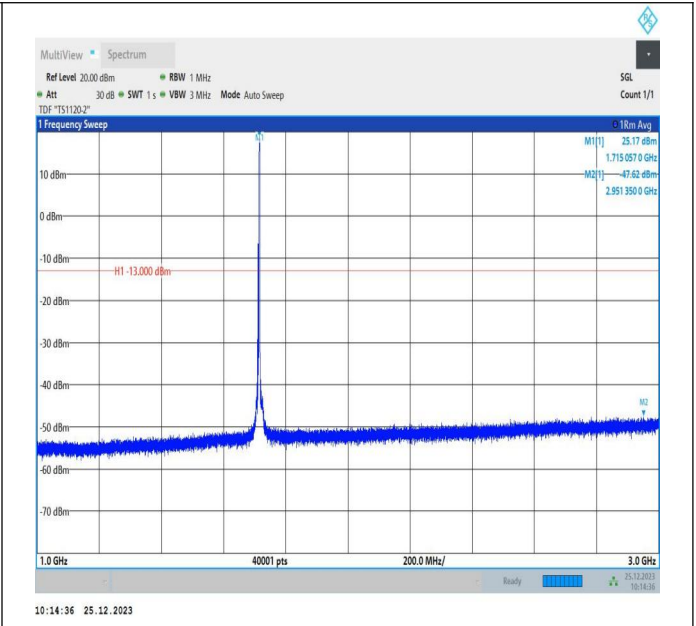
66-66-5MHz-10MHz-QPSK-QPSK-132000-132072-1RB#24-ORB#0-1000~3000MHz-PASS
