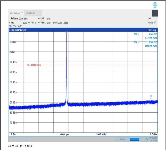
66-66-5MHz-5MHz-QPSK-QPSK-132599-132647-1RB#24-0R B#0-1000~3000MHz-PASS
