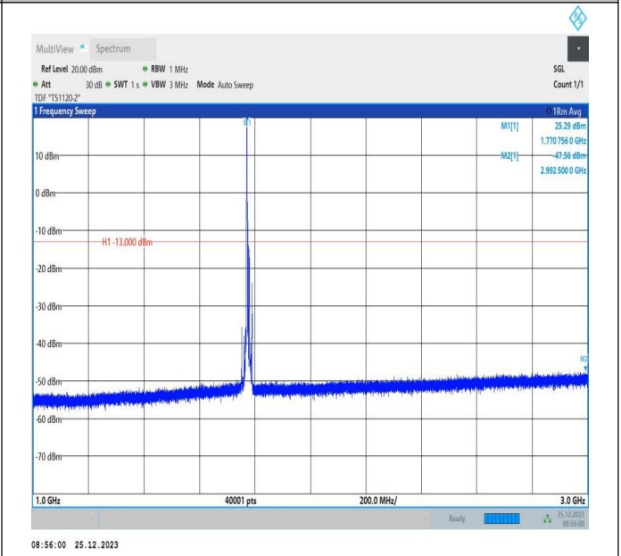
66-66-5MHz-5MHz-QPSK-QPSK-132599-132647-1RB#0-0R B#0-1000~3000MHz-PASS
