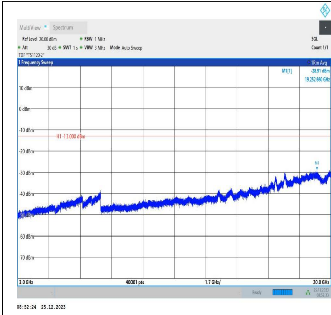
66-66-5MHz-5MHz-QPSK-QPSK-132398-132446-1RB#0-1R B#15-3000~20000MHz-PASS
