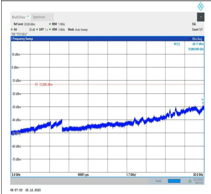
66-66-5MHz-5MHz-QPSK-QPSK-132599-132647-1RB#24-0 RB#0-3000~20000MHz-PASS
