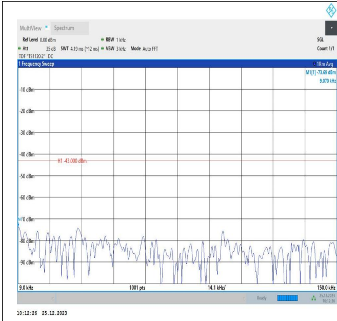
66-66-5MHz-10MHz-QPSK-QPSK-132000-132072-1RB#0-0 RB#0-0.009~0.15MHz-PASS
