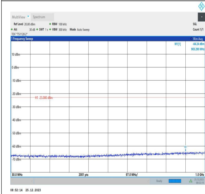
66-66-5MHz-5MHz-QPSK-QPSK-132398-132446-1RB#0-1R B#15-30~1000MHz-PASS
