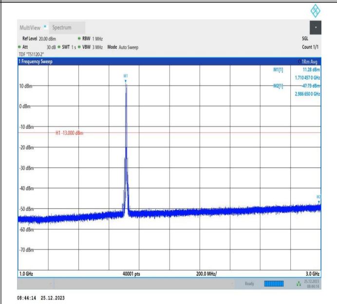
66-66-5MHz-5MHz-QPSK-QPSK-131997-132045-1RB#0-1R B#15-1000~3000MHz-PASS
