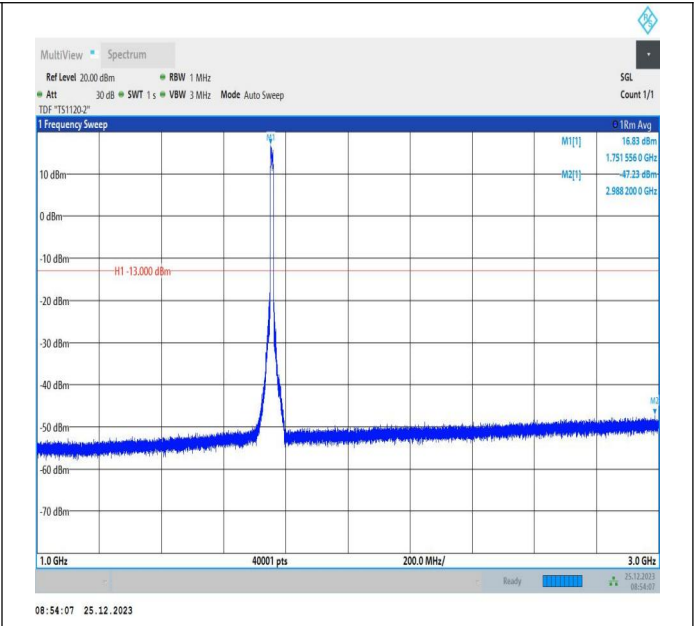
66-66-5MHz-5MHz-QPSK-QPSK-132398-132446-25RB#0-25 RB#0-1000~3000MHz-PASS
