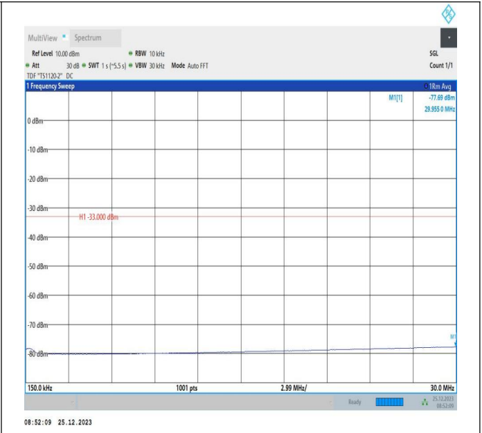
66-66-5MHz-5MHz-QPSK-QPSK-132398-132446-1RB#0-1R B#15-0.15~30MHz-PASS
