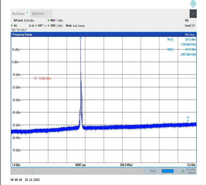
66-66-5MHz-5MHz-QPSK-QPSK-132398-132446-1RB#0-0R B#0-1000~3000MHz-PASS
