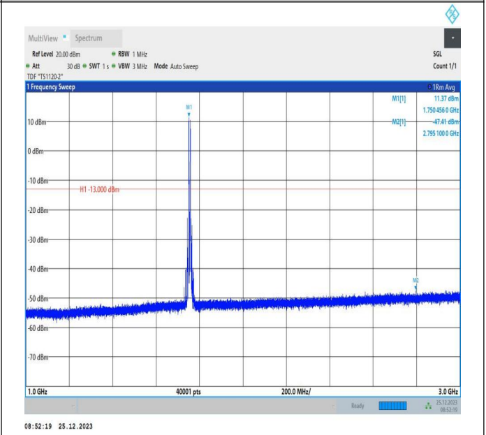
66-66-5MHz-5MHz-QPSK-QPSK-132398-132446-1RB#0-1R B#15-1000~3000MHz-PASS
