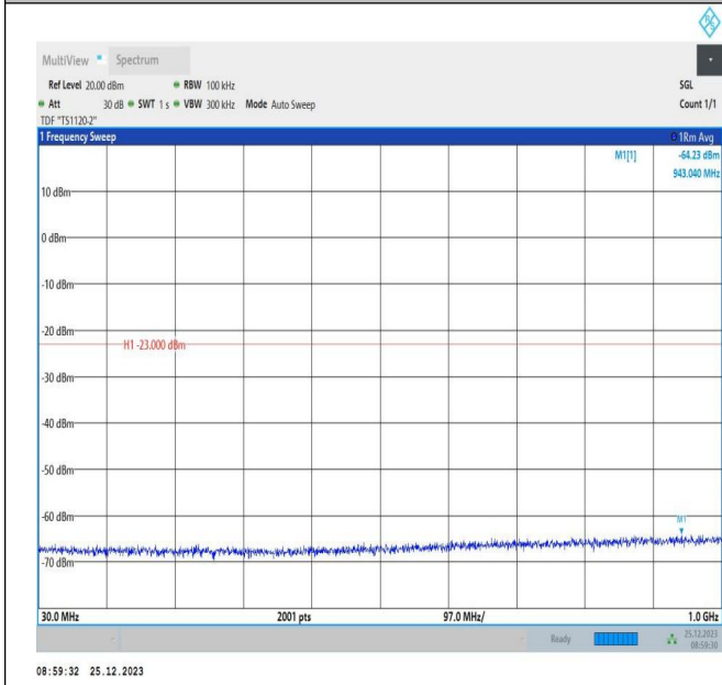
66-66-5MHz-5MHz-QPSK-QPSK-132599-132647-1RB#0-1R B#15-30~1000MHz-PASS
