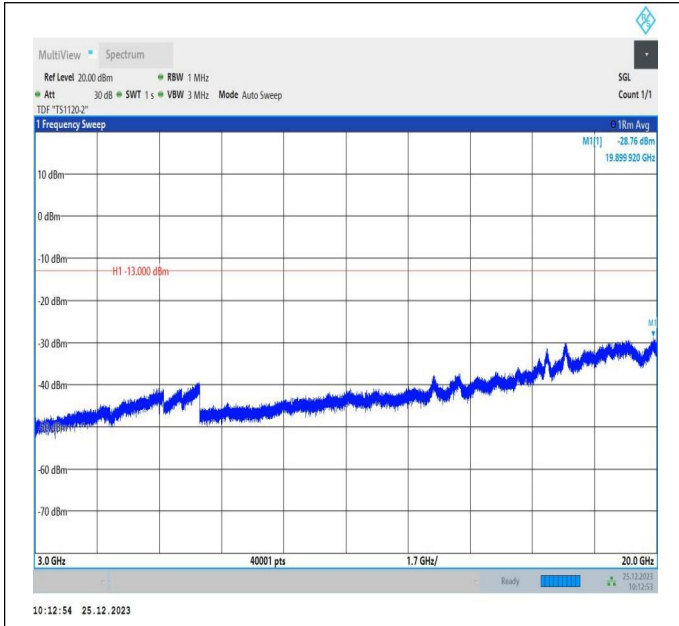
66-66-5MHz-10MHz-QPSK-QPSK-132000-132072-1RB#0-0RB#0-3000~20000MHz-PASS
