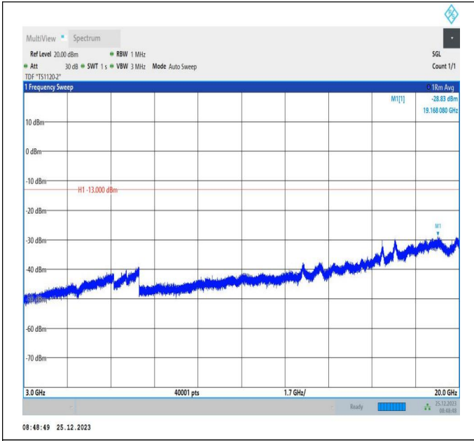
66-66-5MHz-5MHz-QPSK-QPSK-132398-132446-1RB#0-0R B#0-3000~20000MHz-PASS
