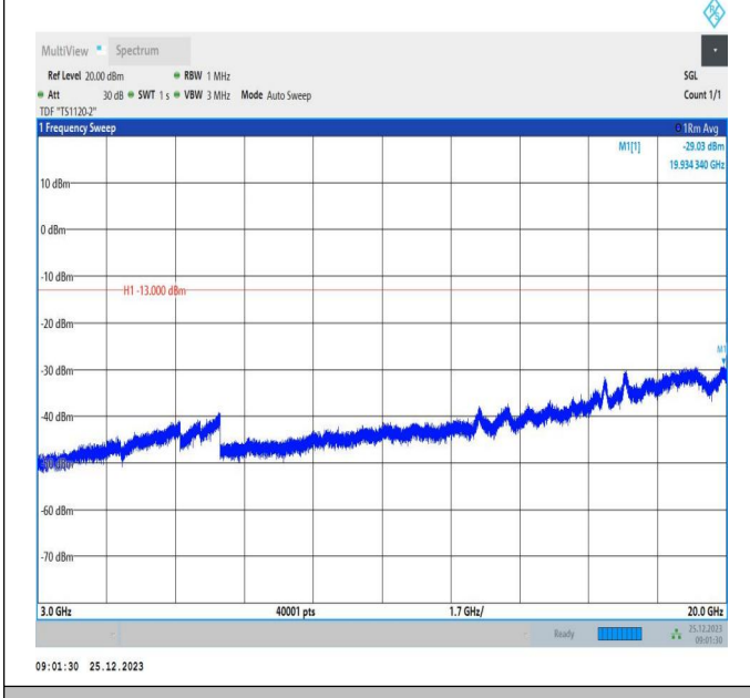
66-66-5MHz-5MHz-QPSK-QPSK-132599-132647-25RB#0-2 5RB#0-3000~20000MHz-PASS
