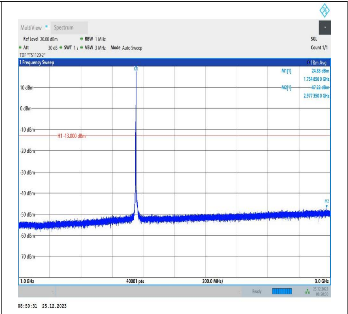
66-66-5MHz-5MHz-QPSK-QPSK-132398-132446-1RB#24-0R B#0-1000~3000MHz-PASS
