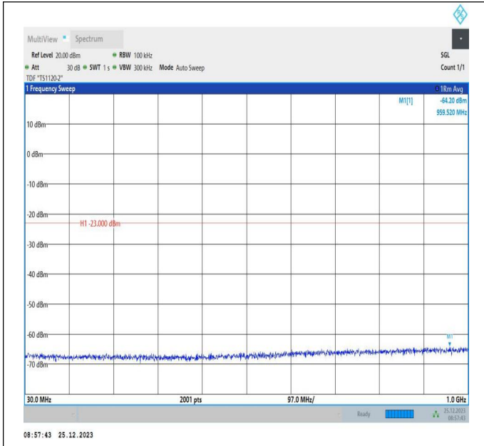
66-66-5MHz-5MHz-QPSK-QPSK-132599-132647-1RB#24-0 RB#0-30~1000MHz-PASS
