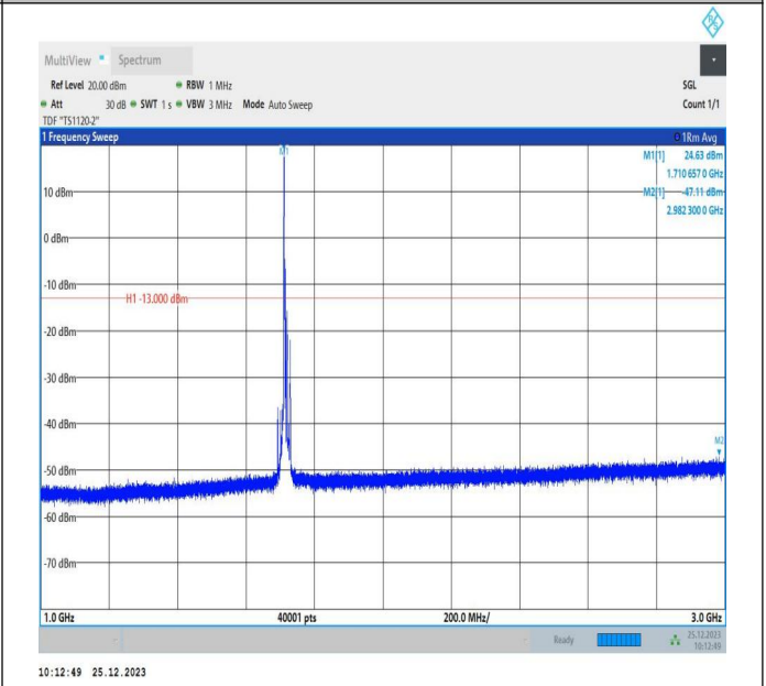
66-66-5MHz-10MHz-QPSK-QPSK-132000-132072-1RB#0-0R B#0-1000~3000MHz-PASS
