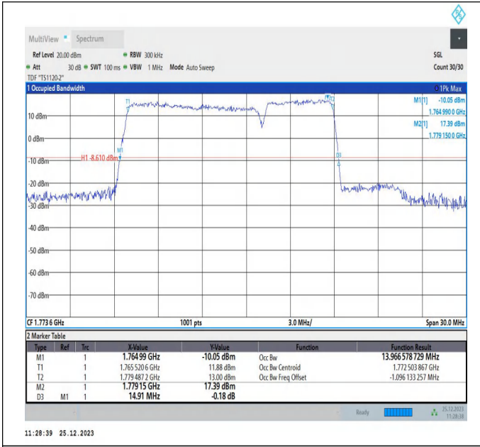
66-66-10MHz-5MHz-QPSK-QPSK-132572-132644-50RB#0-25RB#0-PASS
