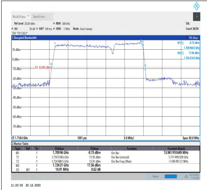
66-66-10MHz-5MHz-QPSK-QPSK-132022-132094-50RB#0-25RB#0-PASS
