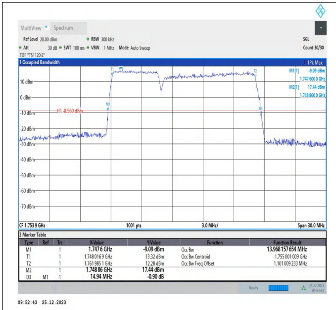
66-66-5MHz-10MHz-QPSK-QPSK-132375-132447-25RB#0-50RB#0-PASS
