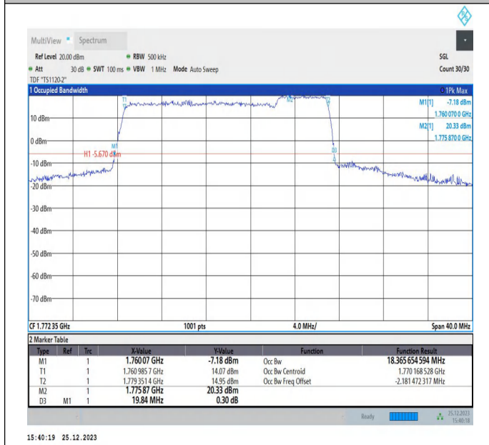
66-66-15MHz-5MHz-QPSK-QPSK-132549-132642-75RB#0-25RB#0-PASS
