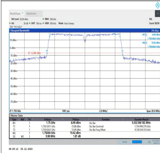
66-66-5MHz-5MHz-QPSK-QPSK-132398-132446-25RB#0-2 5RB#0-PASS
