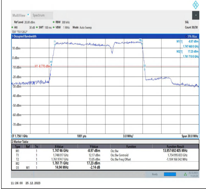
66-66-10MHz-5MHz-QPSK-QPSK-132397-132469-50RB#0-25RB#0-PASS
