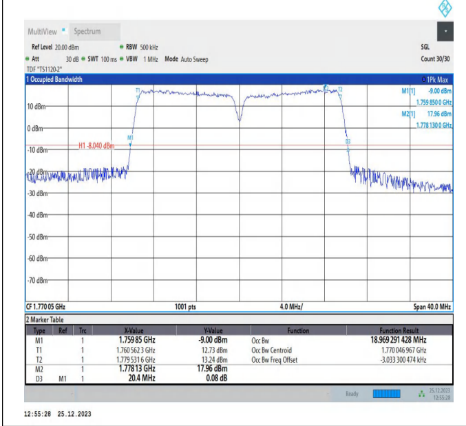
66-66-10MHz-10MHz-QPSK-QPSK-132523-132622-50RB#0 -50RB#0-PASS
