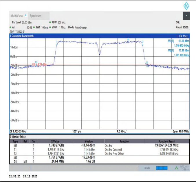
66-66-10MHz-10MHz-16QAM-16QAM-132373-132472-50RB#0-50RB#0-PASS
