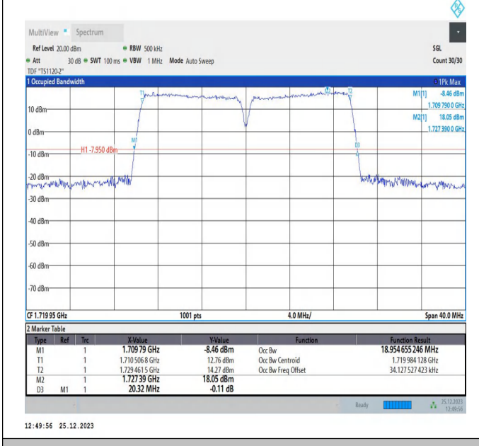
66-66-10MHz-10MHz-QPSK-QPSK-132022-132121-50RB#0-50RB#0-PASS
