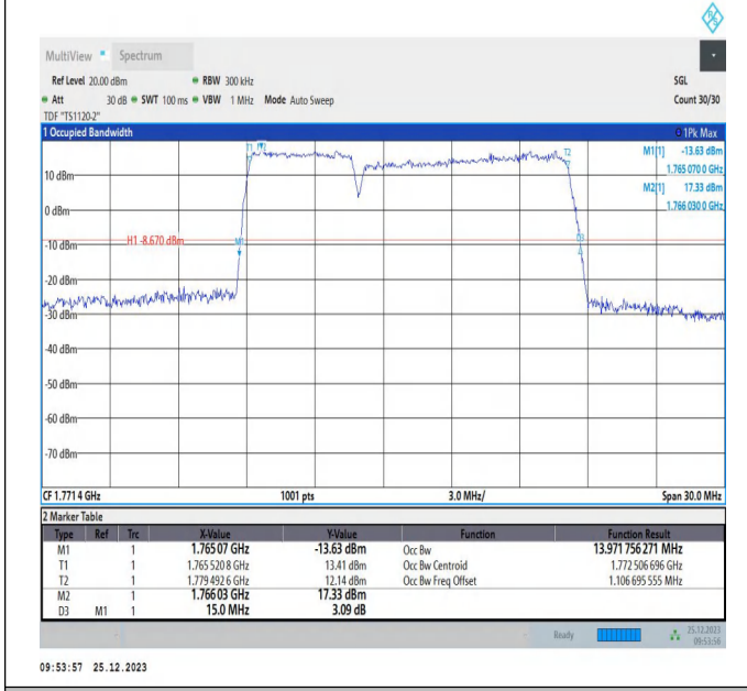
66-66-5MHz-10MHz-QPSK-QPSK-132550-132622-25RB#0-50RB#0-PASS
