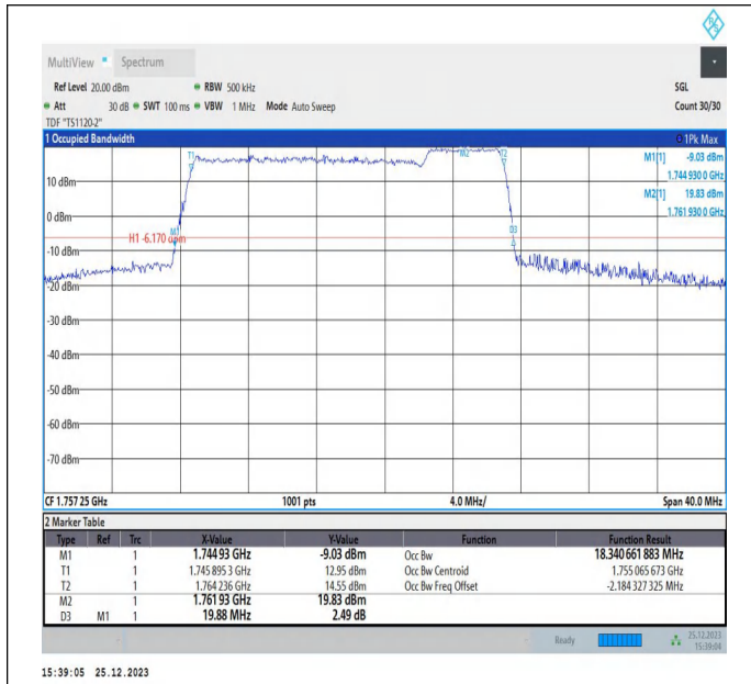
66-66-15MHz-5MHz-QPSK-QPSK-132398-132491-75RB#0-25RB#0-PASS
