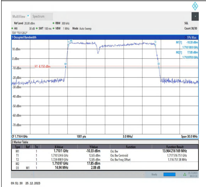
66-66-5MHz-10MHz-QPSK-QPSK-132000-132072-25RB#0-50RB#0-PASS
