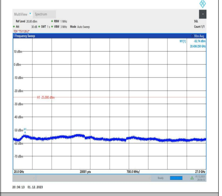
7-7-20MHz-20MHz-QPSK-QPSK-20850-21048-1RB#99-0RB# 0-20000~27000MHz-PASS
