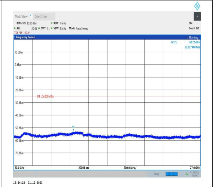
7-7-20MHz-15MHz-QPSK-QPSK-21201-21372-1RB#99-0RB# 0-20000~27000MHz-PASS
