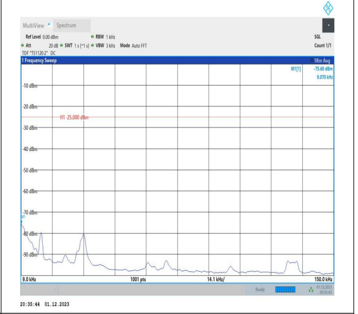
7-7-20MHz-20MHz-QPSK-QPSK-20850-21048-1RB#99-0RB# 0-0.009~0.15MHz-PASS
