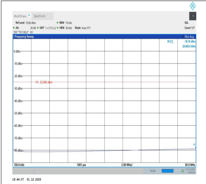
7-7-20MHz-15MHz-QPSK-QPSK-21201-21372-1RB#99-0RB# 0-0.15~30MHz-PASS
