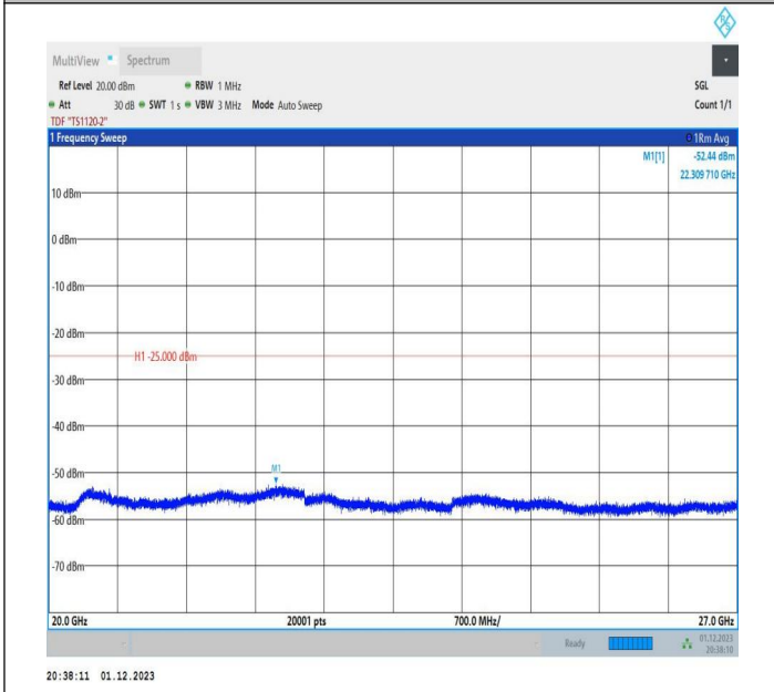
7-7-20MHz-20MHz-QPSK-QPSK-20850-21048-1RB#0-1RB#9 9-20000~27000MHz-PASS
