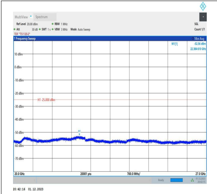
7-7-20MHz-20MHz-QPSK-QPSK-21001-21199-1RB#0-ORB#0-20000~27000MHz-PASS
