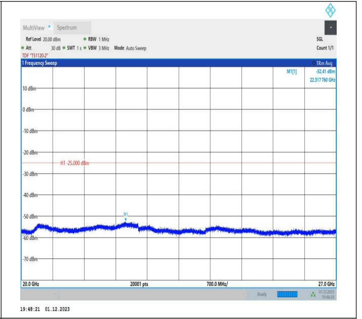
7-7-20MHz-15MHz-QPSK-QPSK-21201-21372-100RB#0-75R B#0-20000~27000MHz-PASS
