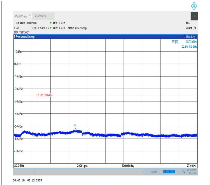
7-7-20MHz-20MHz-QPSK-QPSK-20850-21048-100RB#0-100 RB#0-20000~27000MHz-PASS
