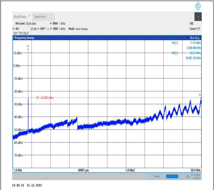
7-7-20MHz-15MHz-QPSK-QPSK-21201-21372-1RB#0-1RB#7 4-1000~20000MHz-PASS
