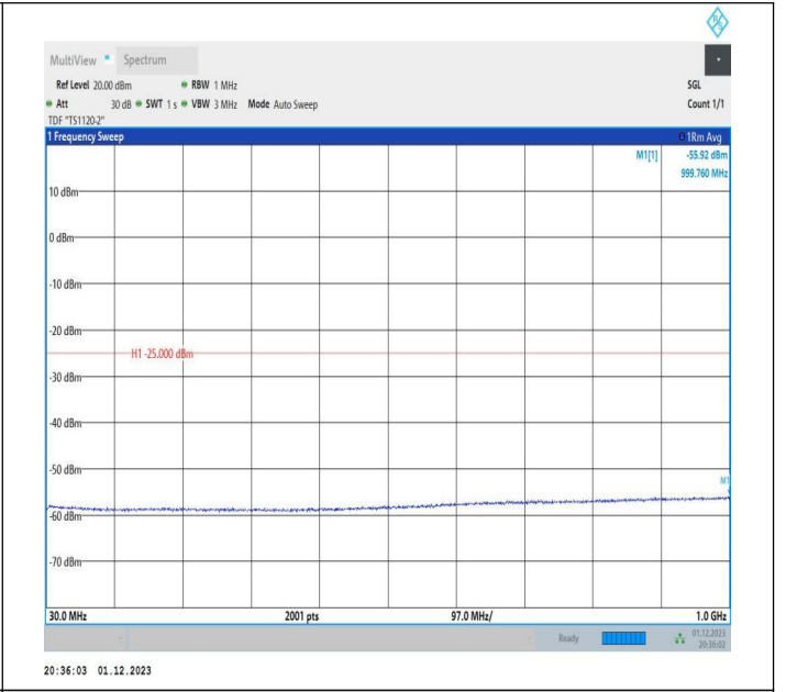
7-7-20MHz-20MHz-QPSK-QPSK-20850-21048-1RB#99-0RB# 0-30~1000MHz-PASS
