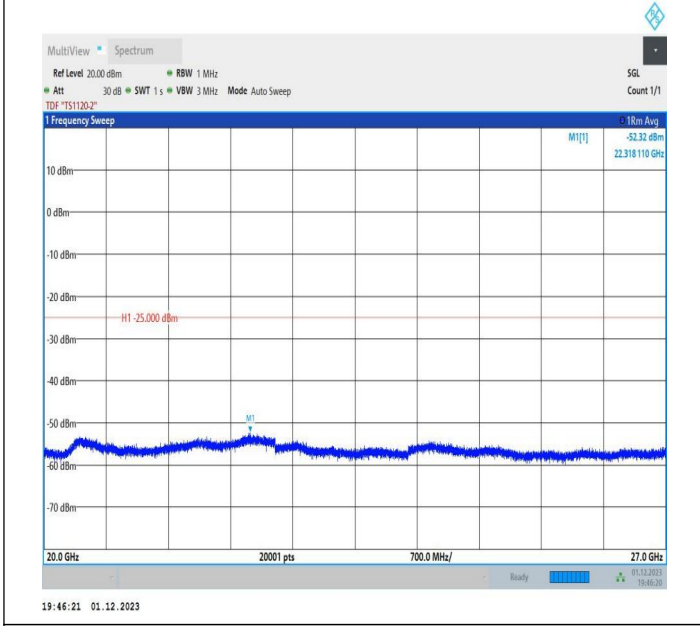
7-7-20MHz-15MHz-QPSK-QPSK-21201-21372-1RB#0-1RB#7 4-20000~27000MHz-PASS
