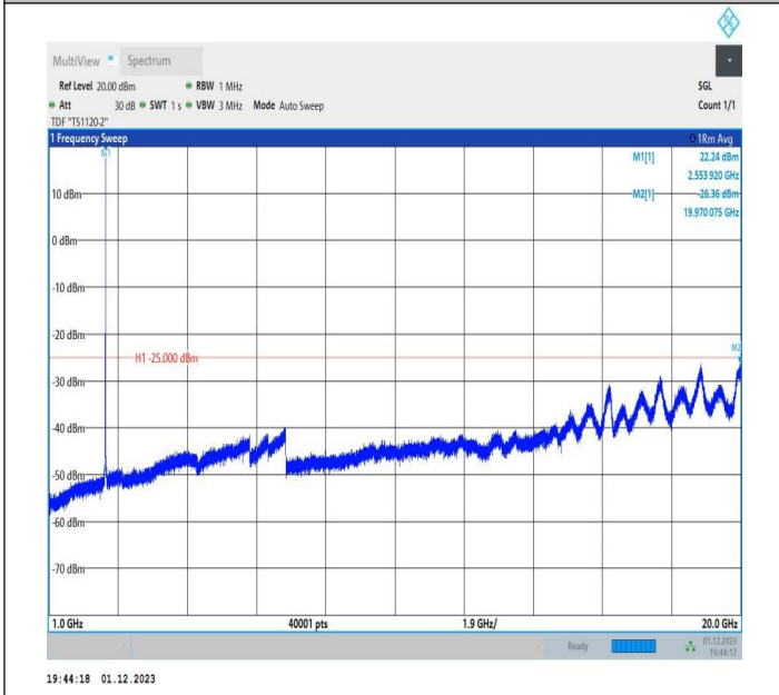
7-7-20MHz-15MHz-QPSK-QPSK-21201-21372-1RB#99-0RB# 0-1000~20000MHz-PASS
