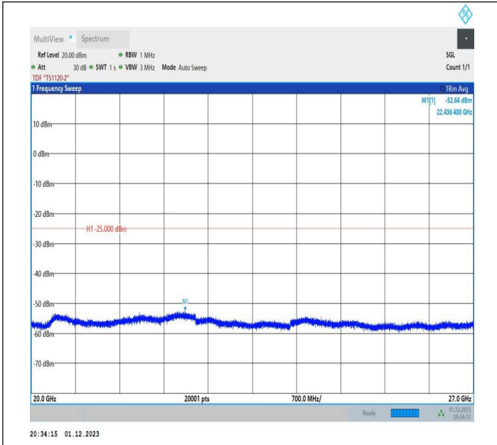
7-7-20MHz-20MHz-QPSK-QPSK-20850-21048-1RB#0-0RB#0 -20000~27000MHz-PASS
