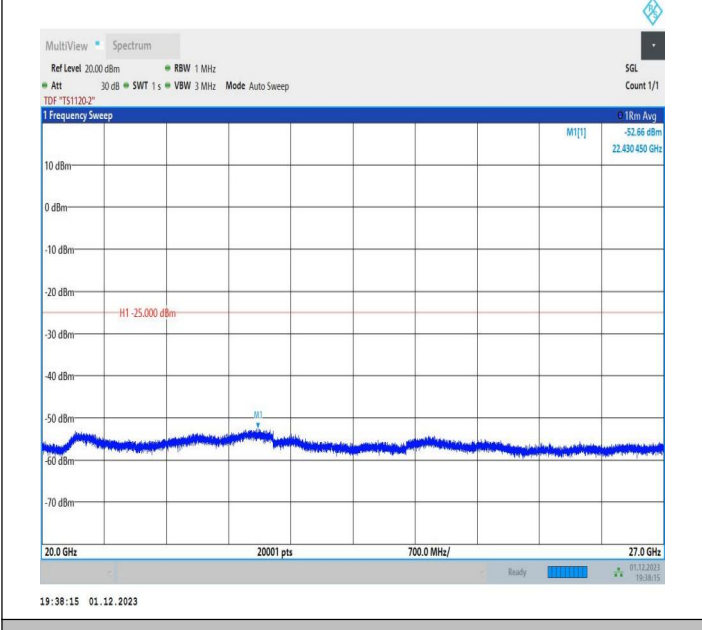
7-7-20MHz-15MHz-QPSK-QPSK-21026-21197-1RB#0-1RB#7 4-20000~27000MHz-PASS
