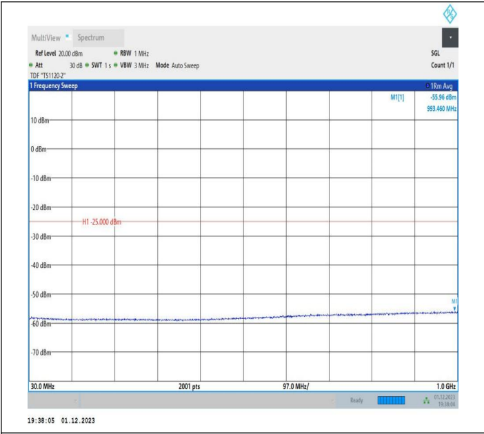
7-7-20MHz-15MHz-QPSK-QPSK-21026-21197-1RB#0-1RB#7 4-30~1000MHz-PASS
