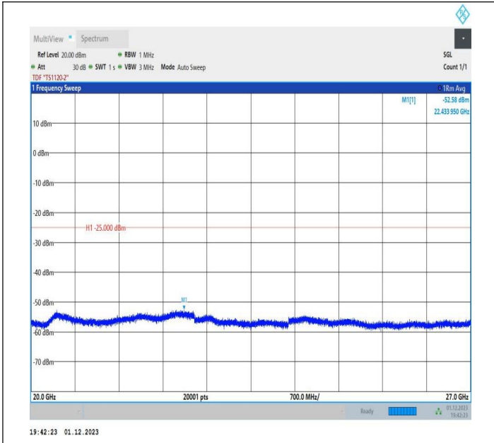
7-7-20MHz-15MHz-QPSK-QPSK-21201-21372-1RB#0-0RB#0 -20000~27000MHz-PASS
