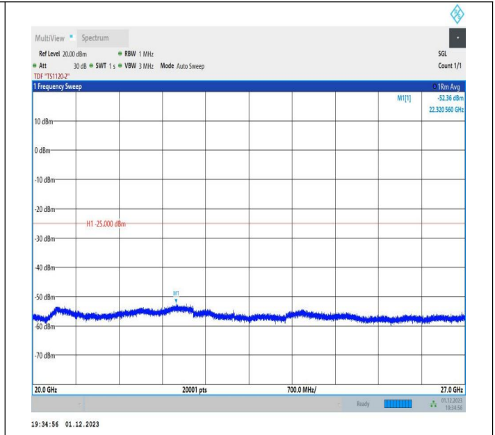
7-7-20MHz-15MHz-16QAM-16QAM-21026-21197-1RB#0-ORB #0-20000~27000MHz-PASS
