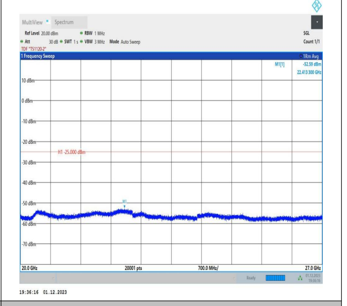
7-7-20MHz-15MHz-QPSK-QPSK-21026-21197-1RB#99-0RB# 0-20000~27000MHz-PASS
