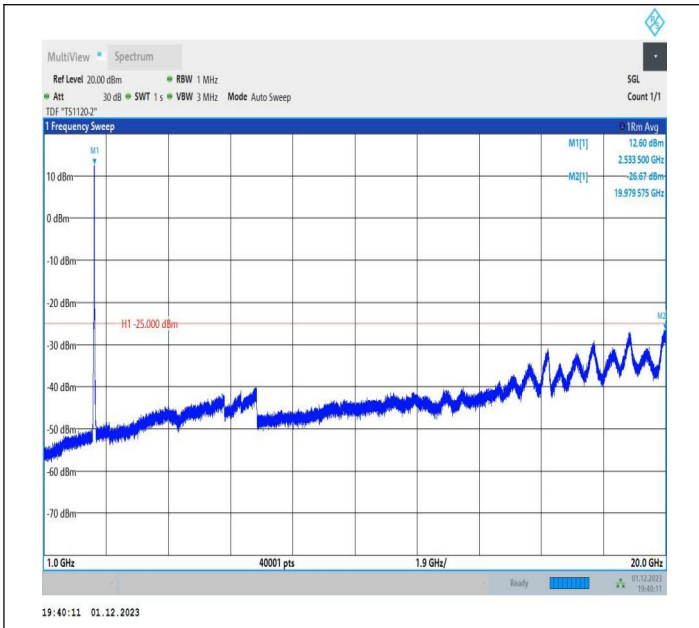
7-7-20MHz-15MHz-QPSK-QPSK-21026-21197-100RB#0-75R B#0-1000~20000MHz-PASS
