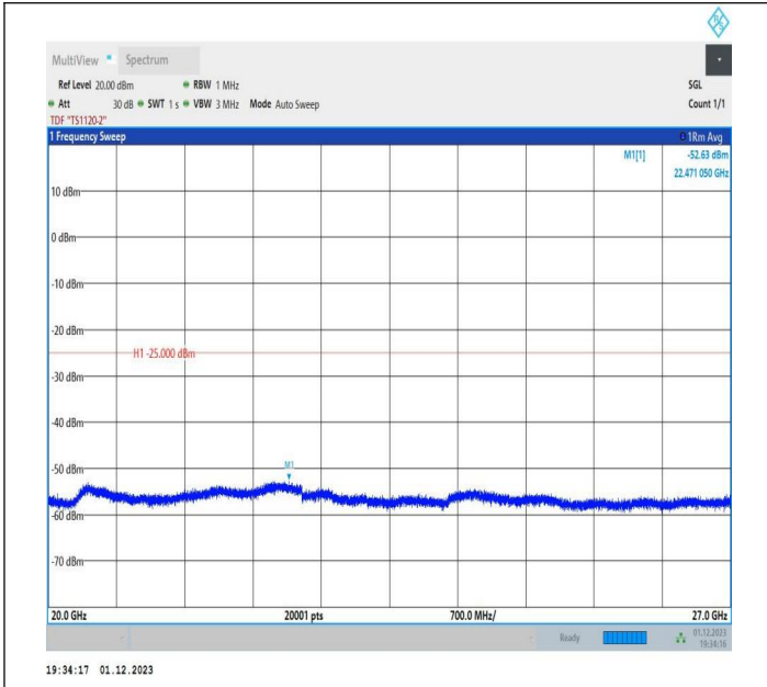
7-7-20MHz-15MHz-QPSK-QPSK-21026-21197-1RB#0-ORB#0-20000~27000MHz-PASS
