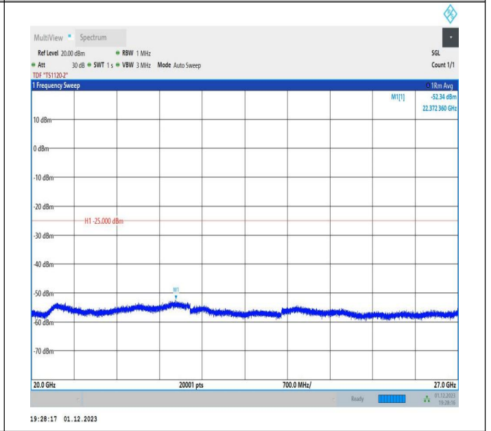
7-7-20MHz-15MHz-QPSK-QPSK-20850-21021-1RB#99-0RB# 0-20000~27000MHz-PASS
