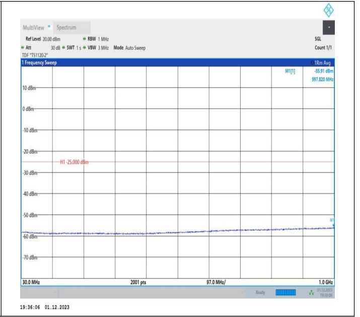
7-7-20MHz-15MHz-QPSK-QPSK-21026-21197-1RB#99-0RB# 0-30~1000MHz-PASS
