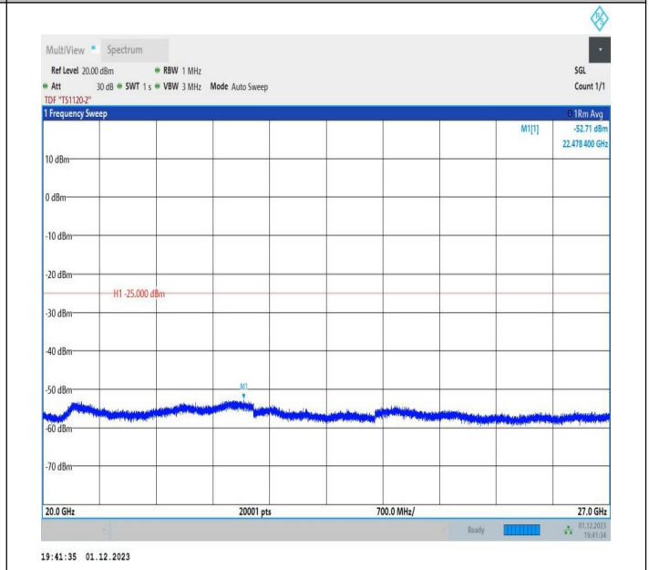
7-7-20MHz-15MHz-64QAM-64QAM-21026-21197-100RB#0-75 RB#0-20000~27000MHz-PASS
