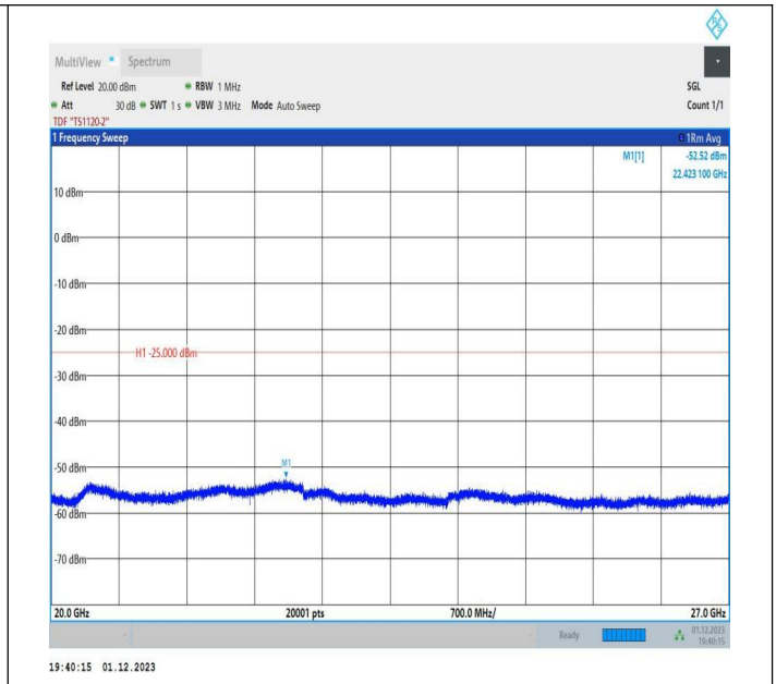
7-7-20MHz-15MHz-QPSK-QPSK-21026-21197-100RB#0-75R B#0-20000~27000MHz-PASS
