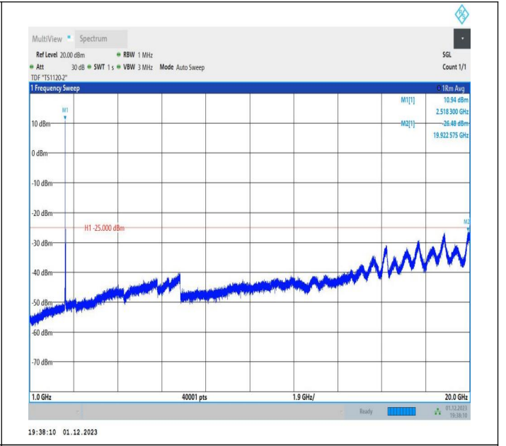
7-7-20MHz-15MHz-QPSK-QPSK-21026-21197-1RB#0-1RB#7 4-1000~20000MHz-PASS
