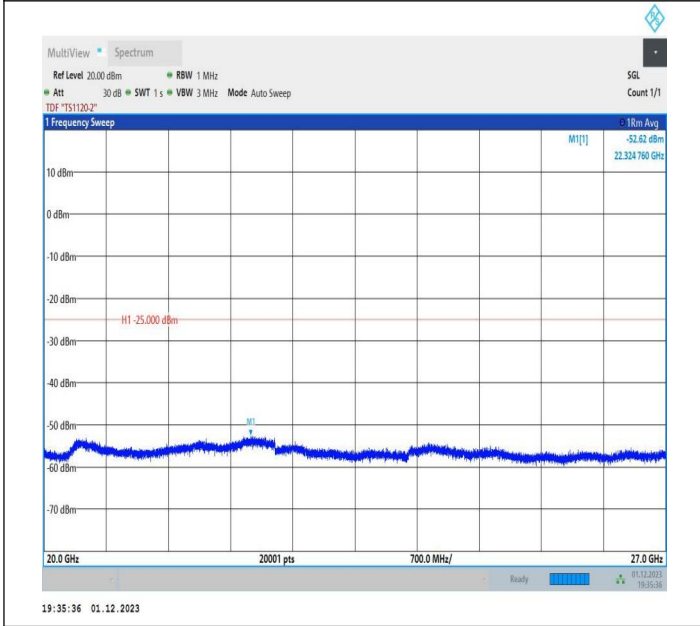
7-7-20MHz-15MHz-64QAM-64QAM-21026-21197-1RB#0-ORB #0-20000~27000MHz-PASS
