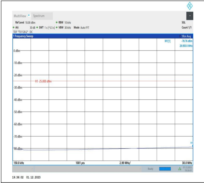
7-7-20MHz-15MHz-QPSK-QPSK-21026-21197-1RB#99-0RB# 0-0.15~30MHz-PASS
