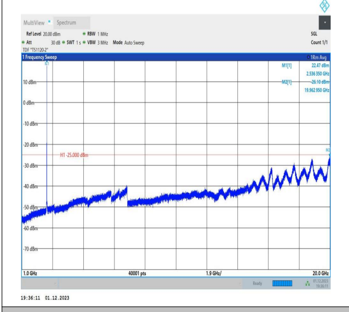
7-7-20MHz-15MHz-QPSK-QPSK-21026-21197-1RB#99-0RB# 0-1000~20000MHz-PASS
