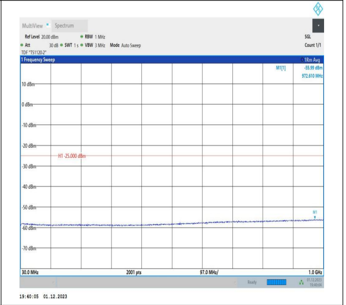
7-7-20MHz-15MHz-QPSK-QPSK-21026-21197-100RB#0-75R B#0-30~1000MHz-PASS
