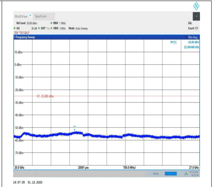
7-7-20MHz-15MHz-64QAM-64QAM-21026-21197-1RB#99-0R B#0-20000~27000MHz-PASS
