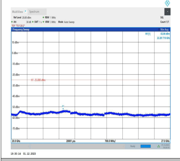
7-7-20MHz-15MHz-QPSK-QPSK-20850-21021-1RB#0-1RB#7 4-20000~27000MHz-PASS
