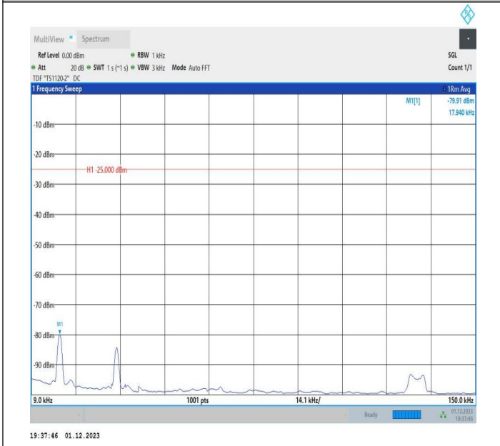
7-7-20MHz-15MHz-QPSK-QPSK-21026-21197-1RB#0-1RB#7 4-0.009~0.15MHz-PASS
