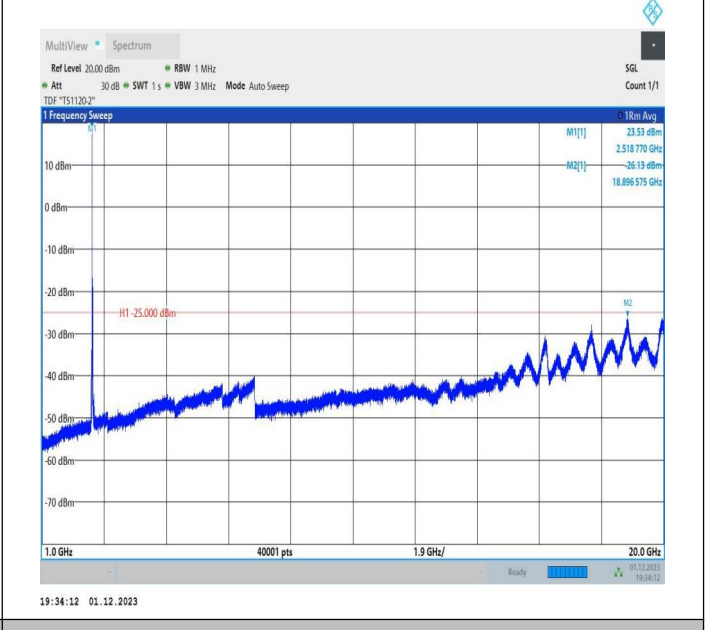
7-7-20MHz-15MHz-QPSK-QPSK-21026-21197-1RB#0-ORB#0-1000~20000MHz-PASS
