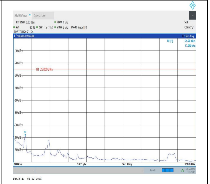
7-7-20MHz-15MHz-QPSK-QPSK-21026-21197-1RB#99-0RB# 0-0.009~0.15MHz-PASS
