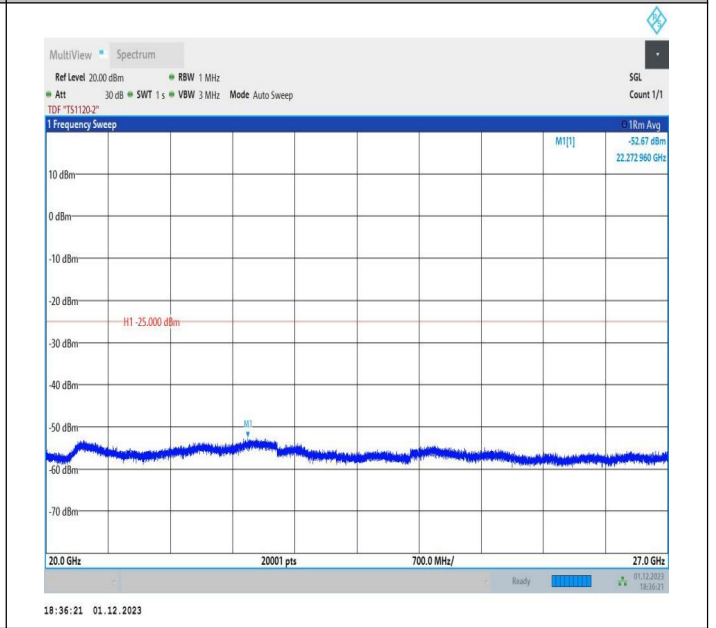
7-7-20MHz-10MHz-QPSK-QPSK-21251-21395-1RB#99-0RB# 0-20000~27000MHz-PASS
