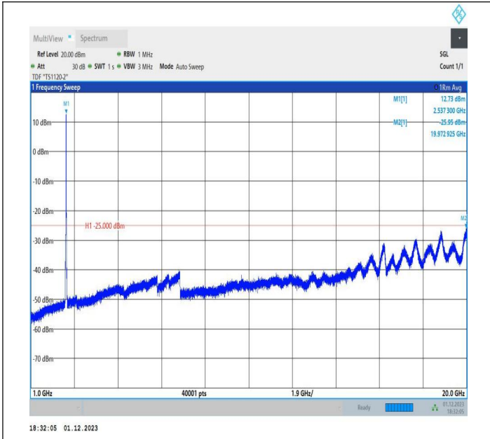
7-7-20MHz-10MHz-QPSK-QPSK-21051-21195-100RB#0-50R B#0-1000~20000MHz-PASS
