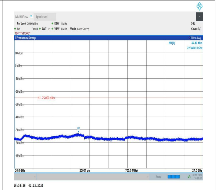
7-7-20MHz-10MHz-64QAM-64QAM-21051-21195-100RB#0-50 RB#0-20000~27000MHz-PASS
