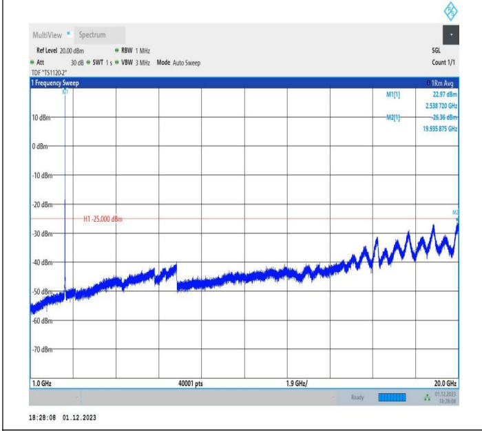
7-7-20MHz-10MHz-QPSK-QPSK-21051-21195-1RB#99-0RB# 0-1000~20000MHz-PASS
