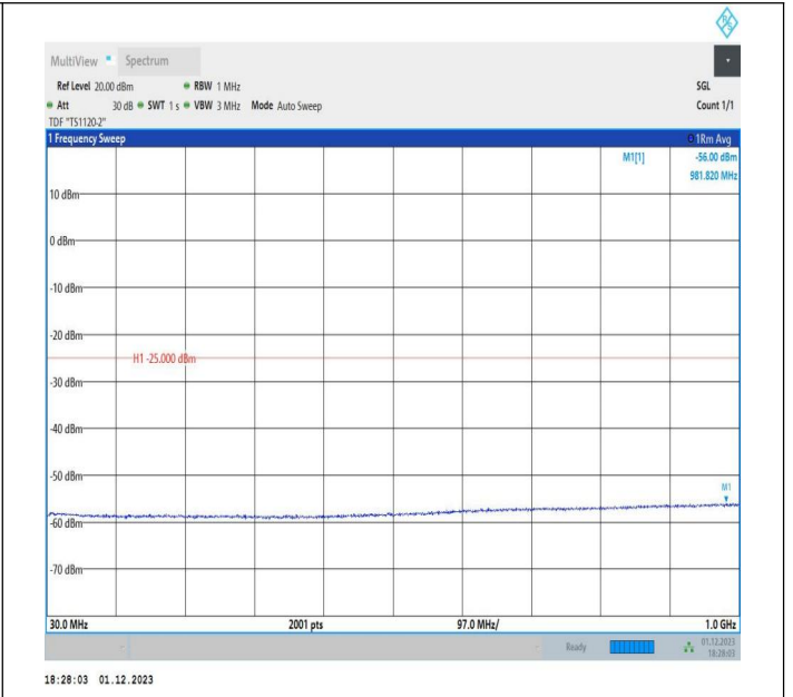
7-7-20MHz-10MHz-QPSK-QPSK-21051-21195-1RB#99-0RB# 0-30~1000MHz-PASS
