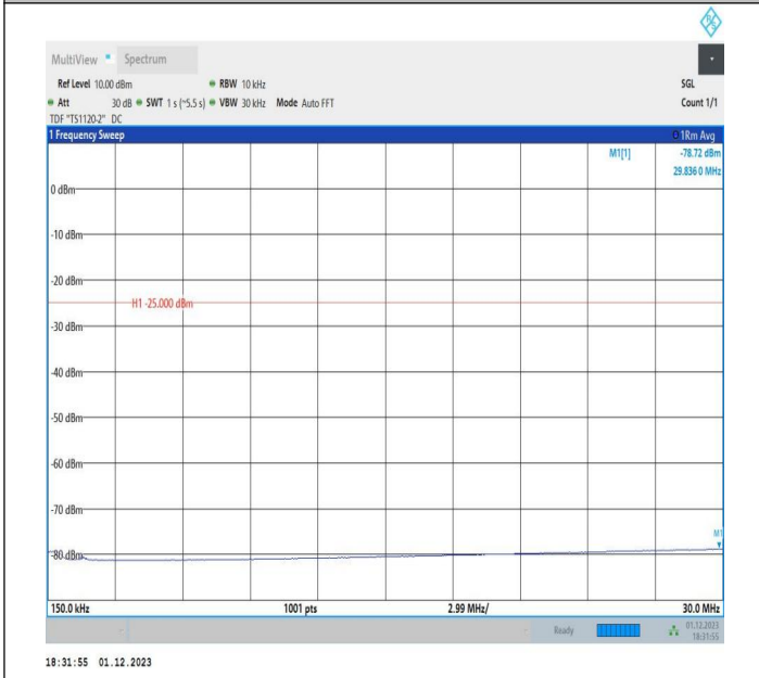
7-7-20MHz-10MHz-QPSK-QPSK-21051-21195-100RB#0-50R B#0-0.15~30MHz-PASS
