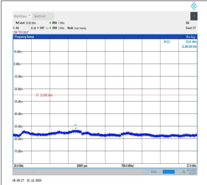
7-7-20MHz-10MHz-QPSK-QPSK-21251-21395-1RB#0-0RB#0 -20000~27000MHz-PASS
