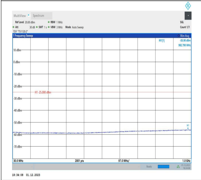
7-7-20MHz-10MHz-QPSK-QPSK-21251-21395-1RB#0-0RB#0 -30~1000MHz-PASS
