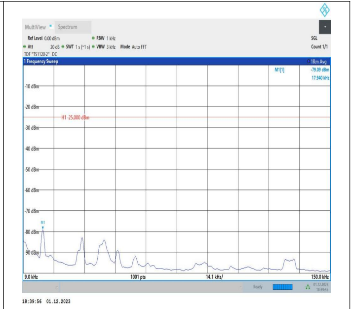
7-7-20MHz-10MHz-QPSK-QPSK-21251-21395-100RB#0-50R B#0-0.009~0.15MHz-PASS
