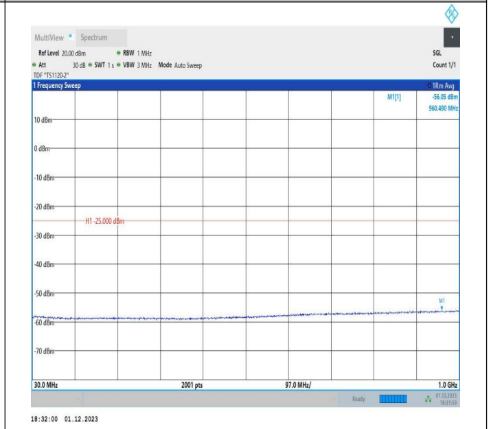
7-7-20MHz-10MHz-QPSK-QPSK-21051-21195-100RB#0-50R B#0-30~1000MHz-PASS
