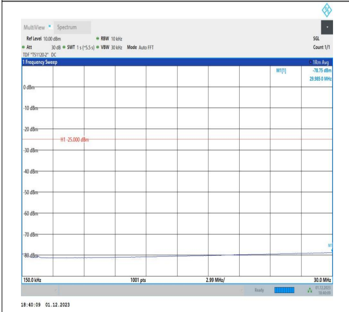
7-7-20MHz-10MHz-QPSK-QPSK-21251-21395-100RB#0-50R B#0-0.15~30MHz-PASS
