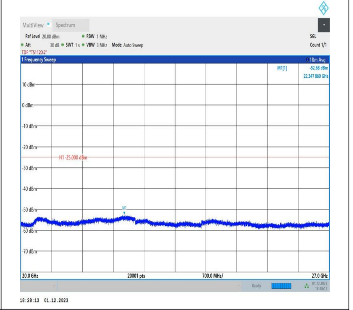
7-7-20MHz-10MHz-QPSK-QPSK-21051-21195-1RB#99-0RB# 0-20000~27000MHz-PASS
