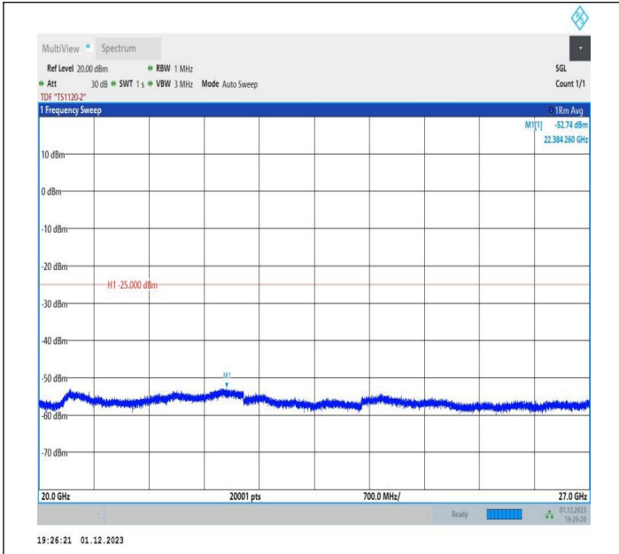
7-7-20MHz-15MHz-QPSK-QPSK-20850-21021-1RB#0-0RB#0 -20000~27000MHz-PASS
