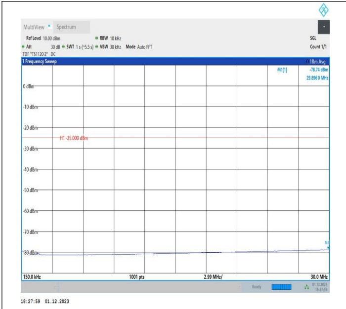
7-7-20MHz-10MHz-QPSK-QPSK-21051-21195-1RB#99-0RB# 0-0.15~30MHz-PASS
