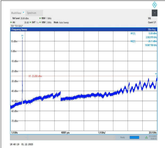
7-7-20MHz-10MHz-QPSK-QPSK-21251-21395-100RB#0-50R B#0-1000~20000MHz-PASS
