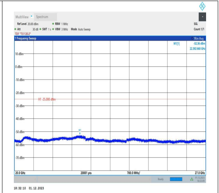
7-7-20MHz-10MHz-QPSK-QPSK-21051-21195-100RB#0-50R B#0-20000~27000MHz-PASS
