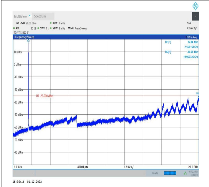
7-7-20MHz-10MHz-QPSK-QPSK-21251-21395-1RB#99-0RB# 0-1000~20000MHz-PASS
