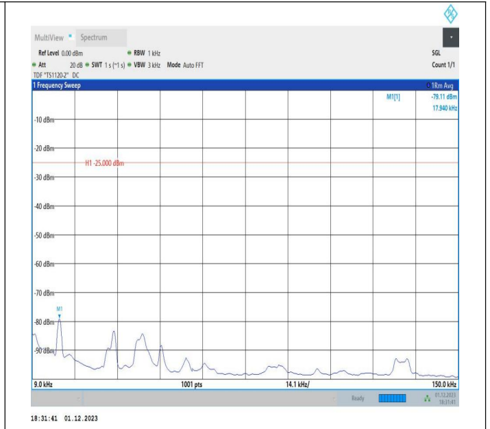
7-7-20MHz-10MHz-QPSK-QPSK-21051-21195-100RB#0-50R B#0-0.009~0.15MHz-PASS
