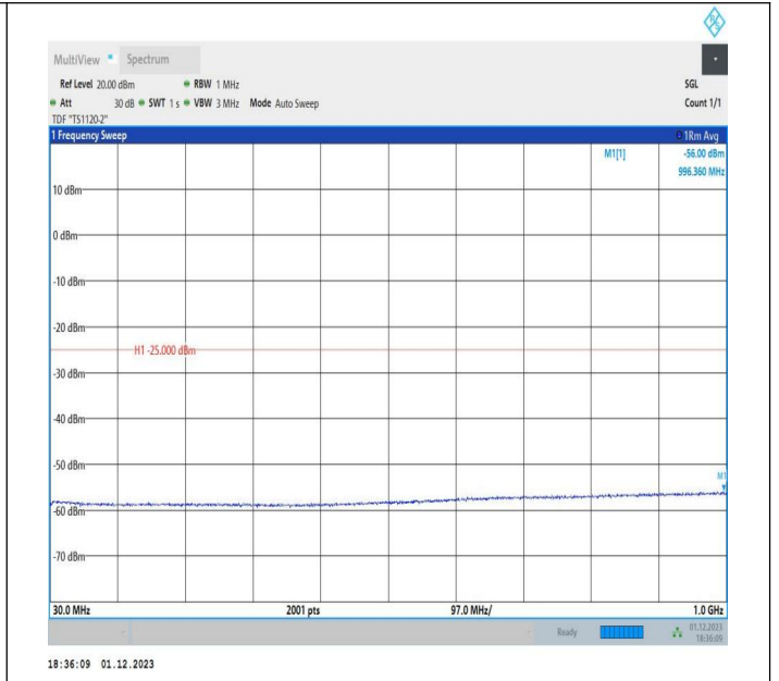
7-7-20MHz-10MHz-QPSK-QPSK-21251-21395-1RB#99-0RB# 0-30~1000MHz-PASS
