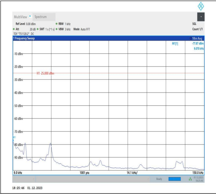
7-7-20MHz-10MHz-QPSK-QPSK-21051-21195-1RB#0-ORB#0-0.009~0.15MHz-PASS
