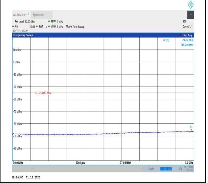
7-7-20MHz-10MHz-QPSK-QPSK-20850-20994-100RB#0-50R B#0-30~1000MHz-PASS
