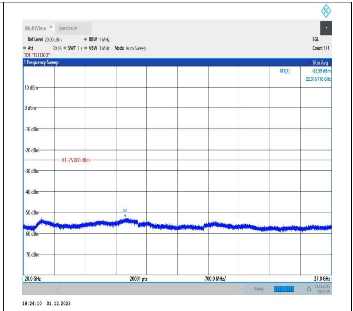
7-7-20MHz-10MHz-QPSK-QPSK-20850-20994-100RB#0-50R B#0-20000~27000MHz-PASS
