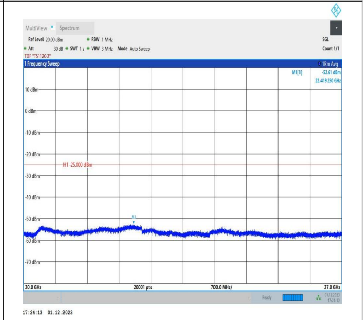
7-7-15MHz-20MHz-QPSK-QPSK-21179-21350-1RB#74-0RB# 0-20000~27000MHz-PASS
