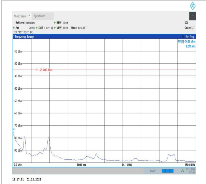
7-7-20MHz-10MHz-QPSK-QPSK-20850-20994-1RB#0-0RB#0 -0.009~0.15MHz-PASS
