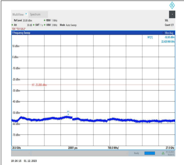
7-7-20MHz-10MHz-QPSK-QPSK-21051-21195-1RB#0-ORB#0-20000~27000MHz-PASS
