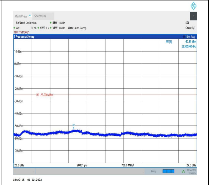
7-7-20MHz-10MHz-QPSK-QPSK-20850-20994-1RB#99-0RB# 0-20000~27000MHz-PASS
