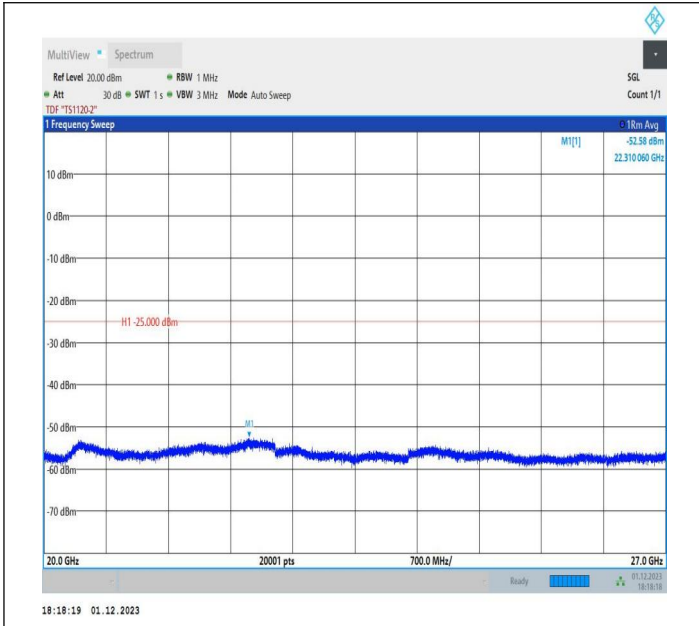
7-7-20MHz-10MHz-QPSK-QPSK-20850-20994-1RB#0-0RB#0 -20000~27000MHz-PASS
