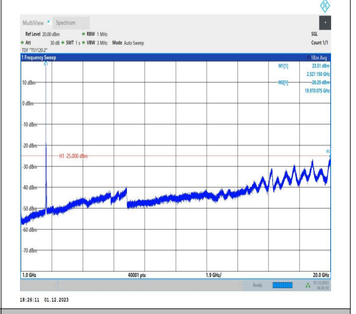
7-7-20MHz-10MHz-QPSK-QPSK-21051-21195-1RB#0-ORB#0-1000~20000MHz-PASS
