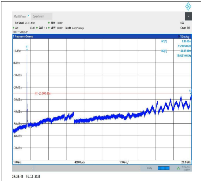
7-7-20MHz-10MHz-QPSK-QPSK-20850-20994-100RB#0-50R B#0-1000~20000MHz-PASS
