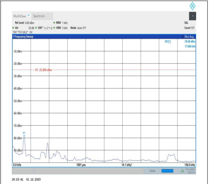
7-7-20MHz-10MHz-QPSK-QPSK-20850-20994-100RB#0-50R B#0-0.009~0.15MHz-PASS
