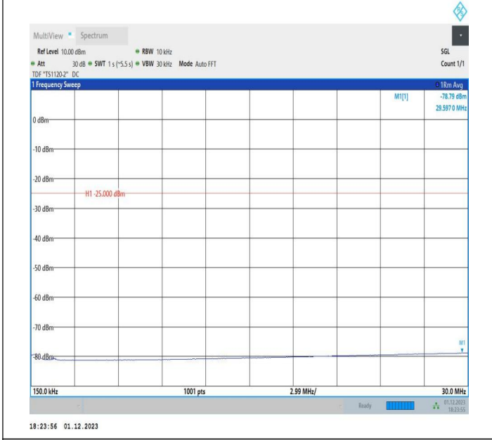
7-7-20MHz-10MHz-QPSK-QPSK-20850-20994-100RB#0-50R B#0-0.15~30MHz-PASS
