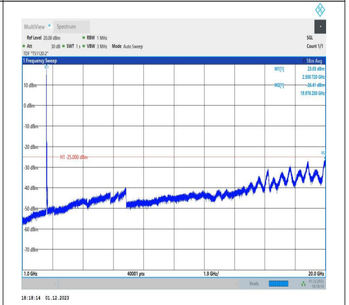
7-7-20MHz-10MHz-QPSK-QPSK-20850-20994-1RB#0-0RB#0 -1000~20000MHz-PASS
