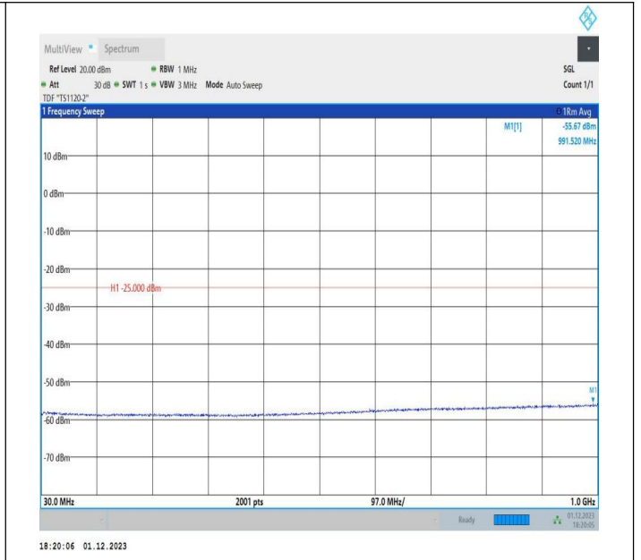
7-7-20MHz-10MHz-QPSK-QPSK-20850-20994-1RB#99-0RB# 0-30~1000MHz-PASS
