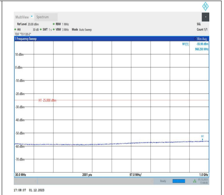
7-7-15MHz-20MHz-QPSK-QPSK-20828-20999-1RB#74-0RB# 0-30~1000MHz-PASS
