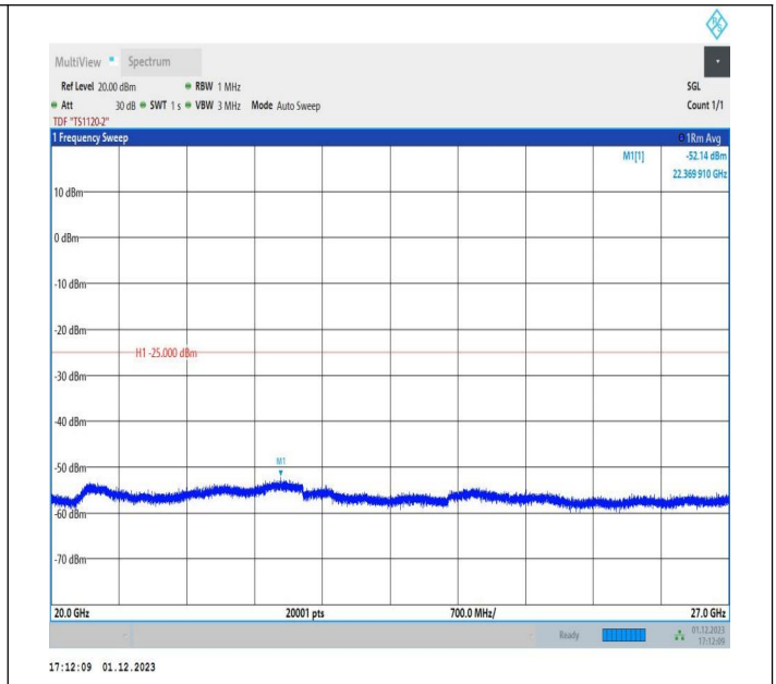
7-7-15MHz-20MHz-QPSK-QPSK-20828-20999-75RB#0-100R B#0-20000~27000MHz-PASS
