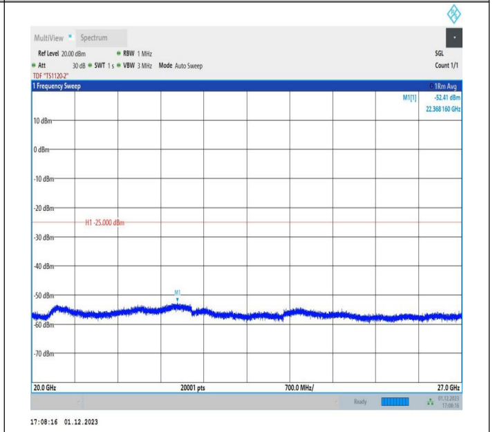
7-7-15MHz-20MHz-QPSK-QPSK-20828-20999-1RB#74-0RB# 0-20000~27000MHz-PASS
