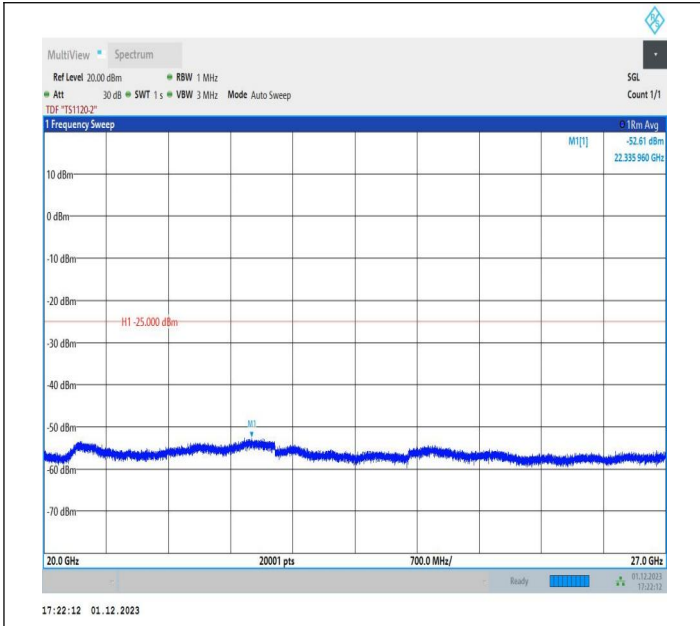
7-7-15MHz-20MHz-QPSK-QPSK-21179-21350-1RB#0-ORB#0-20000~27000MHz-PASS
