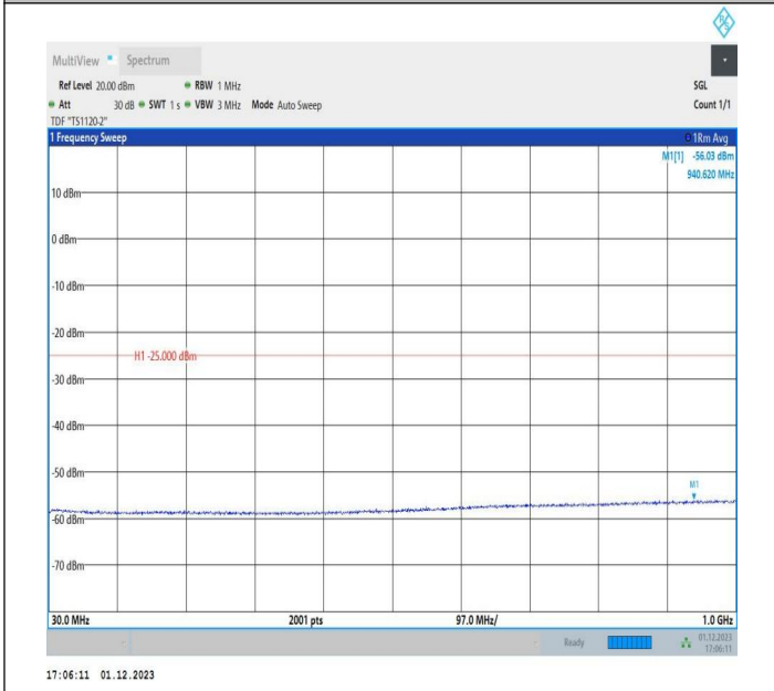
7-7-15MHz-20MHz-QPSK-QPSK-20828-20999-1RB#0-0RB#0 -30~1000MHz-PASS
