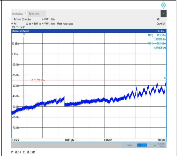
7-7-15MHz-20MHz-QPSK-QPSK-20828-20999-1RB#0-0RB#0 -1000~20000MHz-PASS
