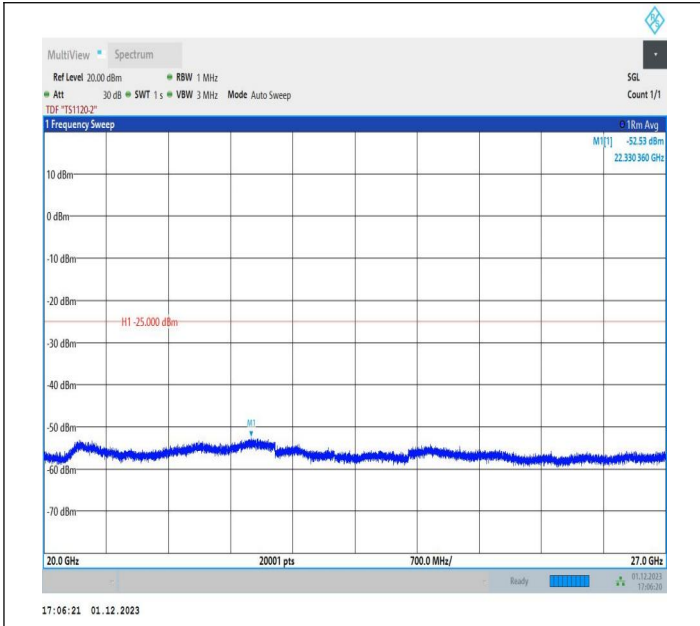
7-7-15MHz-20MHz-QPSK-QPSK-20828-20999-1RB#0-0RB#0 -20000~27000MHz-PASS
