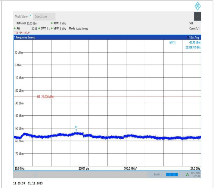
7-7-15MHz-10MHz-QPSK-QPSK-20825-20945-75RB#0-50RB #0-20000~27000MHz-PASS
