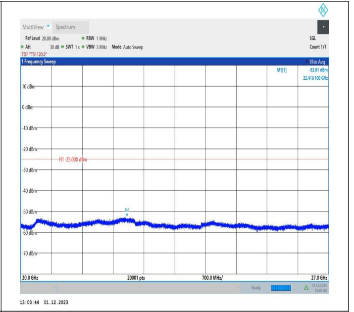
7-7-15MHz-10MHz-QPSK-QPSK-21051-21171-75RB#0-50RB #0-20000~27000MHz-PASS
