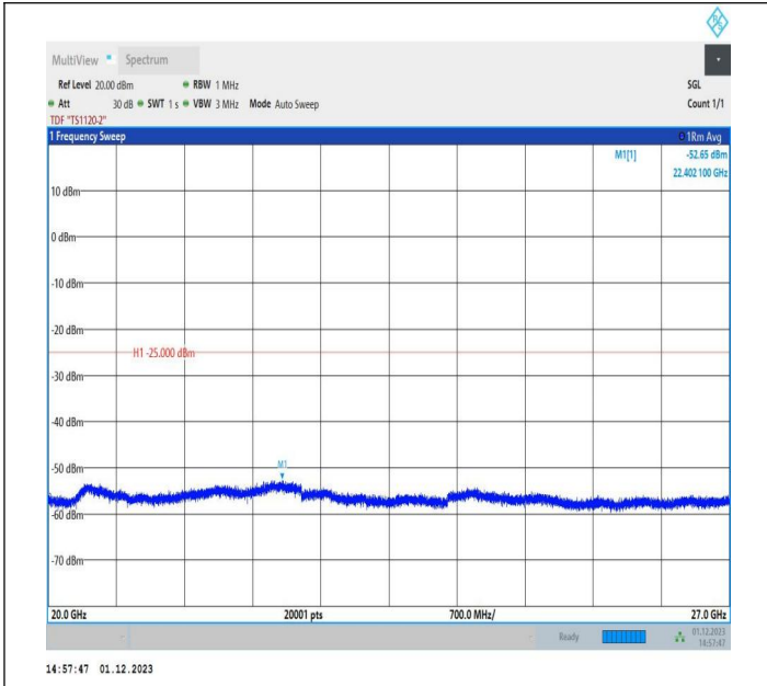
7-7-15MHz-10MHz-QPSK-QPSK-21051-21171-1RB#0-ORB#0-20000~27000MHz-PASS
