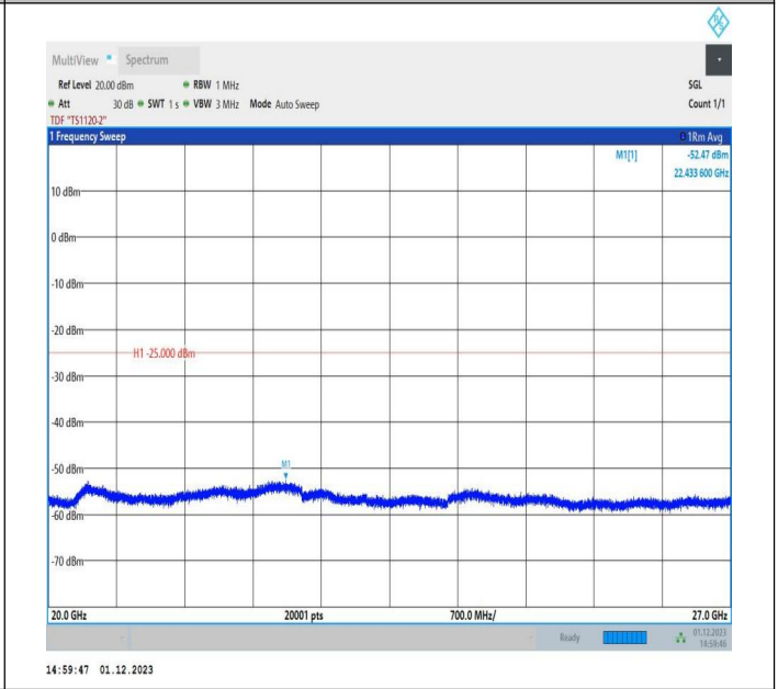
7-7-15MHz-10MHz-QPSK-QPSK-21051-21171-1RB#74-0RB# 0-20000~27000MHz-PASS
