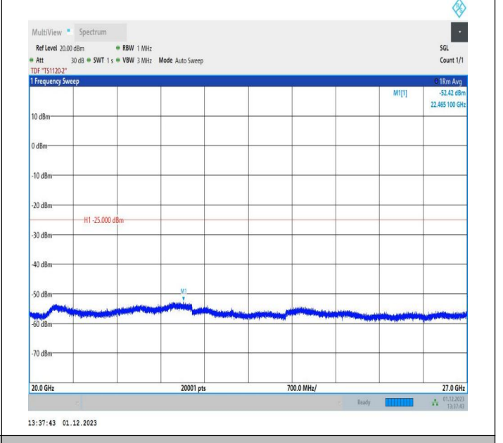
7-7-10MHz-20MHz-QPSK-QPSK-21206-21350-1RB#49-0RB# 0-20000~27000MHz-PASS
