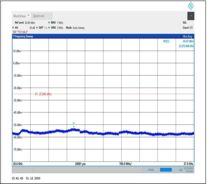
7-7-10MHz-20MHz-QPSK-QPSK-21206-21350-50RB#0-100R B#0-20000~27000MHz-PASS
