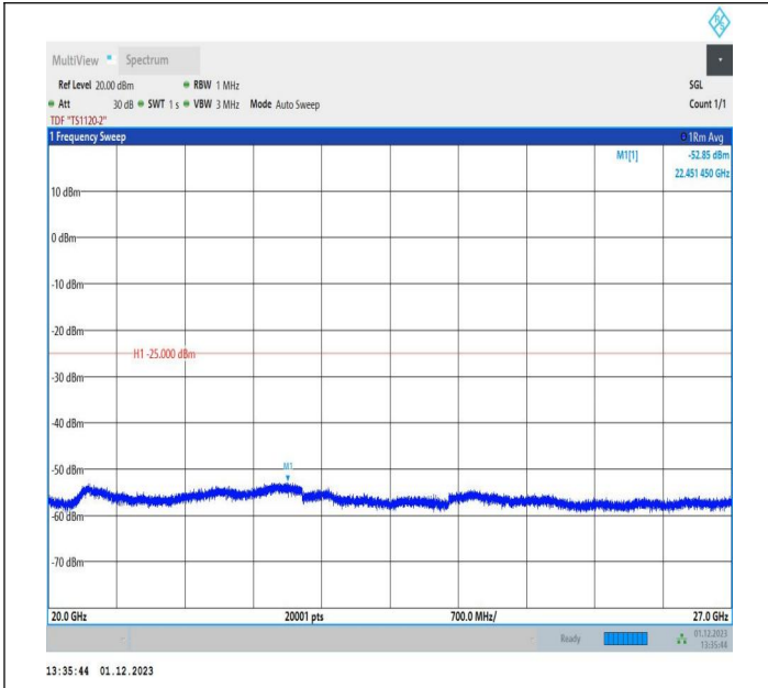
7-7-10MHz-20MHz-QPSK-QPSK-21206-21350-1RB#0-0RB#0 -20000~27000MHz-PASS
