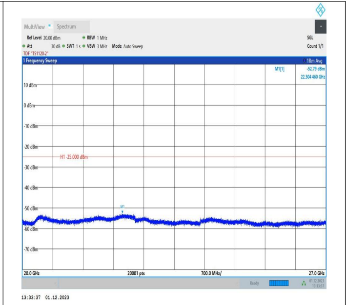
7-7-10MHz-20MHz-QPSK-QPSK-21006-21150-50RB#0-100R B#0-20000~27000MHz-PASS
