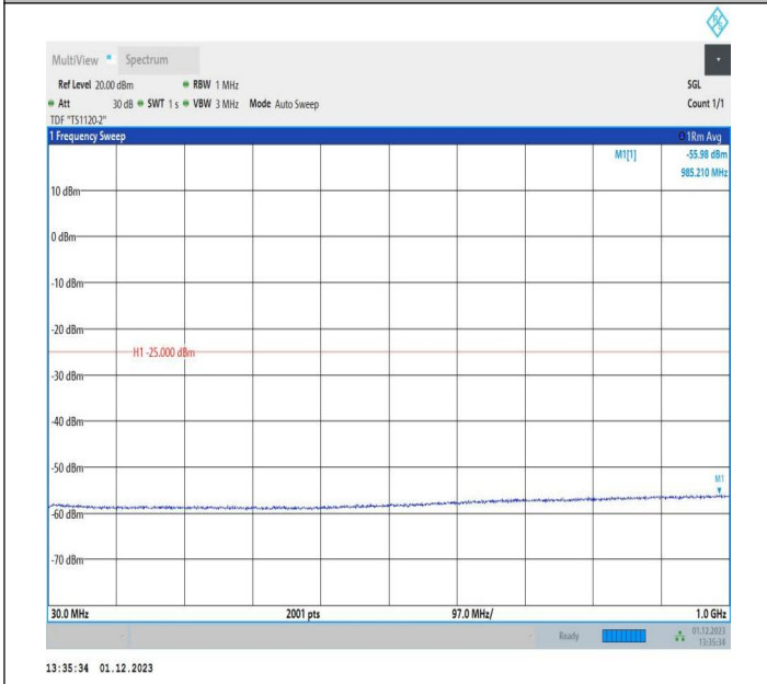
7-7-10MHz-20MHz-QPSK-QPSK-21206-21350-1RB#0-0RB#0 -30~1000MHz-PASS
