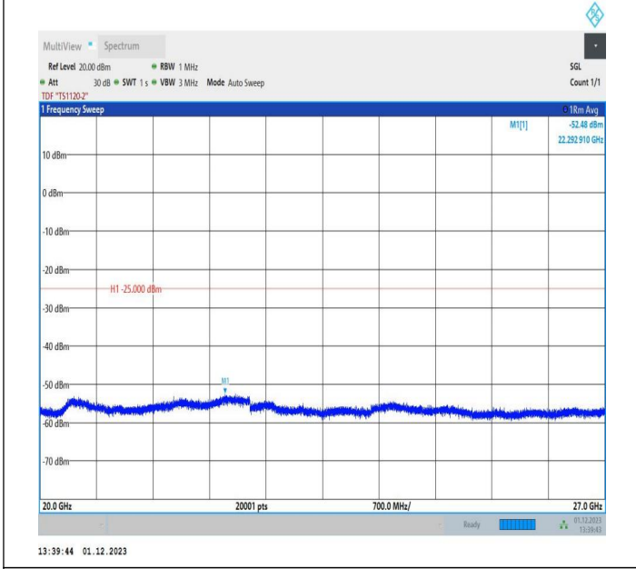
7-7-10MHz-20MHz-QPSK-QPSK-21206-21350-1RB#0-1RB#9 9-20000~27000MHz-PASS
