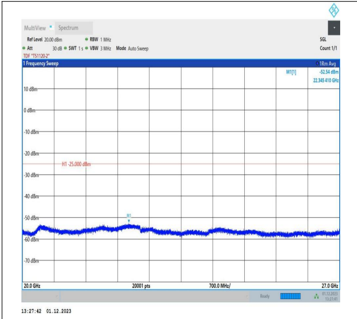
7-7-10MHz-20MHz-QPSK-QPSK-21006-21150-1RB#0-ORB#0-20000~27000MHz-PASS
