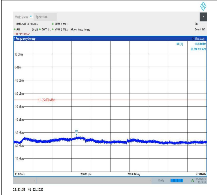
7-7-10MHz-20MHz-QPSK-QPSK-20805-20949-1RB#0-1RB#9 9-20000~27000MHz-PASS
