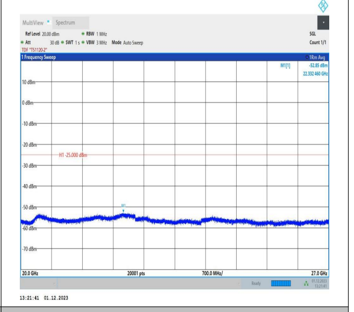
7-7-10MHz-20MHz-QPSK-QPSK-20805-20949-1RB#49-0RB# 0-20000~27000MHz-PASS
