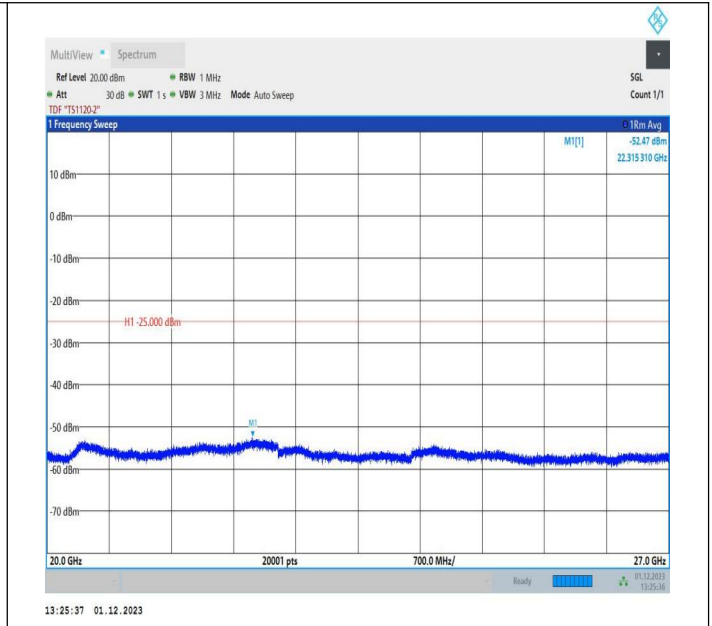
7-7-10MHz-20MHz-QPSK-QPSK-20805-20949-50RB#0-100R B#0-20000~27000MHz-PASS
