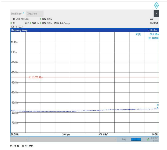
7-7-10MHz-20MHz-QPSK-QPSK-20805-20949-1RB#0-1RB#9 9-30~1000MHz-PASS
