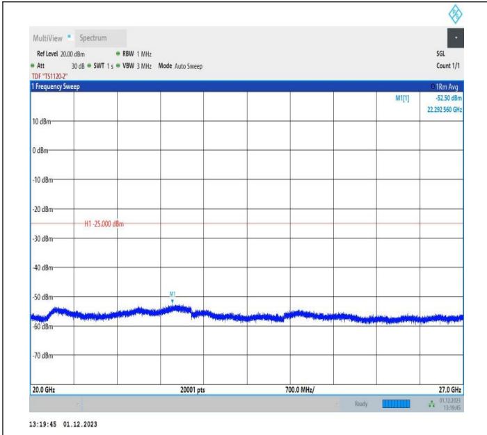
7-7-10MHz-20MHz-QPSK-QPSK-20805-20949-1RB#0-0RB#0 -20000~27000MHz-PASS
